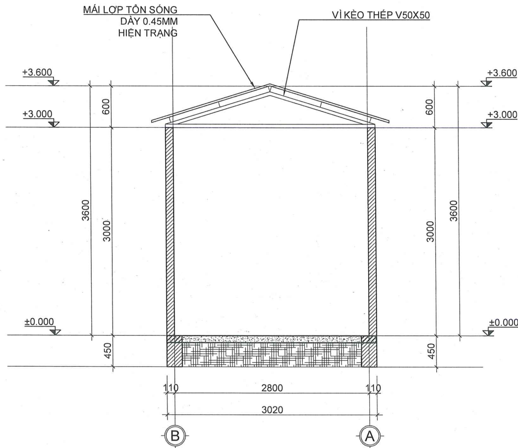
MẶT CẮT A-A HIỆN TRẠNG
