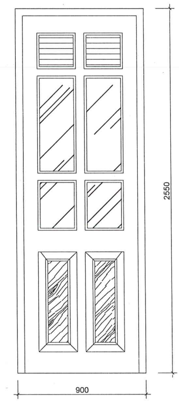
CỬA ĐI D2 CHUNG LOẠI: CỬA GỖ KÍNH KÍNH THƯỚC : 900X2550 SỐ LƯỢNG : 06 CỬA
