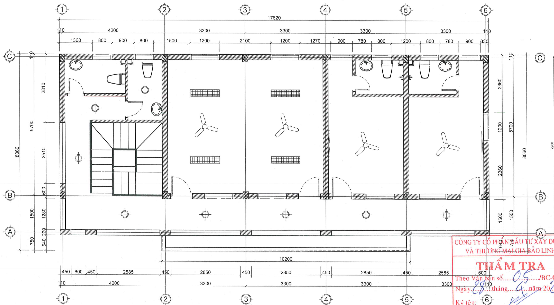
MẶT BẰNG TRẦN TẦNG 2 HIỆN TRẠNG
