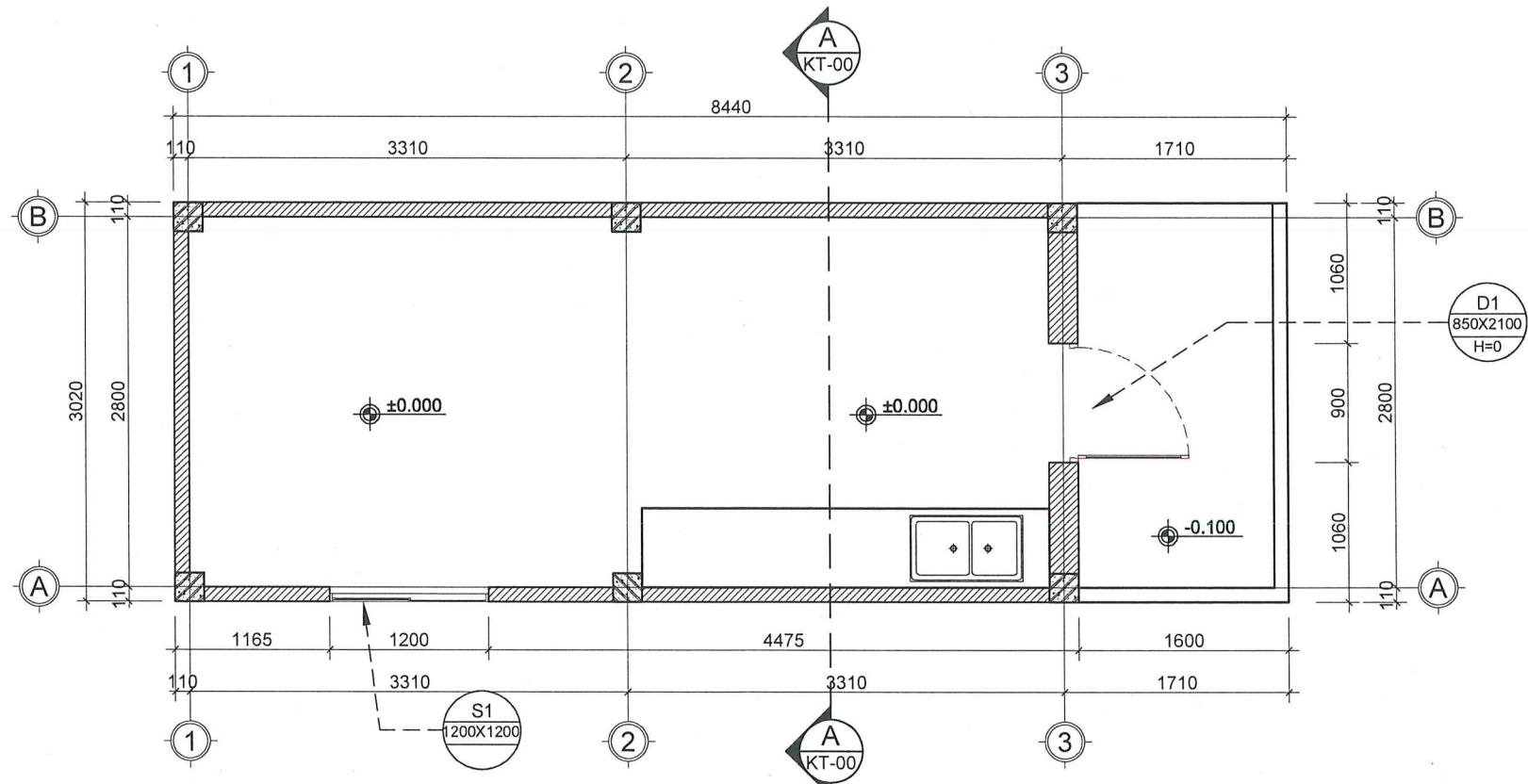
MẶT BẰNG KHU BẾP HIỆN TRẠNG
