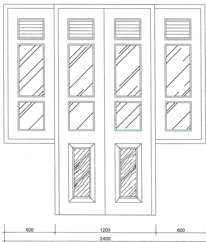
CỬA ĐI D1 CHUNG LOẠI: CỬA ĐI GỖ 2 CÁCH, KHUÔN ĐƠN 60X110, CẢNH DÂY 35, KÍNH 5LY, CÓ Ô FIX VÀ Ô CHỚP TRÊN KÍNH THƯỚC : 2400X2500 SỐ LƯỢNG : 04 CỬA
