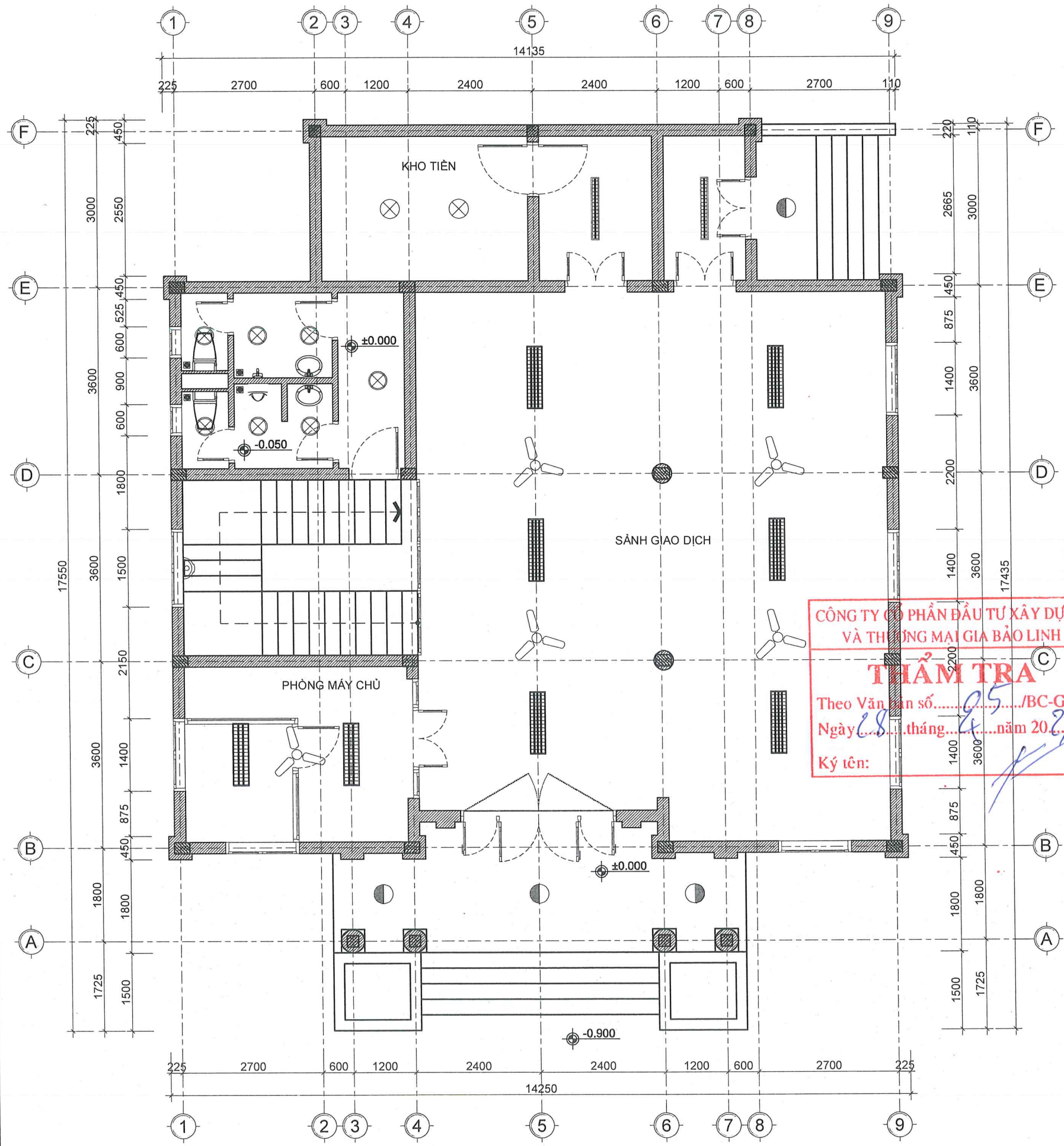
MẶT BẰNG HIỆN TRẠNG TRẦN TẦNG 1
