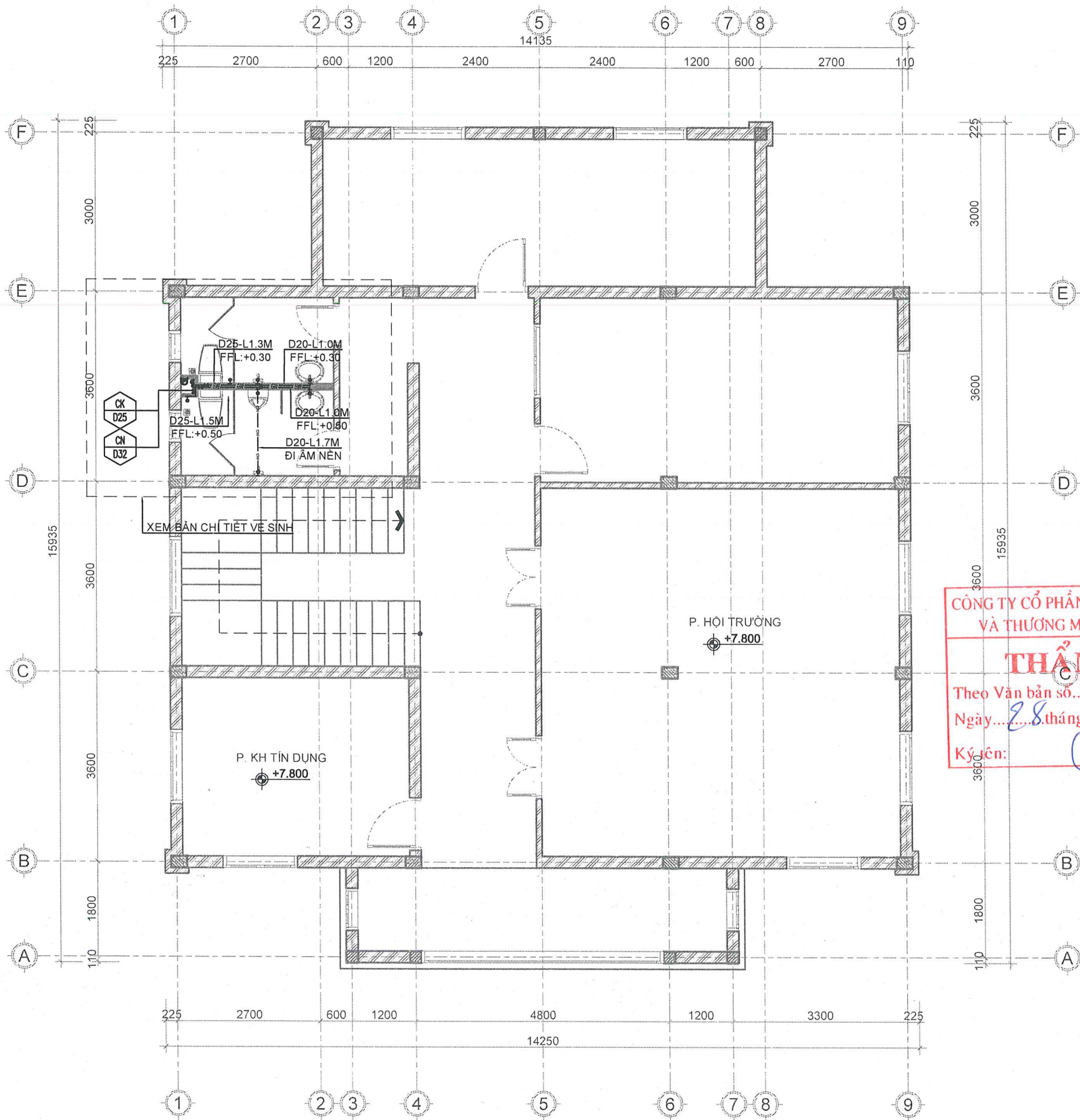
MẶT BẰNG CẤP NƯỚC CẢI TẠO TẦNG 3
