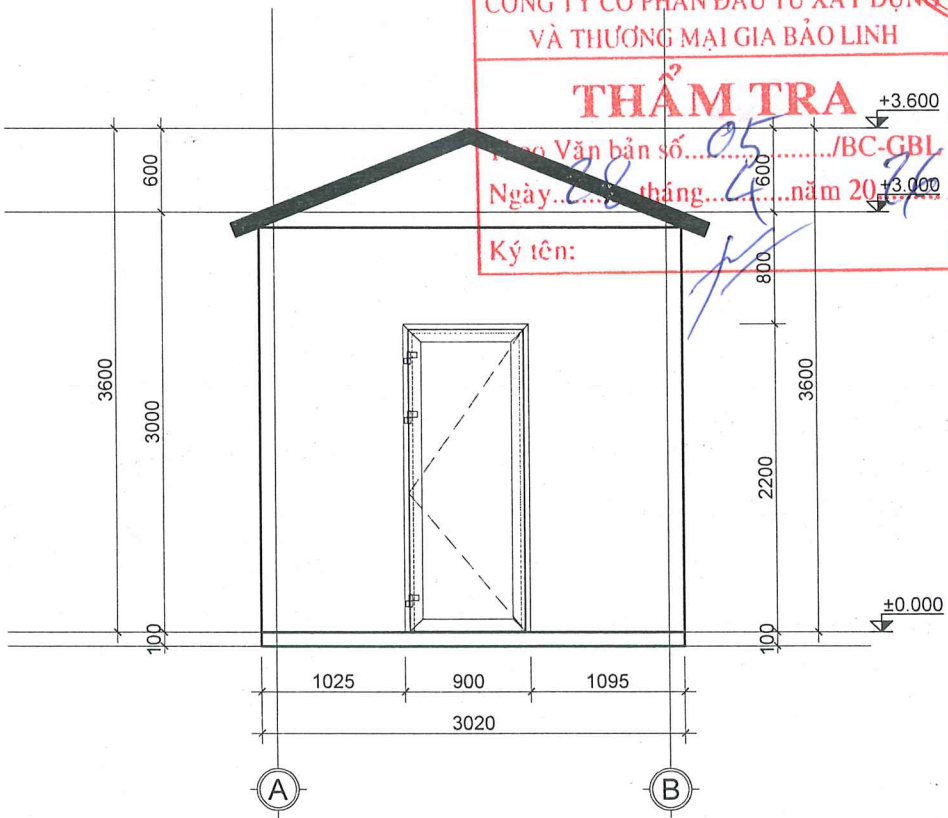
MẶT ĐỨNG TRỰC A-B CẢI TẠO
