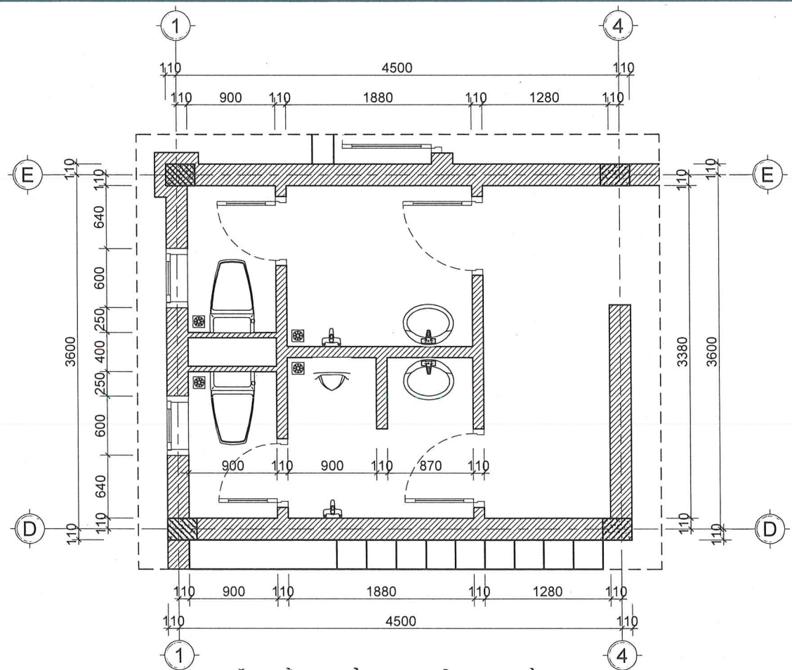
MẶT BẰNG CẢI TẠO VỆ SINH TẦNG 2
