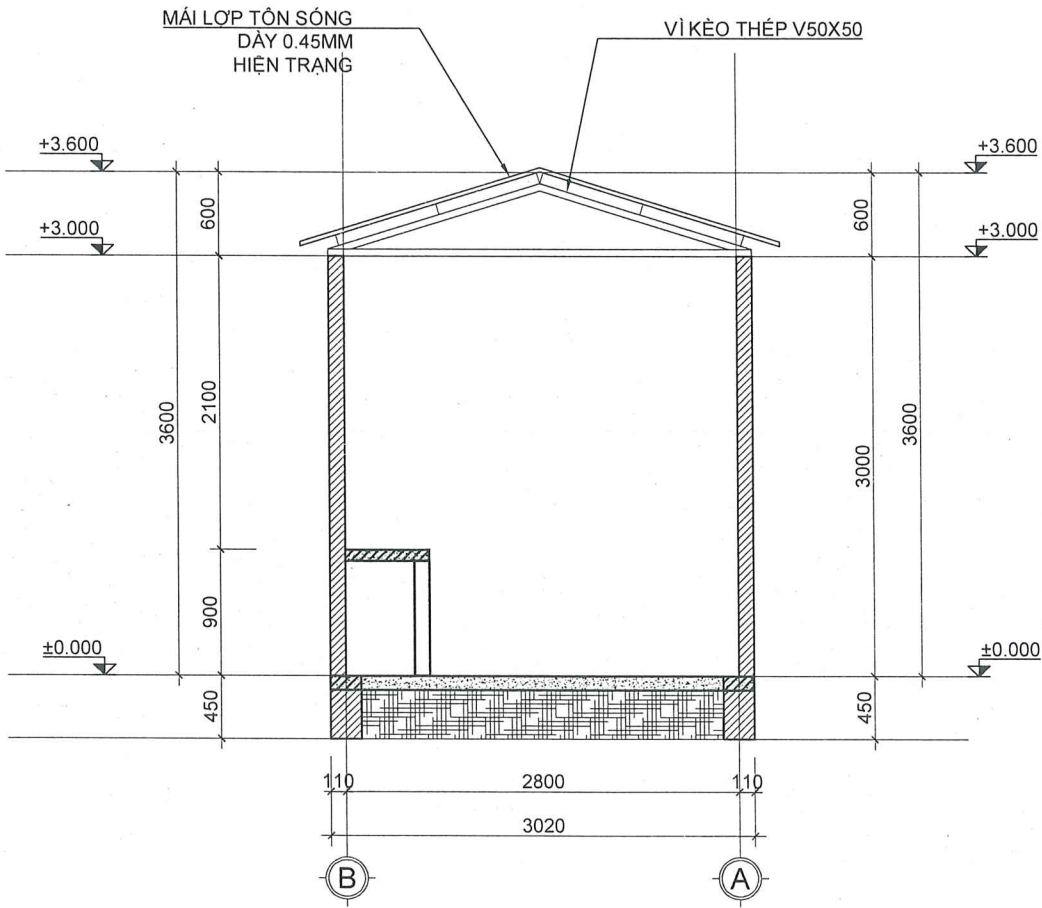
MẶT CẮT A-A CẢI TẠO
