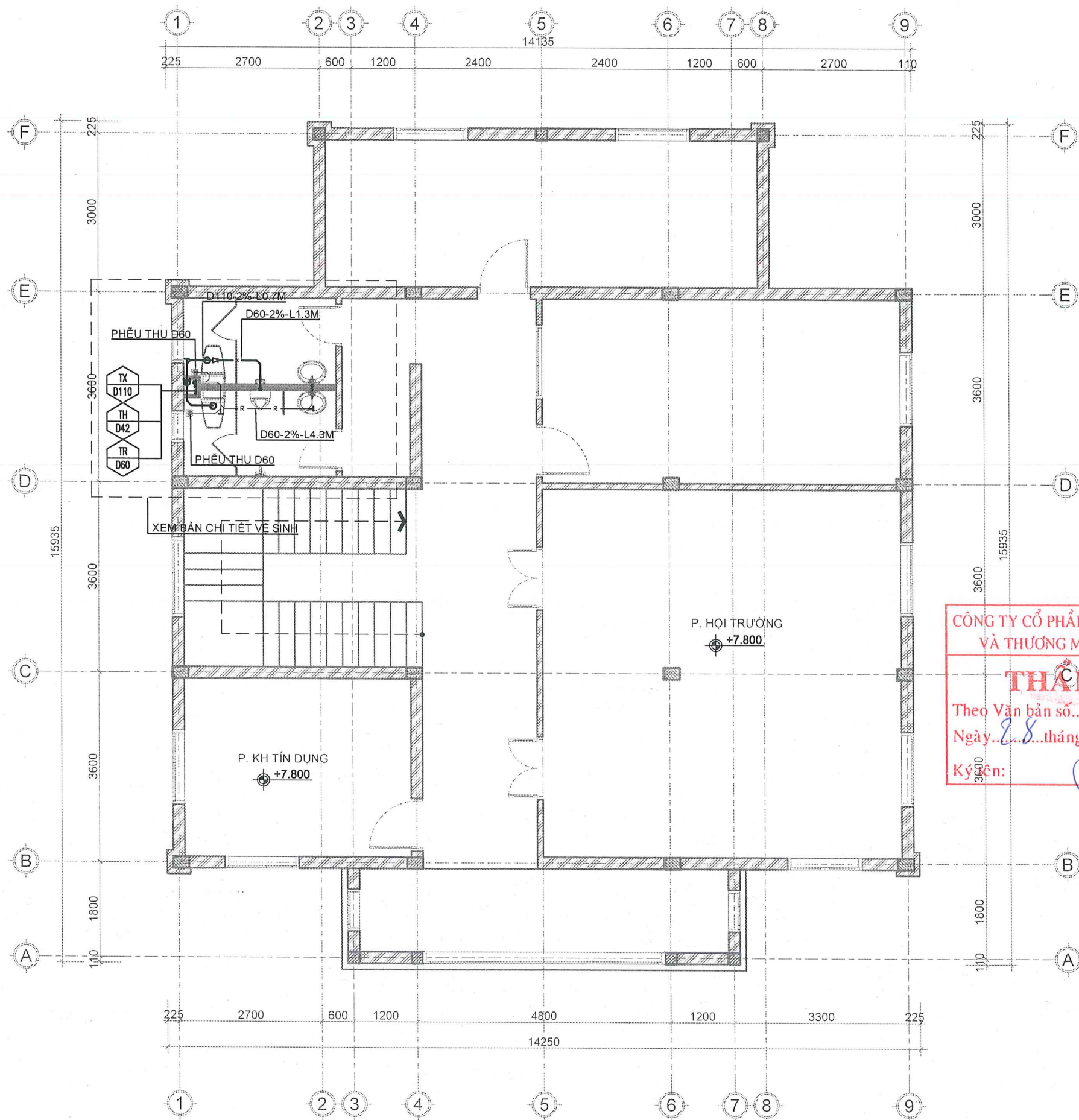
MẶT BẰNG THOÁT NƯỚC CẢI TẠO TẦNG 3
