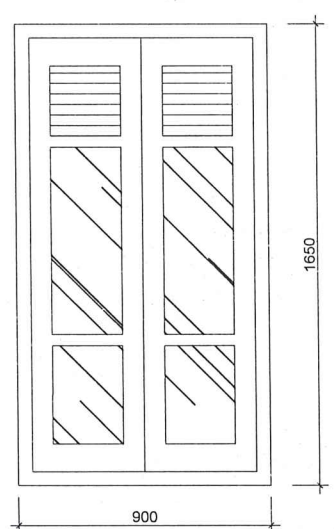
CỬA SỐ S2 CHUNG LOẠI: CỬA GỖ KÍNH KÍNH THƯỚC : 900x1650 MM SỐ LƯỢNG : 02 CỬA
