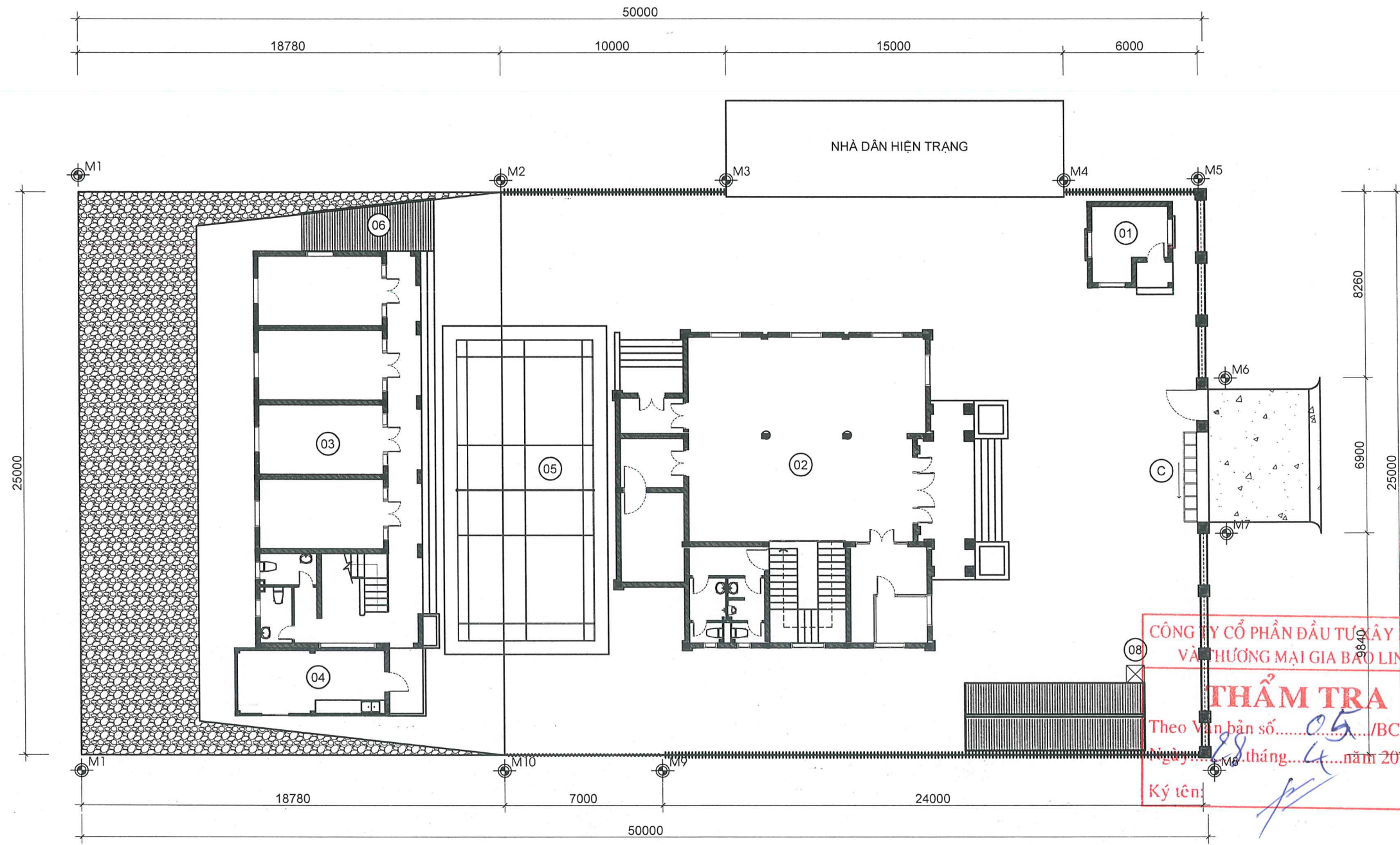
TỔNG MẶT BẰNG HIỆN TRẠNG
