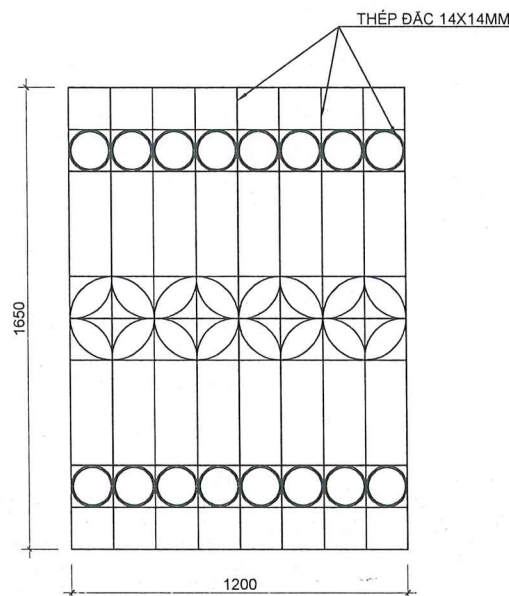
HOA SẮT CỬA SỐ S1 CHUNG LOẠI: THÉP ĐẮC KÍNH THƯỚC : 1200x1650 SỐ LƯỢNG : 12 CỬA
