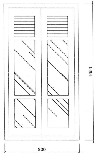
CỬA SỐ S2 CHUNG LOẠI: CỬA GỖ KÍNH KÍNH THƯỚC : 900x1650 SỐ LƯỢNG : 02 CỬA
