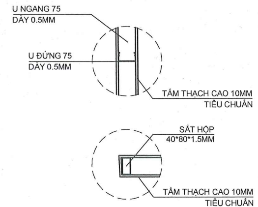
CHI TIẾT VÁCH
