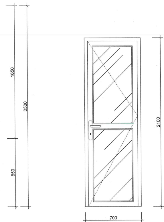
CỬA ĐI DW CHUNG LOẠI: CỬA NHÔM KÍNH KÍNH THƯỚC : 700X2100 SỐ LƯỢNG : 06 CỬA
