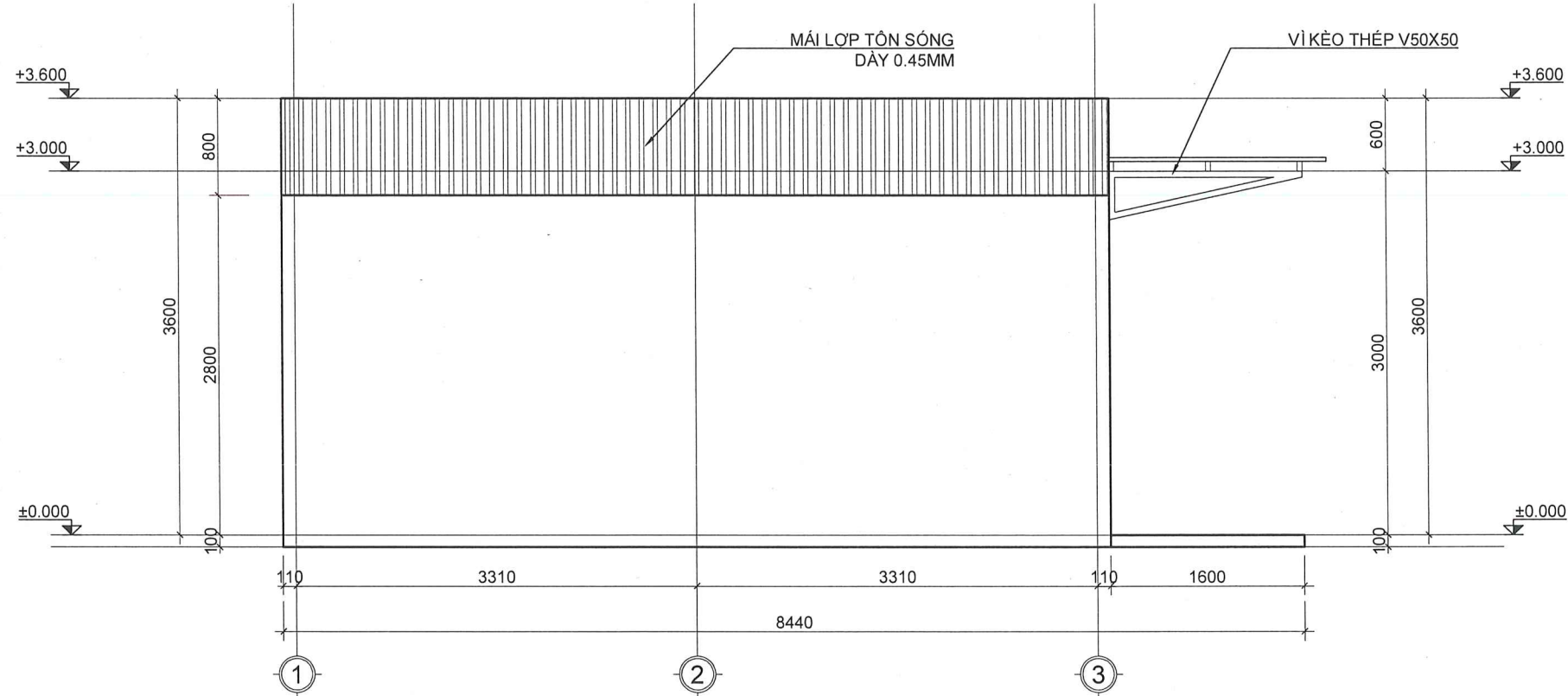
MẶT ĐỨNG TRỤC 1-3 KHU BẾP HIỆN TRẠNG
