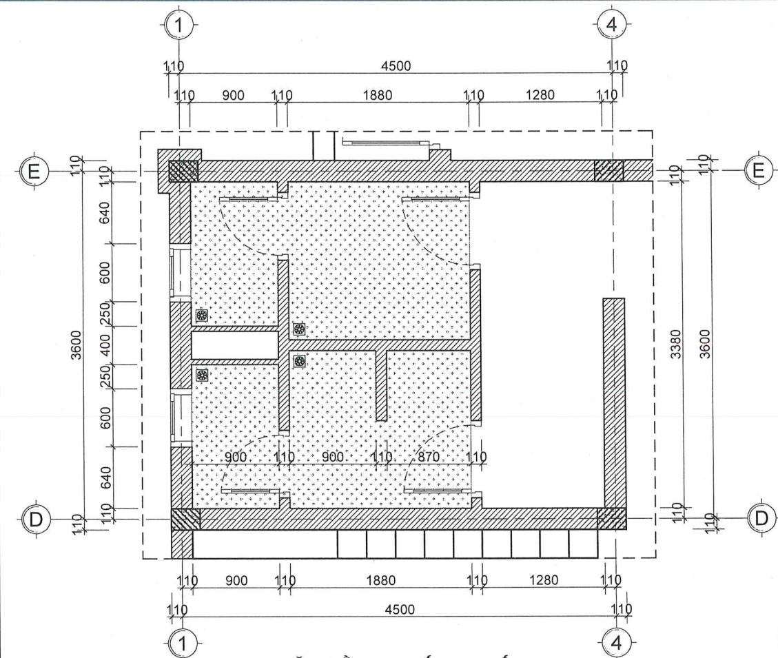
MẶT BẰNG CHỐNG THẨM
