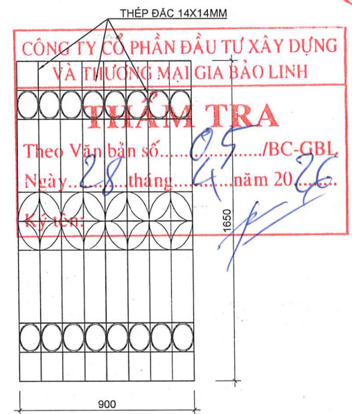
HOA SẮT CỬA SỐ S2 CHUNG LOẠI: THÉP ĐẶC KÍNH THƯỚC : 900x1650 MM SỐ LƯỢNG : 02 CỬA
