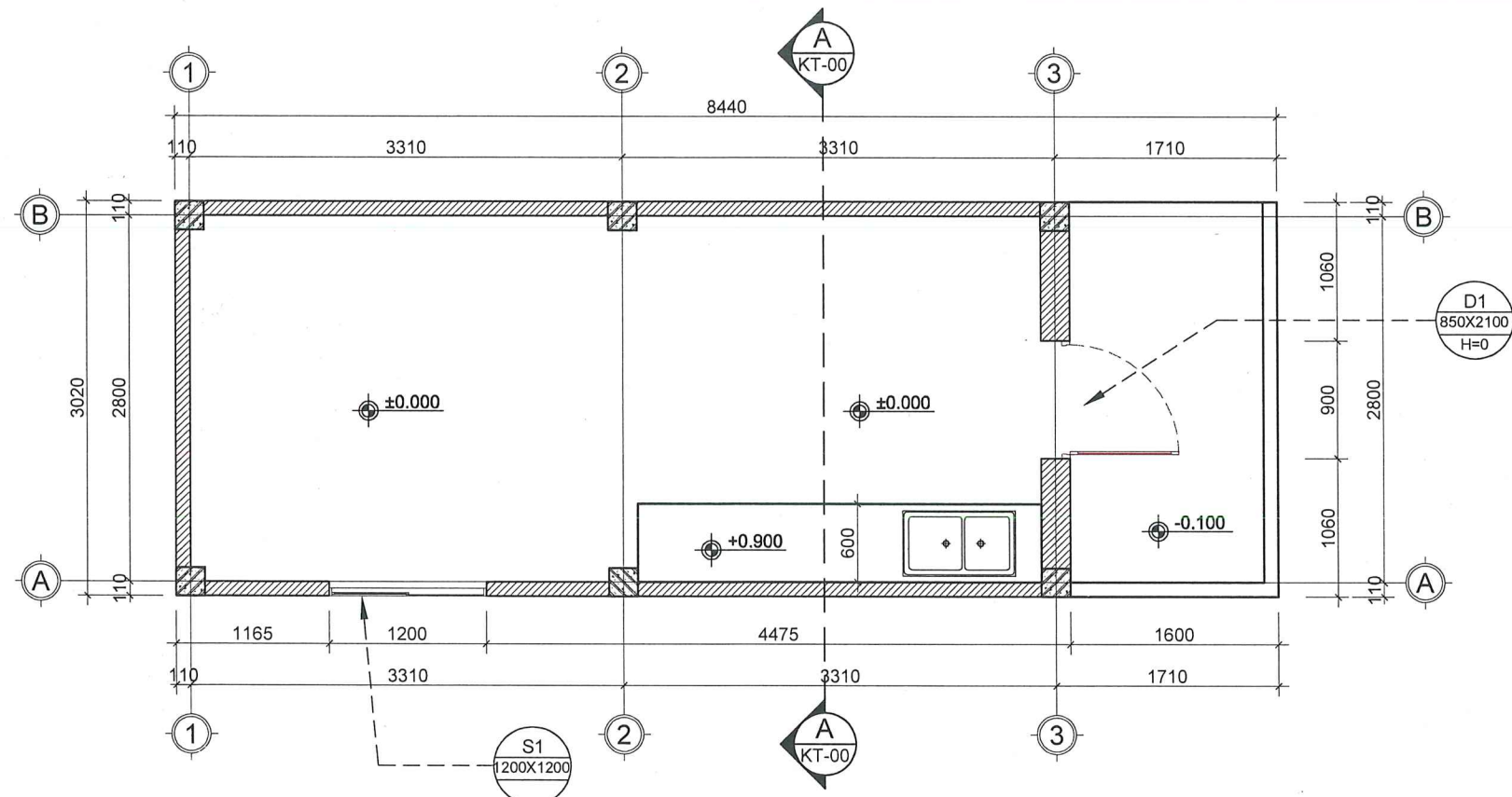
MẶT BẰNG KHU BẾP CẢI TẠO
