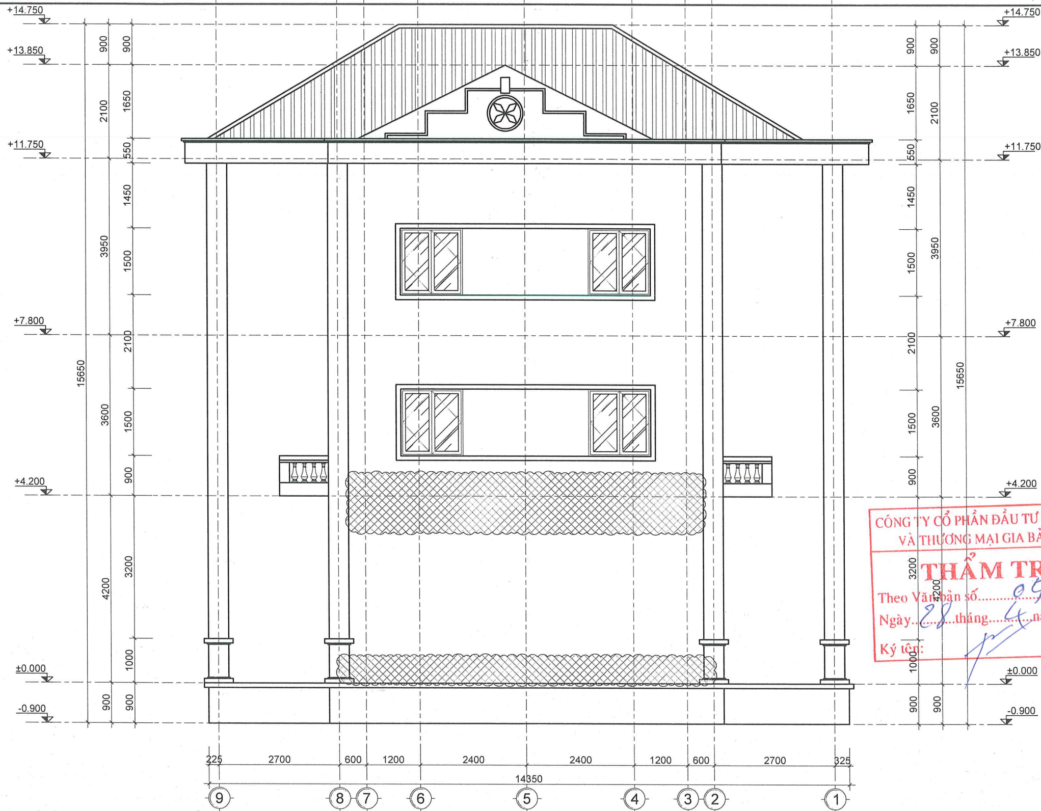
MẶT ĐỨNG CẢI TẠO TRỤC 9-1
