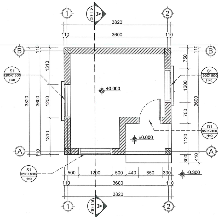
MẶT BẰNG NHÀ BẢO VỆ
