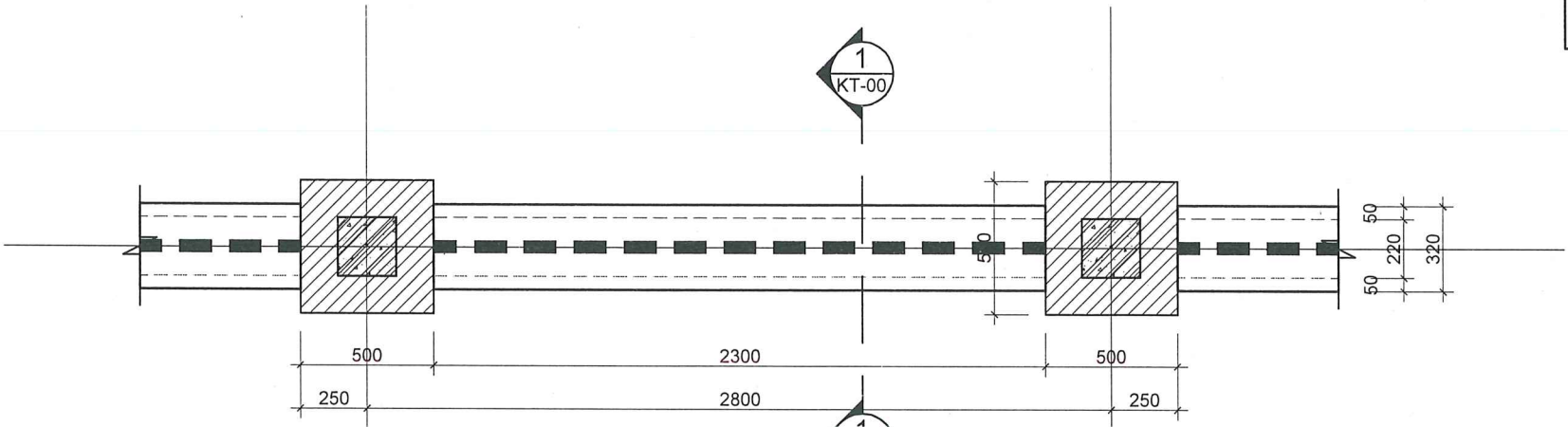
MẶT BẰNG ĐIỆN HÌNH TƯỜNG RÀO THOÁNG HIỆN TRẠNG TỔNG CHIỀU DÀI: 18.24M SỐ LƯỢNG TRỤ: 07
