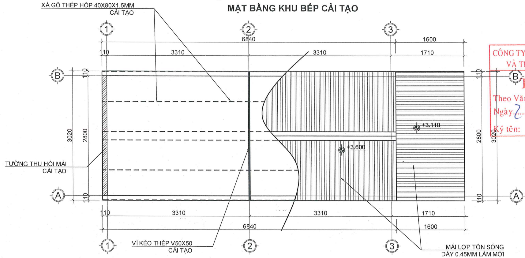
MẶT BẰNG MÁI CẢI TẠO
