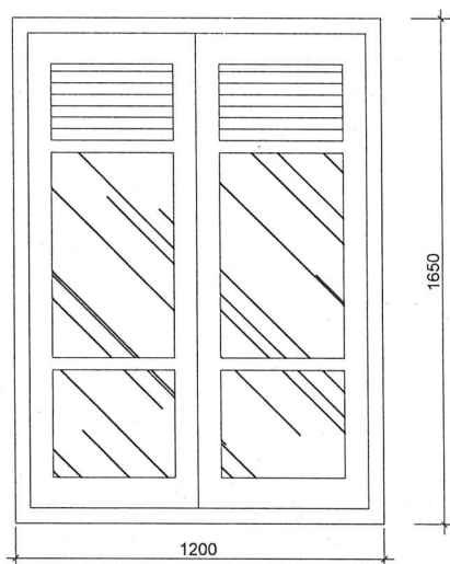
CỬA SỐ S1 CHUNG LOẠI: CỬA GỖ KÍNH KÍNH THƯỚC : 1200x1650 SỐ LƯỢNG : 12 CỬA
