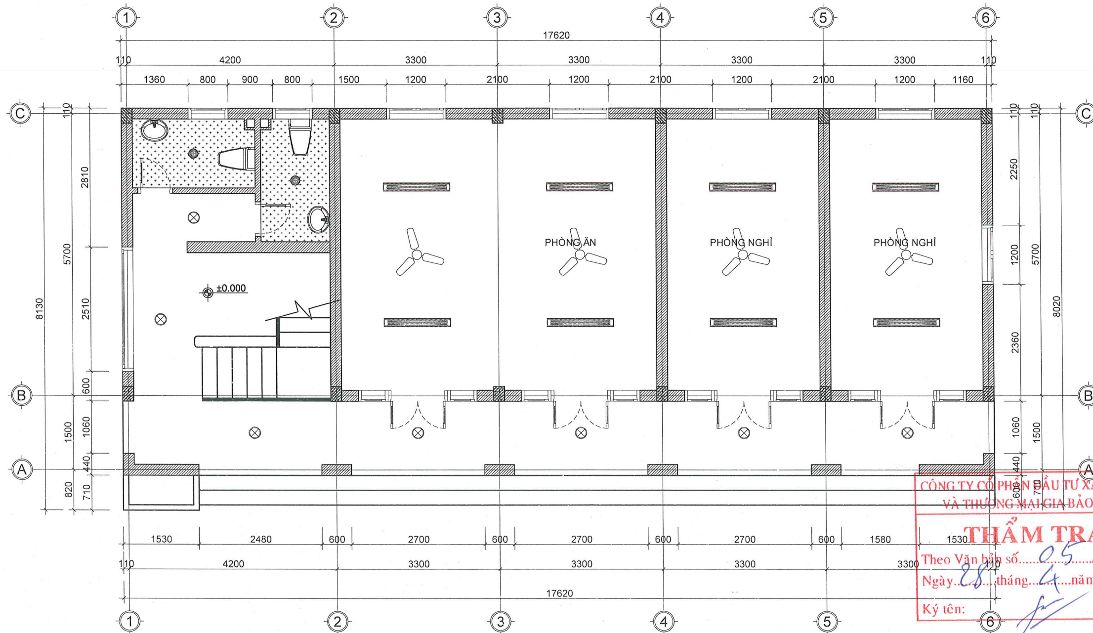
MẶT BẰNG TRẦN TẦNG 1 CẢI TẠO
