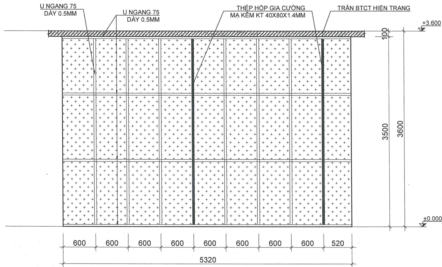
MẶT ĐỨNG VÁCH THẠCH CAO
