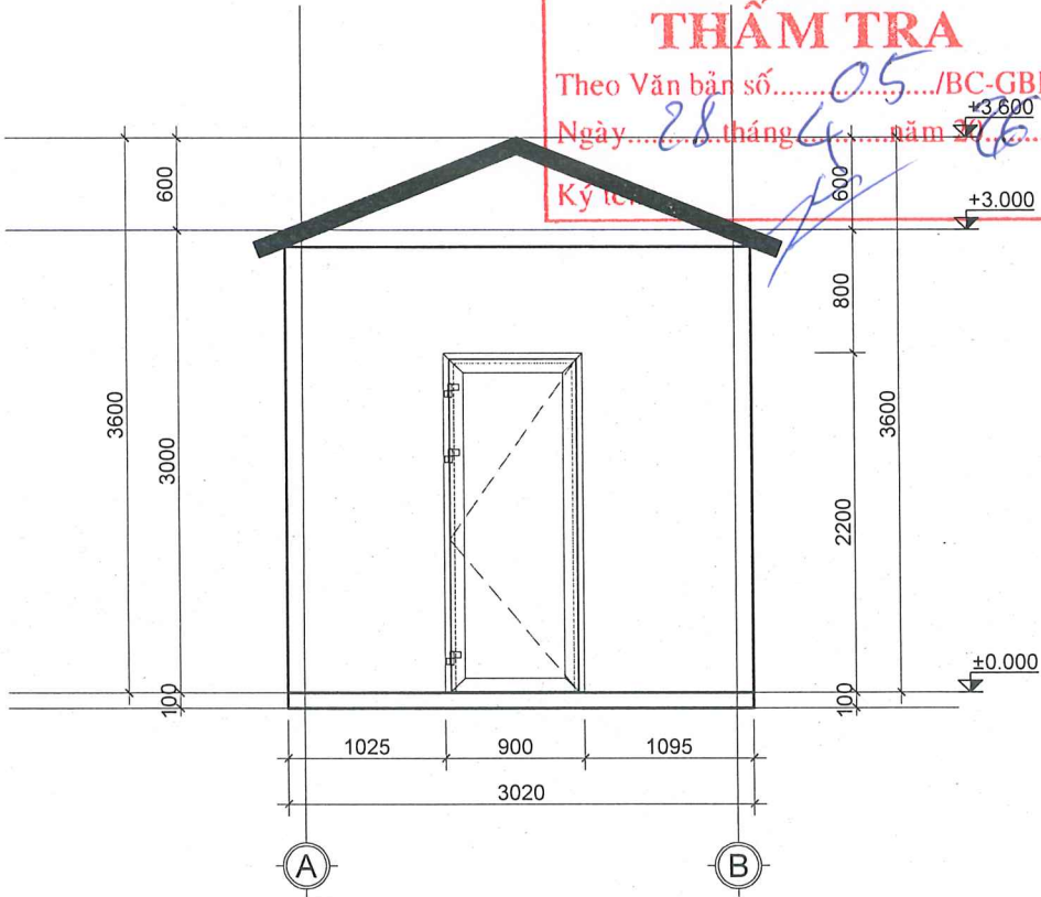
MẶT ĐỨNG TRỤC A-B HIỆN TRẠNG
