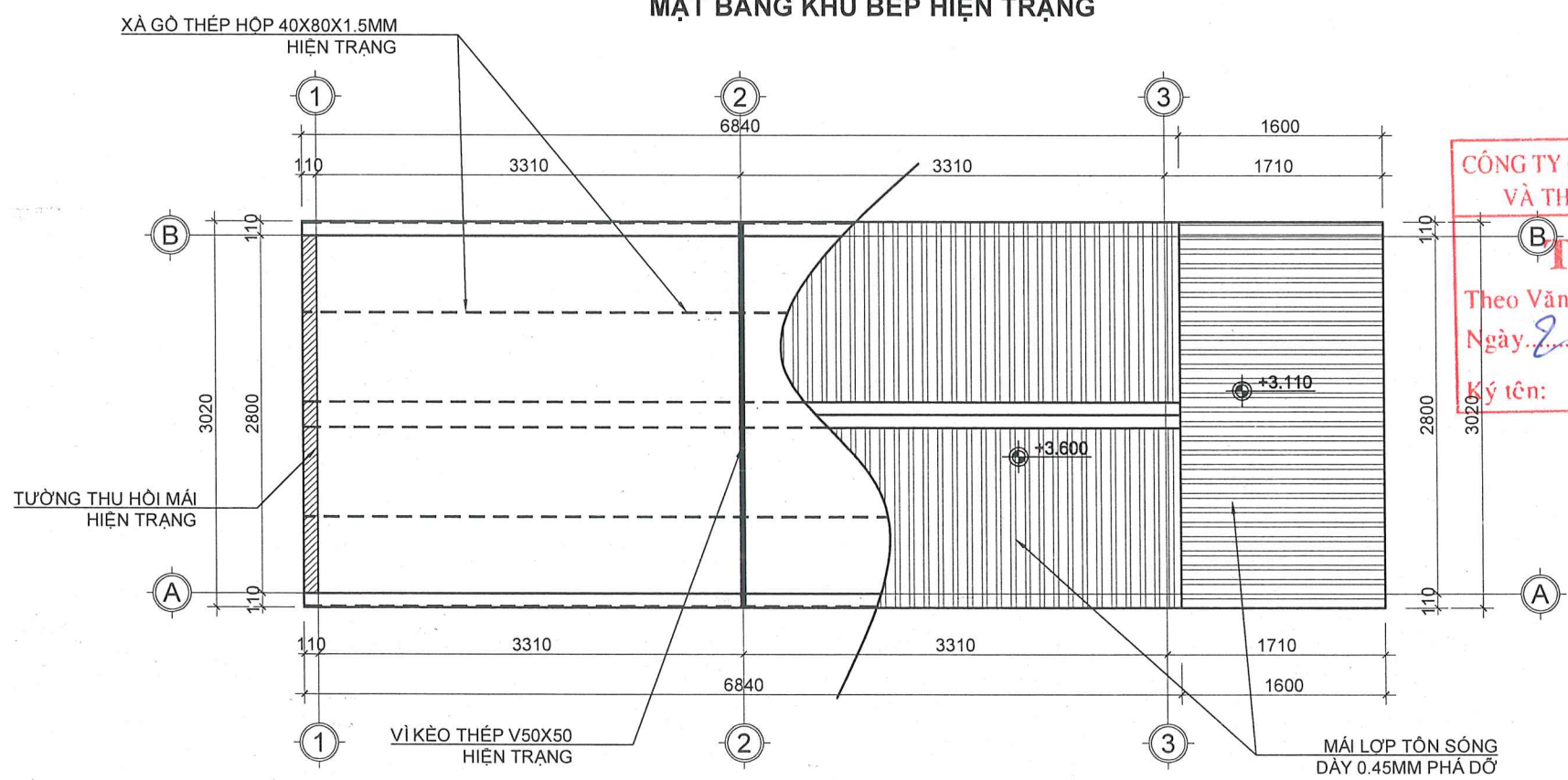
MẶT BẰNG MÁI HIỆN TRẠNG
