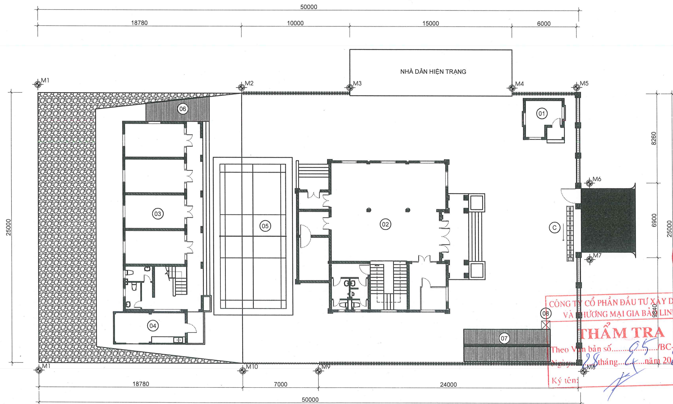
TỔNG MẶT BẰNG CẢI TẠO
