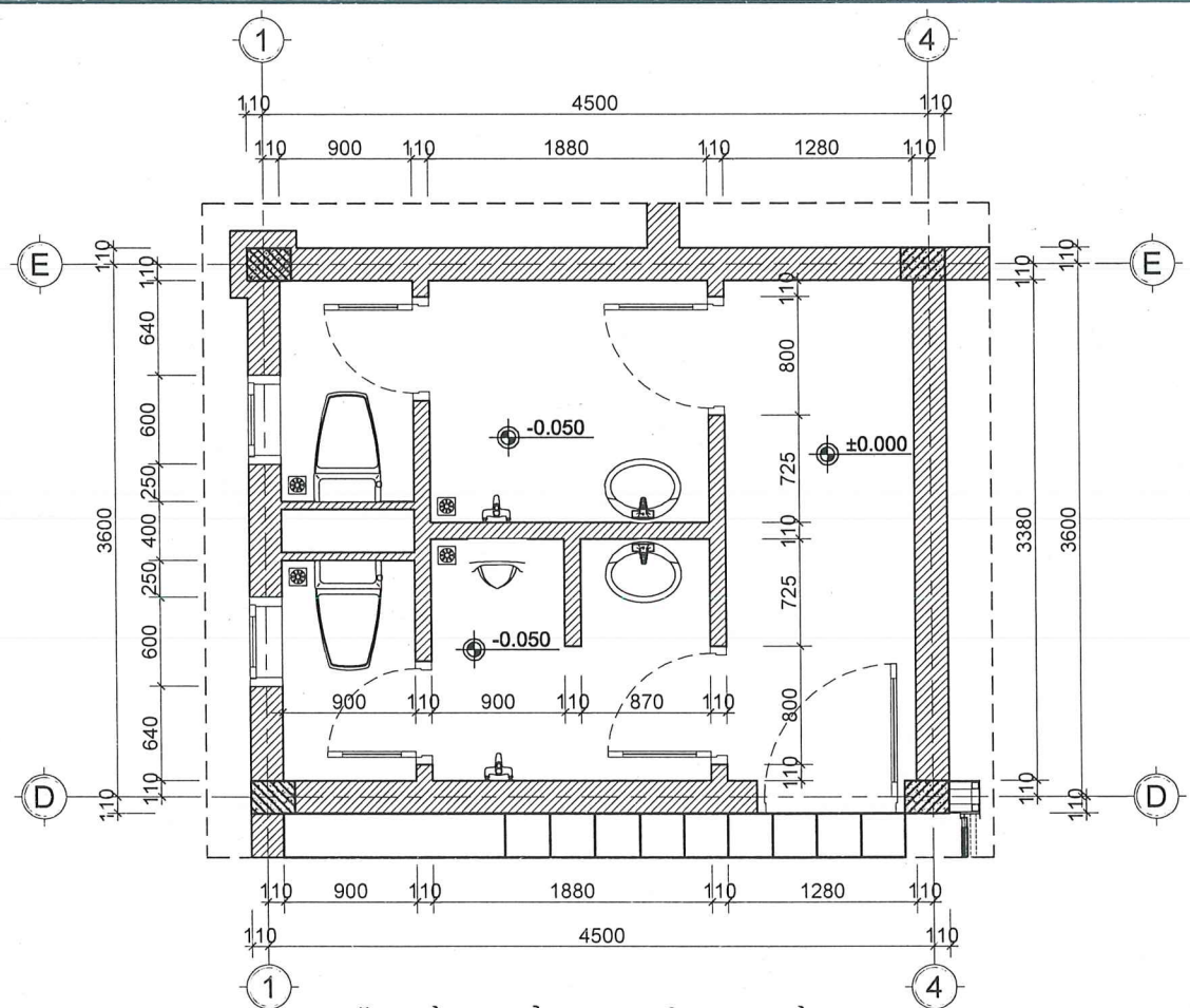
MẶT BẰNG CẢI TẠO VỆ SINH TẦNG 1
