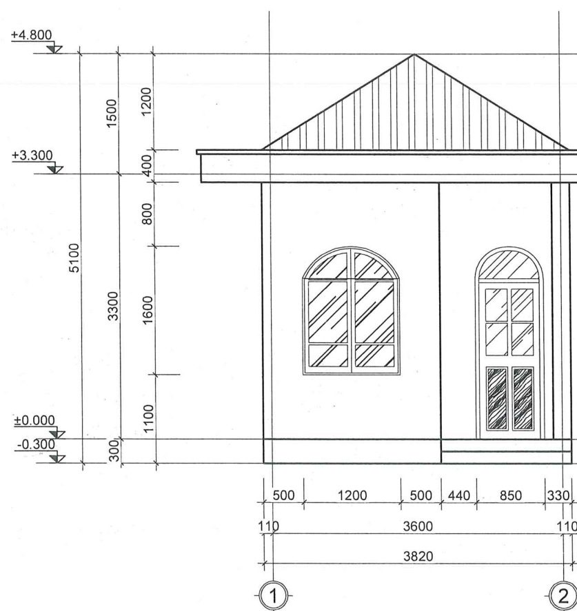
MẶT ĐỨNG TRỰC 1-2
