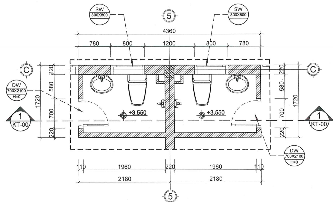
MẶT BẰNG WC HIỆN TRẠNG TẦNG 2
