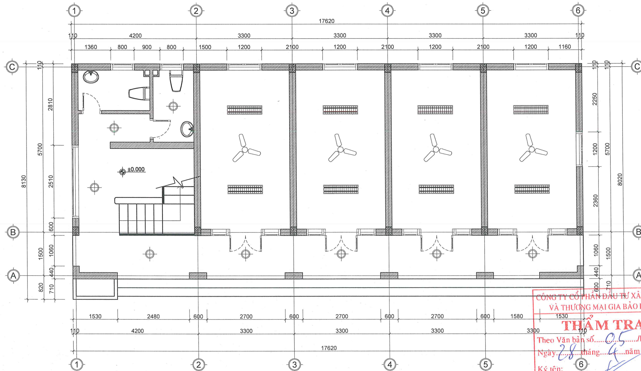
MẶT BẰNG TRẦN TẦNG 1 HIỆN TRẠNG
