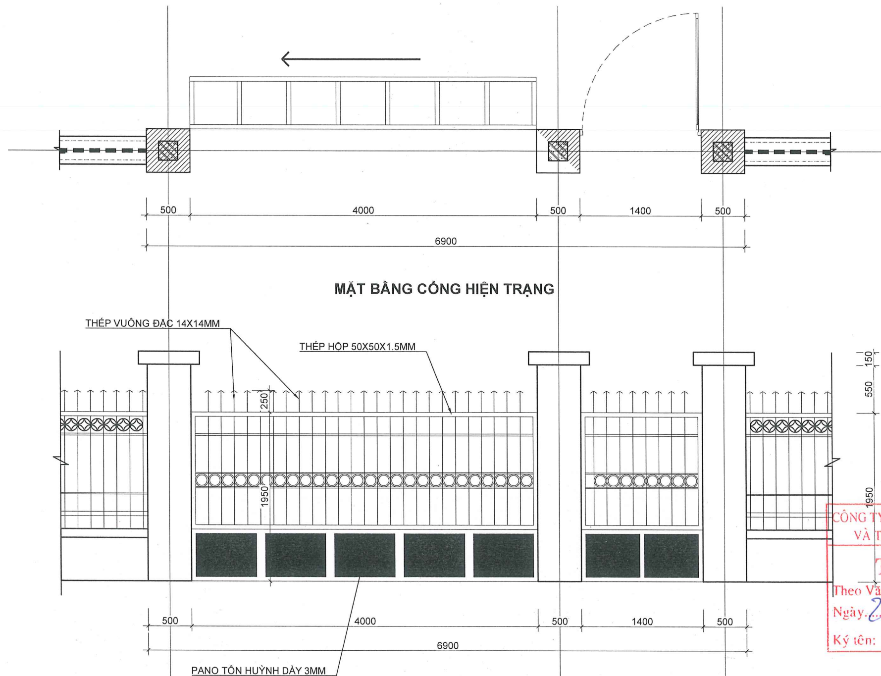
MẶT ĐỨNG CÔNG HIỆN TRẠNG
