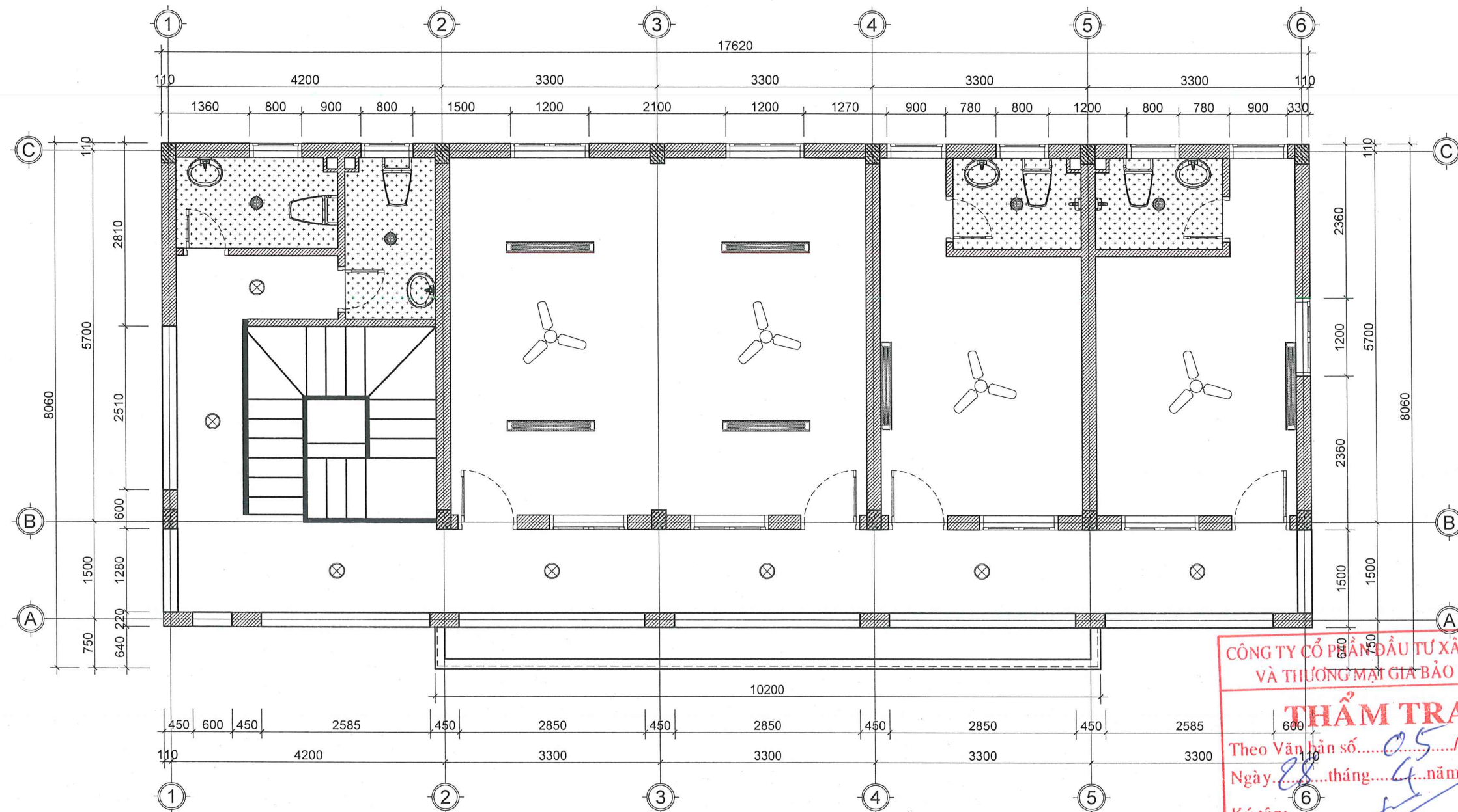
MẶT BẰNG TRẦN TẦNG 2 CẢI TẠO
