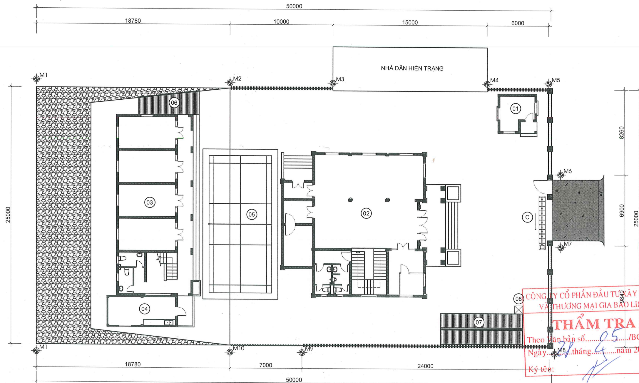
TỔNG MẶT BẰNG SÂN ĐƯỜNG CẢI TẠO
