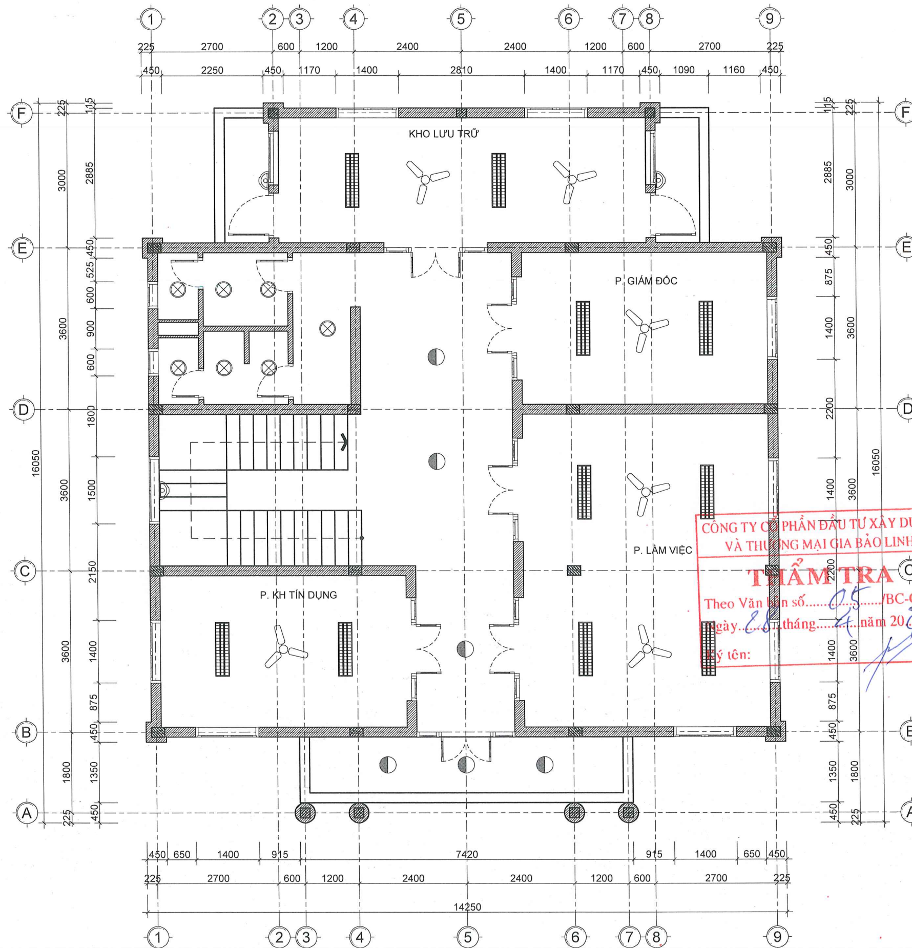
MẶT BẰNG HIỆN TRẠNG TRẦN TẦNG 2
