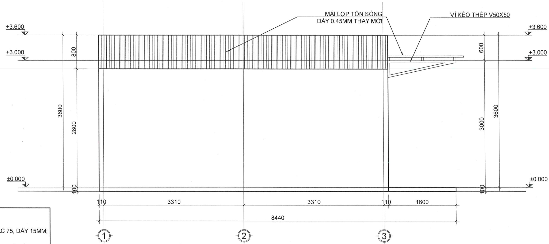
MẶT ĐỨNG TRỰC 1-3 KHU BẾP CẢI TẠO
