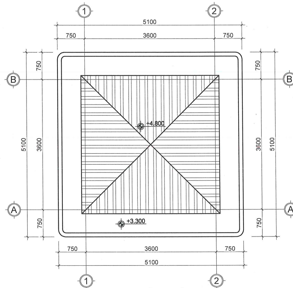
MẶT BẰNG MÁI
