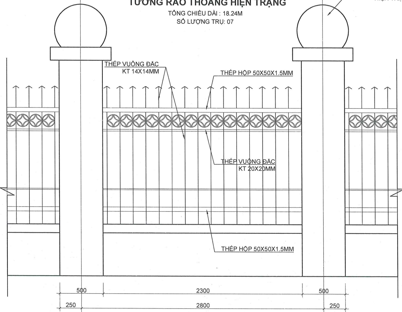
MẶT ĐỨNG ĐIỆN HÌNH TƯỜNG RÀO THOÁNG HIỆN TRẠNG TỔNG CHIỀU DÀI: 18.24M SỐ LƯỢNG TRỤ: 07
