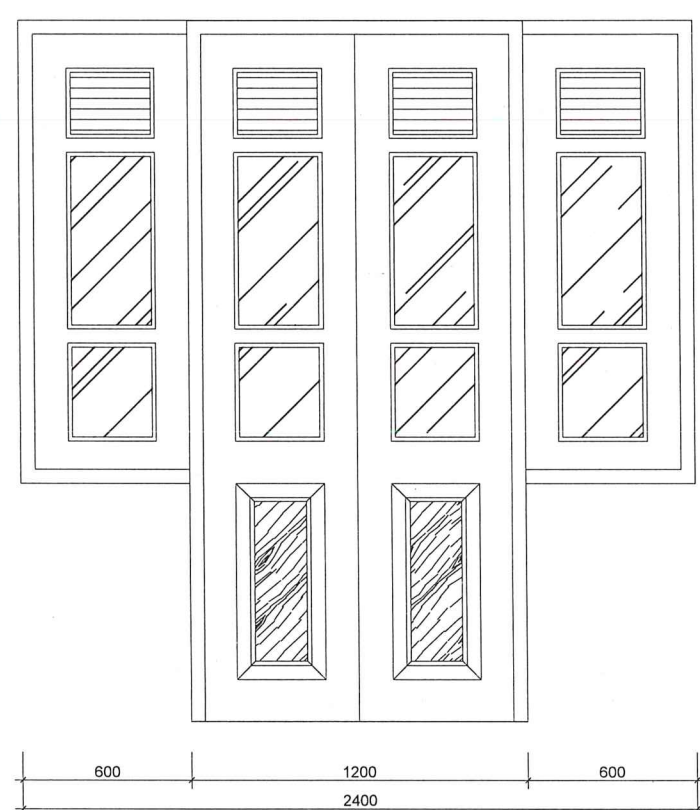
CỬA ĐI D1 CHUNG LOẠI: CỬA ĐI GỖ 2 CÁNH, KHUÔN ĐƠN 60X110, CÁNH DÂY 35, KÍNH 5LY, CÓ Ô FIX VÀ Ô CHỚP TRÊN KÍNH THƯỚC : 2400X2500 SỐ LƯỢNG : 04 CỬA
