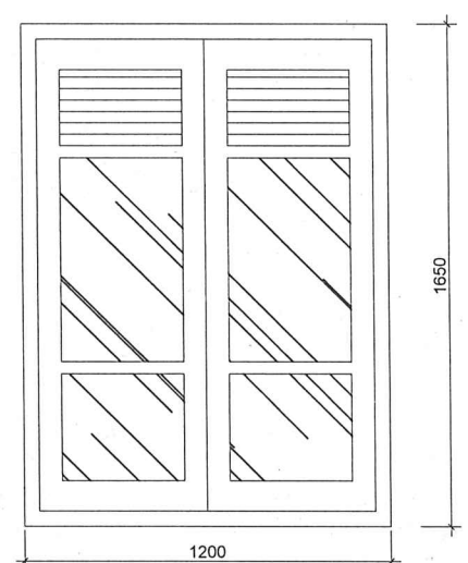
CỬA SỐ S1 CHUNG LOẠI: CỬA GỖ KÍNH KÍNH THƯỚC : 1200x1650 SỐ LƯỢNG : 12 CỬA
