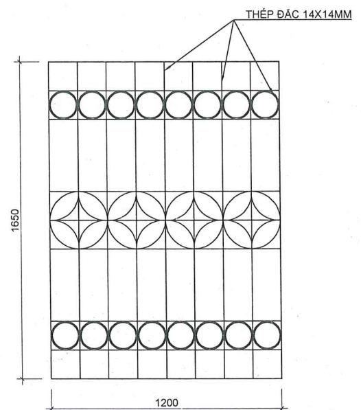
HOA SẮT CỬA SỐ S1 CHUNG LOẠI: THÉP ĐẶC KÍNH THƯỚC : 1200x1650 SỐ LƯỢNG : 12 CỬA
