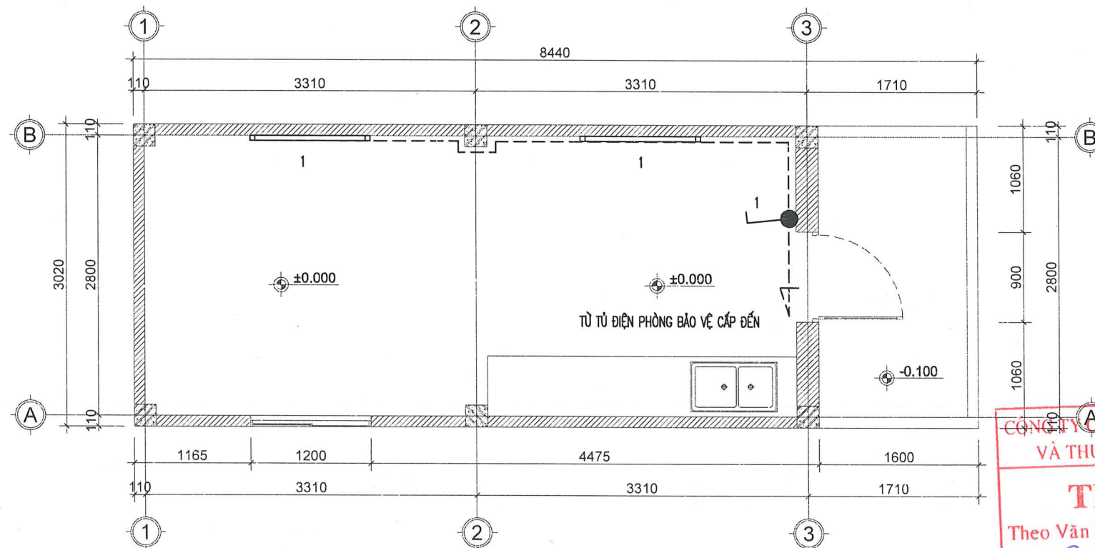
MẶT BẰNG CẤP ĐIỆN KHU BẾP
