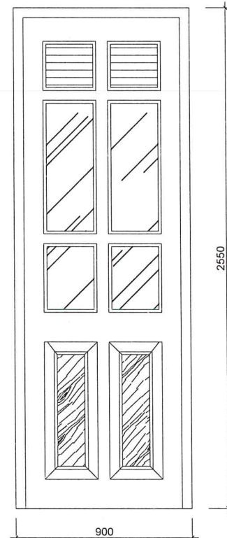
CỬA ĐI D2 CHUNG LOẠI: CỬA GỖ KÍNH KÍNH THƯỚC : 900X2550 SỐ LƯỢNG : 06 CỬA
