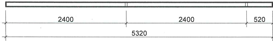
MẶT BẰNG VÁCH THẠCH CAO
