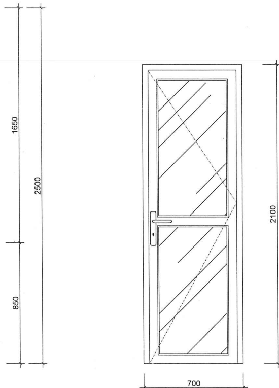
CỬA ĐI DW CHUNG LOẠI: CỬA NHÔM KÍNH KÍNH THƯỚC : 700X2100 SỐ LƯỢNG : 06 CỬA
