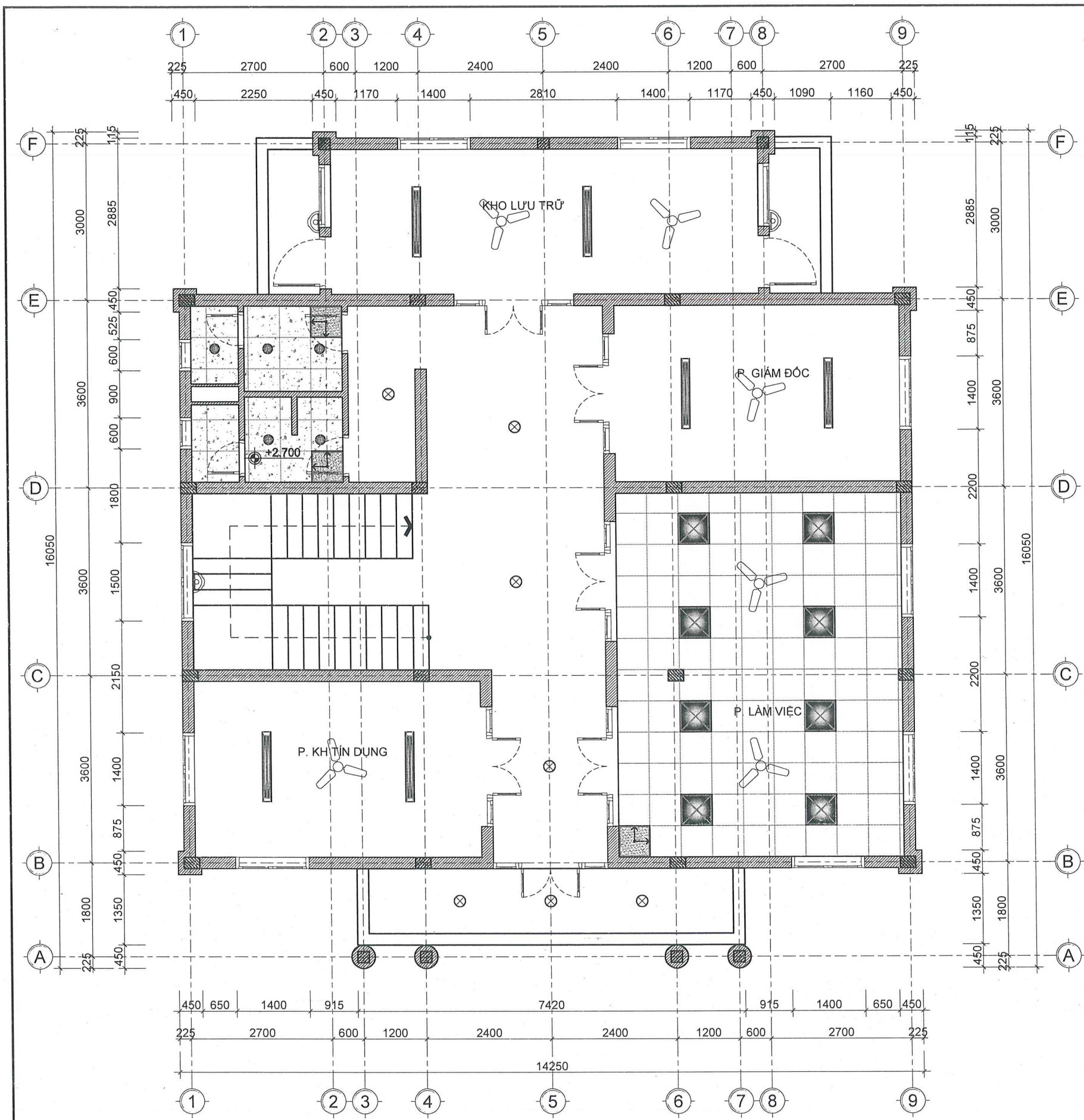
MẶT BẰNG CẢI TẠO TRẦN, ĐÈN TẦNG 2
