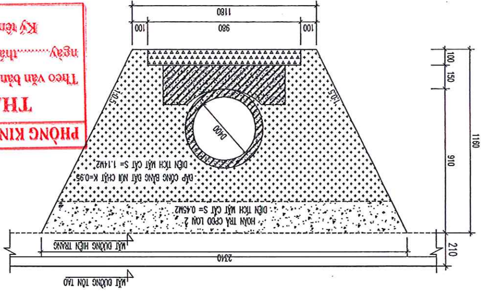
MẶT CẮT CỖNG D400
