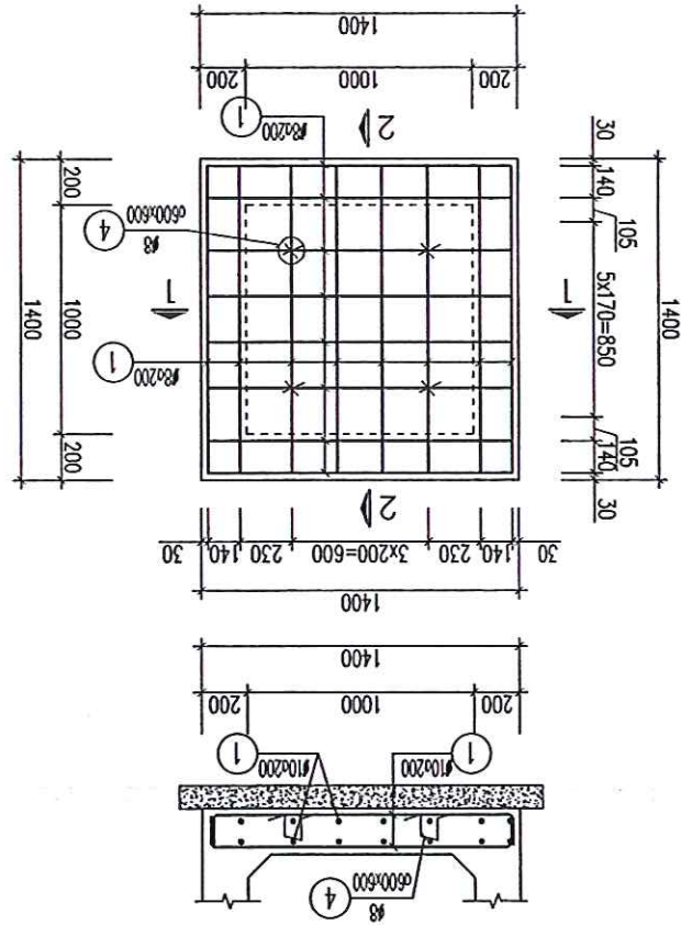
MẶT BẰNG THẺ DÂY
