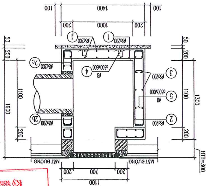
CHI TIẾT HỒ GÁ LOẠI 1 MẶT CẮT 1 - 1
