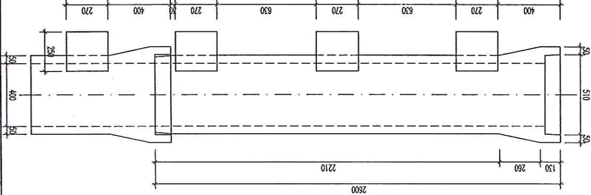
CHI TIẾT CÔNG - BỐ TRÍ DỆ CỒNG D400
