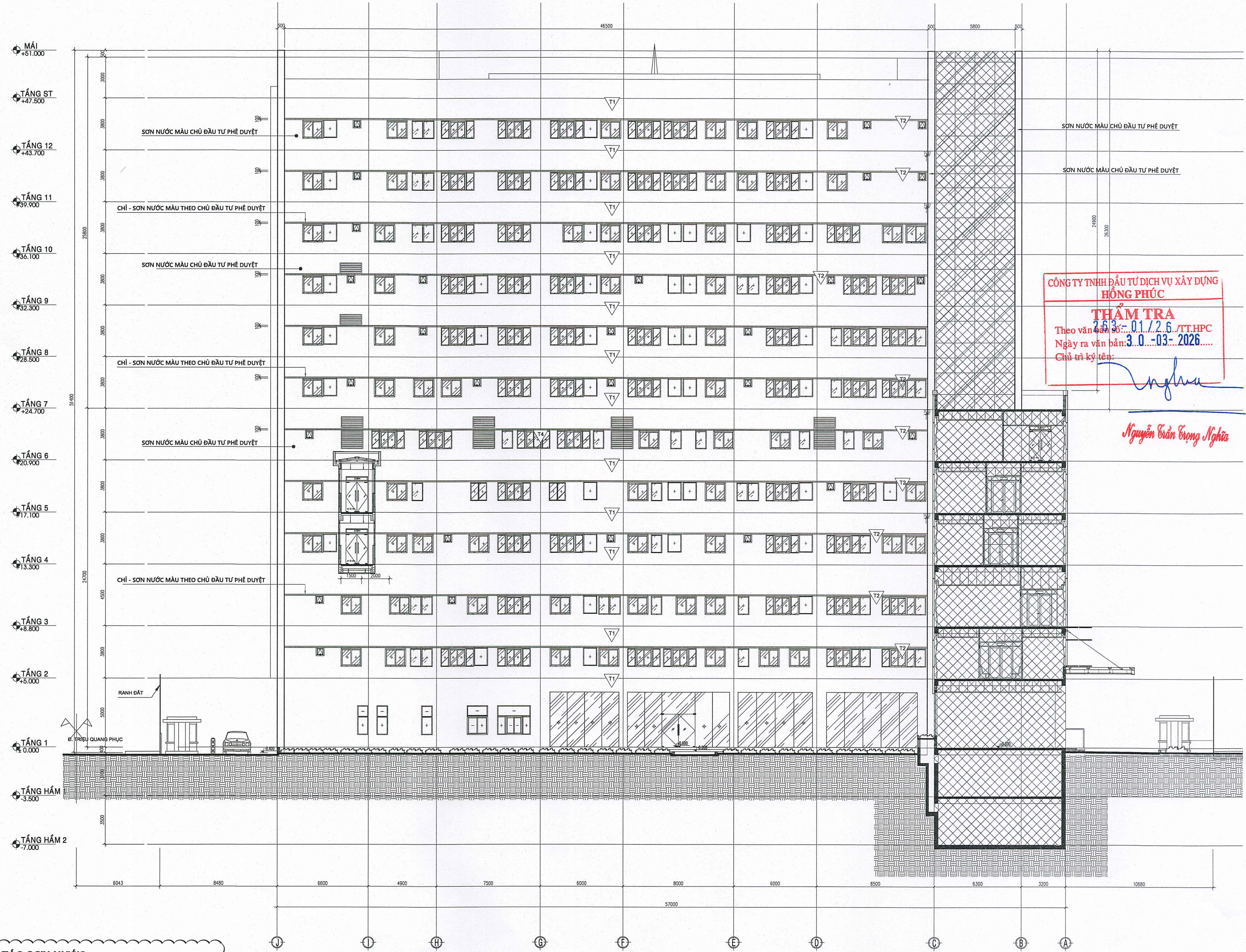
MẶT CẮT B-B - MẶT BÊN TRỰC J-A TL: 1/200 (ÁP DỤNG CHO MẶT BÊN CÒN LẠI)
