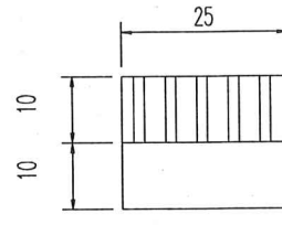
CHI TIẾT BÓ VỈA ĐÁ LOẠI 2 KT: 200X300X250MM (TL:1/25)
