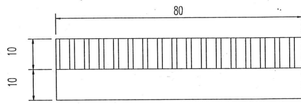
CHI TIẾT BÓ VỈA ĐÁ LOẠI 1 KT: 200X300X800MM (TL:1/25)
