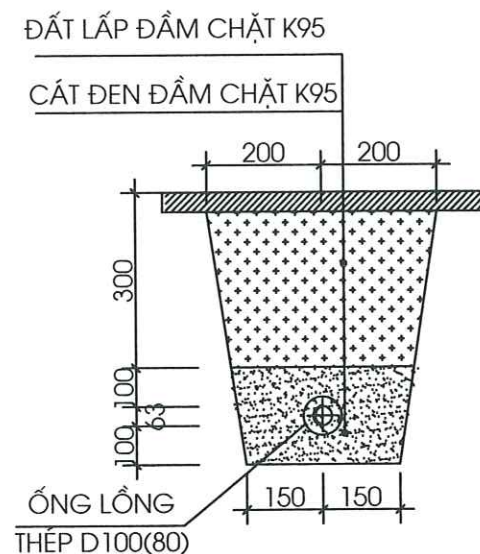
MẶT CẮT MƯƠNG CHÔN ỐNG D63 DƯỚI ĐƯỜNG
