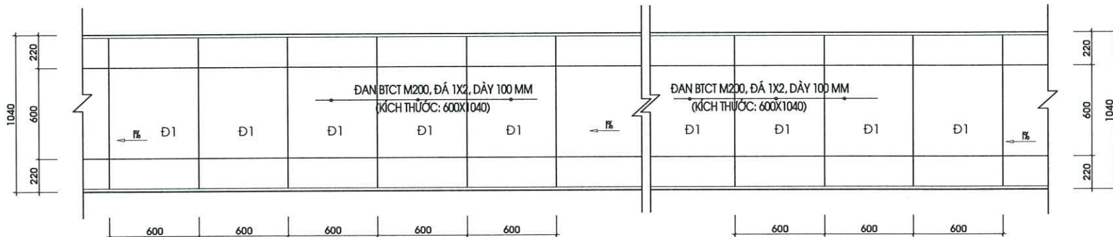
MẶT BẰNG ĐIỂN HÌNH ĐOẠN RÃNH B600 THƯỜNG
