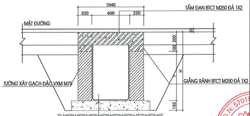
CẮT NGANG ĐOẠN RÃNH CHỊU LỰC B600
