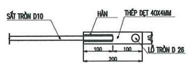
TẠI BẮT TIẾP ĐỊA
