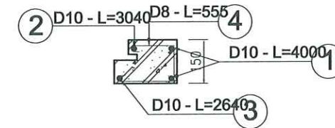
CT BỐ TRÍ THÉP GIẢNG MŨ MỖ
