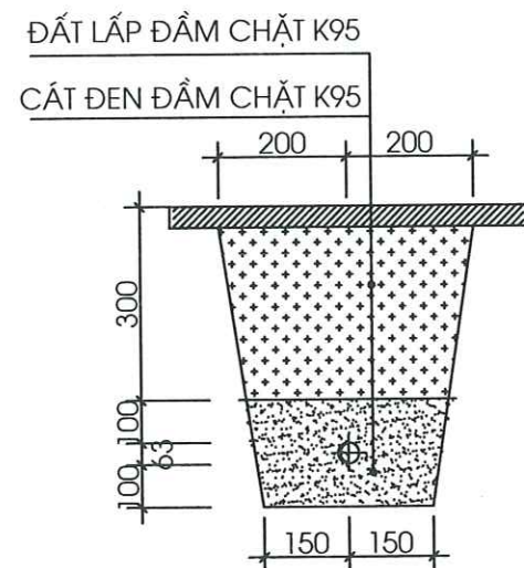
MẶT CẮT MƯƠNG CHÔN ỐNG D63 TRÊN HÈ
