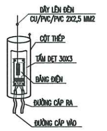
CHI TIẾT BẢNG ĐIỆN
