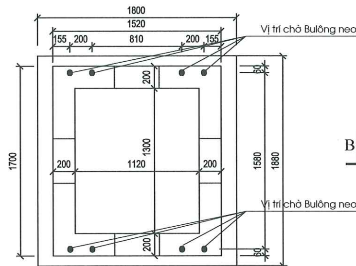
MẶT BẰNG ĐỂ TBA
