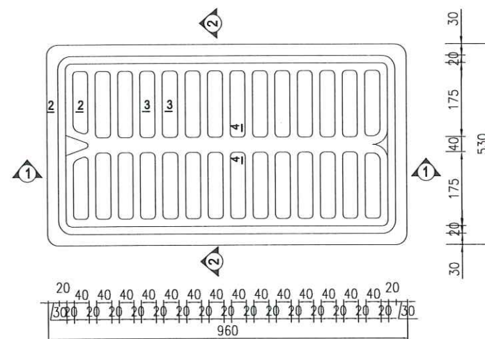
MẶT BẰNG SONG CHẮN RÁC
