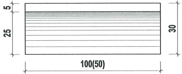
MẶT BẰNG VIÊN VÍA
