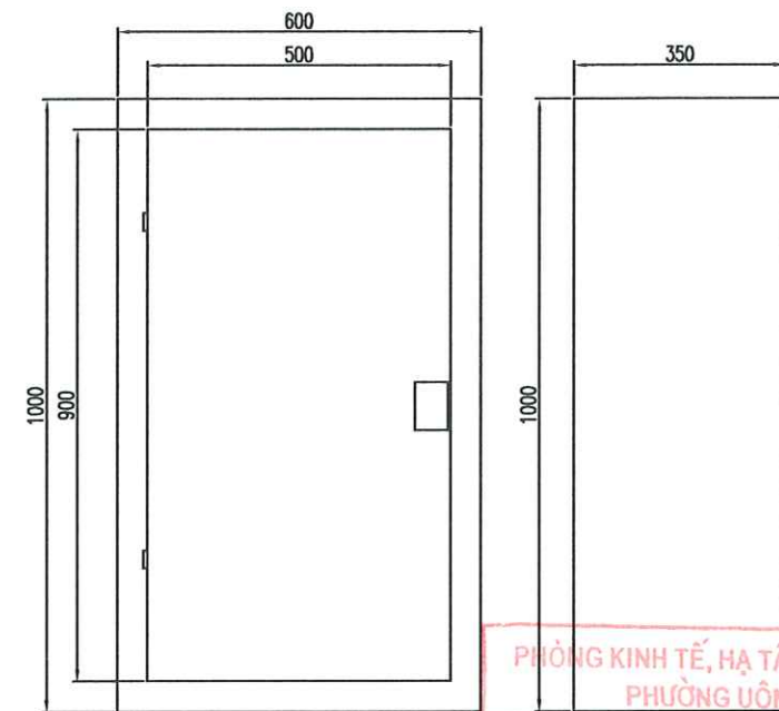
VỎ TỦ ĐIỆN
