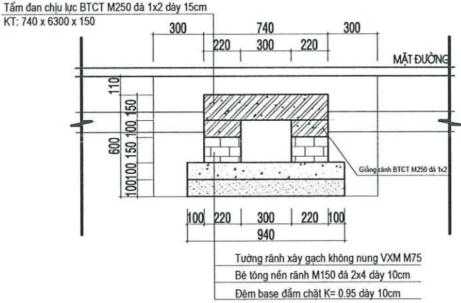
MẶT CẮT RÃNH B300 QUA ĐƯỜNG
