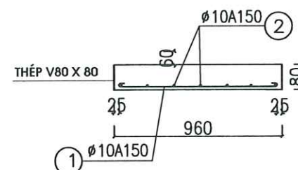
THỐNG KÊ CỐT THÉP HỒ ĐỒNG HỒ DN100
