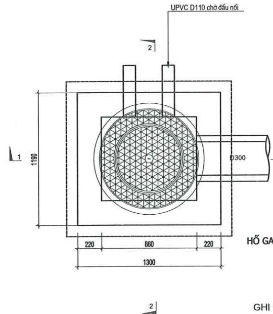
MẶT BẰNG HỐ GA LOẠI 1
