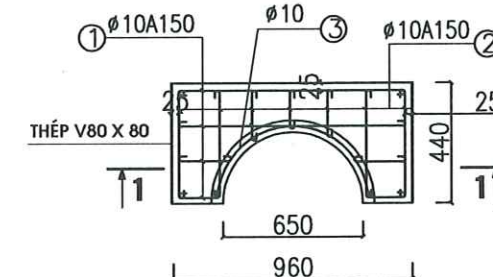
BỐ TRÍ THÉP TẤM ĐAN D2 (02 Tấm)
