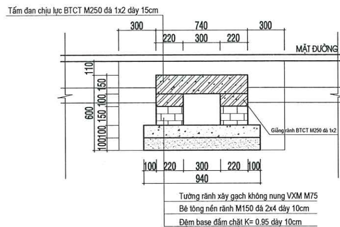
MẶT CẮT B - B RÃNH QUA ĐƯỜNG
