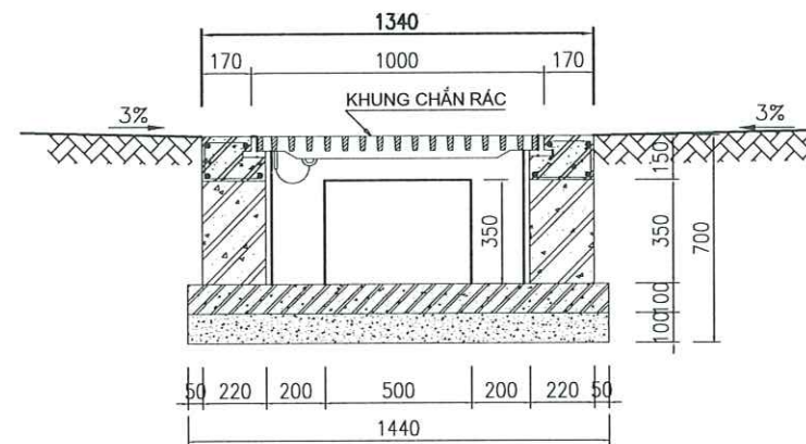
MẶT CẮT D-D
