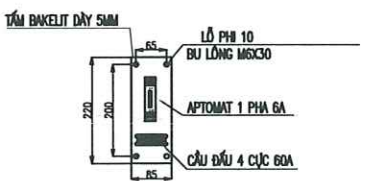
TẠI BẮT TIẾP ĐỊA
