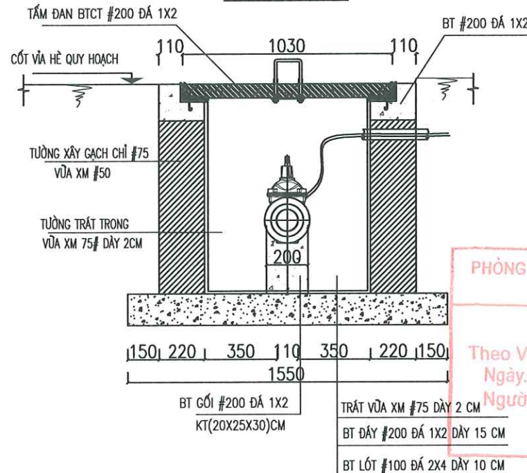
MẶT CẮT B - B
