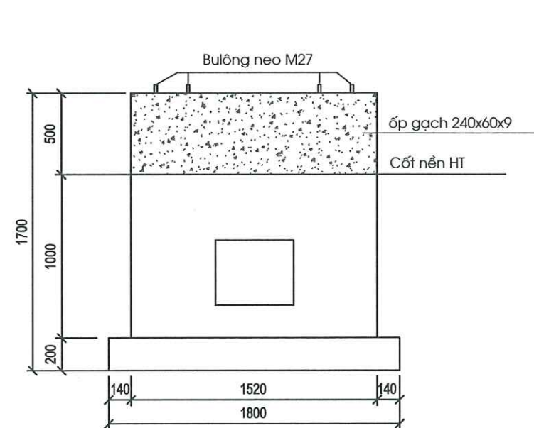
MẶT ĐÚNG 1 ĐỂ TBA
