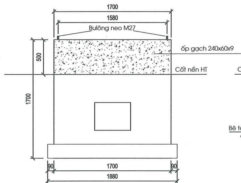
MẶT ĐÚNG 2 ĐỂ TBA
