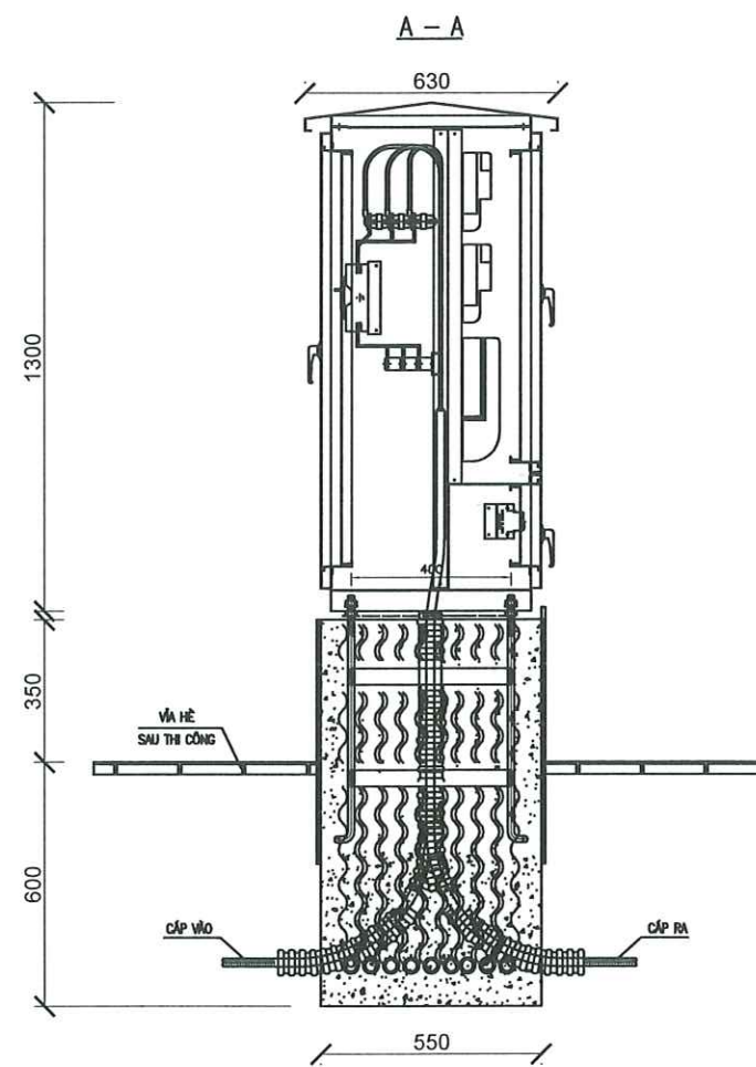
THỐNG KÊ VẬT LIỆU CHO 1 MÓNG TỦ ĐIỆN
