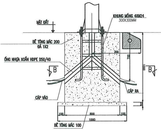
MÓNG CỘT ĐÈN CHIẾU SÁNG - CỘT 8M
