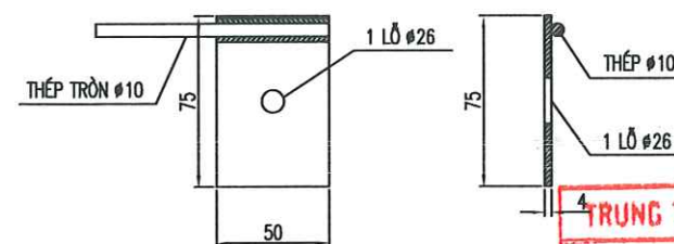
TAI BẮT TIẾP ĐỊA
