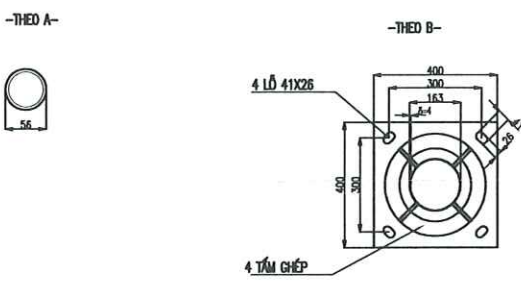
KHUNG MÓNG CỘT ĐÈN CHIẾU SÁNG
