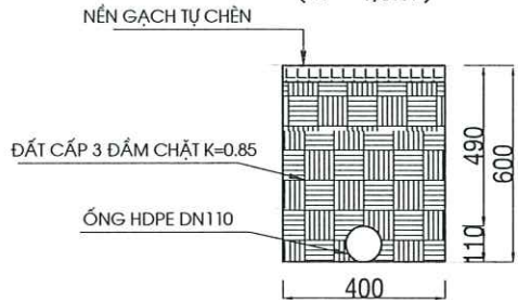
MẶT CẮT ĐÀO MƯƠNG ĐẶT ỚNG ( L = 4,5M )
