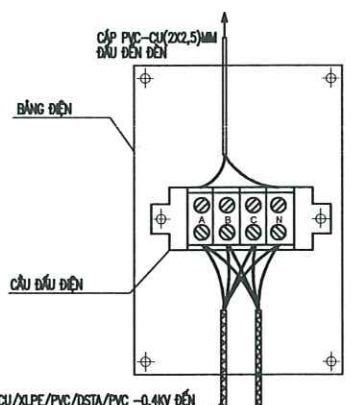
PHƯƠNG THỨC ĐẦU NỐI TẠI CỘT
