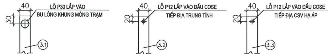
CHI TIẾT ĐẦU DÂY NỐI TIẾP ĐỊA
