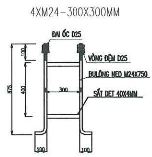
KHUNG MÓNG CỘT ĐÈN CHIẾU SÁNG
