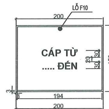
BIỂN TÊN LỘ ĐƯỜNG DÂY ĐẾN TỦ RMU
