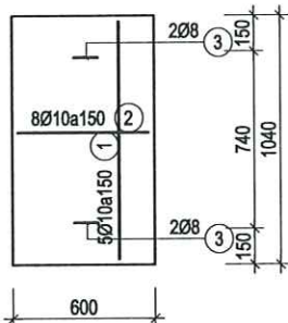
CHI TIẾT TẮM ĐẠN Đ1
