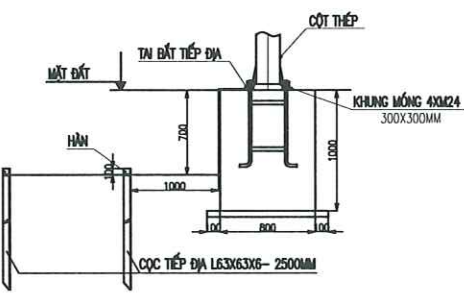
TIẾP ĐỊA CHO CỘT ĐÈN
