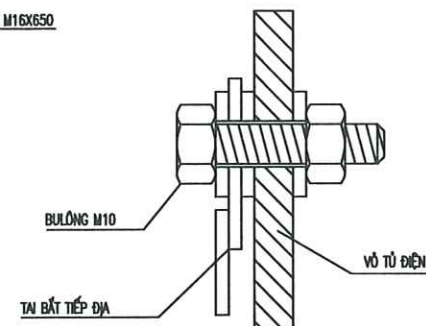
BẮT DÂY TIẾP ĐỊA
