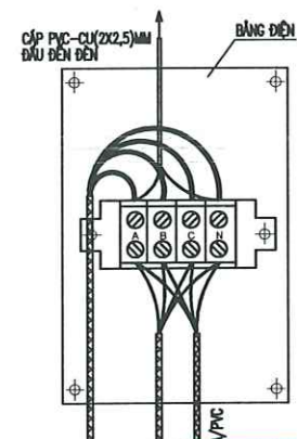
PHƯƠNG THỨC ĐẦU NỐI TẠI CỘT RẾ NHÁNH
