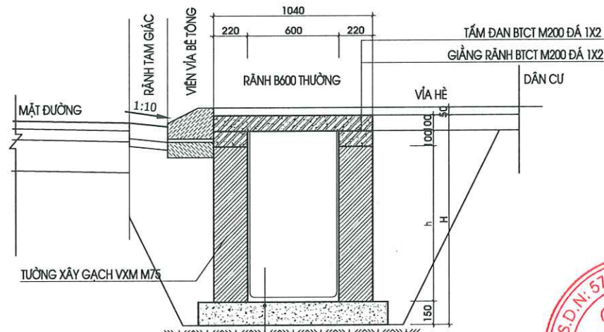
CẮT NGANG RÃNH B600 THƯỜNG
