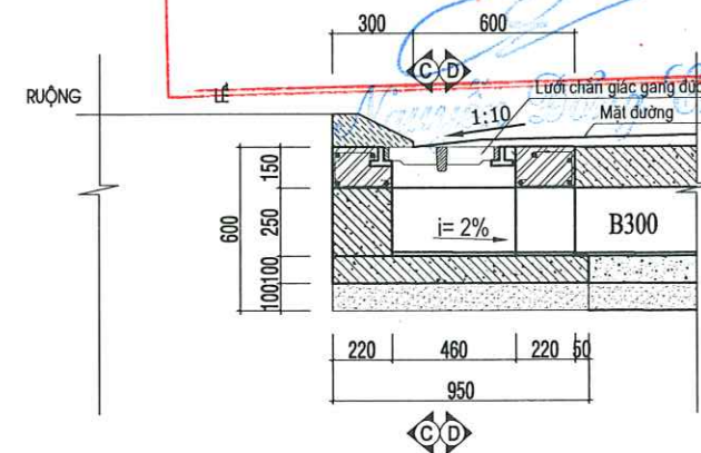
MẮT CẮT HỔ THU CT 1
