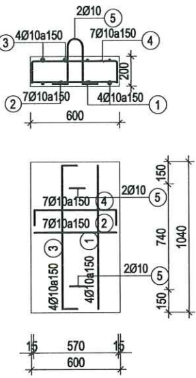
CHI TIẾT TẦM ĐAN Đ2
