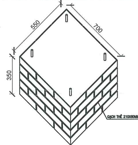
CHI TIẾT ỚP GẠCH THÈ MÓNG TỦ ĐIỆN CÔNG TỬ
