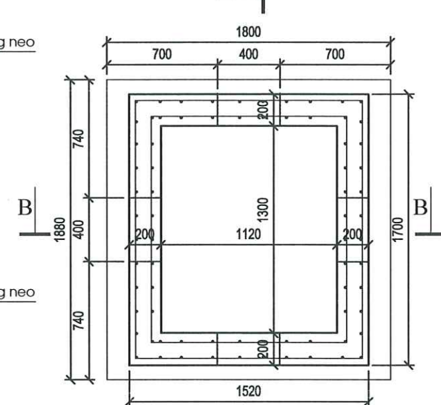
MẶT BẰNG BỐ TRÍ CỐT THÉP
