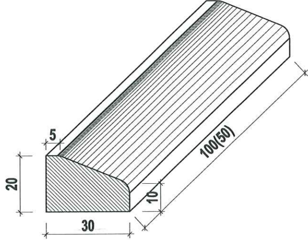
HÌNH CHIẾU VIÊN VÍA
