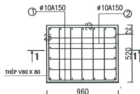
BỐ TRÍ THÉP TẤM ĐAN D1 (02 Tấm)
