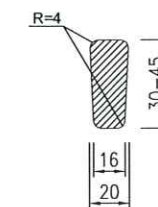
CẮT 3-3
