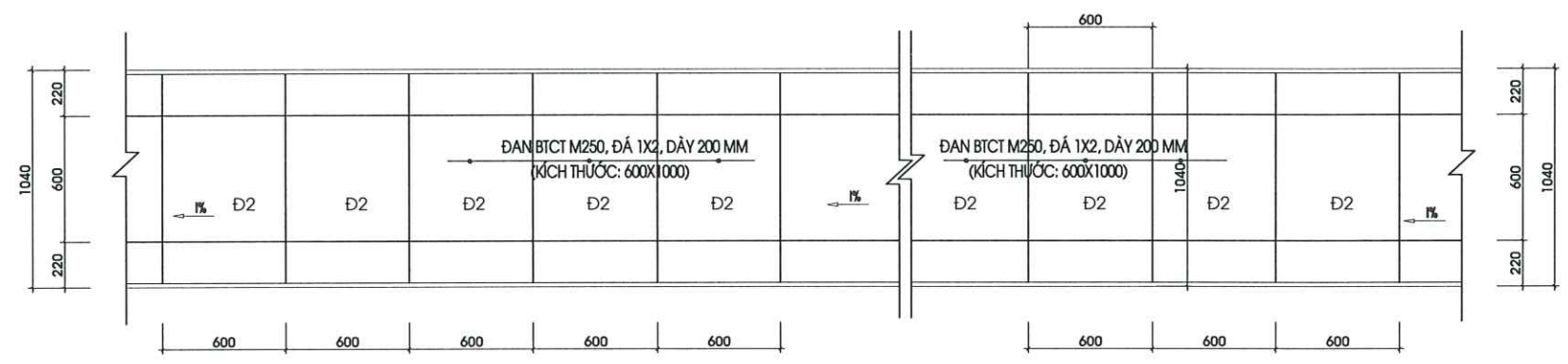
MẶT BẰNG ĐIỂN HÌNH RÃNH CHỊU LỰC B600
