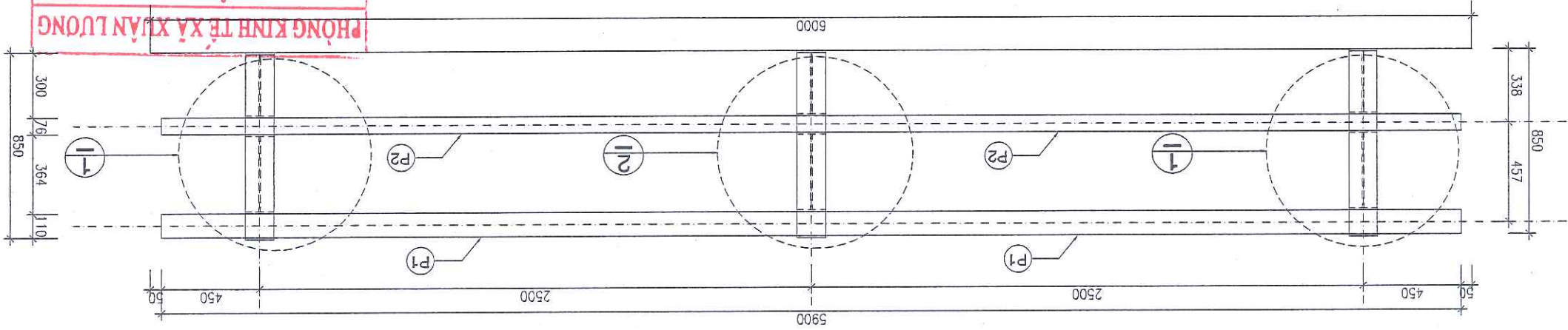
BỐ TRÍ LAN CAN TRÊN NHỊP TL:1/25 - SL:04
