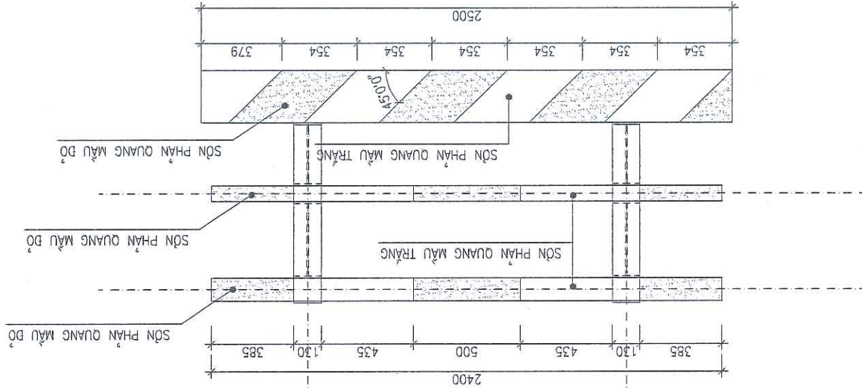
BỐ TRÍ SƠN PHẢN QUANG LAN CÁN, GỖ CHẴN MỖ CẦU TL:1/25 - SL:04
