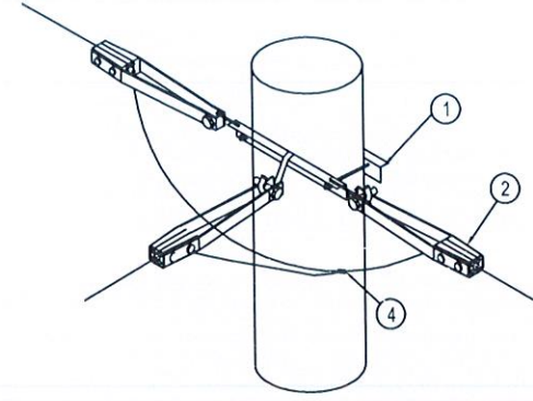
CỘT NÉO THẲNG, NÉO GÓC ĐƠN RỄ NHÁNH
