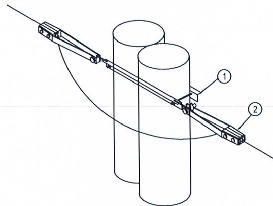
CỘT NÉO THẲNG ĐÚP
