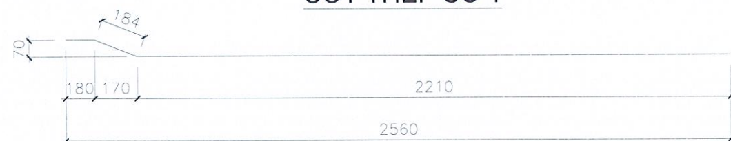
CỐT THÉP SỐ 2
