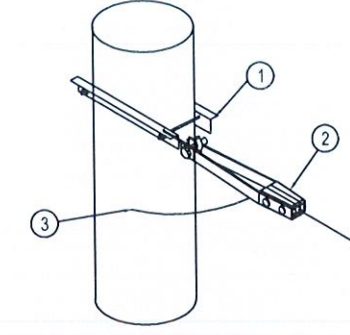
CỘT NÉO CUỐI ĐƠN
