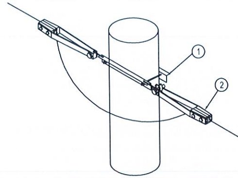
CỘT NÉO THẲNG, NÉO GÓC ĐƠN
