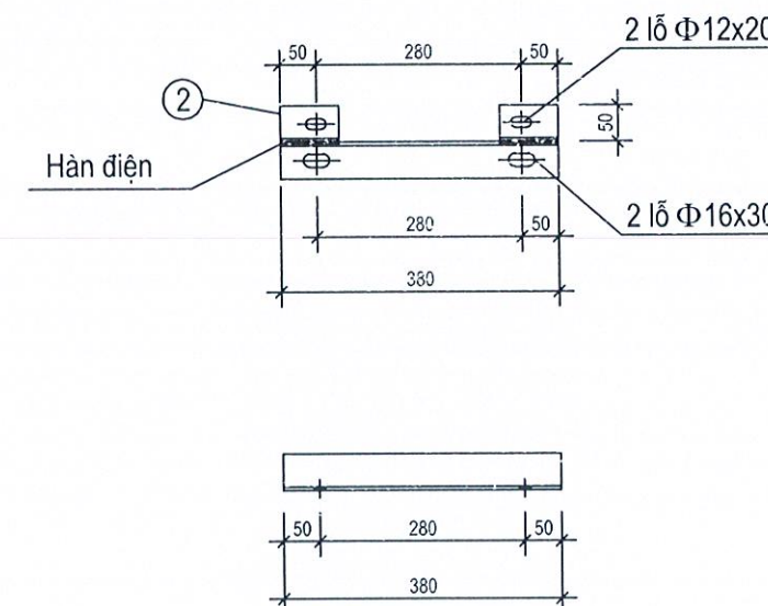
Thanh xà đỡ hòm công tơ
