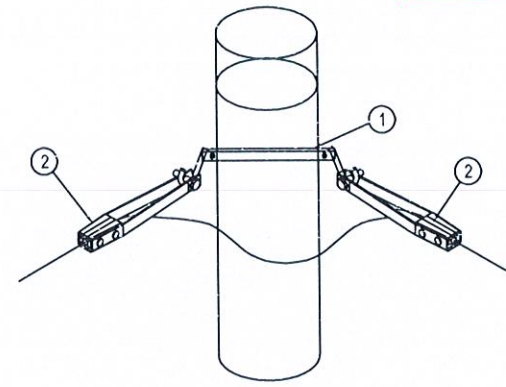
CỘT NÉO GÓC ĐÚP
