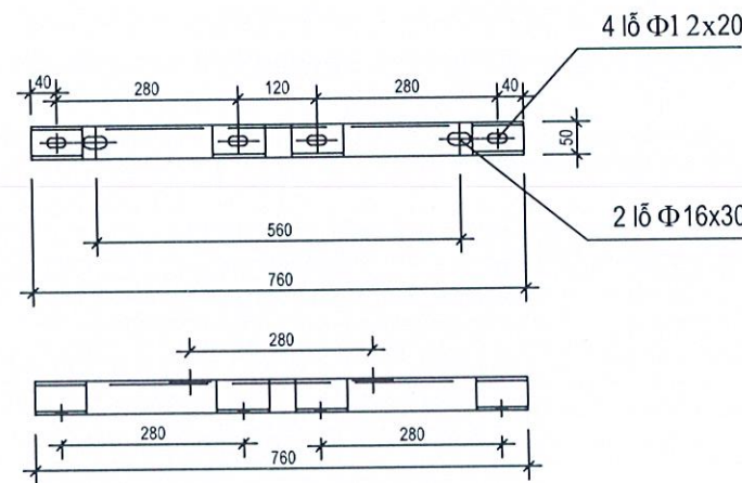
Thanh xà đỡ hòm công tơ
