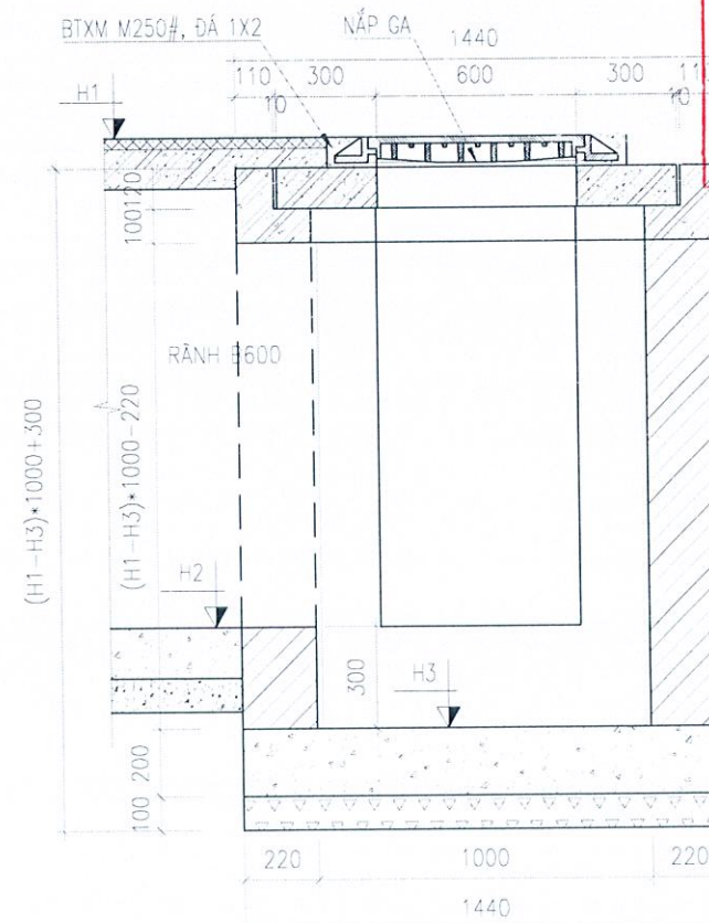
MẶT CẮT 2-2 TỶ LỆ: 1/25
