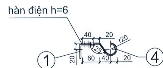
4-MỐC NÉO (TREO)
