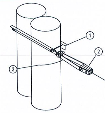
CỘT NÉO CUỐI ĐÚP
