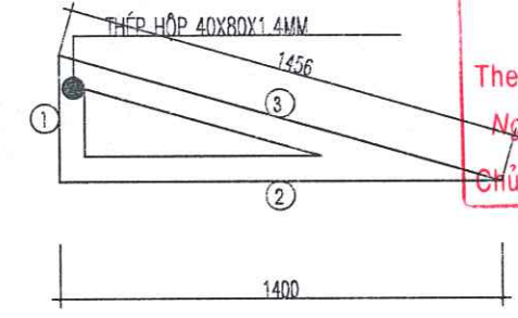
VÌ KÈO VK-2 (SL=01CK)
