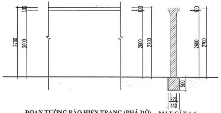
ĐOẠN TƯỜNG RÀO HIỆN TRẠNG (PHÁ DỠ) ĐOẠN A-B (L=3500MM) MẶT CẮT 1-1
