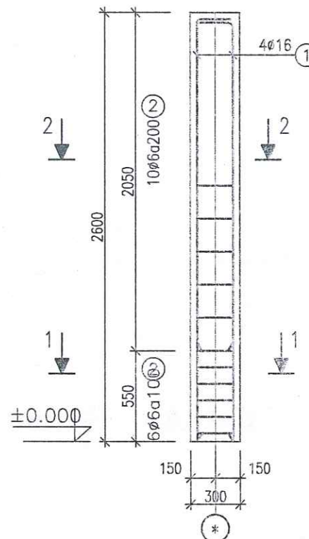
CỘT C1 (SL: 02)
