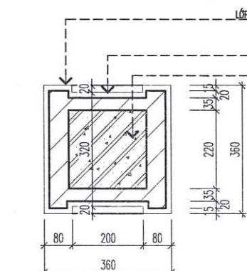
CHI TIẾT CỘT ( SL :02)
