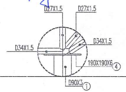
CHI TIẾT: CT2
