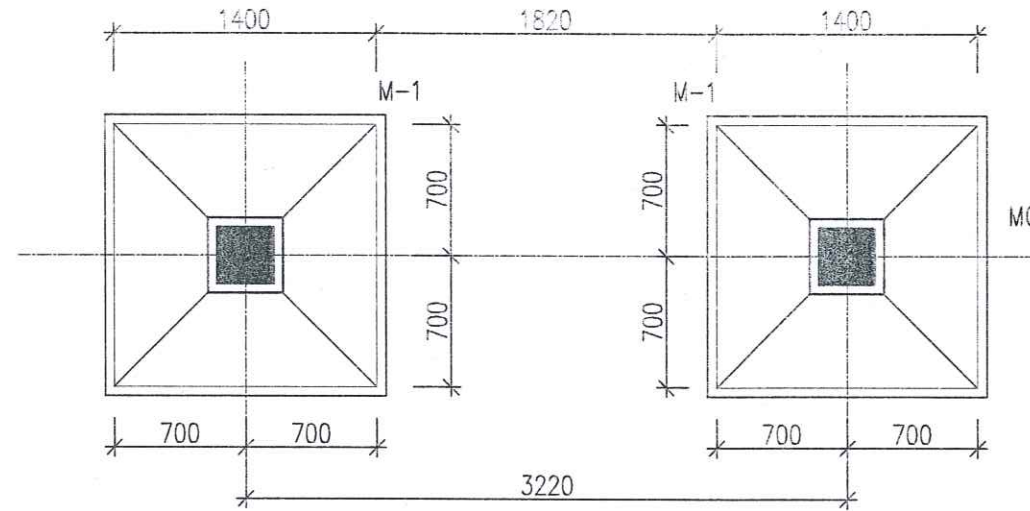
MẶT BẰNG MÓNG CỎNG
