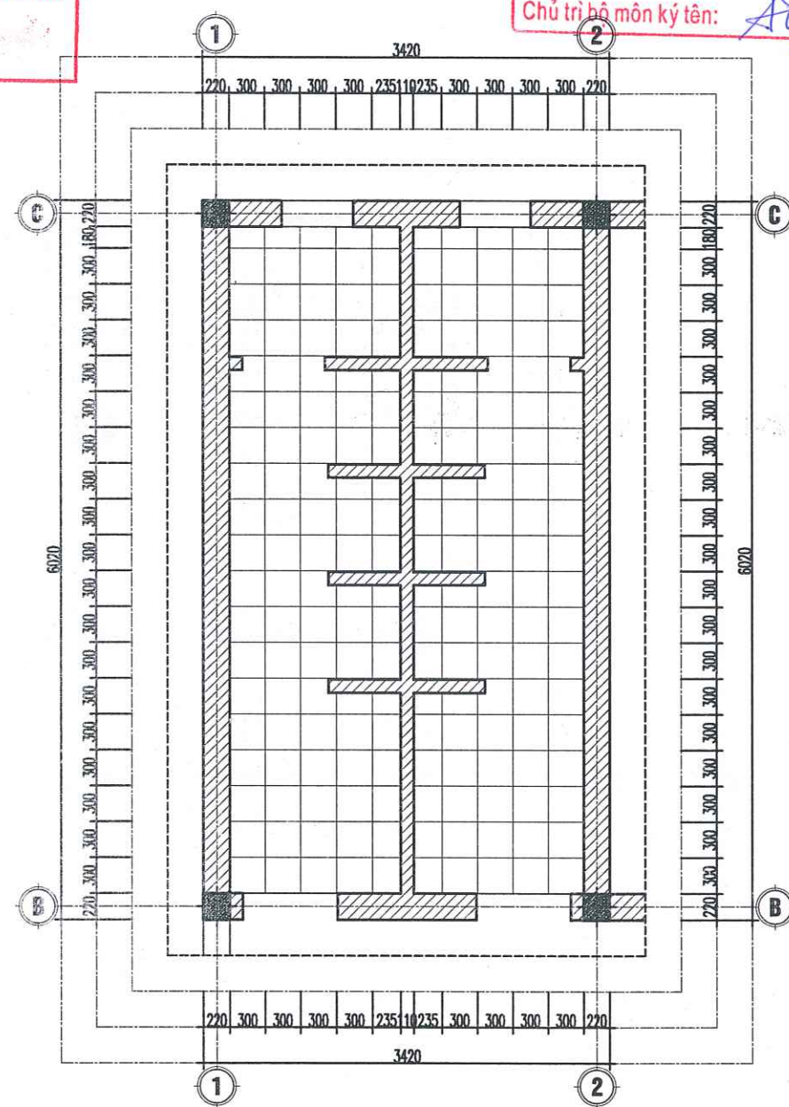
MẶT BẰNG LÁT SÀN WC TẦNG 1 + TẦNG 2 HIỆN TRẠNG
