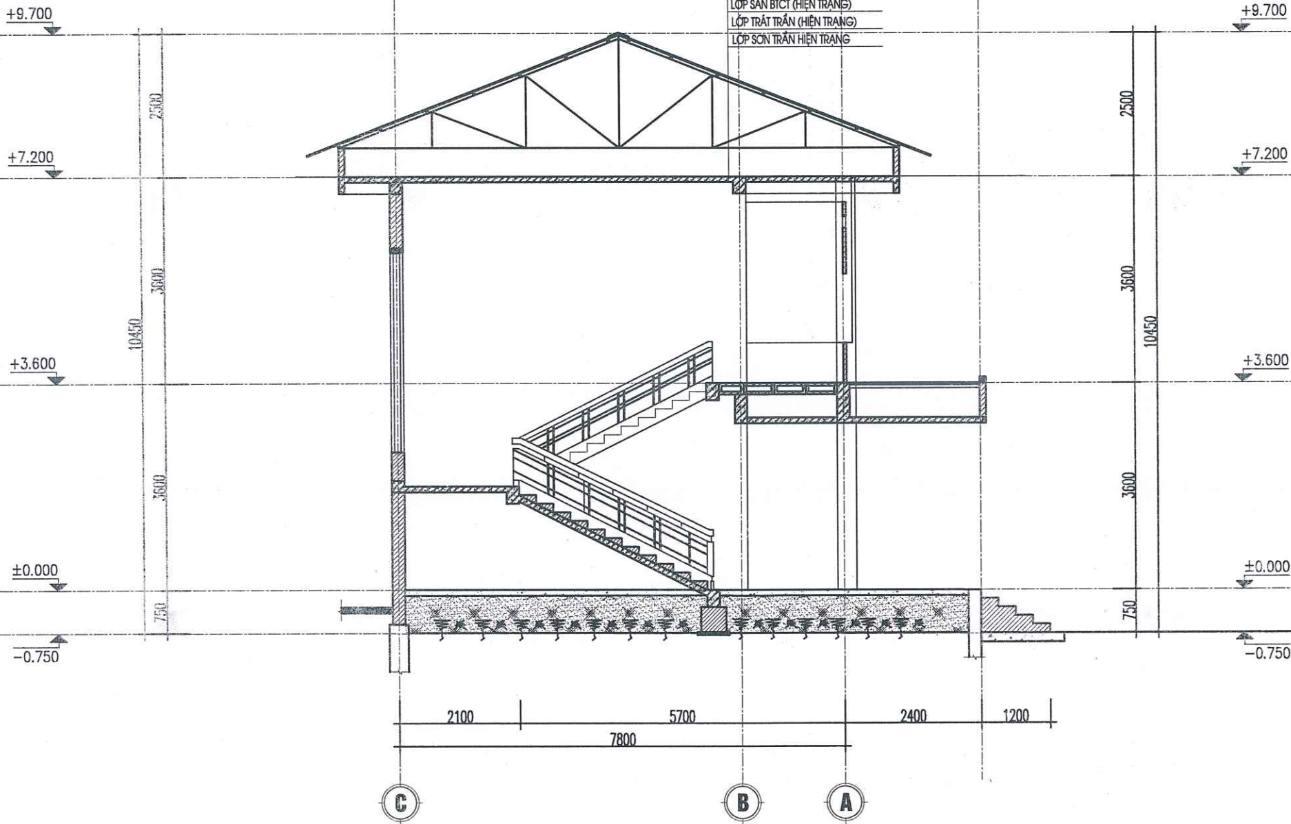
MẶT CẮT HIỆN TRẠNG 2-2
