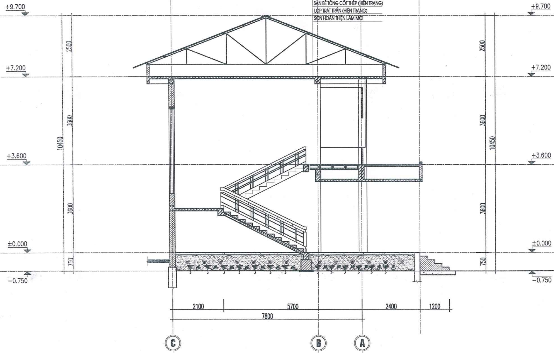
MẶT CẮT TRỰC 2-2
