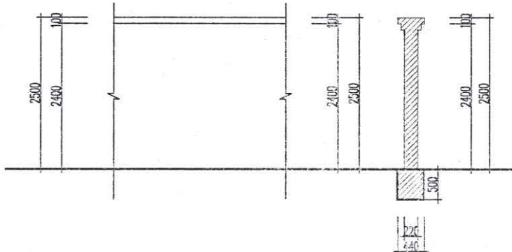
ĐOẠN TƯỜNG RÀO HIỆN TRẠNG (PHÁ DỠ) ĐOẠN E-F (L=4600MM) MẶT CẮT 1-1
