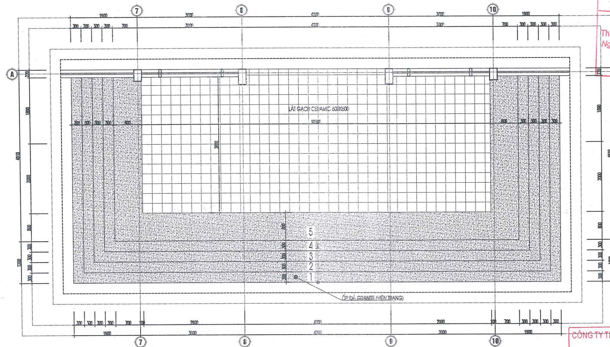
MẶT BẰNG SẴN CHÍNH CẢI TẠO
