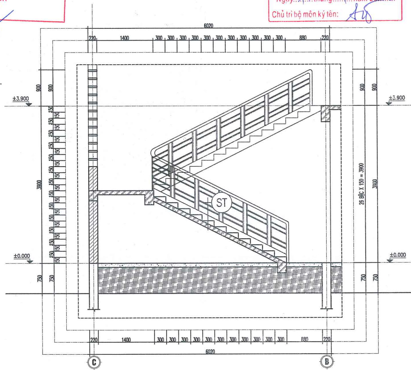
MẶT CẮT THANG HIỆN TRẠNG
