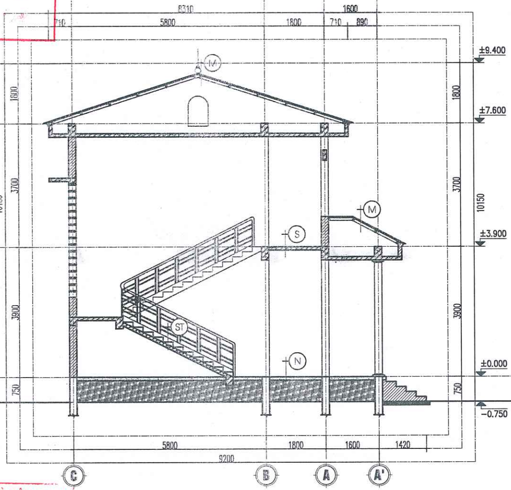
MẶT CẮT 2-2 CẢI TẠO
