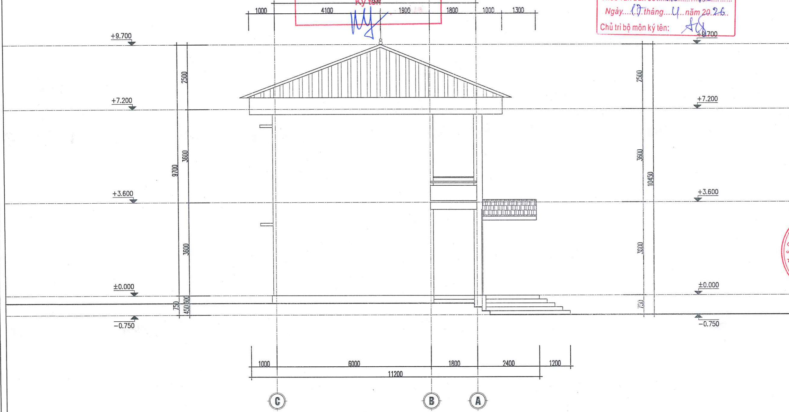
MẶT ĐỨNG HIỆN TRẠNG TRỤC C-A
