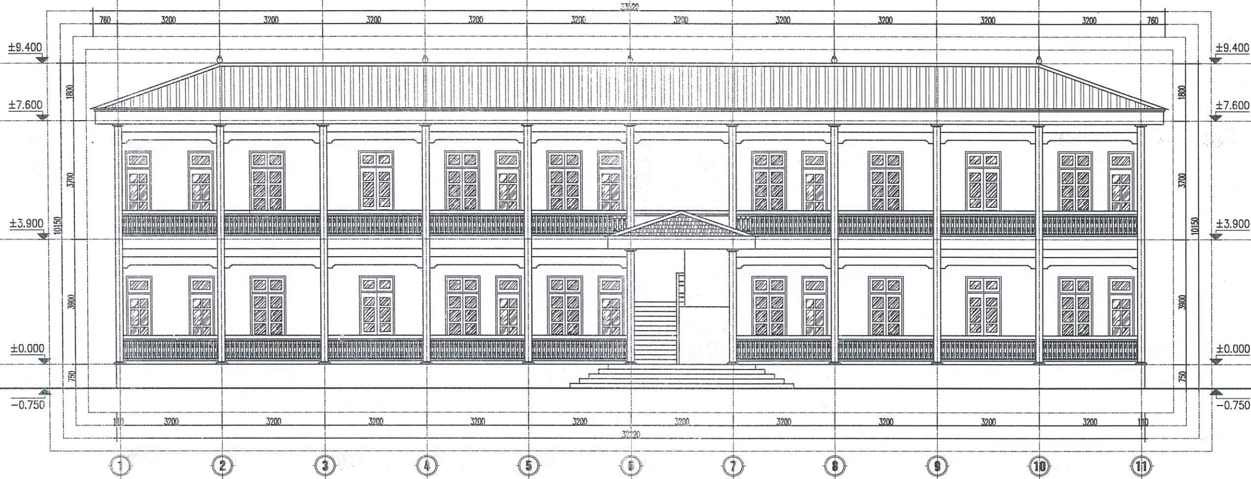
MẶT ĐỨNG TRỤC 1-11 HIỆN TRẠNG
