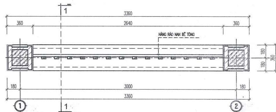
MẶT BẰNG CHI TIẾT ĐIỂN HÌNH
