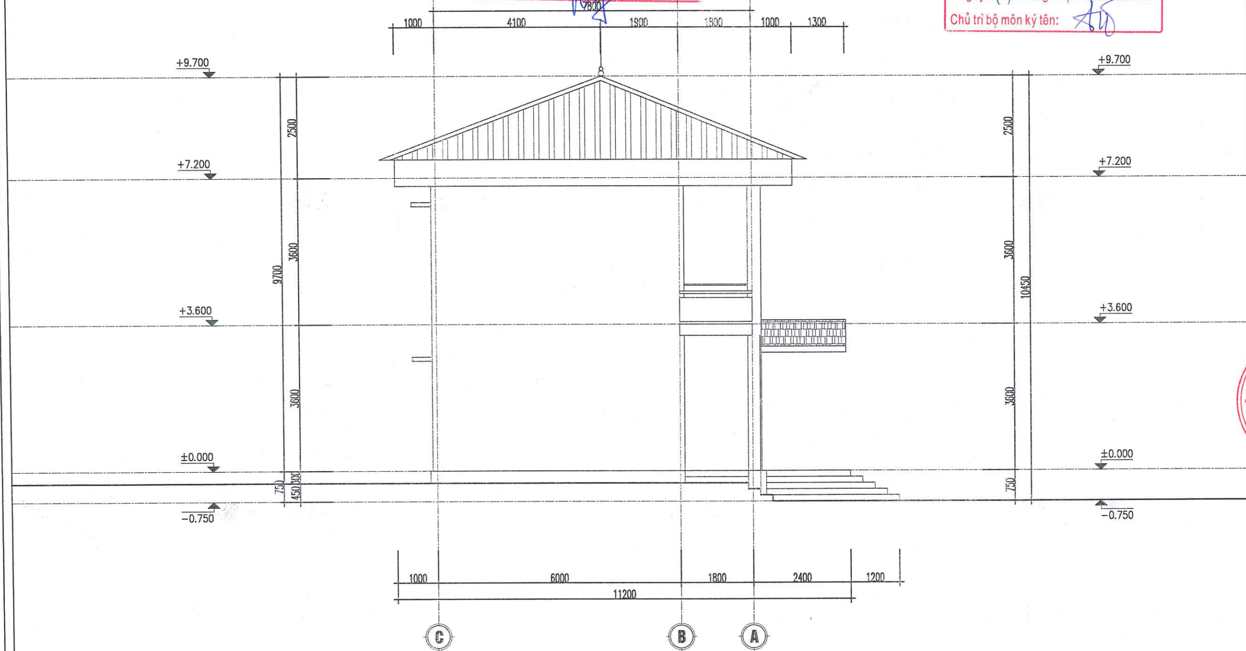
MẶT ĐỨNG TRỤC C-A CẢI TẠO
