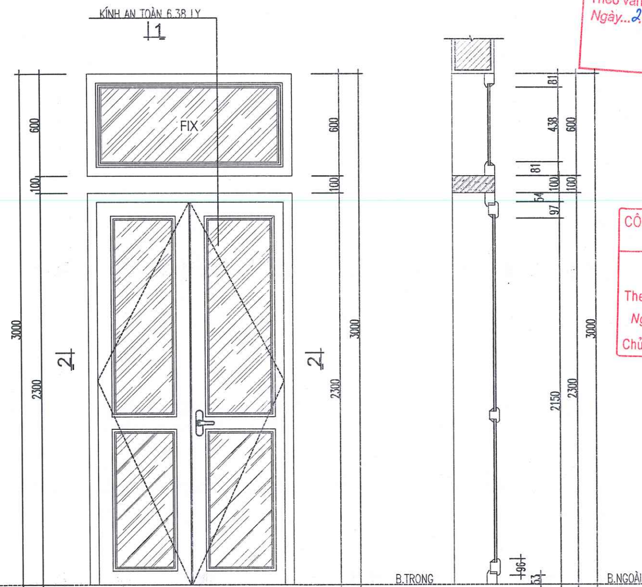
CẮT 1-1
