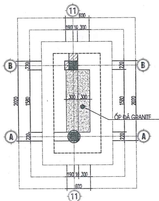
MẶT BẰNG SẢNH PHỤ
