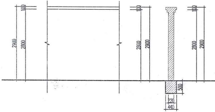
ĐOẠN TƯỜNG RÀO HIỆN TRẠNG (PHÁ DỠ) ĐOẠN B-C (L=18900MM) MẶT CẮT 1-1
