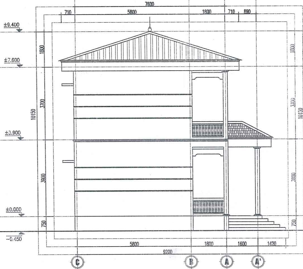
MẶT ĐỨNG TRỤC C-A' CẢI TẠO
