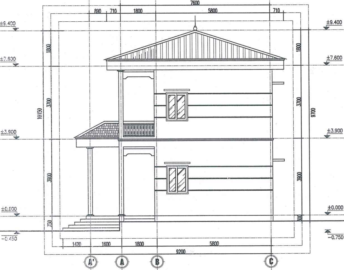
MẶT ĐỨNG TRỤC A'-C CẢI TẠO
