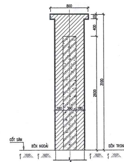
MẶT CẮT 3-3
