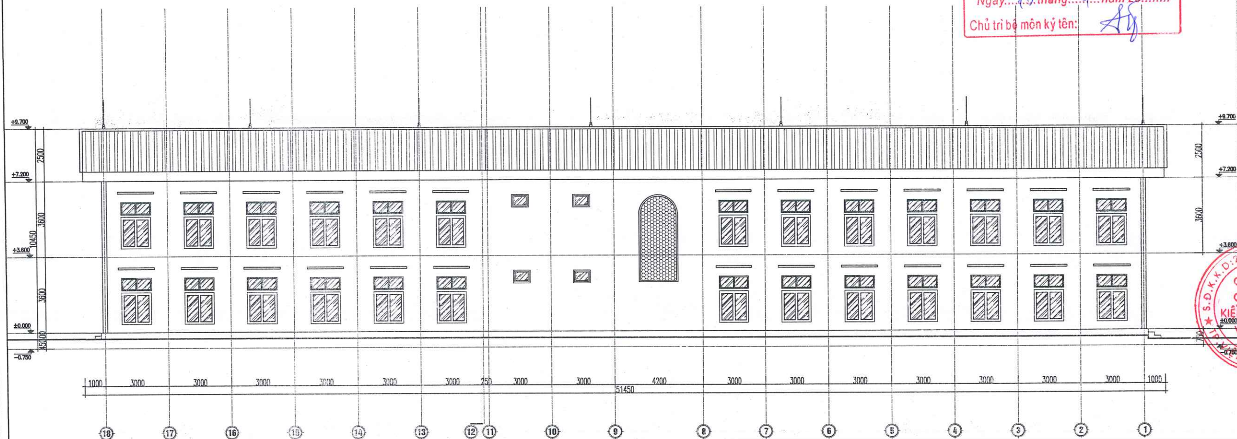
MẶT ĐÚNG CẢI TẠO TRỰC 18-1
