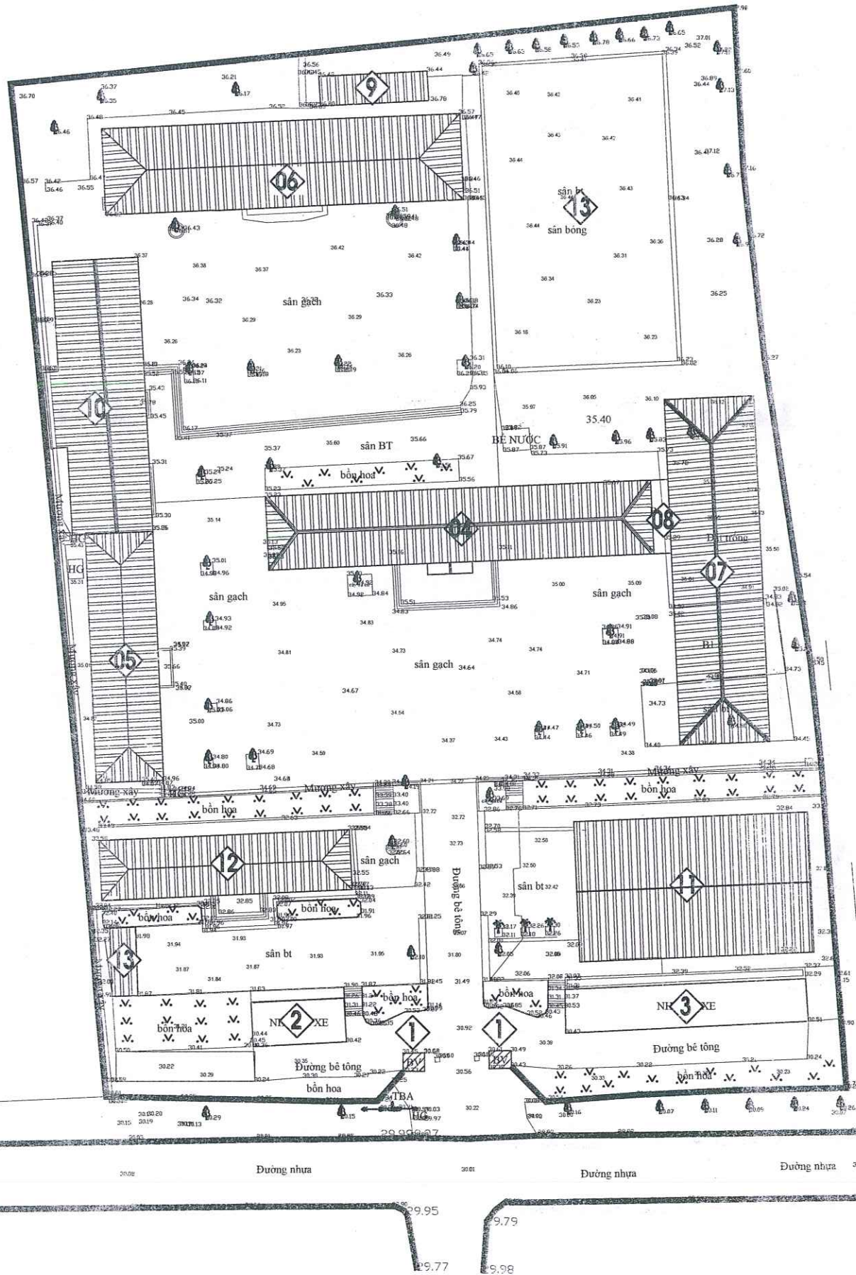
MẶT BẰNG TỔNG THỂ CÔNG TRÌNH (PHẦN HIỆN TRẠNG)
