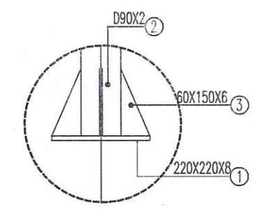
CHI TIẾT: CT1
