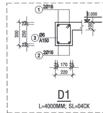
BẢNG THỐNG KÊ CỐT THÉP
