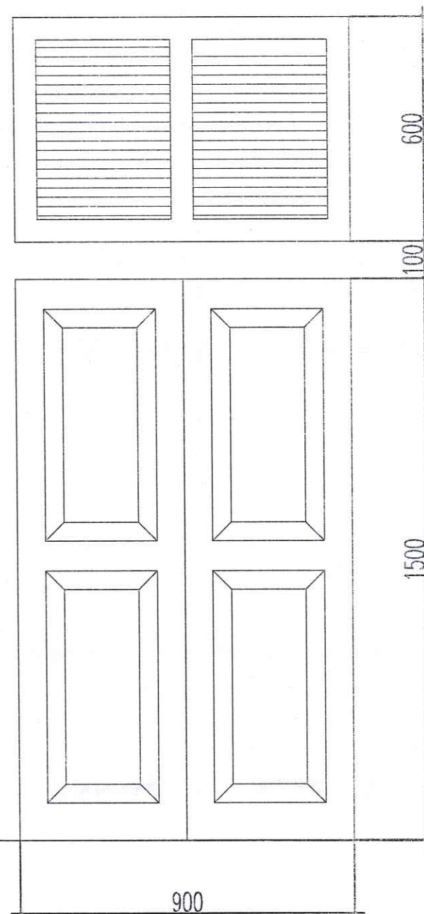
CỬA SỔ S3(SL:2 BỘ)
