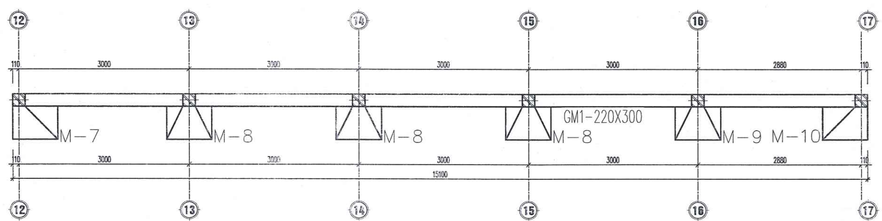
MẶT BẰNG MÓNG TƯỜNG RÀO ĐOẠN D-F
