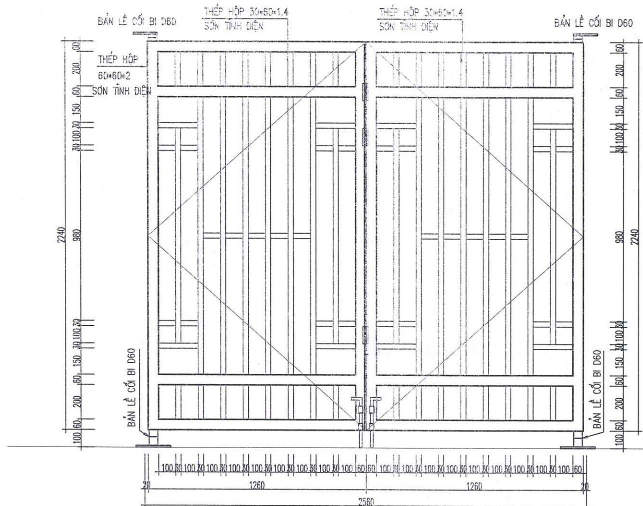
CHI TIẾT CỔNG PHỤ (SL: 01 BỘ)
