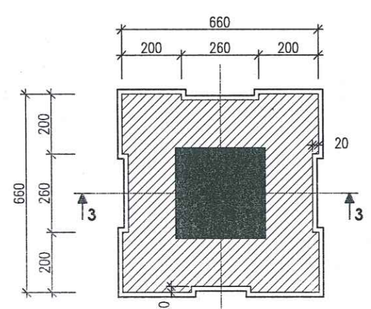
TRỤ CỔNG CHÍNH (SL: 02)
