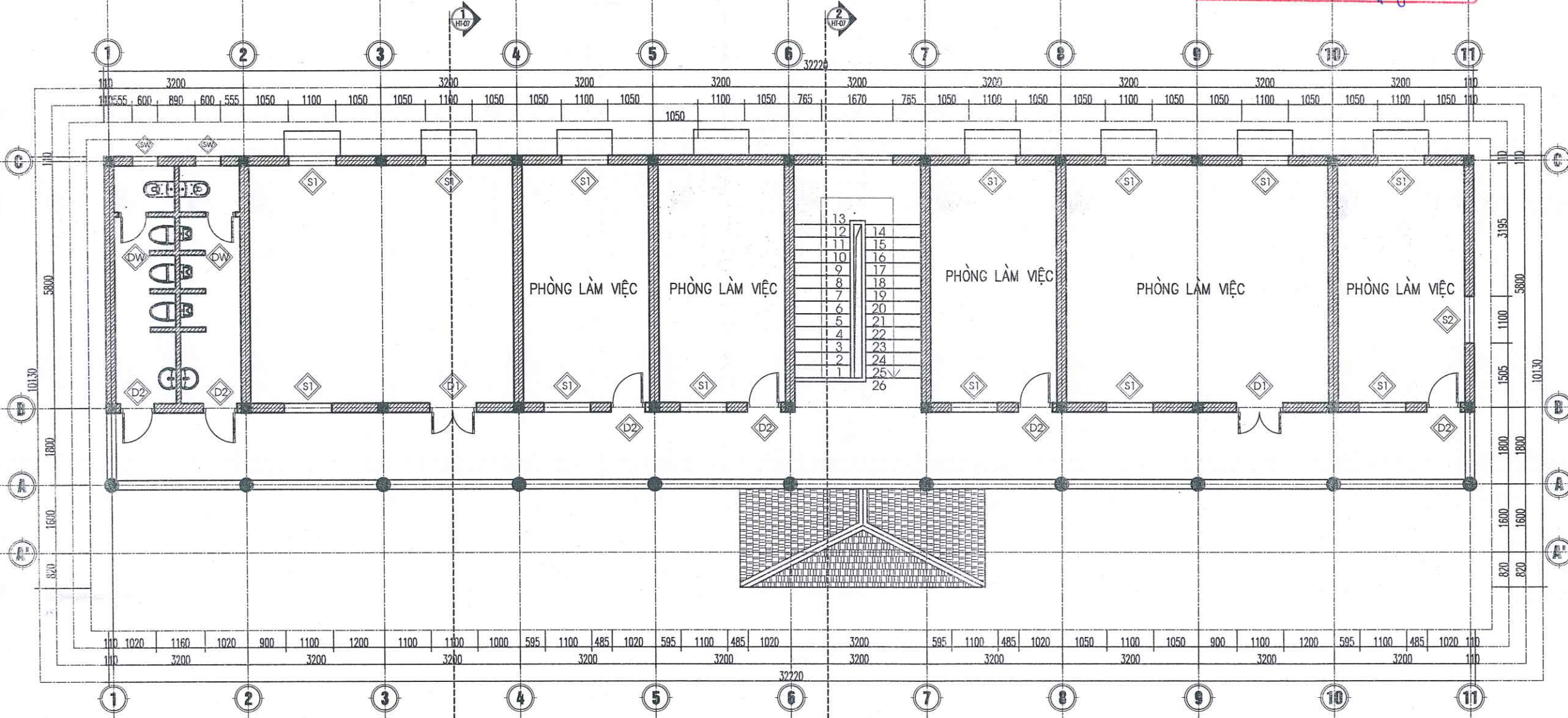
MẶT BẰNG HIỆN TRẠNG TẦNG 2
