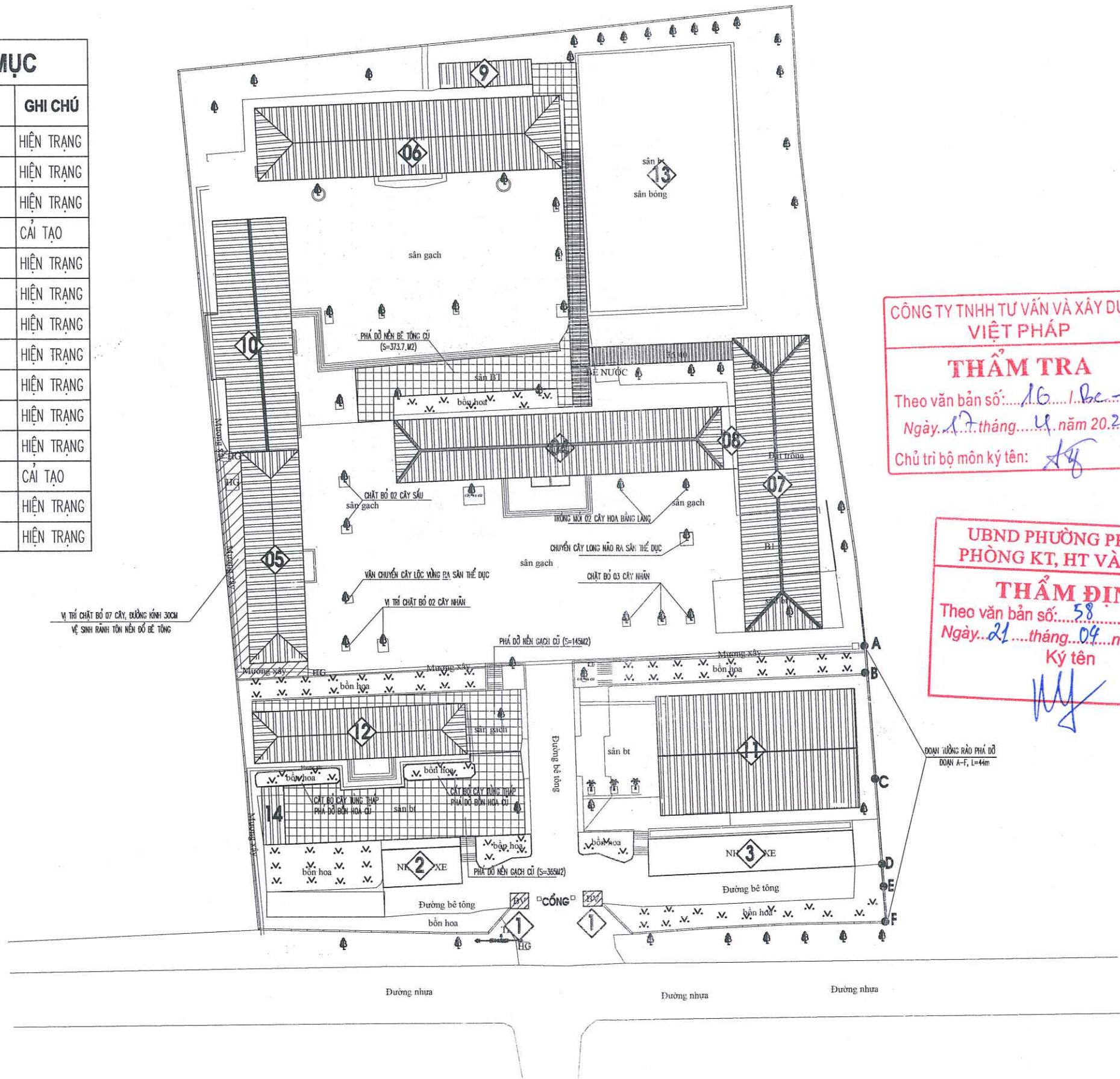
MẶT BẰNG TỔNG THỂ CÔNG TRÌNH (PHẦN PHÁ DỠ)
