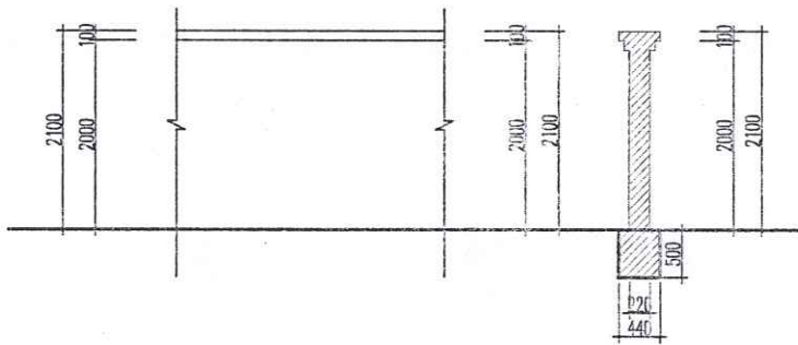
ĐOẠN TƯỜNG RÀO HIỆN TRẠNG (PHÁ DỠ) ĐOẠN C-D (L=6500MM) MẶT CẮT 1-1
