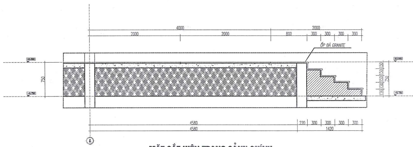
MẶT CẮT HIỆN TRẠNG SẢNH CHÍNH
