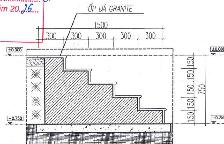
MẶT CẮT BẬC SẢNH CHÍNH
