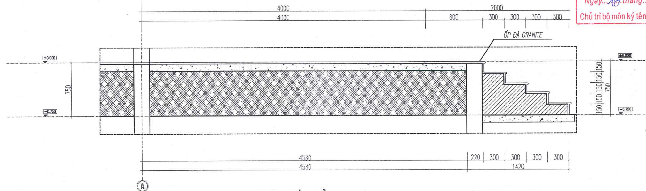
MẶT CẮT SẴN CHÍNH
