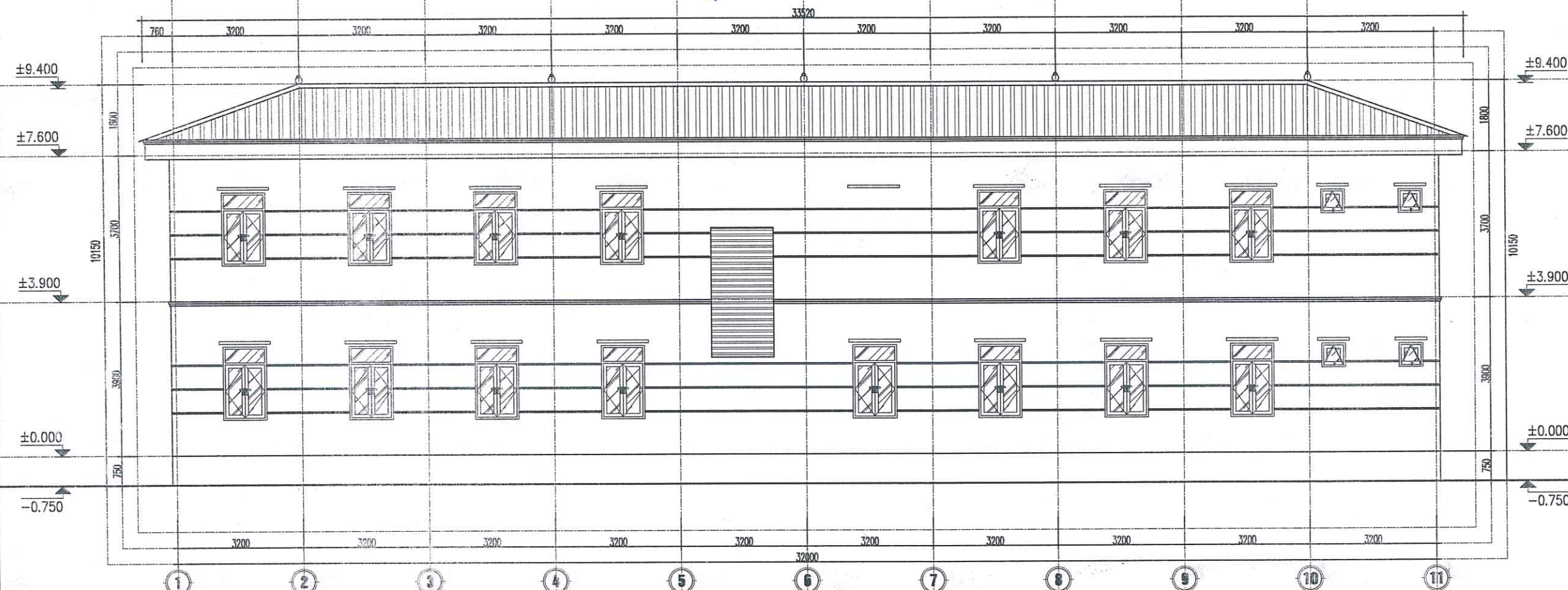
MẶT ĐỨNG TRỤC 11-1 CẢI TẠO
