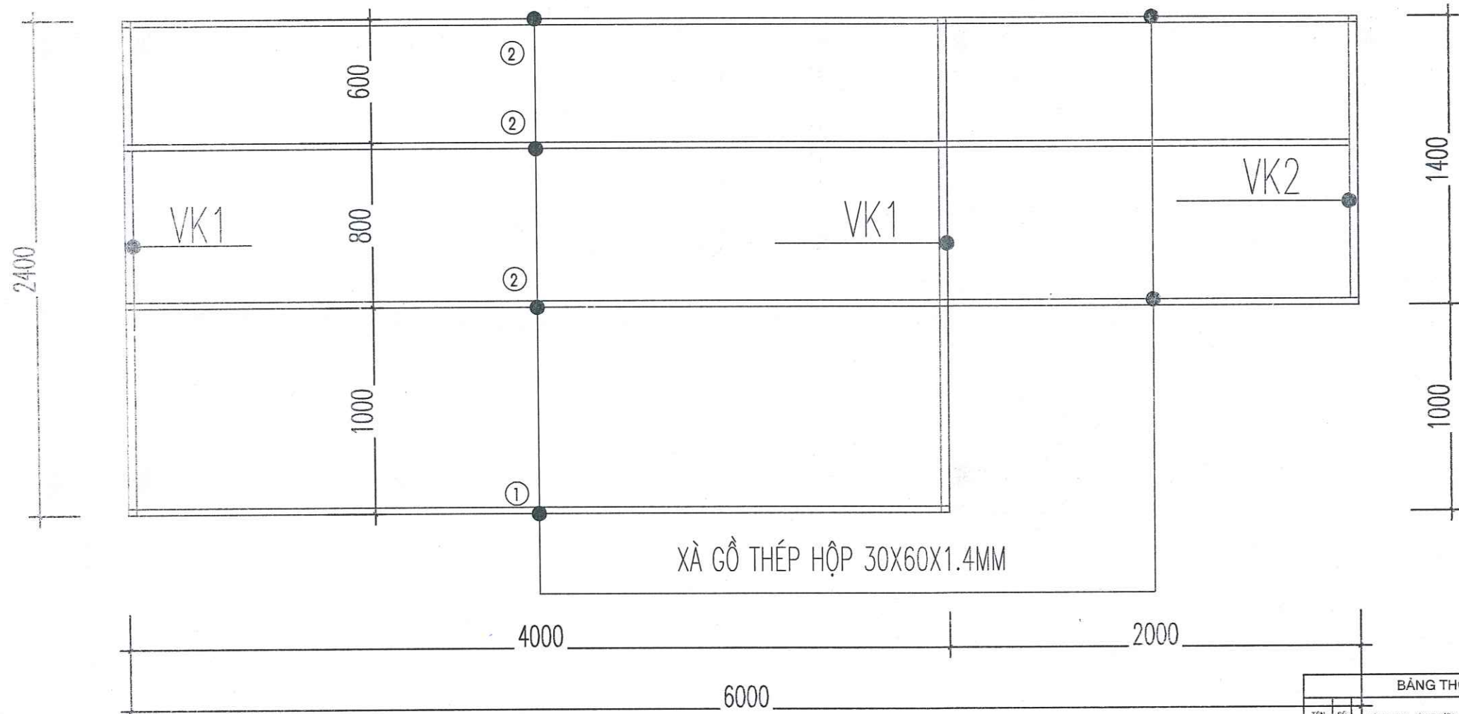
MẶT BẰNG XÀ GỖ MÁI
