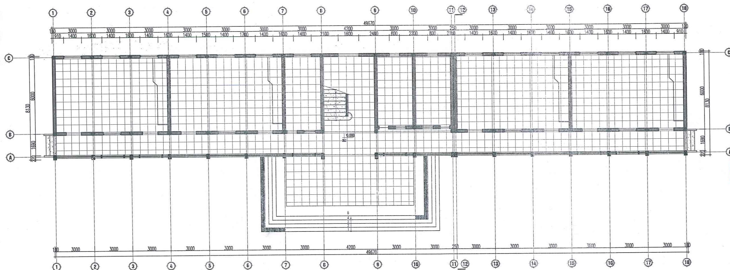
MẶT BẰNG LÁT SÀN CẢI TẠO TẦNG 1
