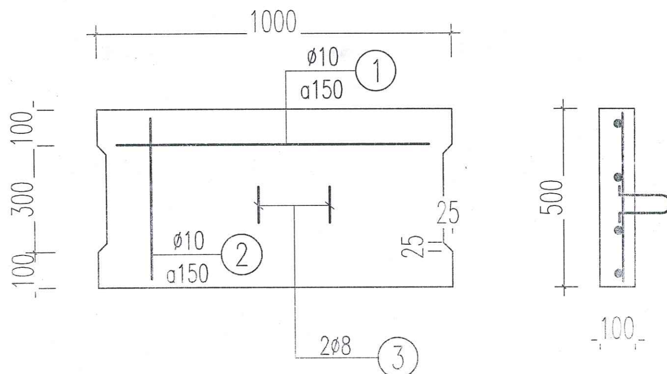
CHI TIẾT TẤM ĐẠN (số lượng =177 CK)
