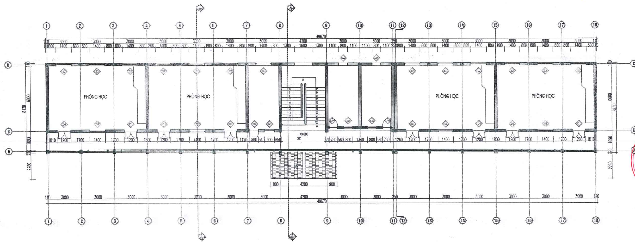
MẶT BẰNG HIỆN TRẠNG TẦNG 2
