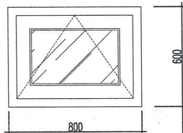
CỬA SỔ SW(SL:08 BỘ)
