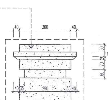
CHI TIẾT ĐẦU CỘT(SL:02)
