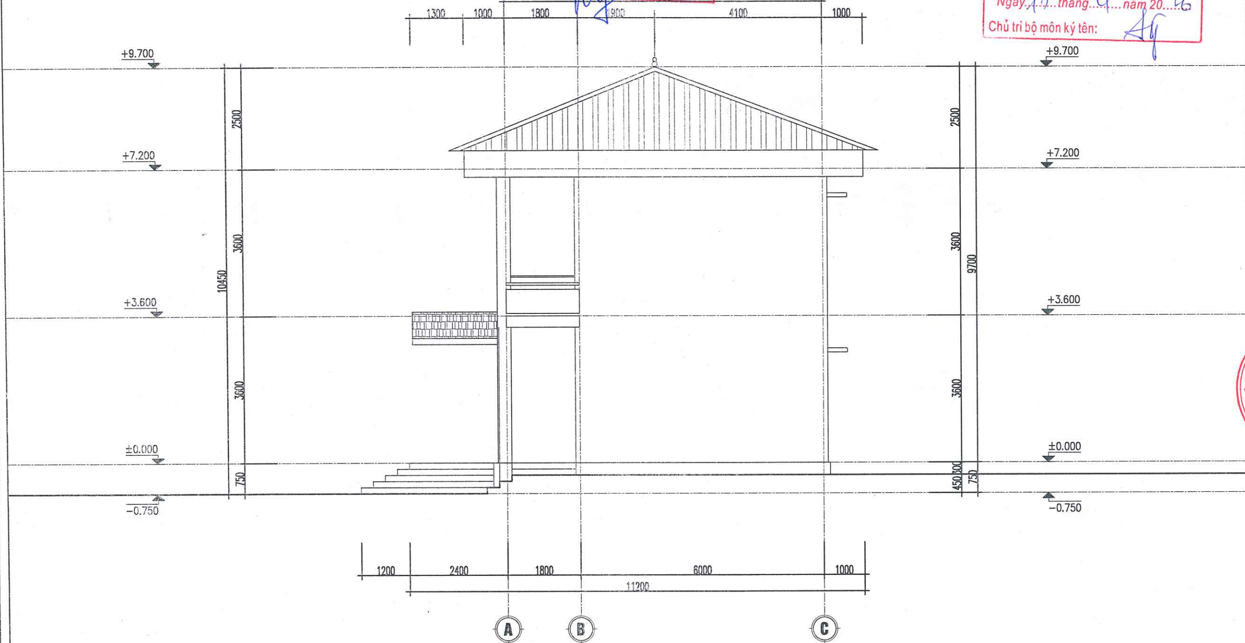
MẶT ĐỨNG HIỆN TRẠNG TRỤC A-C
