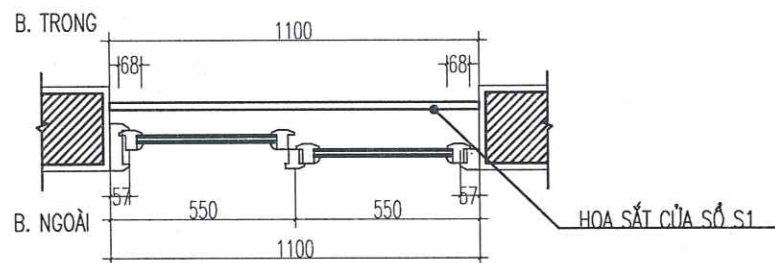
CẮT 2-2 CHI TIẾT CỬA SỔ S1 (LÀM MỚI) (SL :27 BỘ)
