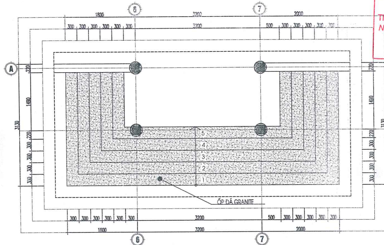
MẶT BẰNG SẢNH CHÍNH
