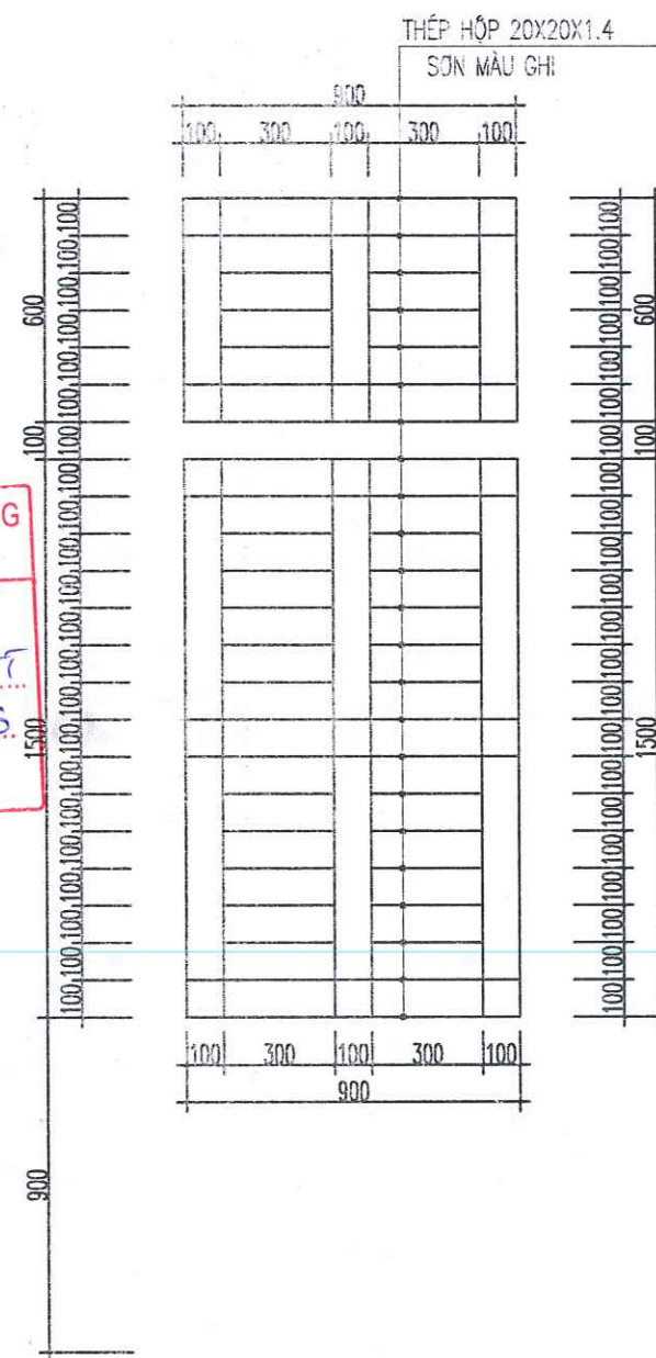
HOA HOA SẮT SỔ S2 (HIỆN TRẠNG) (SL :02 BỘ )
