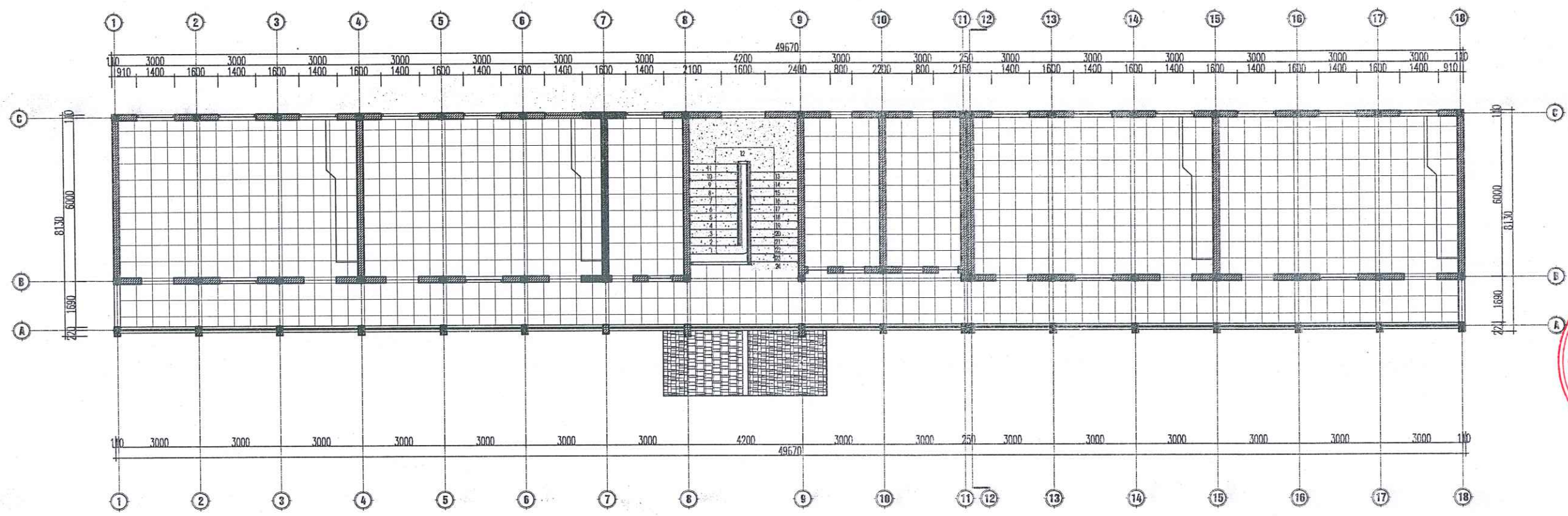
MẶT BẰNG LÁT SÀN CẢI TẠO TẦNG 2
