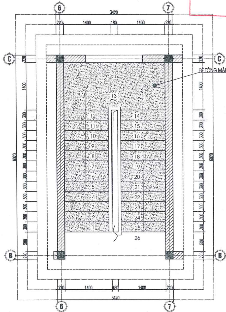
MẶT BẰNG THANG HIỆN TRẠNG
