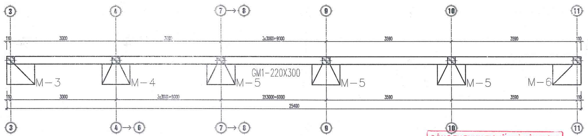
MẶT BẰNG MÓNG TƯỜNG RÀO ĐOẠN A-B
