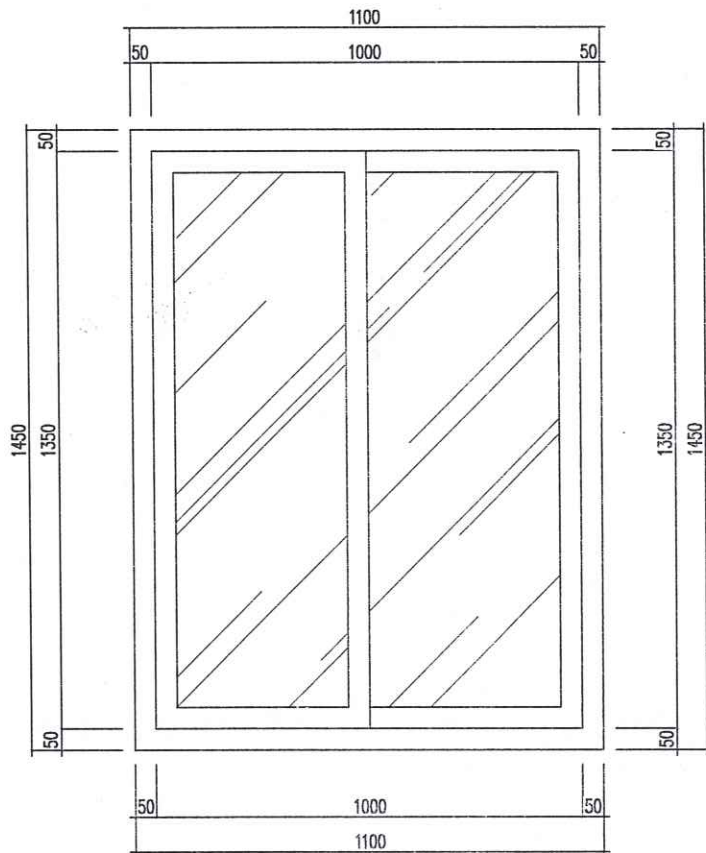
CỬA SỔ S2 CHUNG LOẠI: CỬA NHÔM KÍNH, SL: 02 BỘ
