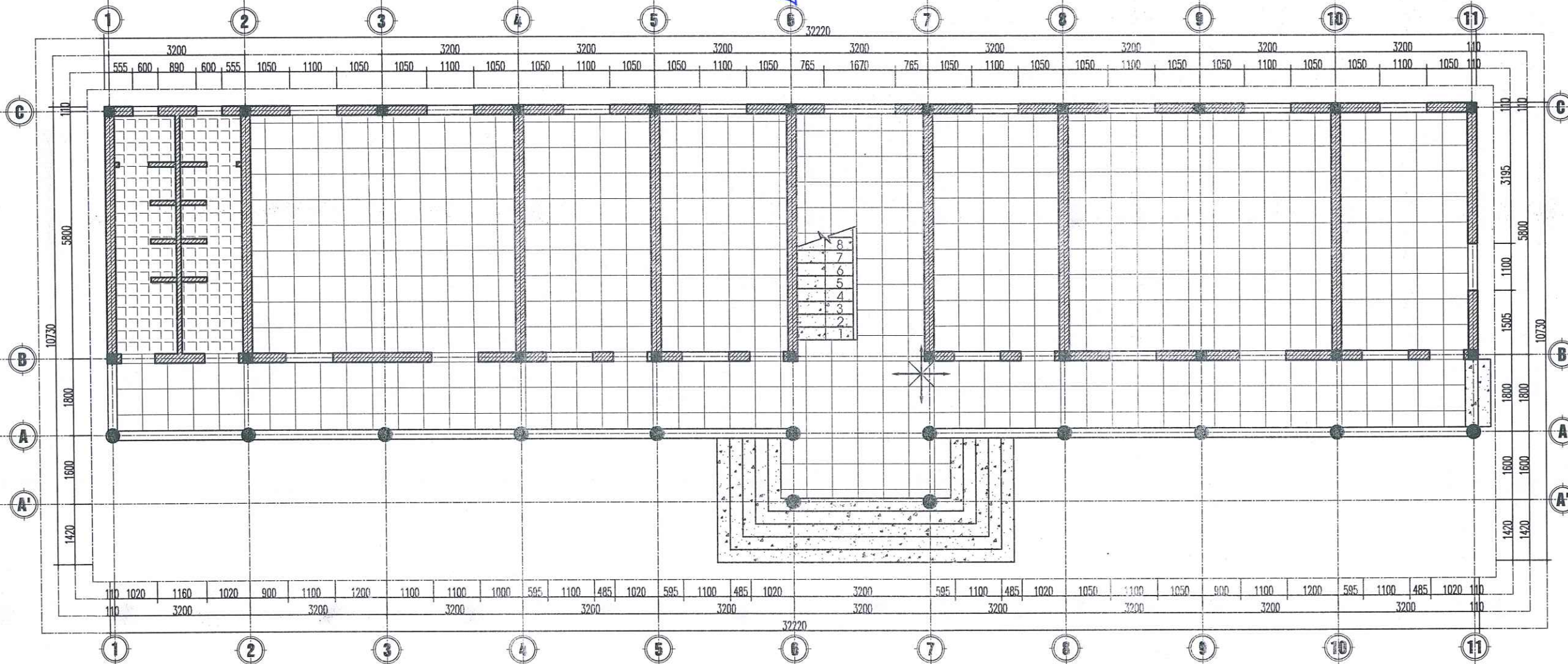
MẶT BẰNG LÁT SÀN TẦNG 1 CẢI TẠO
