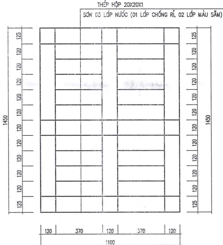
HOA SẮT CỬA SỔ S2 SL: 02 BỘ
