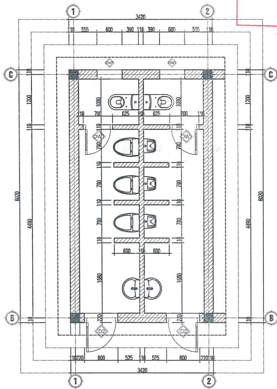
MẶT BẰNG WC TẦNG 1 + TẦNG 2 HIỆN TRẠNG
