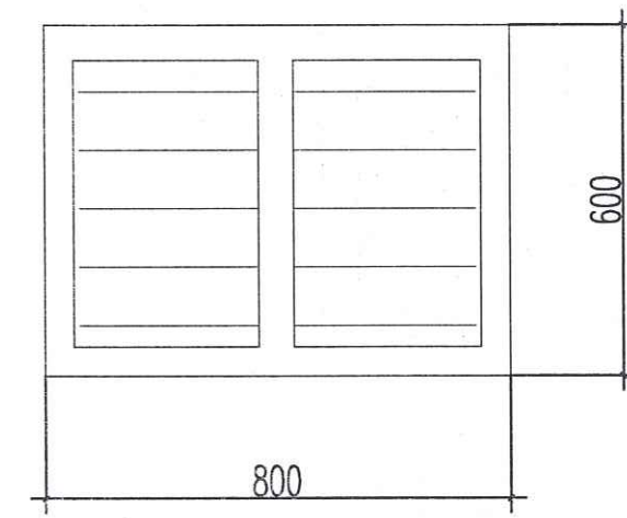
CỬA SỔ SW(SL:8 BỘ)
