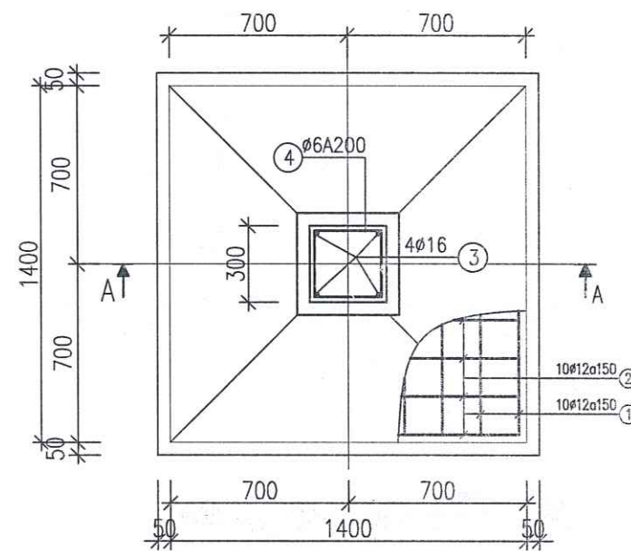
MÓNG M-1 (SL: 02)
