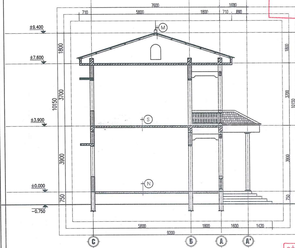
MẶT CẮT 1-1 CẢI TẠO
