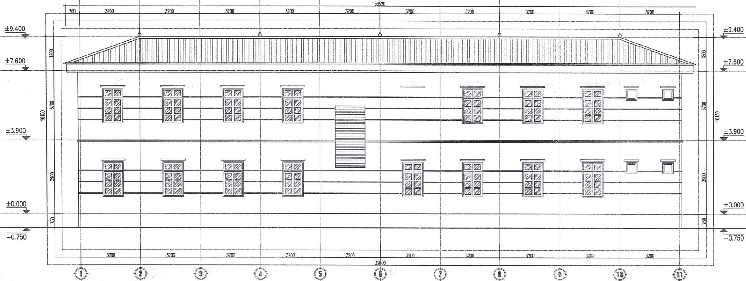
MẶT ĐỨNG TRỤC 1-11 HIỆN TRẠNG
