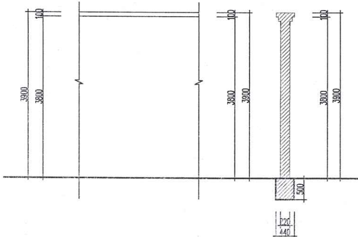
ĐOẠN TƯỜNG RÀO HIỆN TRẠNG (PHÁ DỠ) ĐOẠN D-E (L=10500MM) MẶT CẮT 1-1
