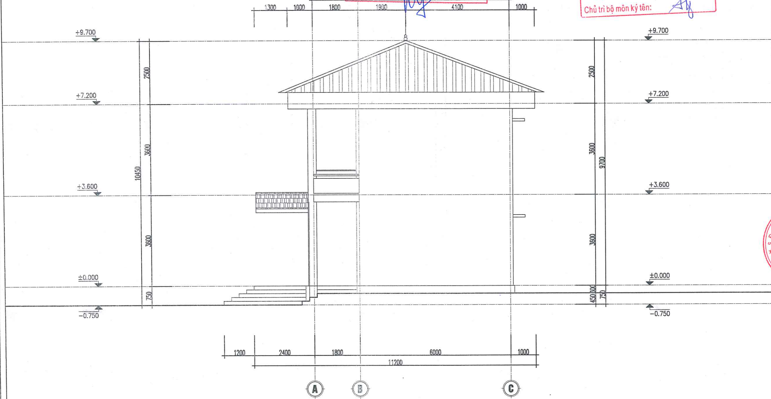
MẶT ĐỨNG TRỤC A-C CẢI TẠO
