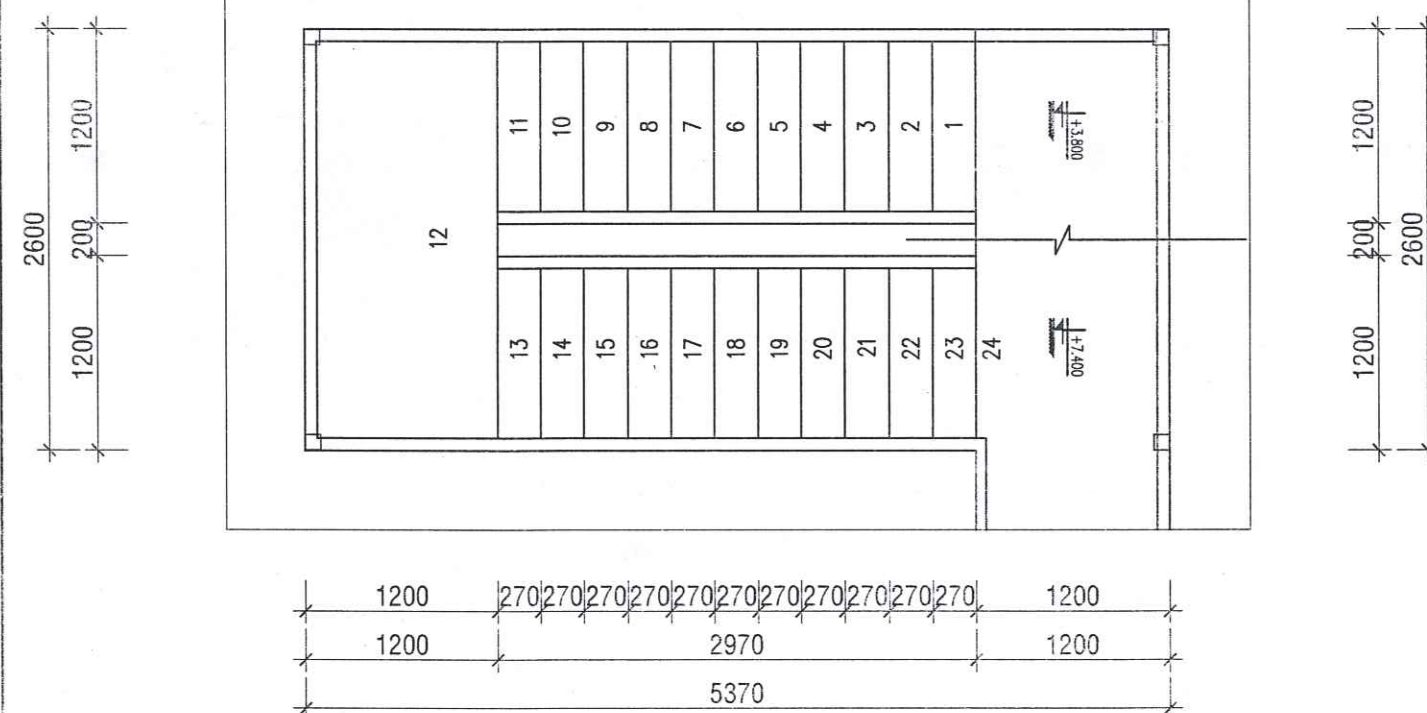
MẶT BẰNG CẦU THANG T.2-T.3 CÔNG TRÌNH
