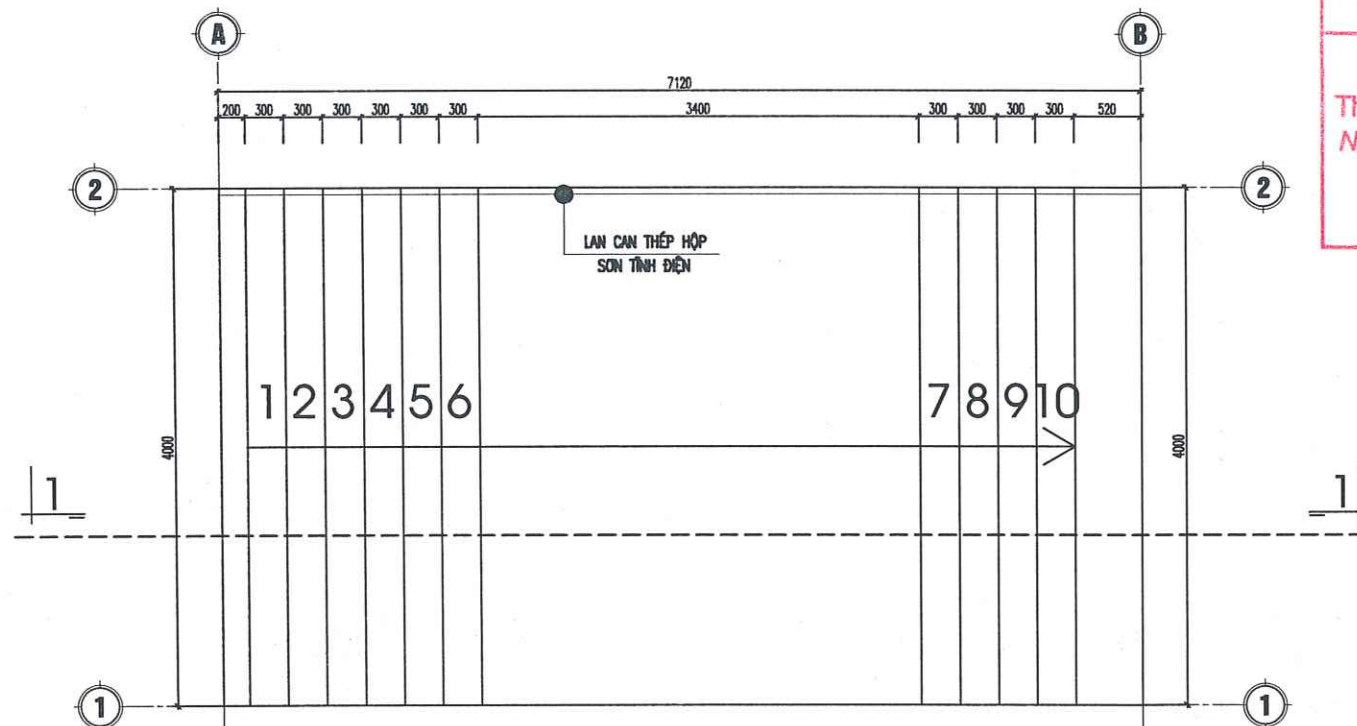
MẶT BẰNG BẬC THANG SỐ 1
