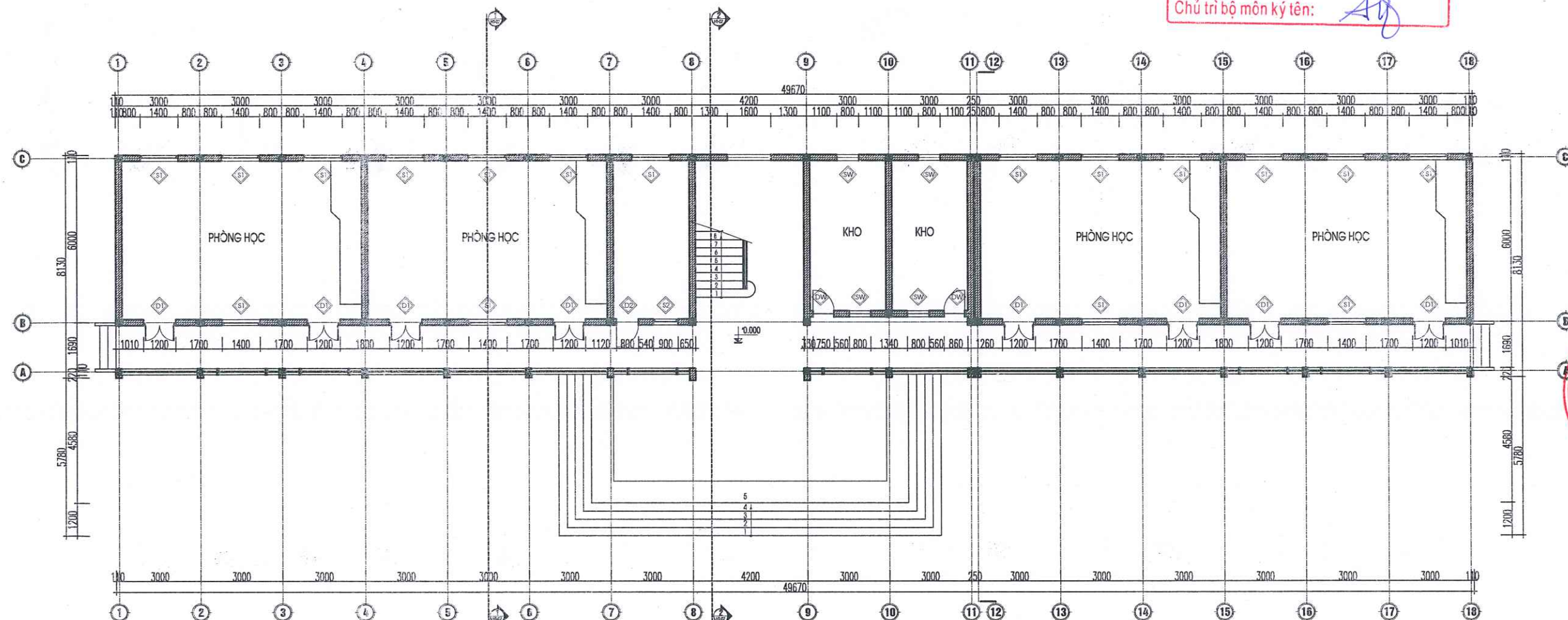
MẶT BẰNG CẢI TẠO TẦNG 1
