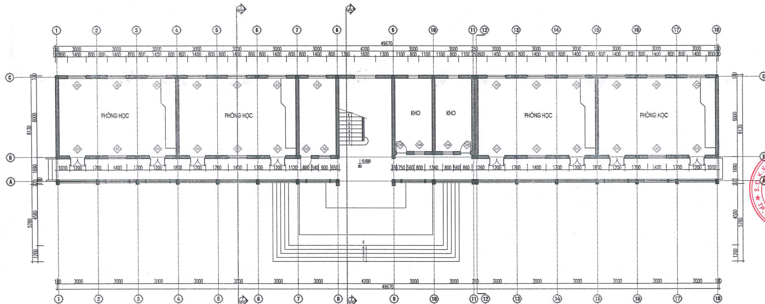
MẶT BẰNG HIỆN TRẠNG TẦNG 1
