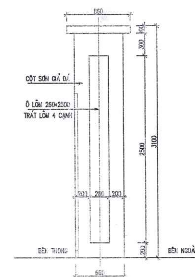
TRỤ CỔNG CHÍNH (SL: 02)
