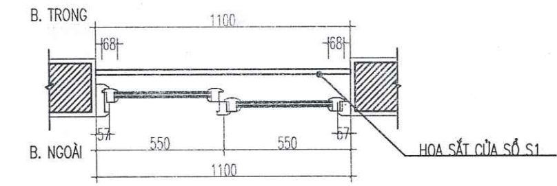
CHI TIẾT CỬA SỐ S2 (LÀM MỚI) (SL :02 BỘ )
