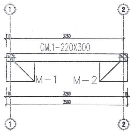
MẶT BẰNG MÓNG TƯỜNG RÀO ĐOẠN A-B
