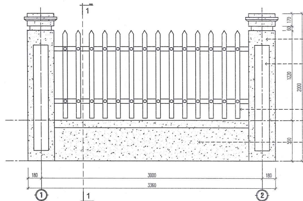
MẶT ĐỨNG CHI TIẾT ĐIỂN HÌNH TƯỜNG RÀO ĐOẠN D-B L=4 M
