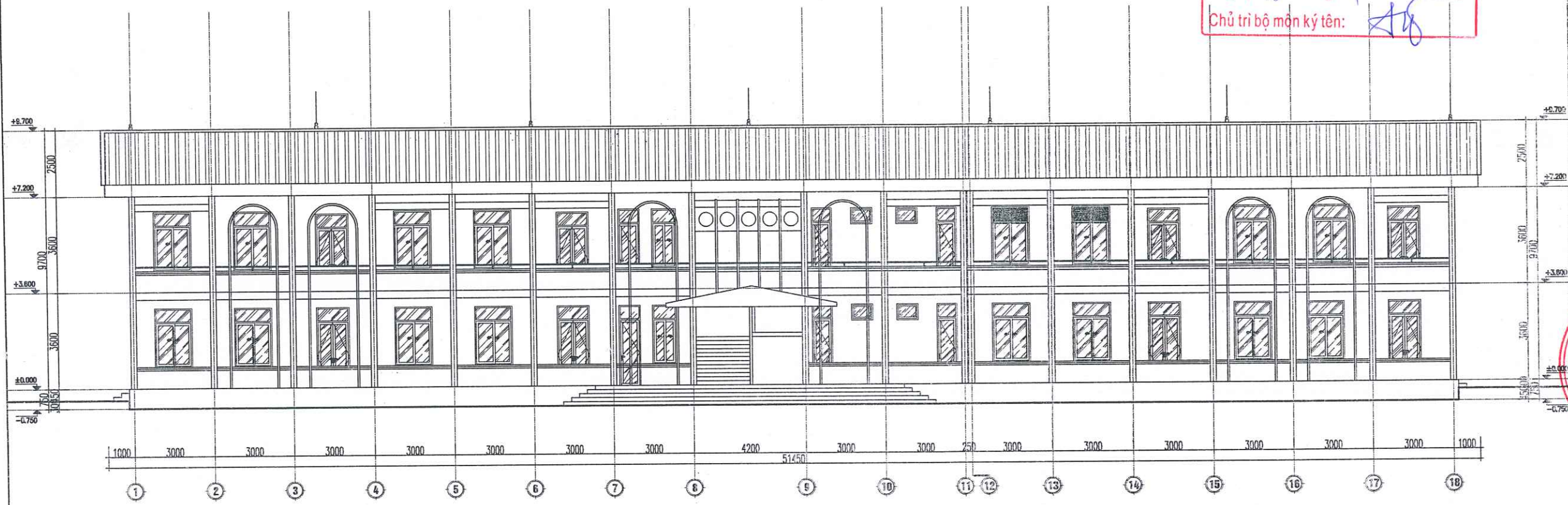
MẶT ĐỨNG CẢI TẠO TRỤC 1-18
