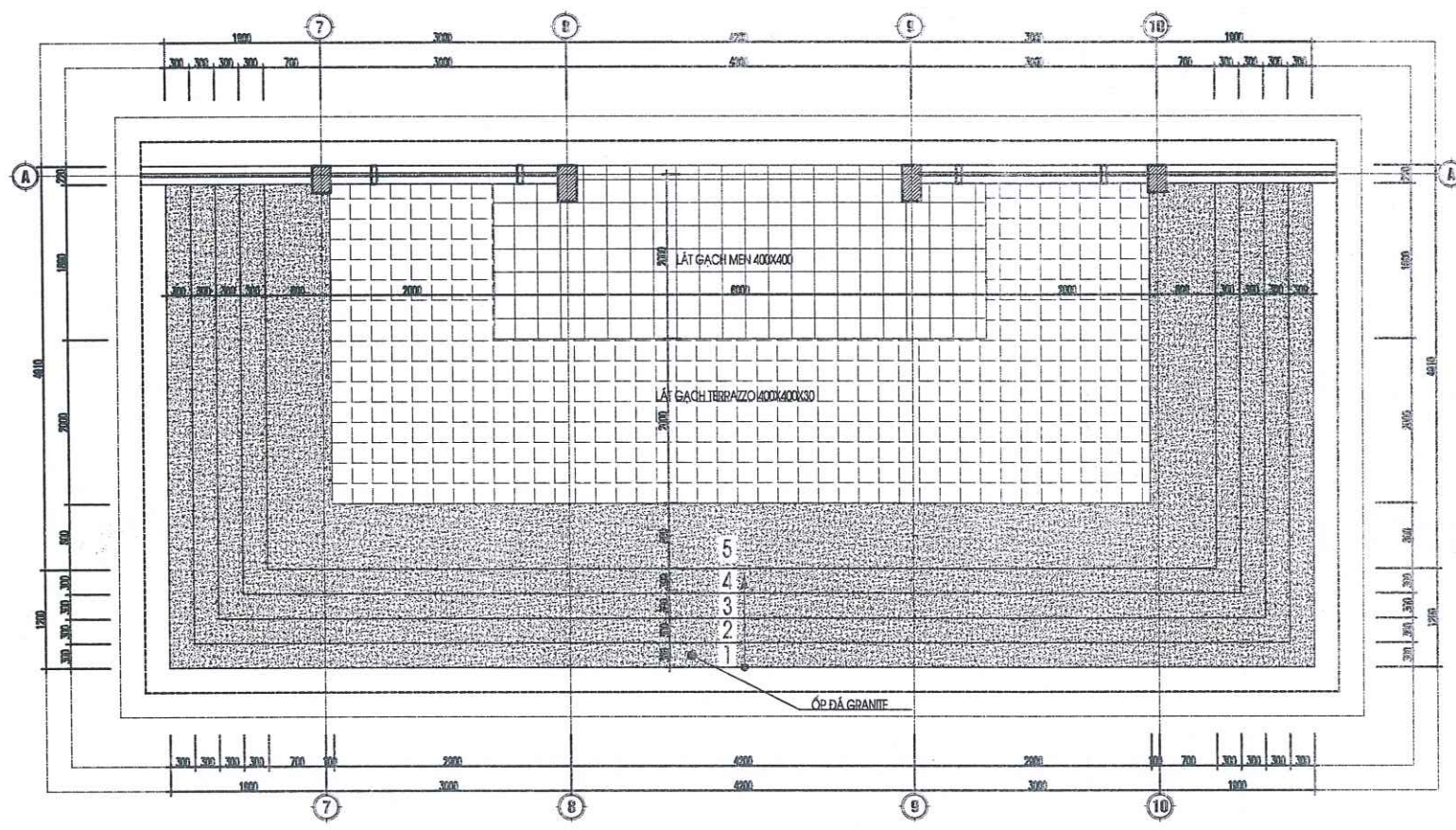
MẶT BẰNG HIỆN TRẠNG SẢNH CHÍNH
