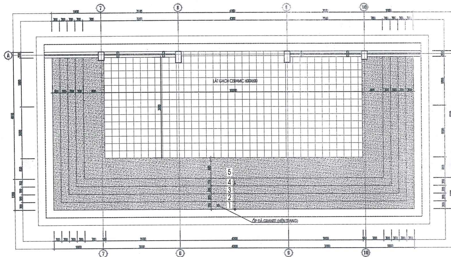
MẶT BẰNG SẴN CHÍNH CẢI TẠO
