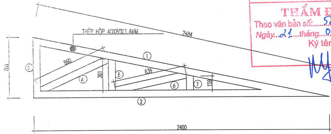
VÌ KÈO VK-1 (SL=02CK)
