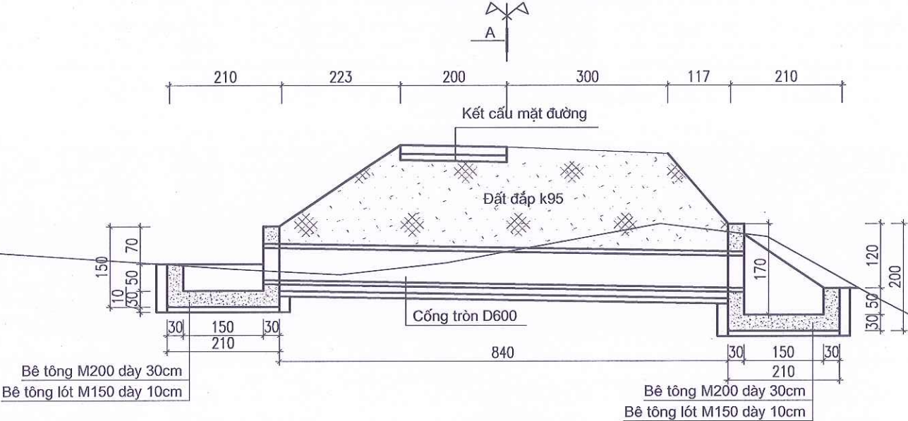
CẮT DỌC CỐNG TIÊU (1/100)
