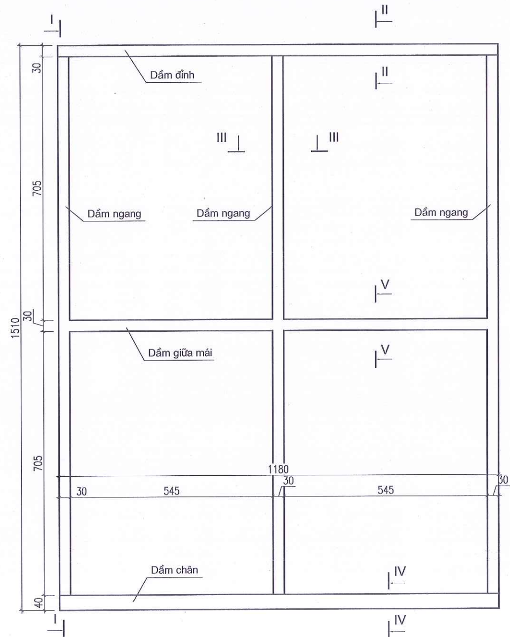
MẶT BẰNG KHUNG DẦM GIA CỐ MÁI ĐẬP (1/100)
