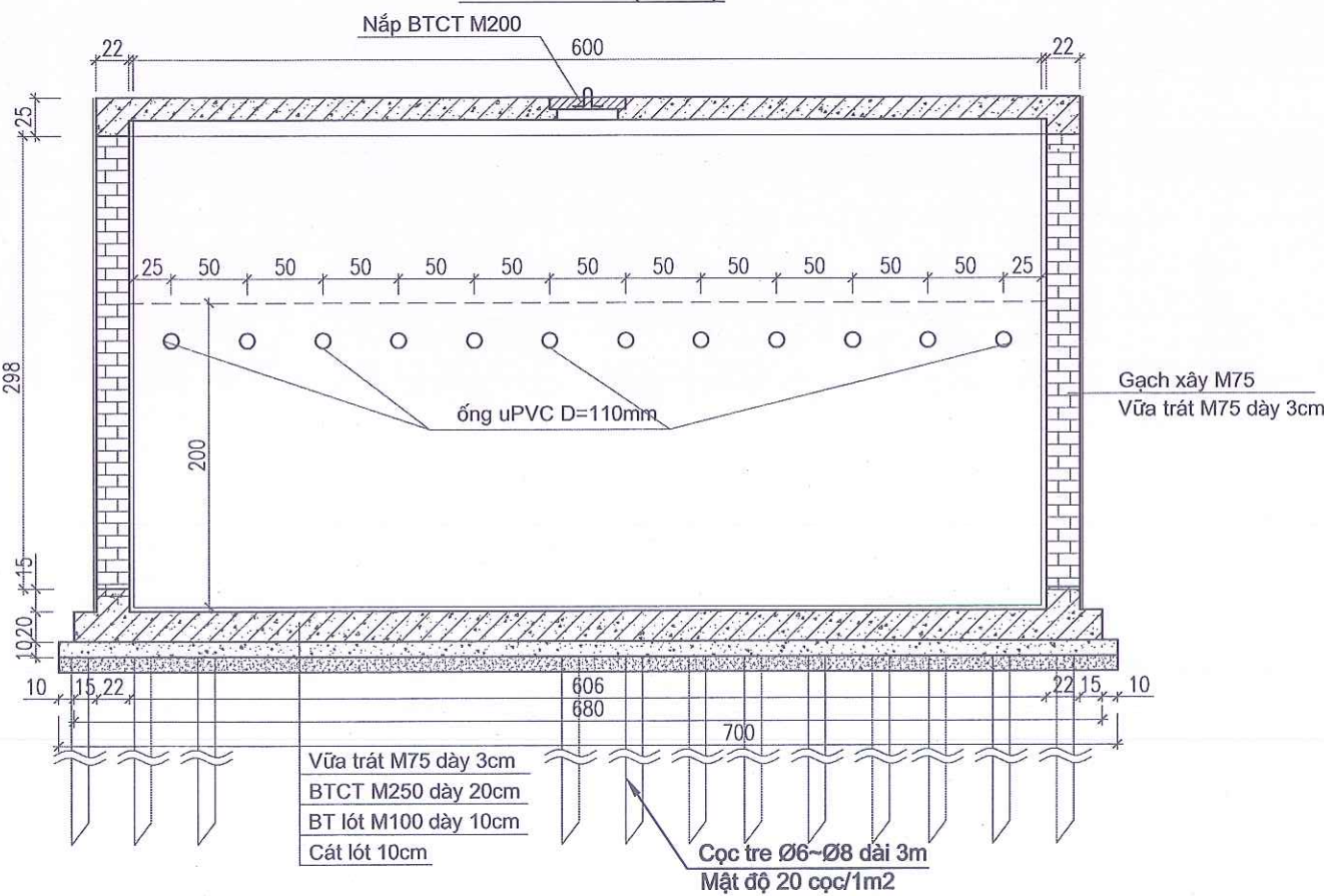
CẮT 3 - 3 (1/50)
