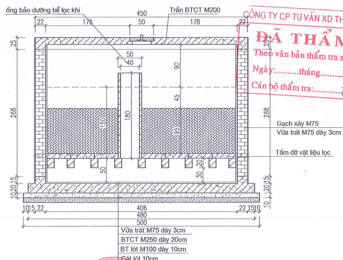
CẮT 7 - 7 (1/50)
