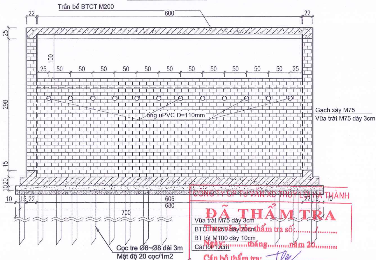
CẮT 4 - 4 (1/50)
