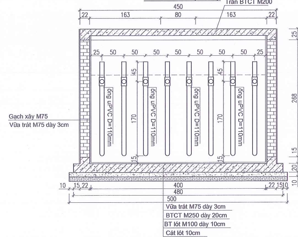
CẮT 4 - 4 (1/50)
