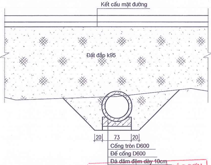
CẮT NGANG CỐNG TIÊU (1/50)
