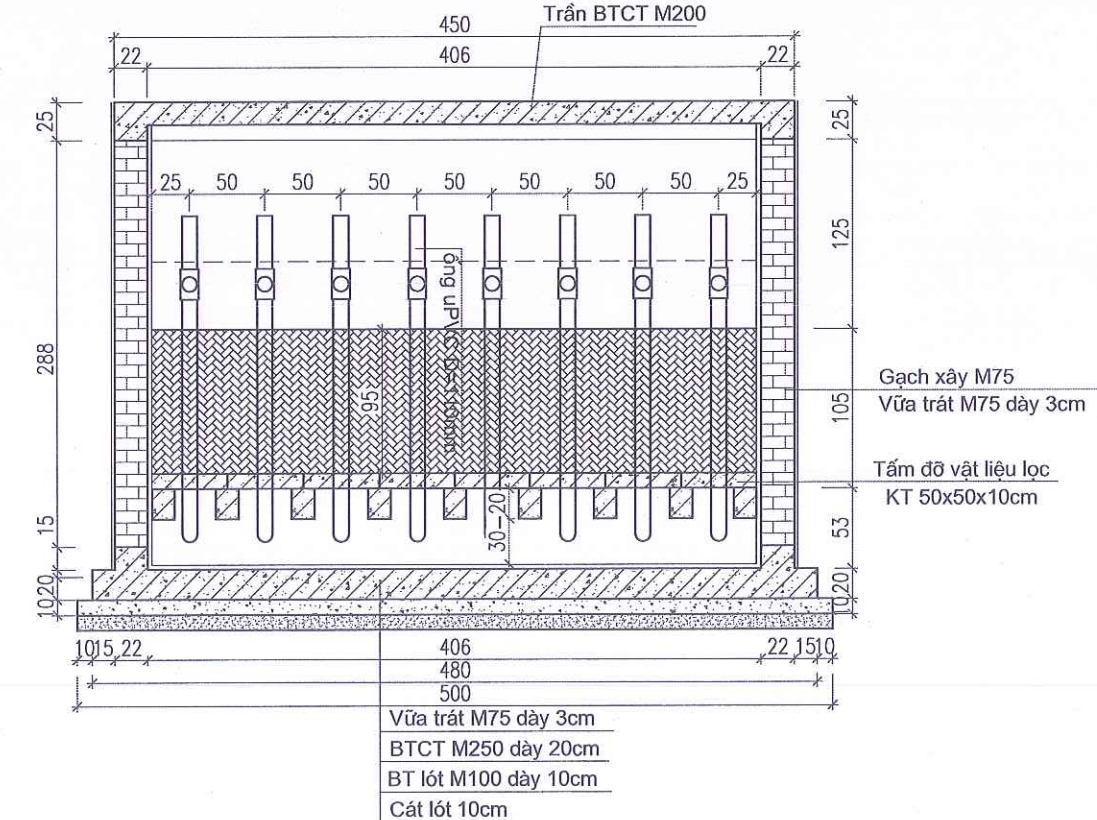
CẮT 6 - 6 (1/50)
