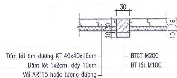
MẶT CẮT A-A (1/50)
