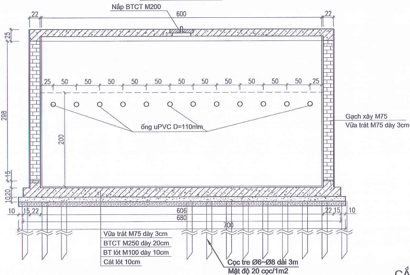
CẮT 5 - 5 (1/50)
