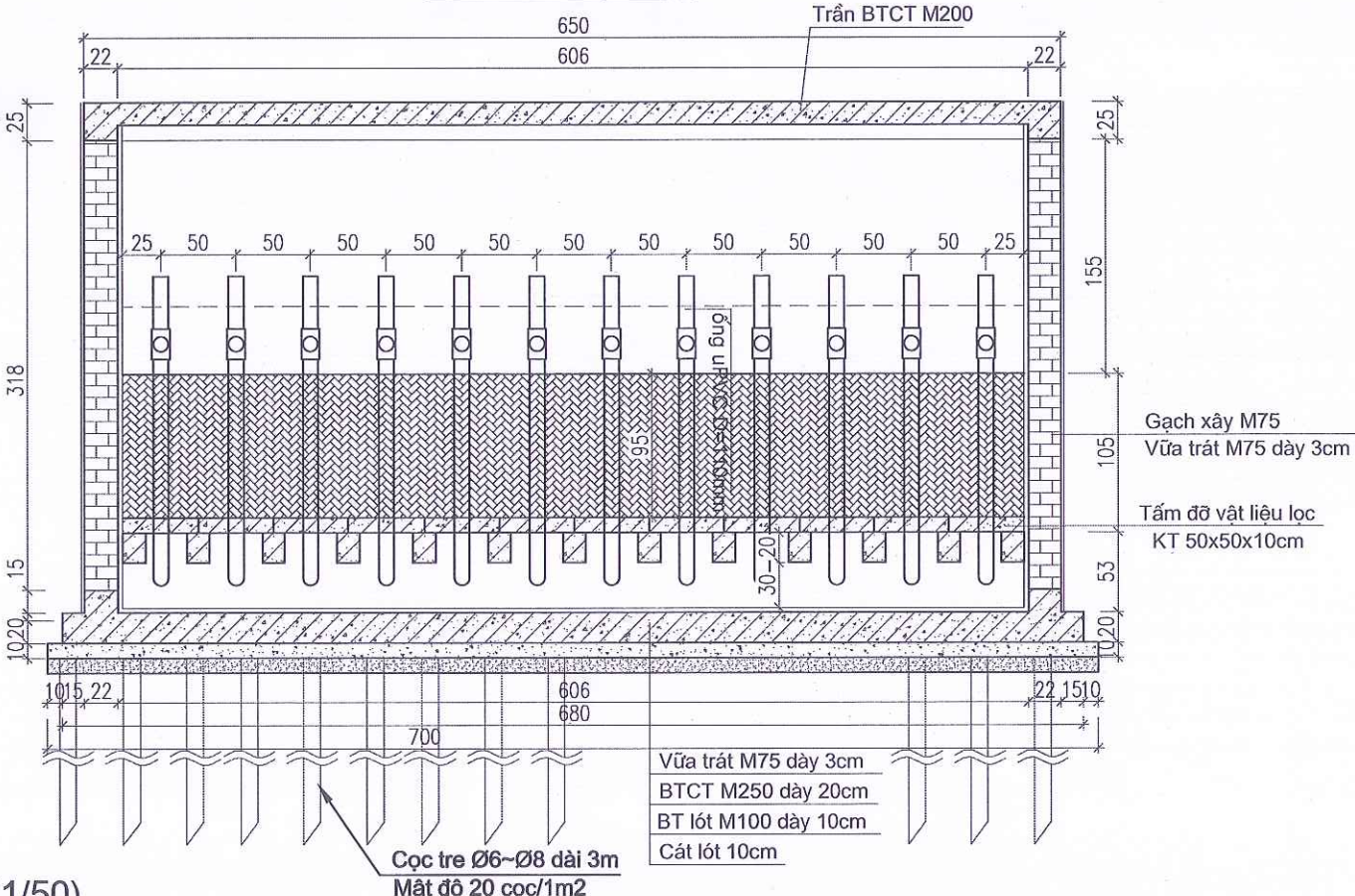
CẮT 6 - 6 (1/50)
