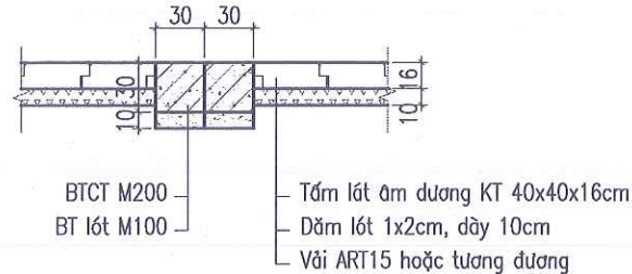
MẶT CẮT B-B (1/50)
