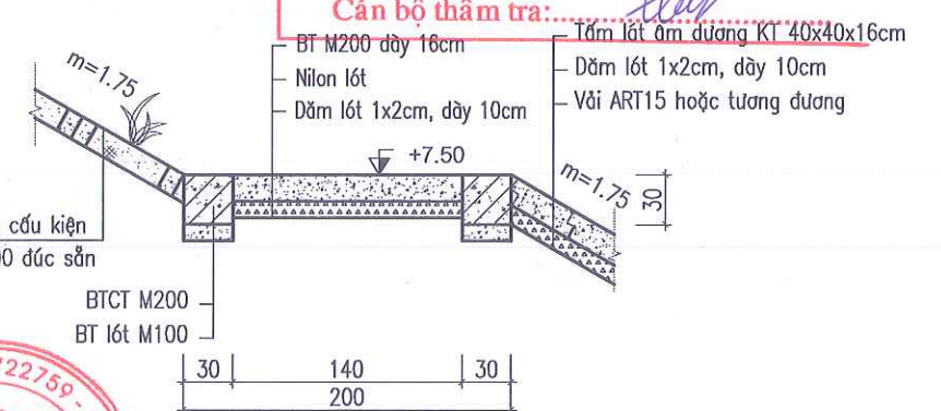
MẶT CẮT C-C (1/50)
