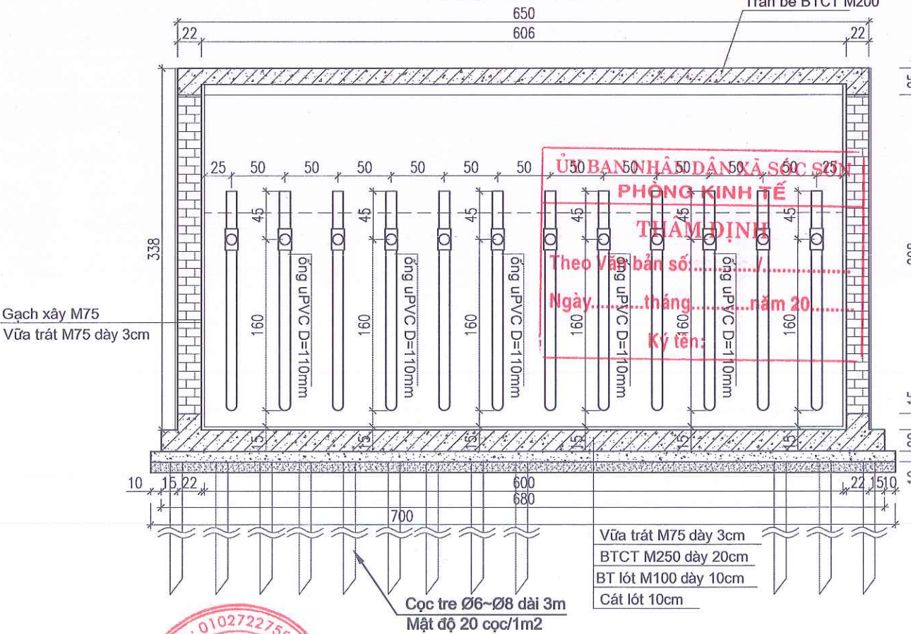
CẮT 4 - 4 (1/50)
