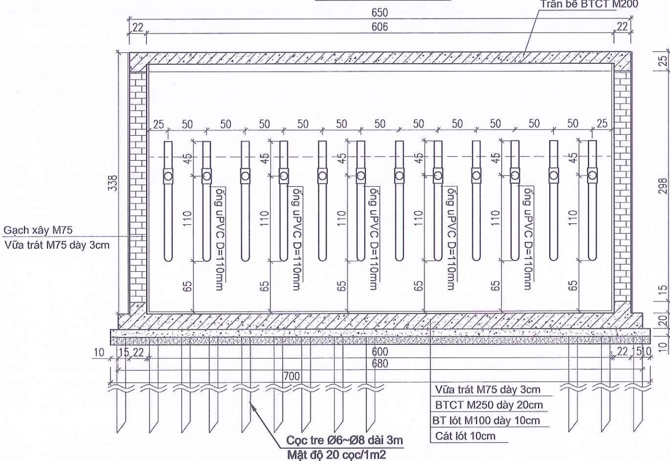
CẮT 3 - 3 (1/50)
