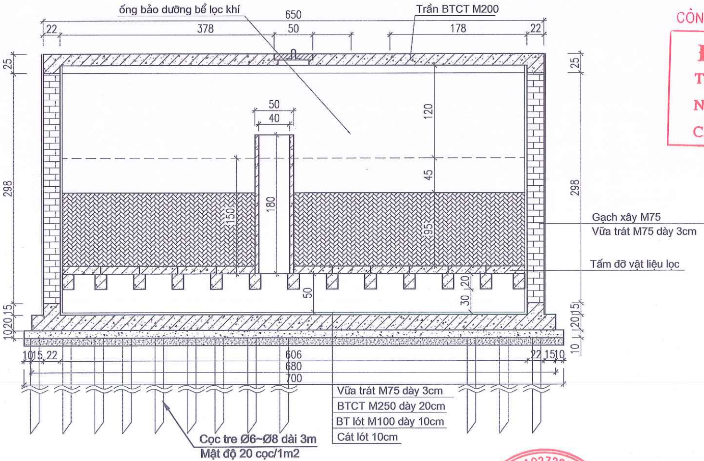
CẮT 7 - 7 (1/50)
