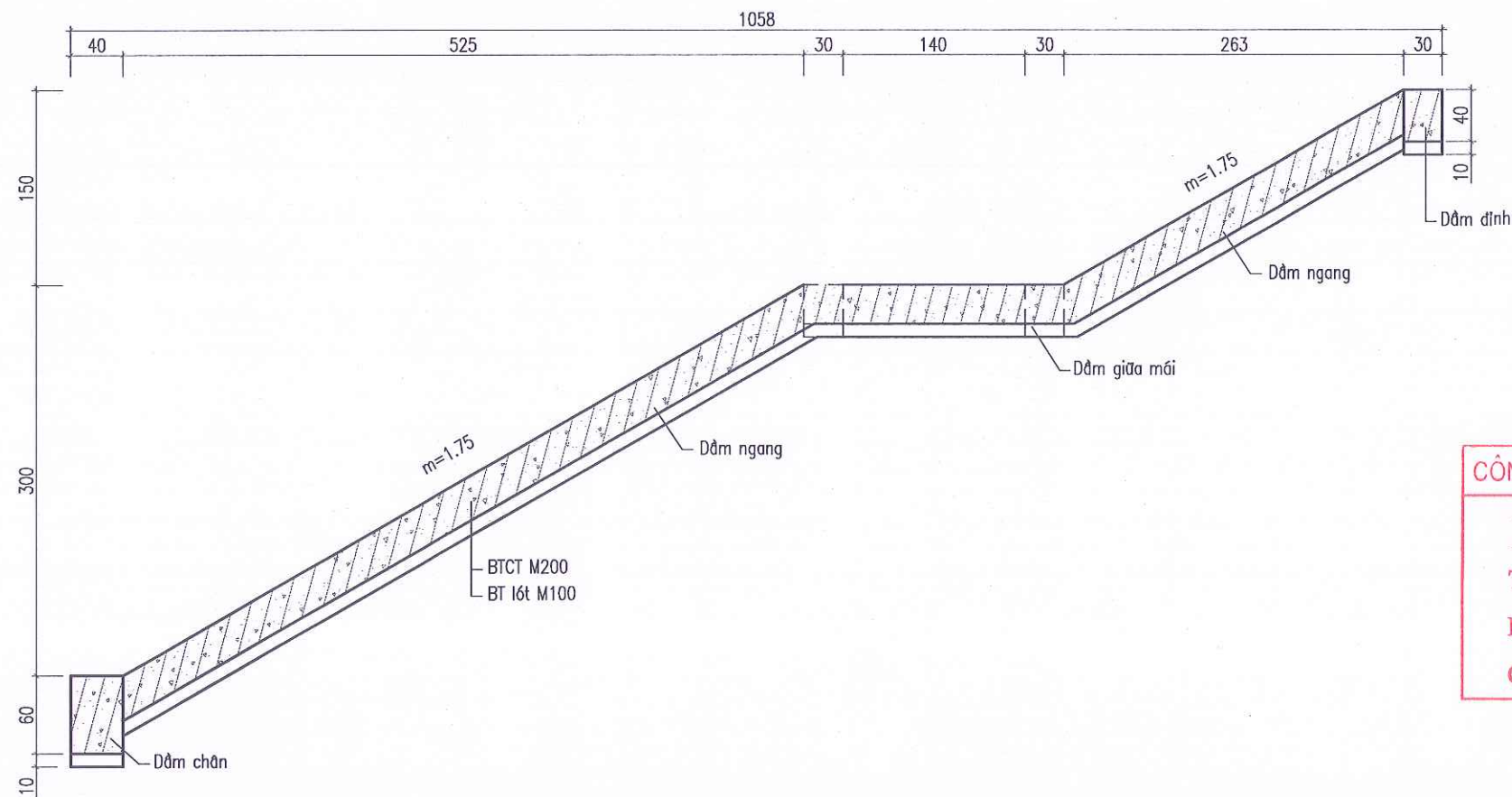
CẮT I - I (1/50)
