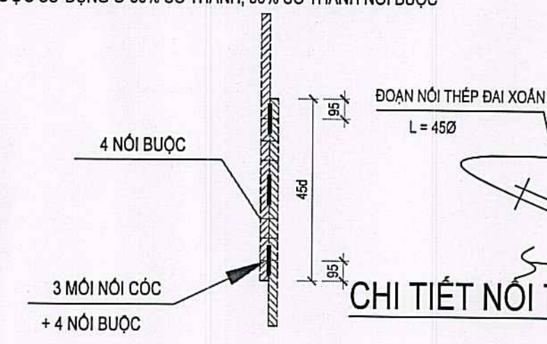
CHI TIẾT NỐI CỐC NỐI 2 LÔNG THÉP
