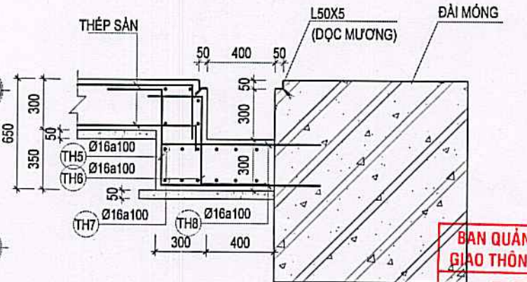
MC 2-2 (ÁP DỤNG MƯƠNG NƯỚC) TỶ LỆ: 1:25
