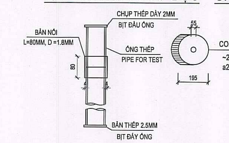
CHI TIẾT ỚNG TN
