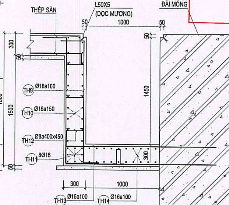
MC 3-3 (ÁP DỤNG HỒ GÀ) TỶ LỆ: 1:25
