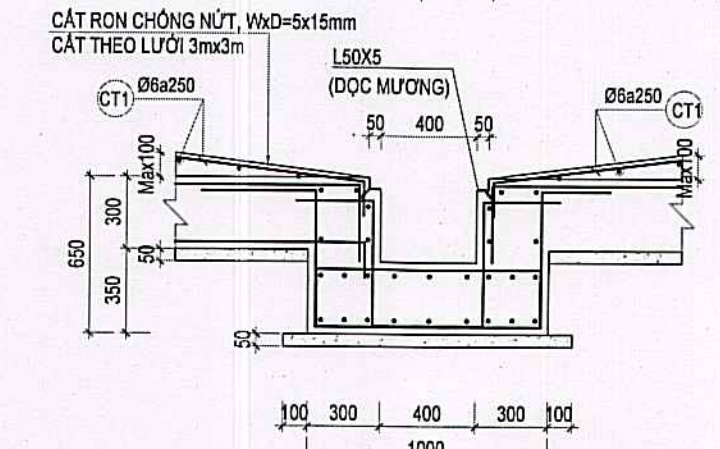
CÁI TẠO THÉP CHỐNG NỨT CHO LỚP TẠO DỐC HOÀN THIỆN TỶ LỆ: 1:25
