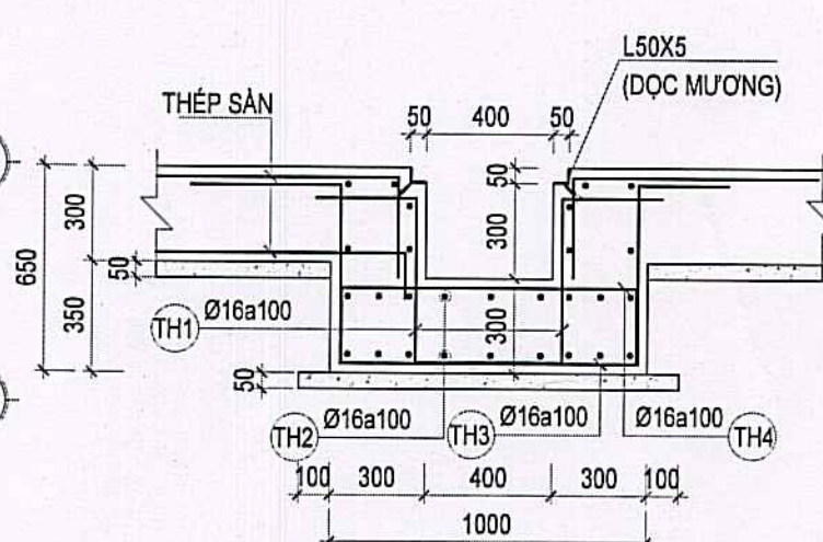
MC 1-1 (ÁP DỤNG MƯƠNG NƯỚC) TỶ LỆ: 1:25
