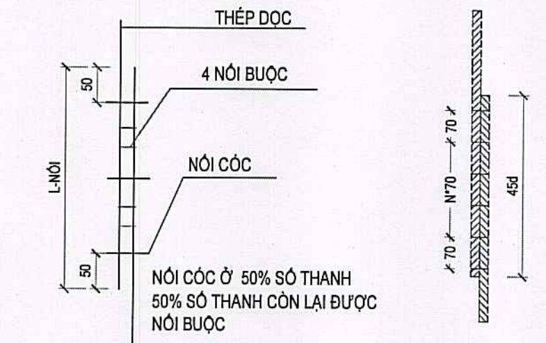
CHÚ Ý: CÁN CỨ THỰC TẾ THI CÔNG, NHÀ THẦU CẦN ĐẢM BẢO LÔNG THÉP KHÔNG BỊ TỤT TRONG QUÁ TRÌNH THI CÔNG CỌC
