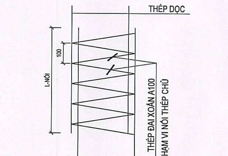
QUI CÁCH THÉP ĐAI VỊ TRÍ NỐI THÉP DỌC
