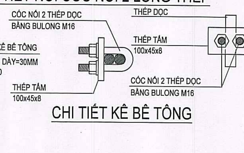
CHI TIẾT KÊ BÊ TÔNG
