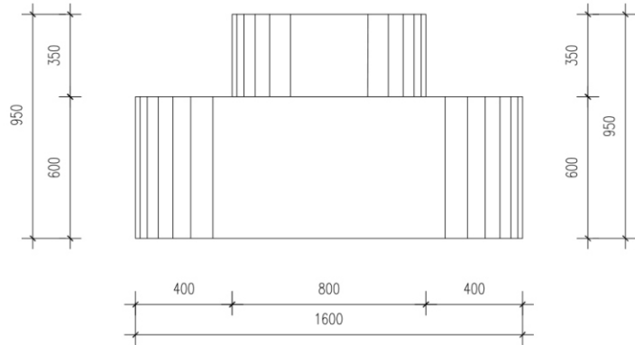
MẶT ĐỨNG BỤC A4
