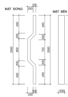
CHI TIẾT CỘT 4
