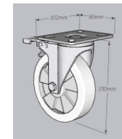
Kích thước bánh xe Số lượng: 16 chiếc (8 chiếc/1 bên)
