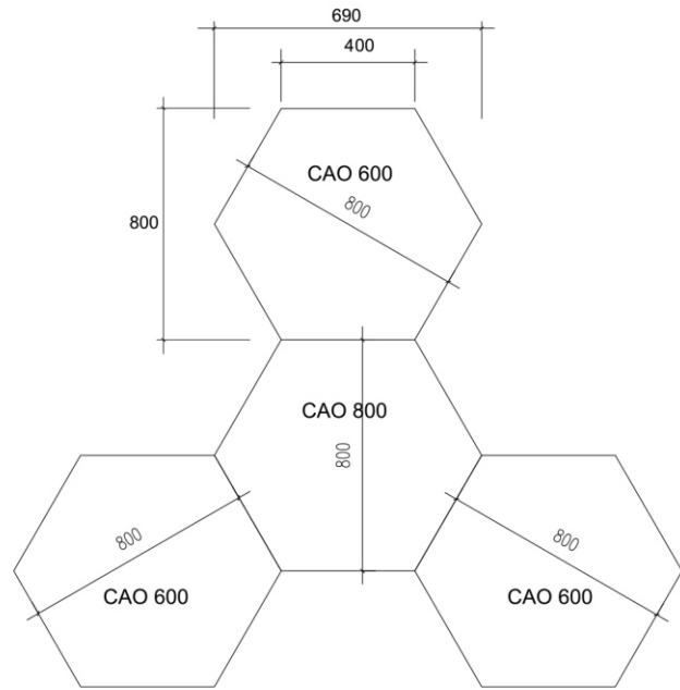
CHI TIẾT BUC A5
