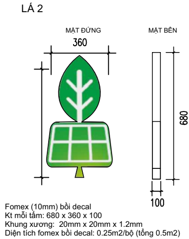
PIN NĂNG LƯỢNG
