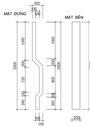
CHI TIẾT CỘT 3
