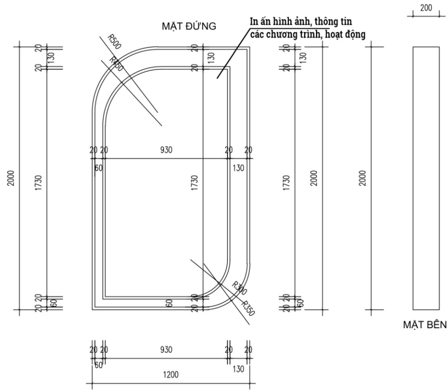
CHI TIẾT BỤC P
