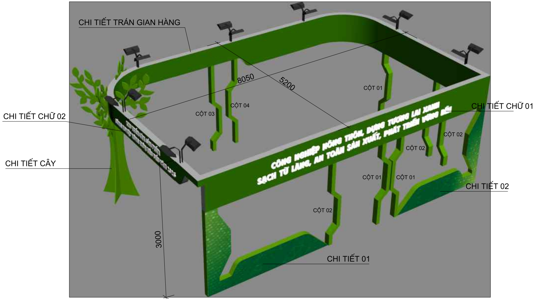
CHI TIẾT TC01 + TC02 (LƯU Ý: TC02 ĐỐI XỨNG TC01)
