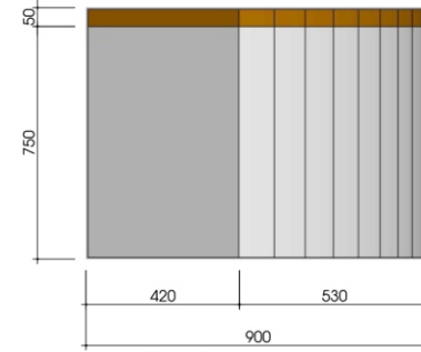
MẶT BÊN BỤC C2
