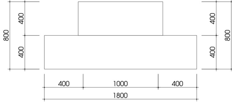
MẶT ĐỨNG BỤC A1
