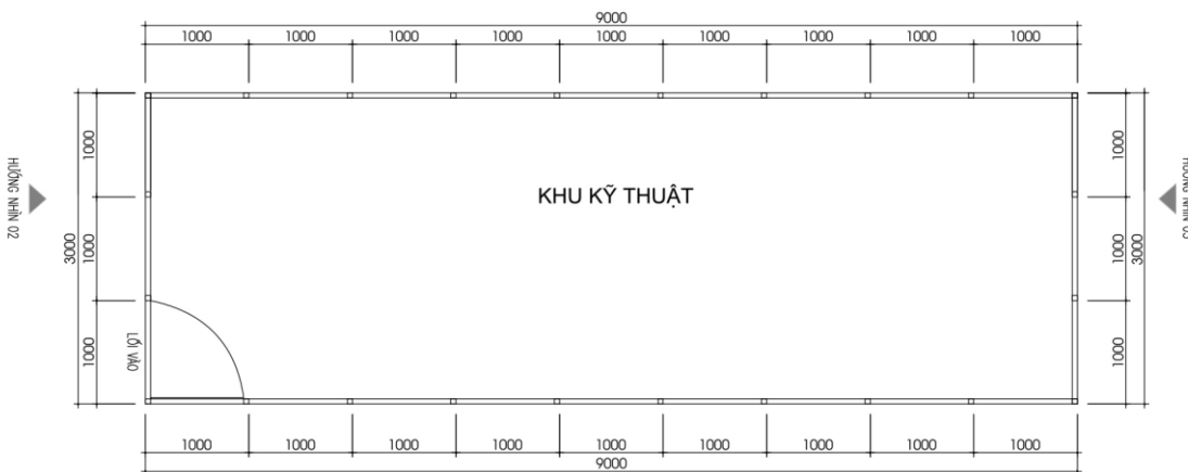
MẶT BẰNG CHI TIẾT KHU KỸ THUẬT (HỆ VÁCH CADIVI)
