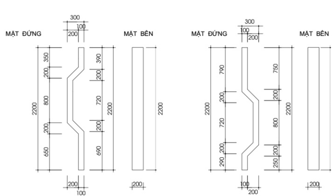
CHI TIẾT CỘT 1
