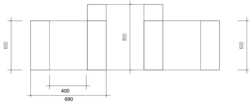
MẪU CHI TIẾT BỤC A5
