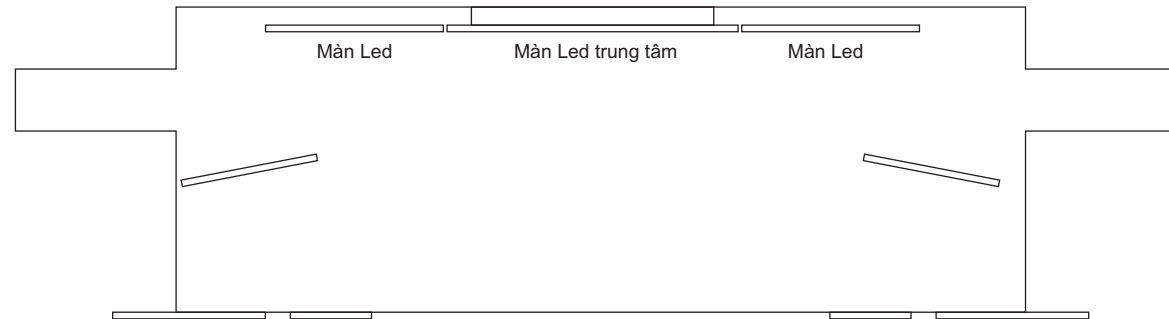
SƠ ĐỒ BỐ TRÍ CÁC HẠNG MỤC TRÊN SÂN KHẤU
