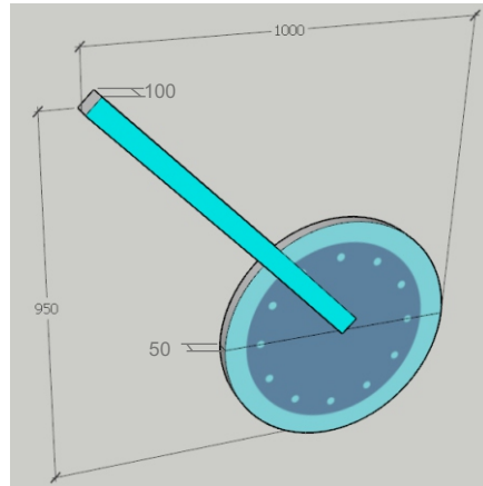
HỌA TIẾT TRUNG TÂM VÁCH TRÒN BÊN PHẢI
