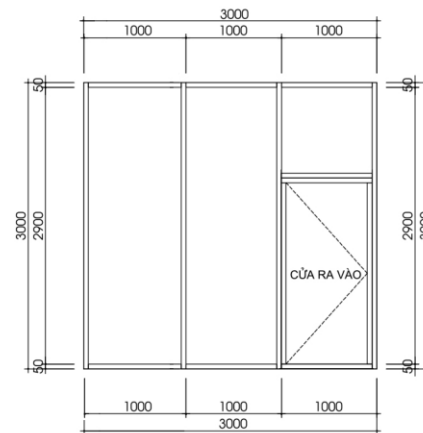
MẶT ĐỨNG CHI TIẾT KHU KỸ THUẬT HƯỚNG NHÌN 02
