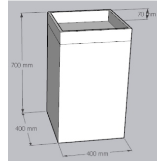
Kích thước bục gỗ
