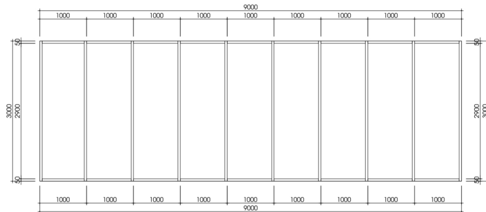
MẶT ĐỨNG CHI TIẾT KHU KỸ THUẬT HƯỚNG NHÌN 01
