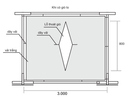
PHƯƠNG ÁN THI CÔNG HÀNG RÀO
