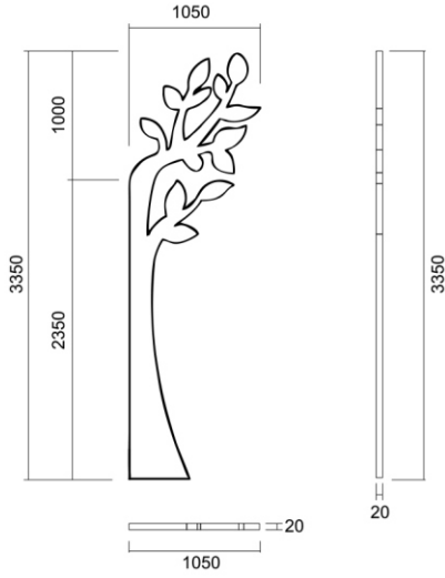
CHI TIẾT 1 VẼ CÂY
