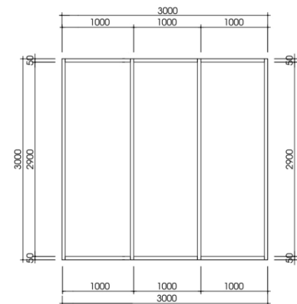
MẶT ĐỨNG CHI TIẾT KHU KỸ THUẬT HƯỚNG NHÌN 03
