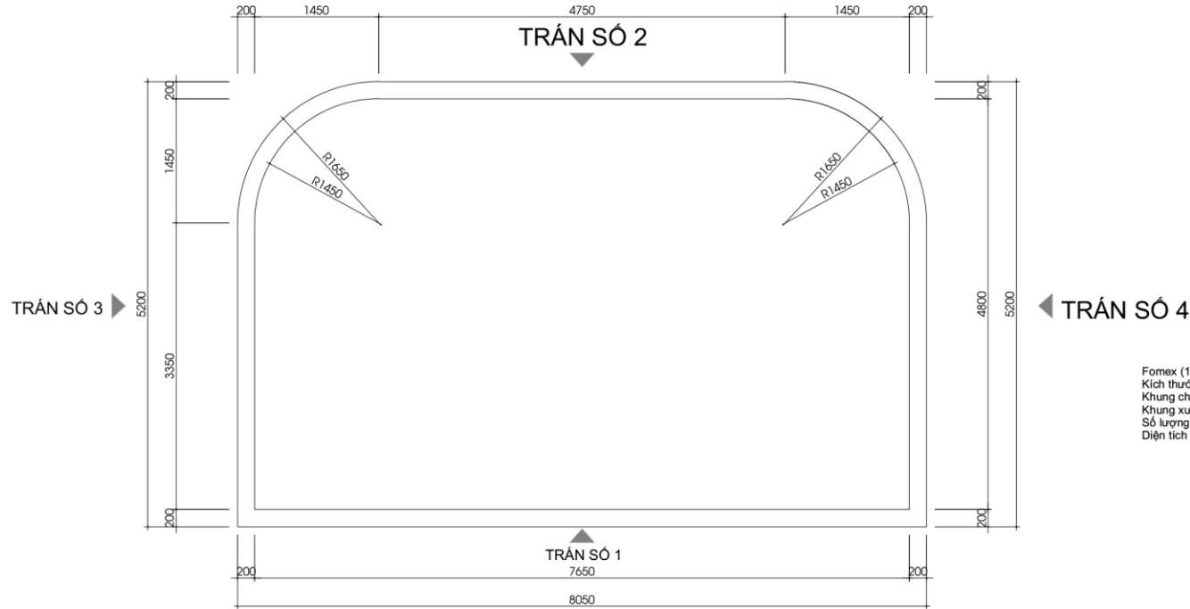
CHI TIẾT TRẦN GIAN HÀNG
