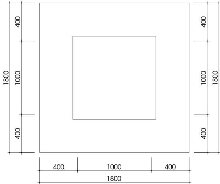
CHI TIẾT BỤC A1
