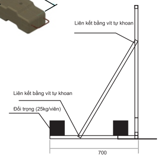
Hình ảnh đối trọng
