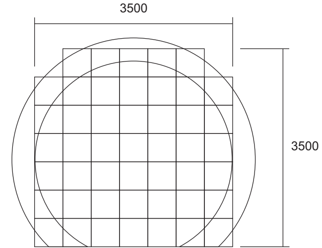
Sơ đồ bố trí led màn led trung tâm, Diện tích led 47 ca-bin x 0.25m = 11.75m 2
