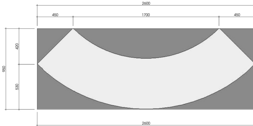
CHI TIẾT BỤC C2
