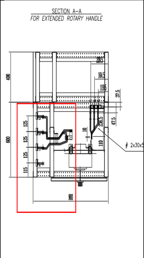
Thiết kế bố trí của các thanh cái trong tủ điện
