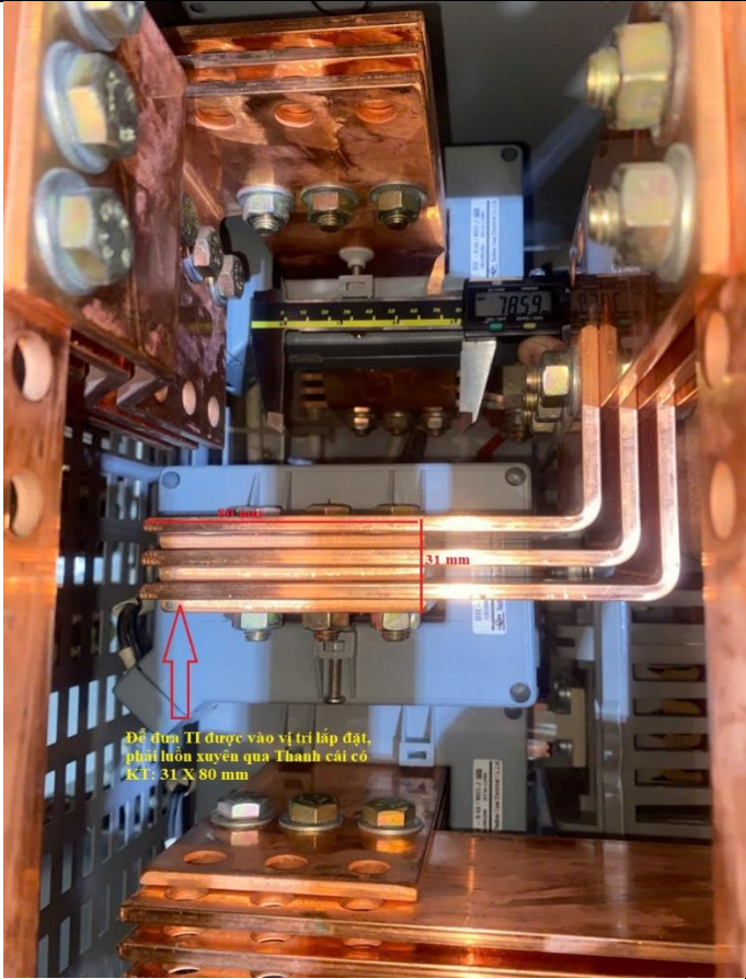
Bố trí lắp đặt của các máy biến dòng điện trong tủ điện phải luôn xuyên qua thanh cái
