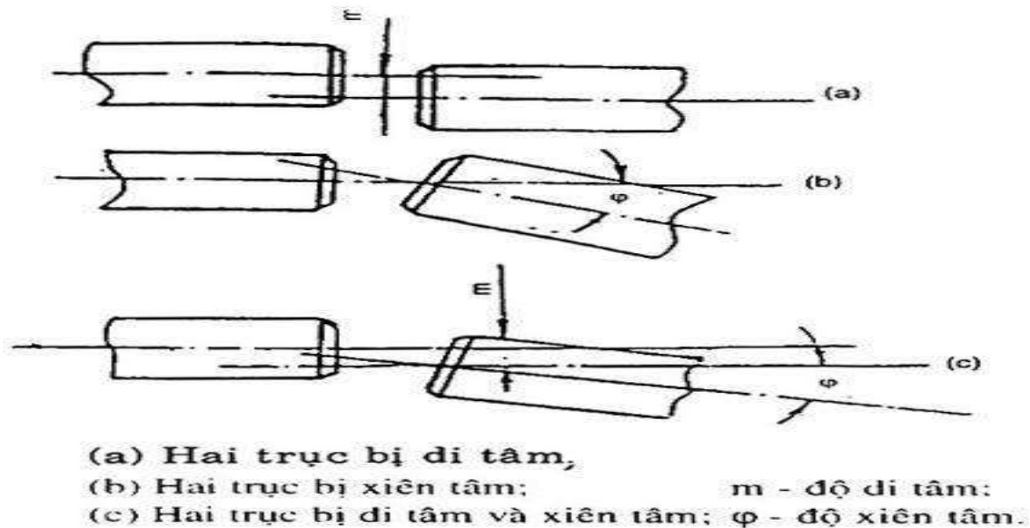
Hình 1 : Độ không đồng tâm của 2 trục
