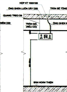
ĐÈN EXIT LOẠI HAI MẶT LOẠI CÓ MỖI TÊN 2 CHIỀU
