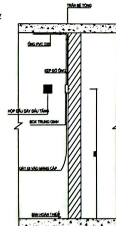
CHI TIẾT LẮP ĐẶT HỘP ĐẤY DÂY ĐẦU TẮNG
