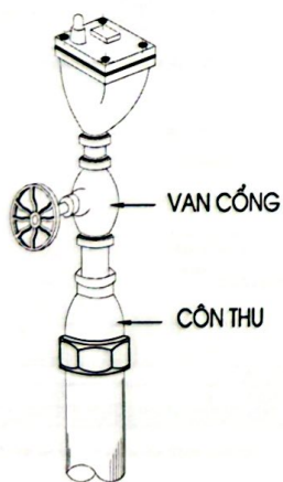
CHI TIẾT LẮP ĐẶT VAN XÁ KHÍ
