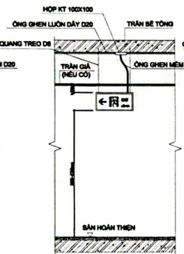
ĐÈN EXIT LOẠI HAI MẶT LOẠI CÓ MỖI TÊN CHỈ TRÁI
