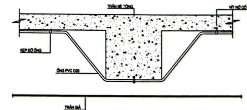
CHI TIẾT LẮP ĐẶT ỚNG QUA DẦM
