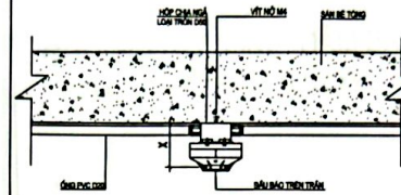
CHI TIẾT LẮP ĐẶT ĐẦU BẢO DƯỠI TRẦN BÊ TÔNG (ỐNG ĐI NỐI)
