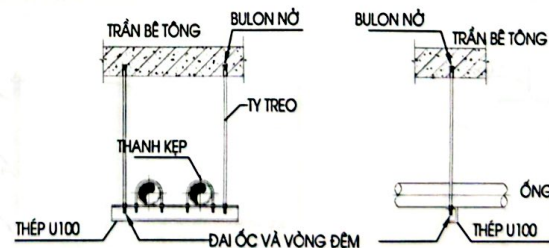
CHI TIẾT TREO ỚNG CHO 2 ỚNG DN80 TRỖ LÊN
