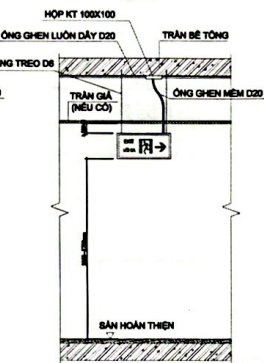
ĐÈN EXIT LOẠI HAI MẶT LOẠI CÓ MỖI TÊN CHỈ PHẢI
