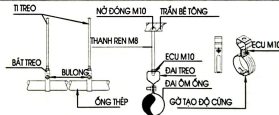
CHI TIẾT TREO ỚNG CHO 1 ỚNG DN80 TRỖ XƯỚNG
