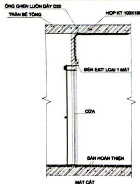
CỬA RA VÀO HOẶC CỬA THANG THOÁT HIỂM
