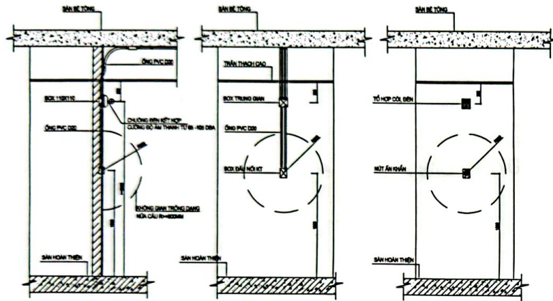
CHI TIẾT LẮP ĐẶT CHUÔNG ĐÈN NÚT ẮN KHẨN
