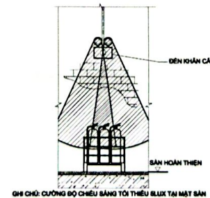
GHI CHÚ: CƯỜNG ĐỘ CHIẾU SÁNG TỐI THIỂU BLUX TÀI MẶT SÀN
