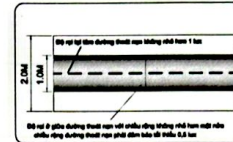
ĐỘ RỘNG CỦA CHIẾU SÁNG SỰ CỎ ĐƯỜNG THOÁT NẠN
