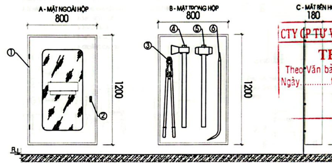
CHI TIẾT LẮP ĐẶT TỦ CHỮA DUNG CỤ PHÒNG CHÁY CHỮA CHÁY
