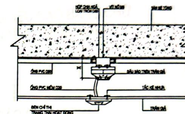
CHI TIẾT LẮP ĐẶT ĐẦU BÊN TRÊN TRẦN GIẢ
