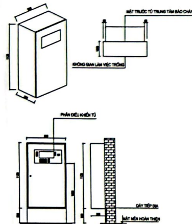
CHI TIẾT LẮP ĐẶT TRUNG TÂM BẢO CHÁY TẠI PHÒNG BẢO VỆ
