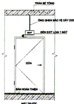
CỬA RA VÀO HOẶC CỬA THANG THOÁT HIỂM
