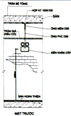
CHI TIẾT LẮP ĐẶT ĐÈN SỰ CỎ LOẠI TREO TƯỜNG
