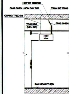
ĐÈN EXIT LOẠI HAI MẶT
