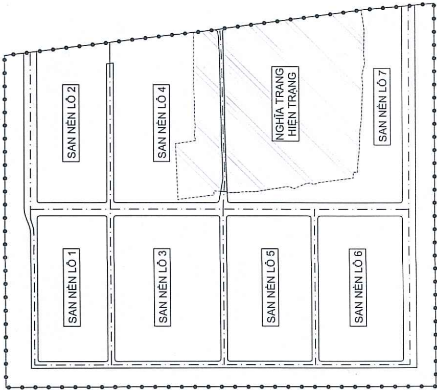
SƠ HẠ VỊ TRÍ CÁC LÔ SÂN NỀN
