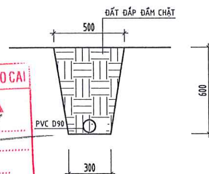
MC RÃNH CHÔN ỐNG THOÁT NƯỚC D90 (L=9m)
