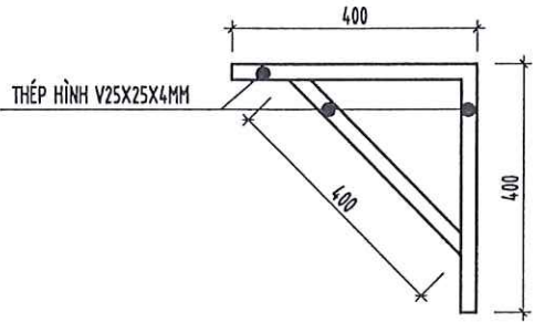
CHI TIẾT CON SƠN ĐÓN ĐIỆN
