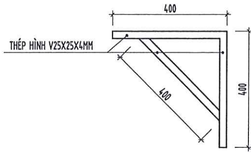
CHI TIẾT CON SƠN ĐÓN ĐIỆN
