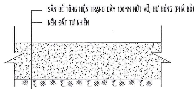
MẶT CẮT SÂN BÊ TÔNG S = 75M2 HIỆN TRẠNG
