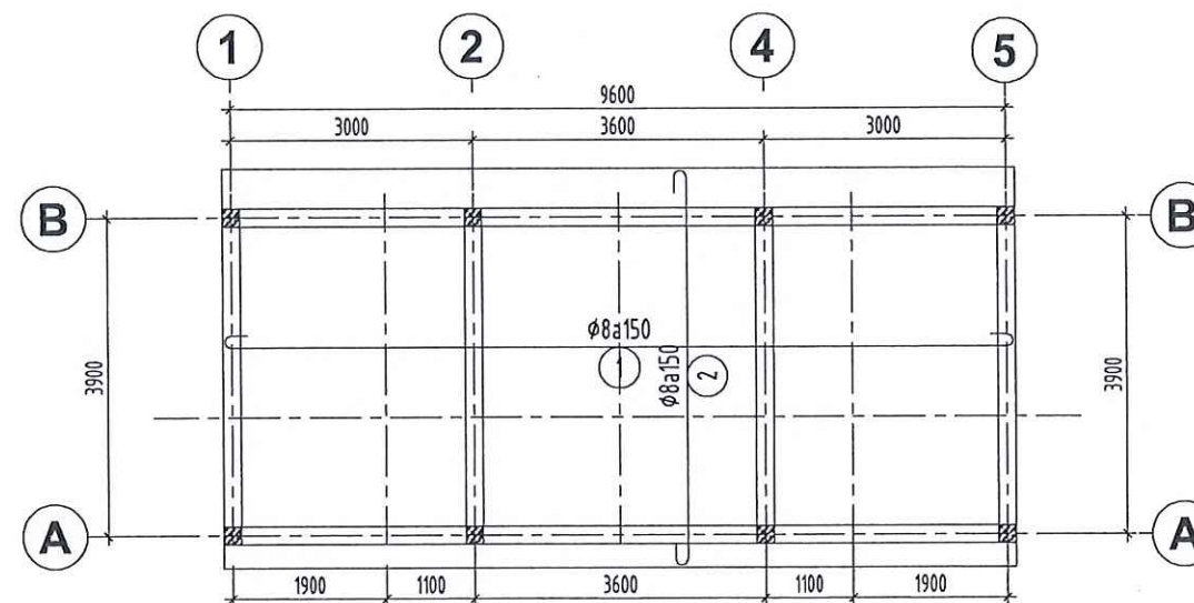
MẶT BẰNG THÉP SÀN LỚP DƯỚI CỐT +7.200
