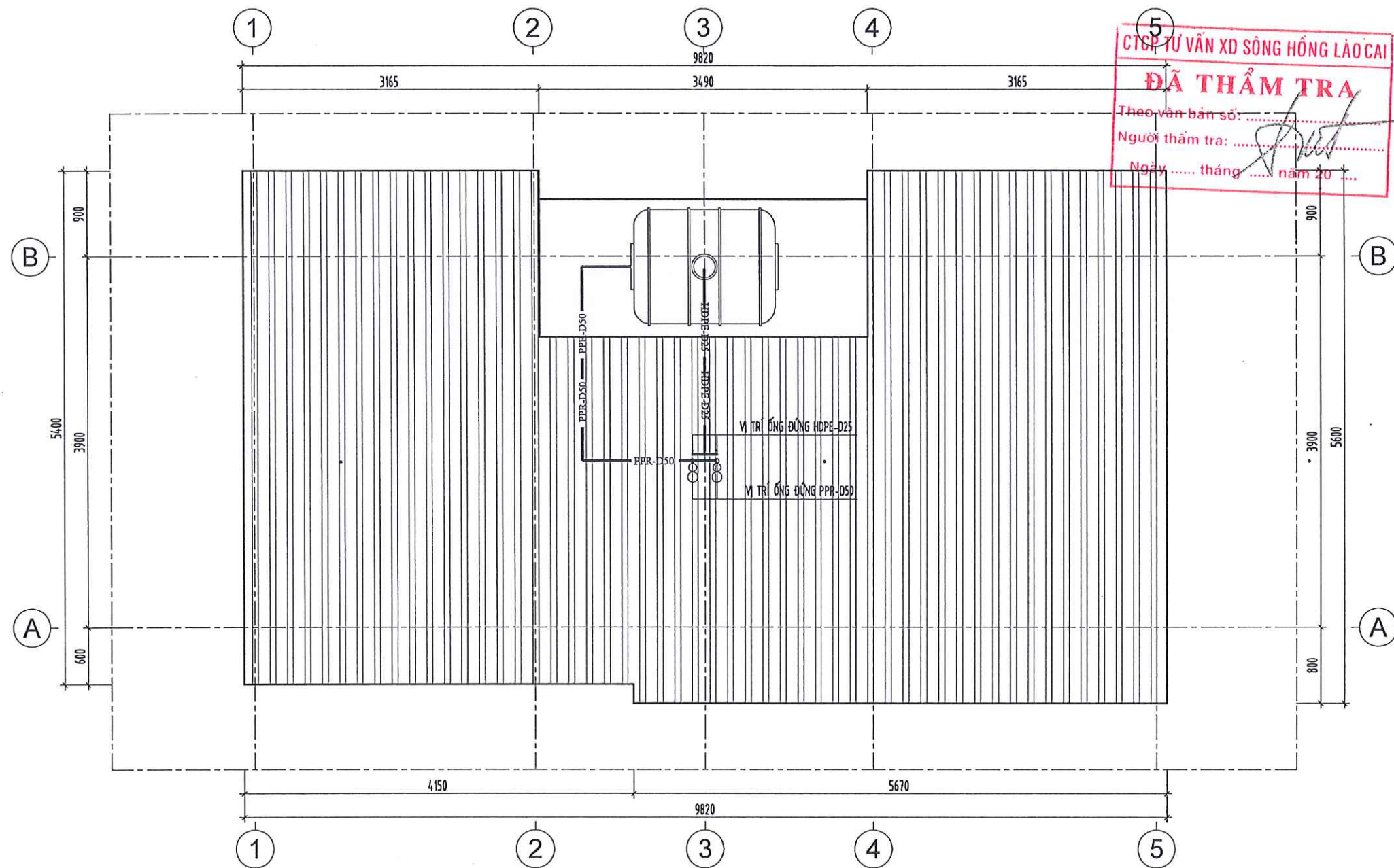
MẶT BẰNG CẤP NƯỚC MÁI
