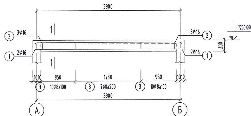
D2-2 (SL= 04, L= 4.12m)
