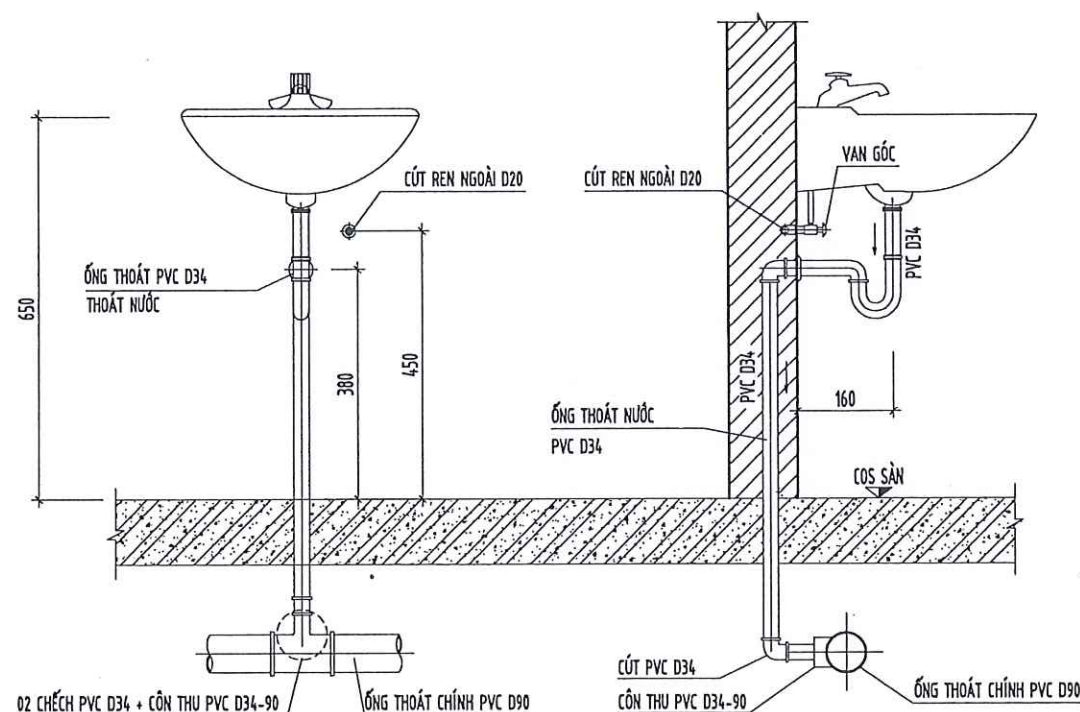
CHI TIẾT LẮP ĐẶT LAVABO
