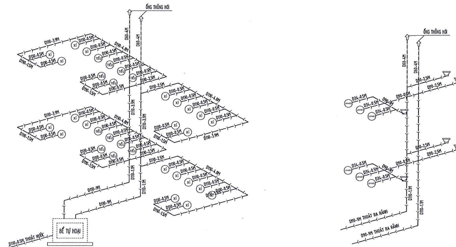
SƠ ĐỒ THOÁT NƯỚC XÍ + BỆT
