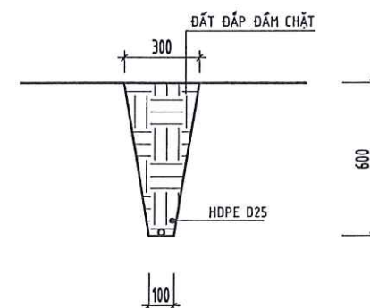
MC RÃNH CHÔN ỐNG CẤP NƯỚC HDPE D25 (L=40m)
