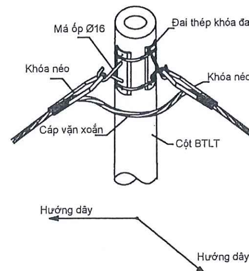
VỊ TRÍ CỘT NEO GÓC
