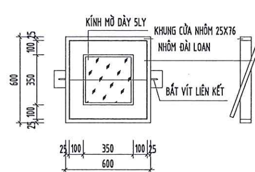
CHI TIẾT CỬA SỔ CÁNH LẠT S2 (SL:08 BỘ)
