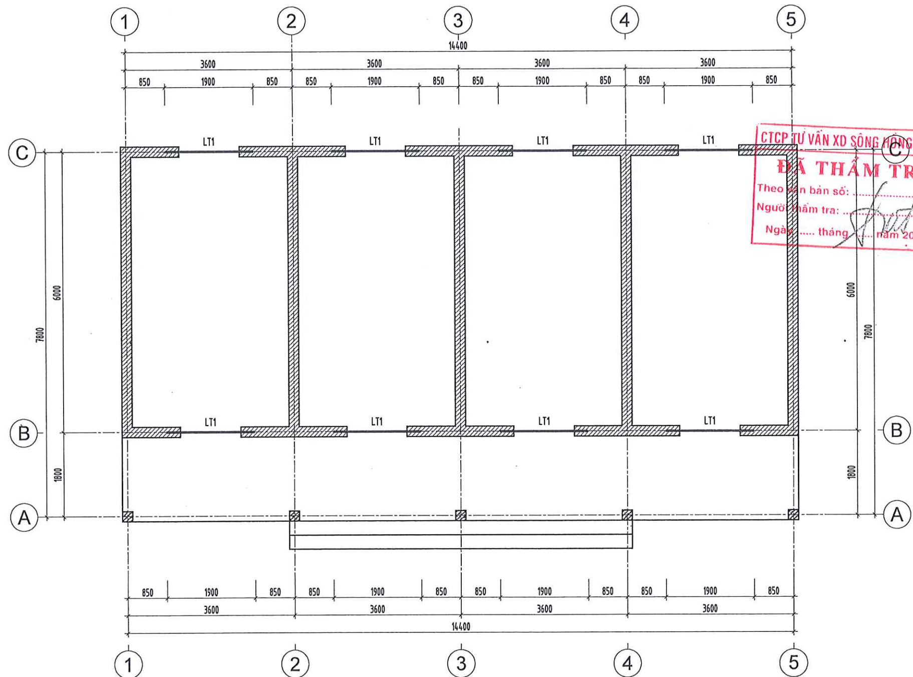
MẶT BẰNG LANH TÔ NHÀ BÁN TRÚ SỐ 3
