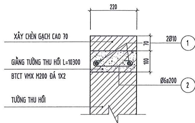
CHI TIẾT TƯỜNG THU HỒI NHÀ VỆ SINH, SL: 04
