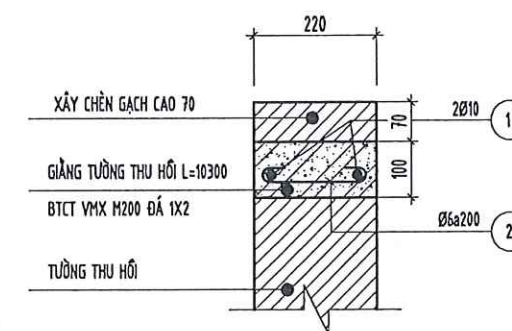
MC GIĂNG MÁI
