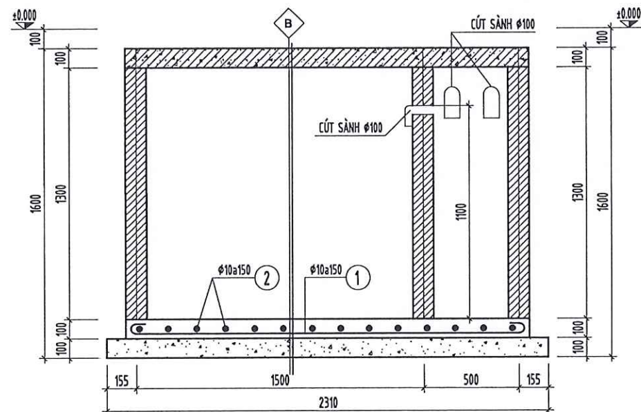
MẶT CẮT 2-2
