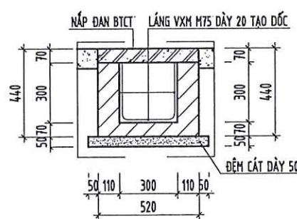
CT RÃNH CÓ NẮP ĐAN LÀM MỚI L= 29.3M
