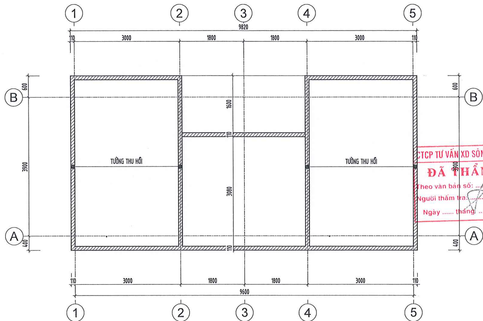
MẶT BẰNG TƯỜNG THU HỒI NHÀ VỆ SINH
