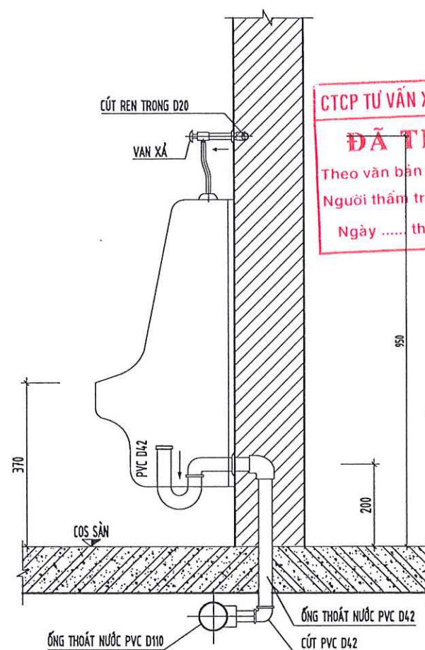
CHI TIẾT LẮP ĐẶT TIÊU TREO
