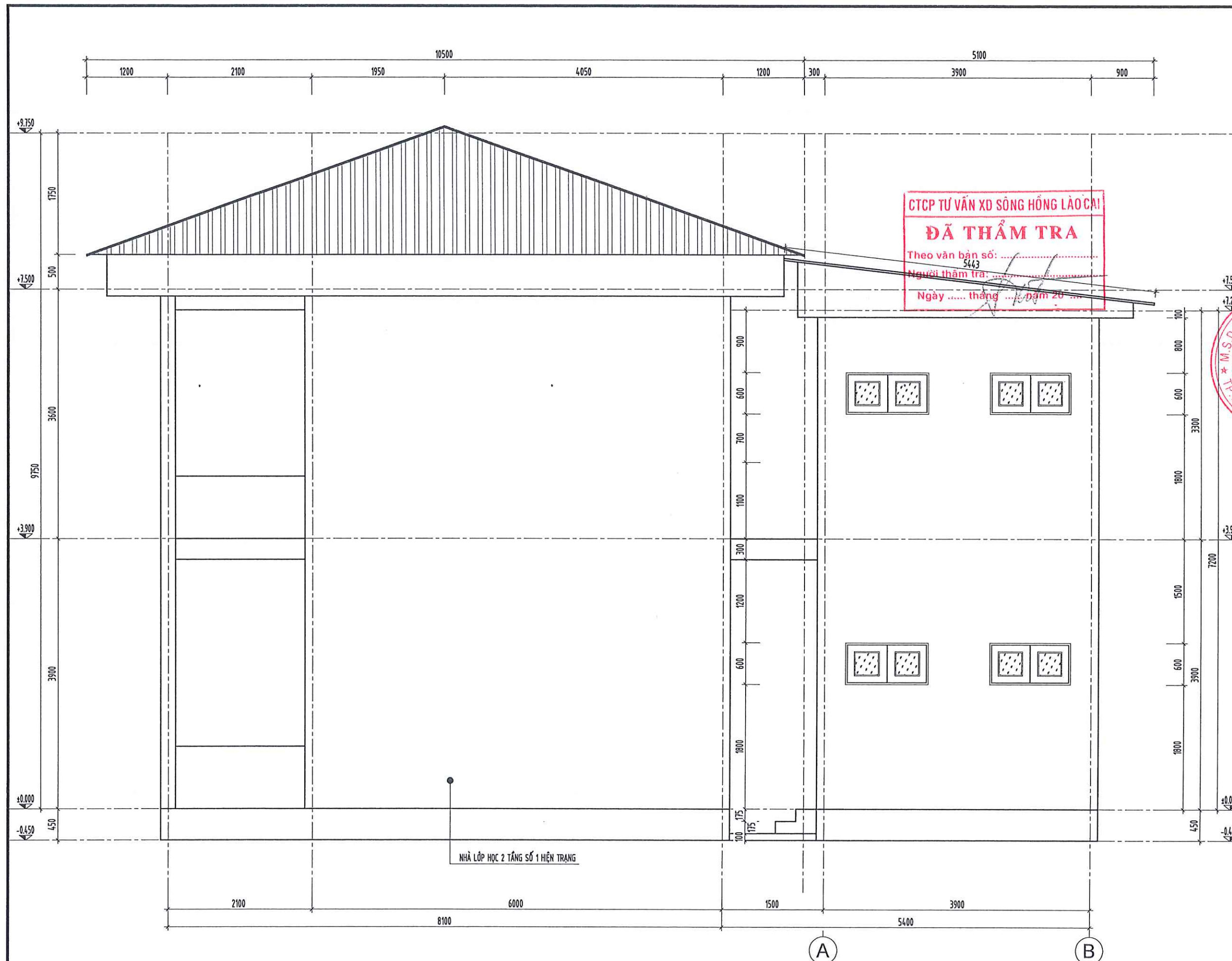
MẶT ĐÚNG A - B NHÀ VỆ SINH
