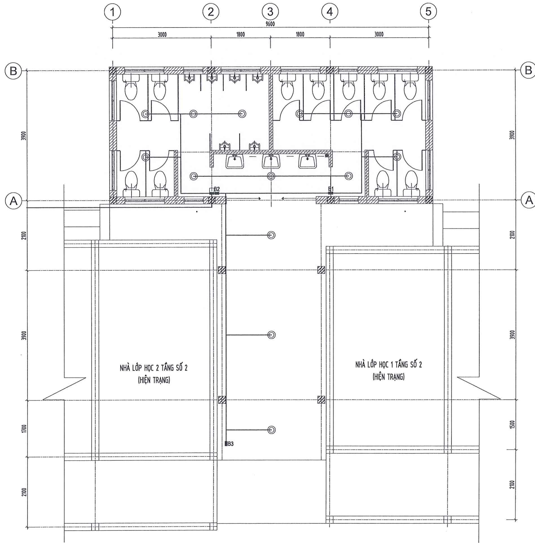
MẶT BẰNG CẤP ĐIỆN TẦNG 1 NHÀ VỆ SINH + NHÀ CẦU
