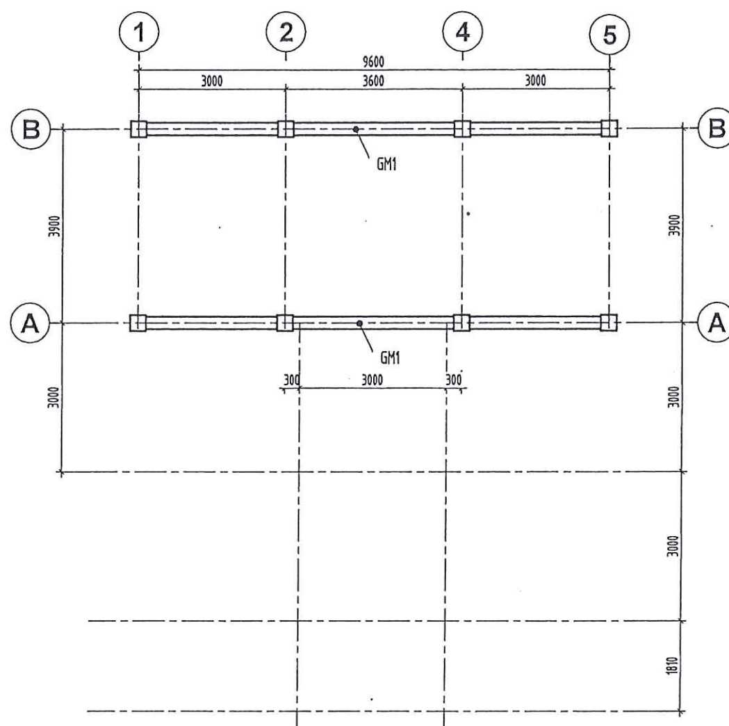
MẶT BẰNG GIẰNG MÓNG -1.700
