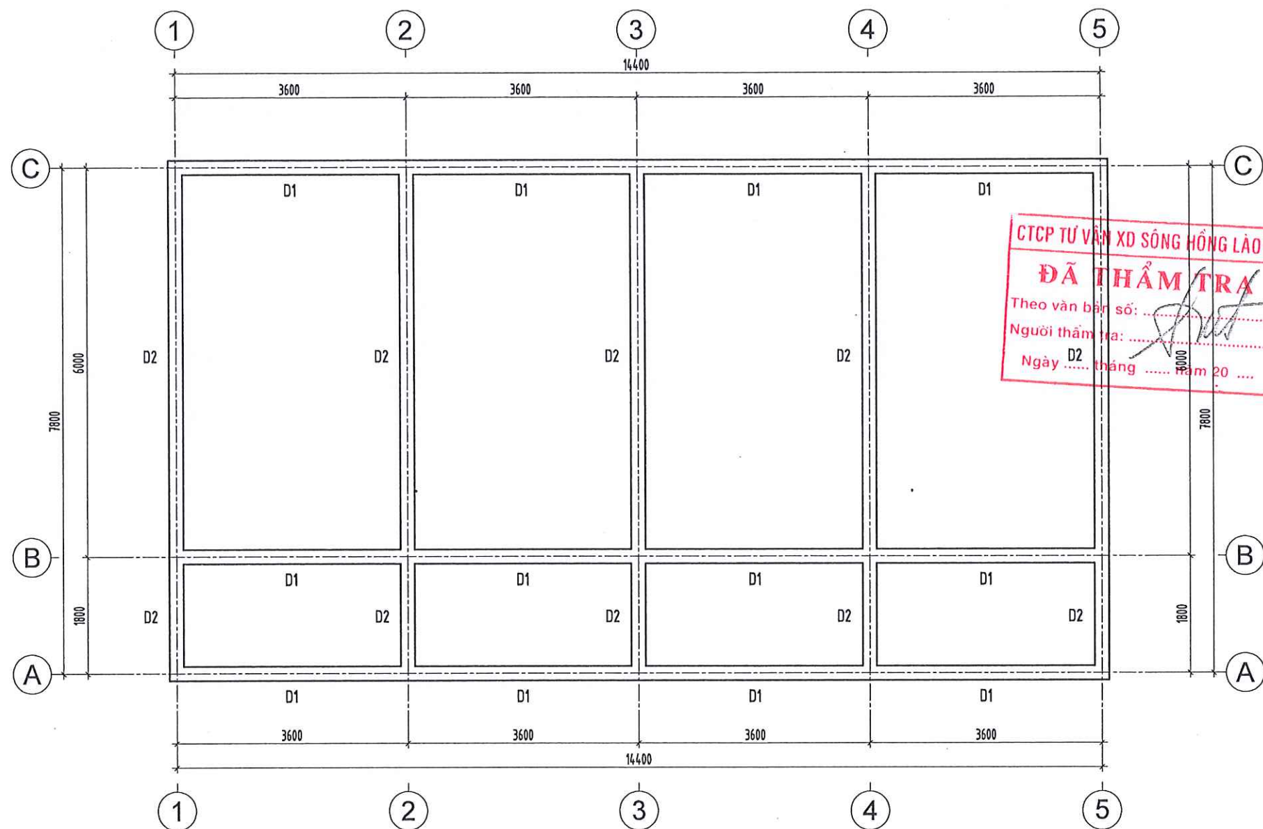
MẶT BẰNG DẦM NHÀ BÁN TRÚ SỐ 3
