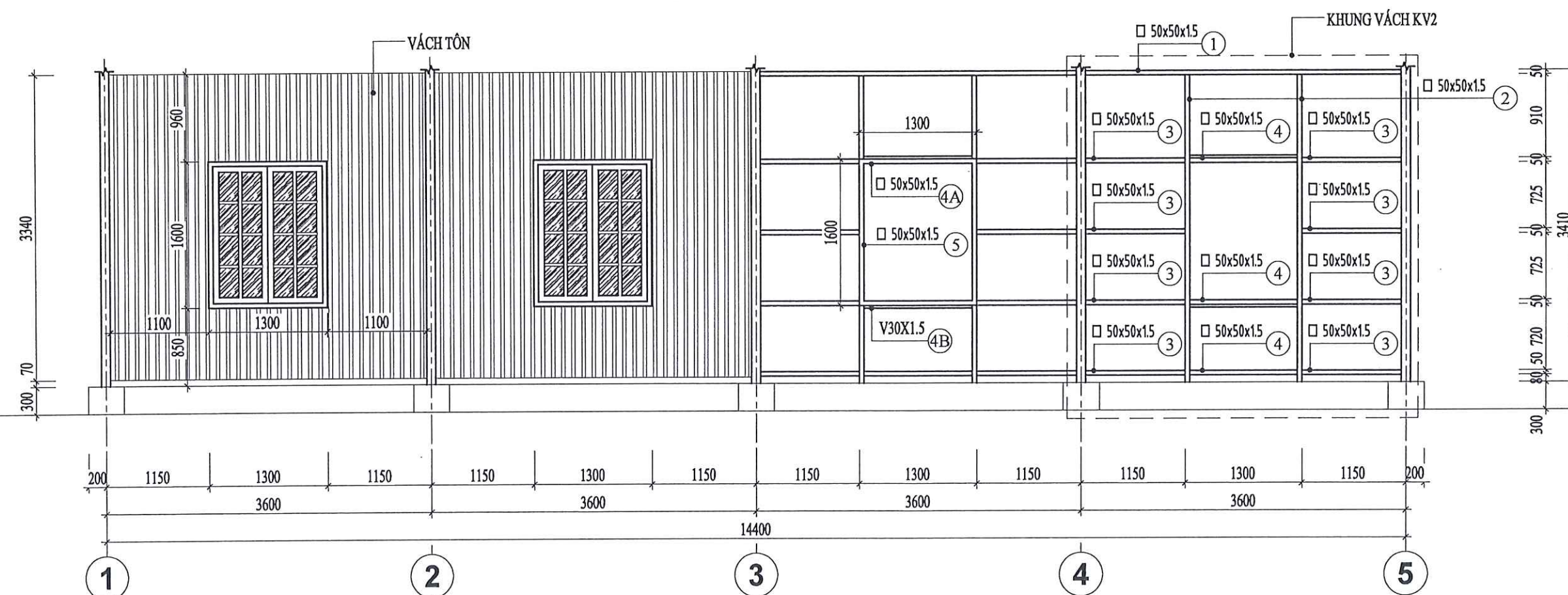
CHI TIẾT KHUNG VÁCH KV2
