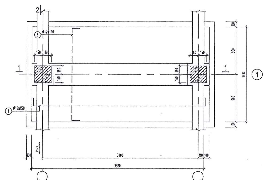
MÓNG M2 (SL: 2)
