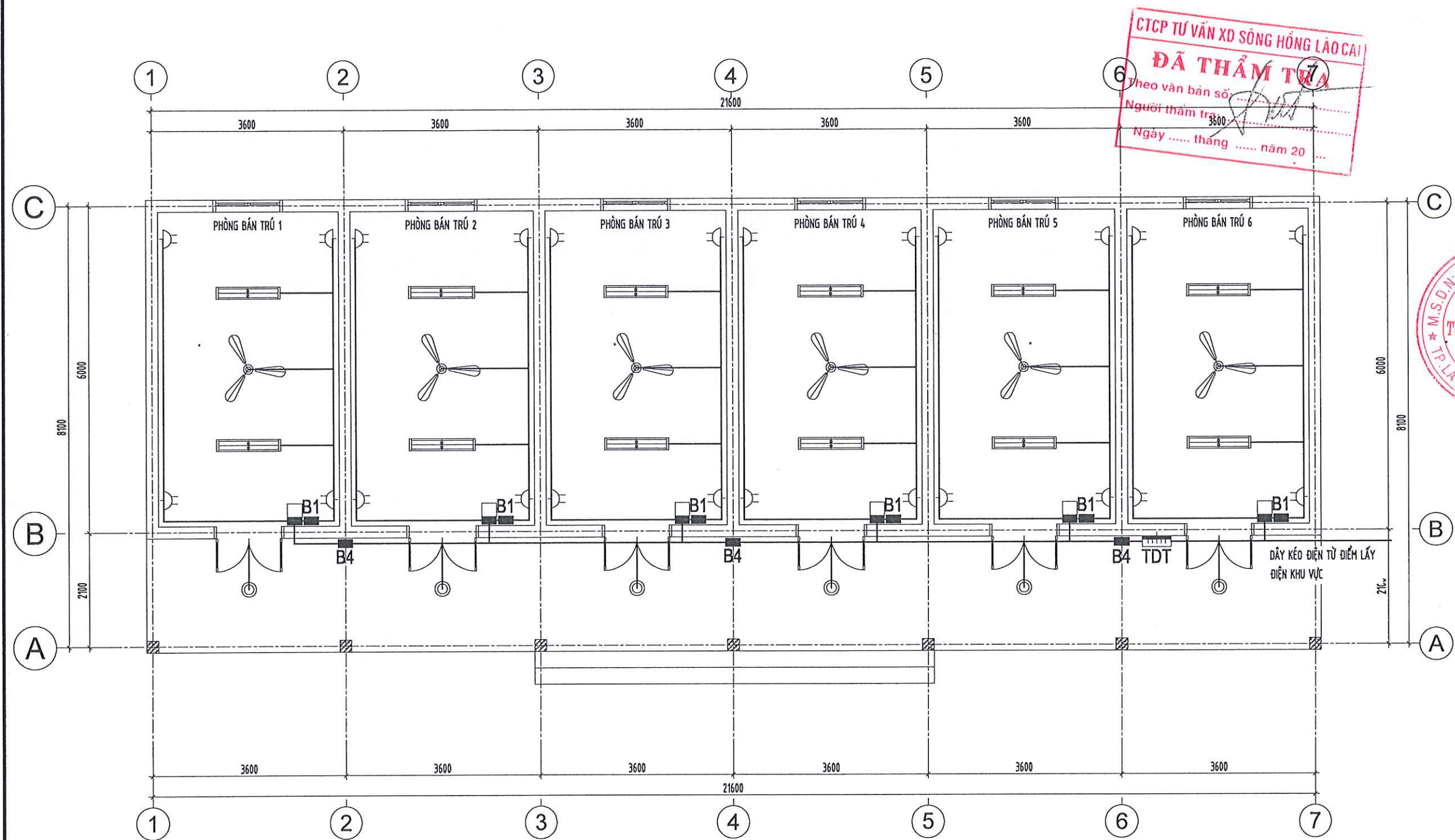
MẶT BẰNG CẤP ĐIỆN NHÀ BÁN TRÚ SỐ 2
