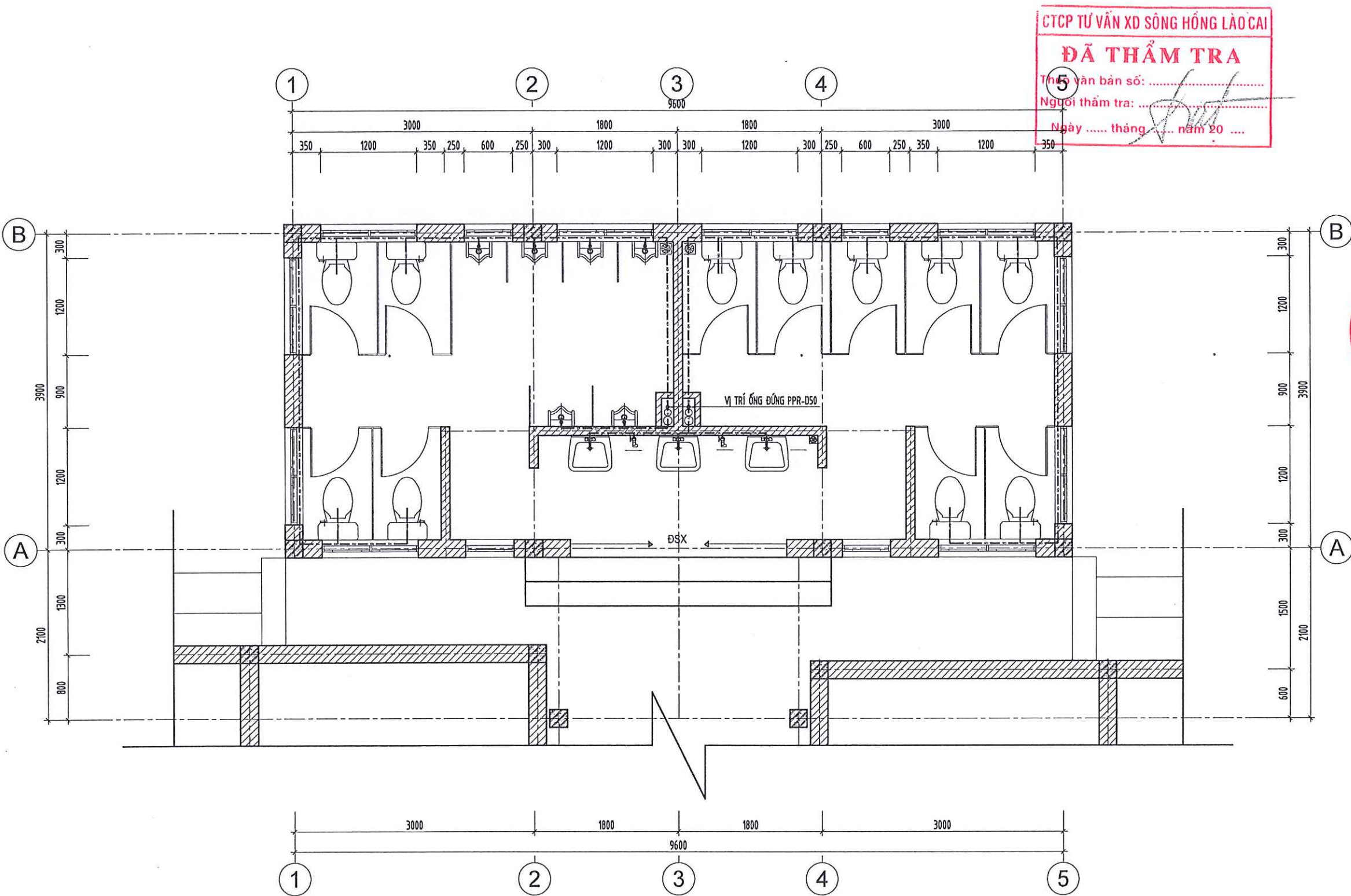
MẶT BẰNG CẤP NƯỚC TẦNG 1
