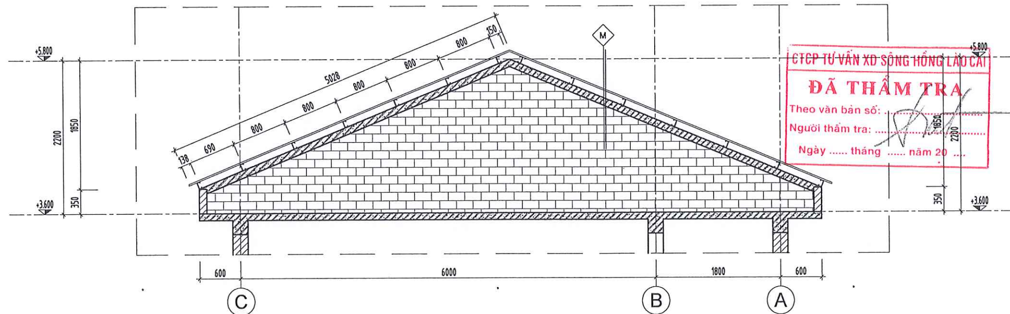
CHI TIẾT TƯỜNG THU HỒI
