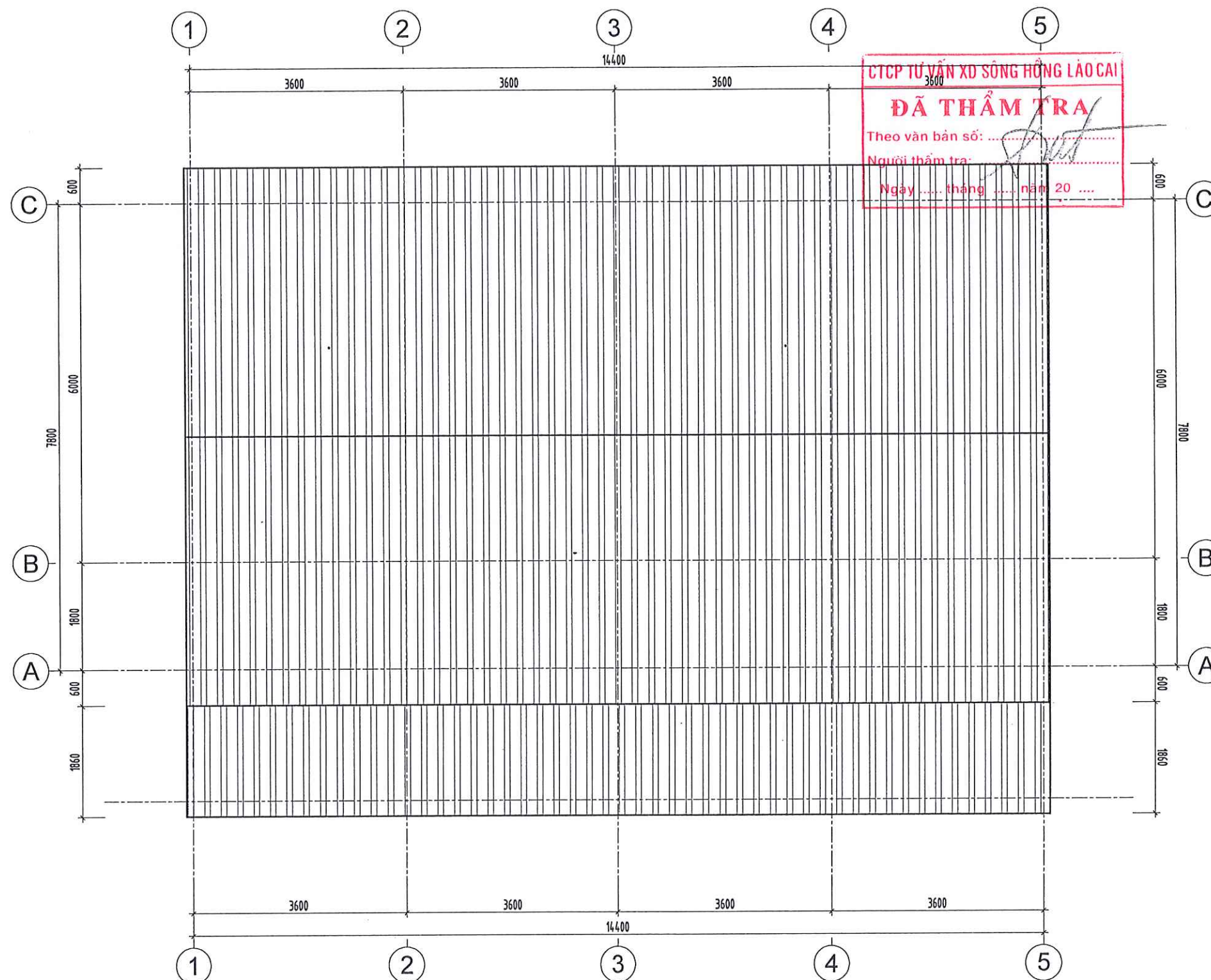
MẶT BẰNG MÁI NHÀ BÁN TRÚ SỐ 3
