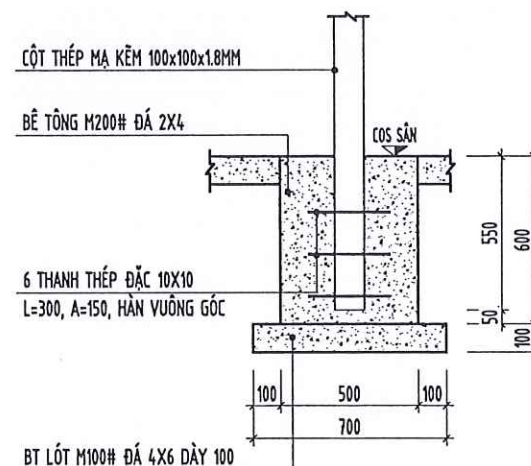
CẮT QUA MÓNG M1
