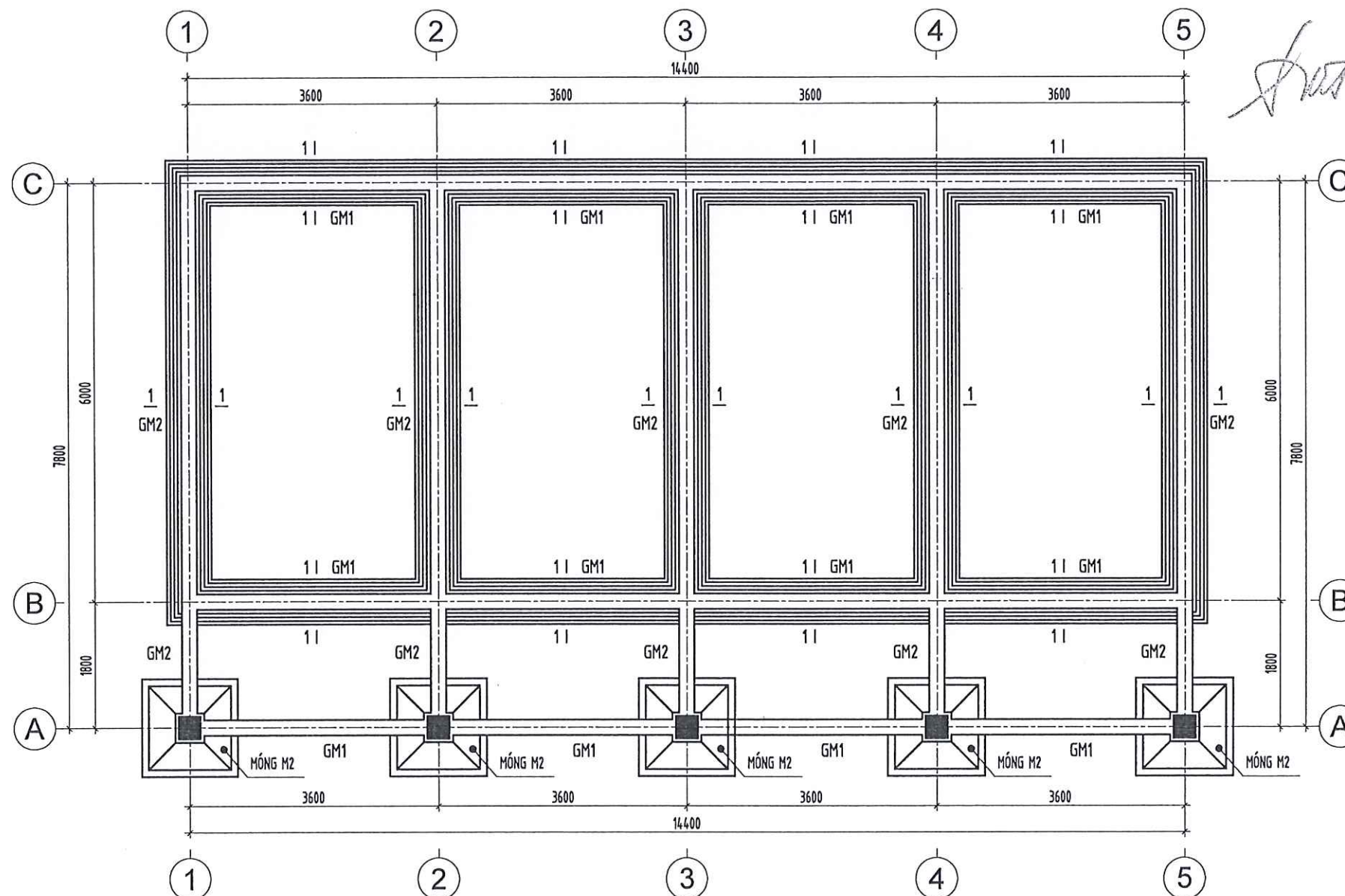
MẶT BẰNG MÓNG NHÀ BÁN TRÚ SỐ 3
