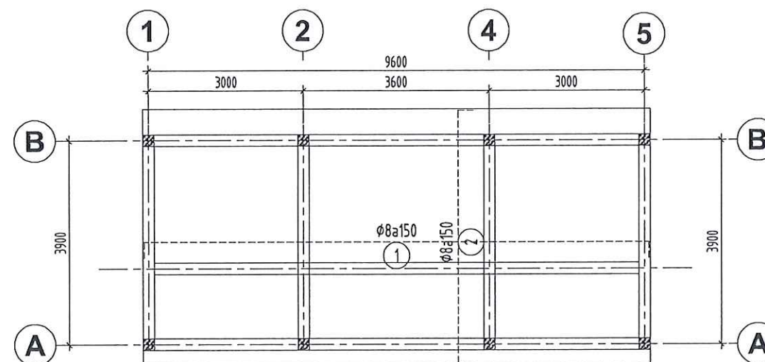
MẶT BẰNG THÉP SÀN LỚP TRÊN CỐT +7.200
