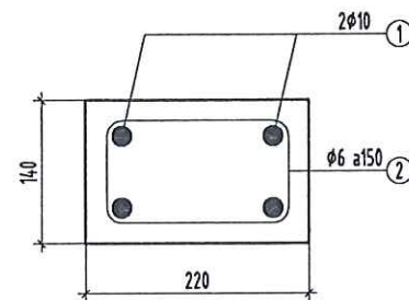
CHI TIẾT LT1 - 1900
