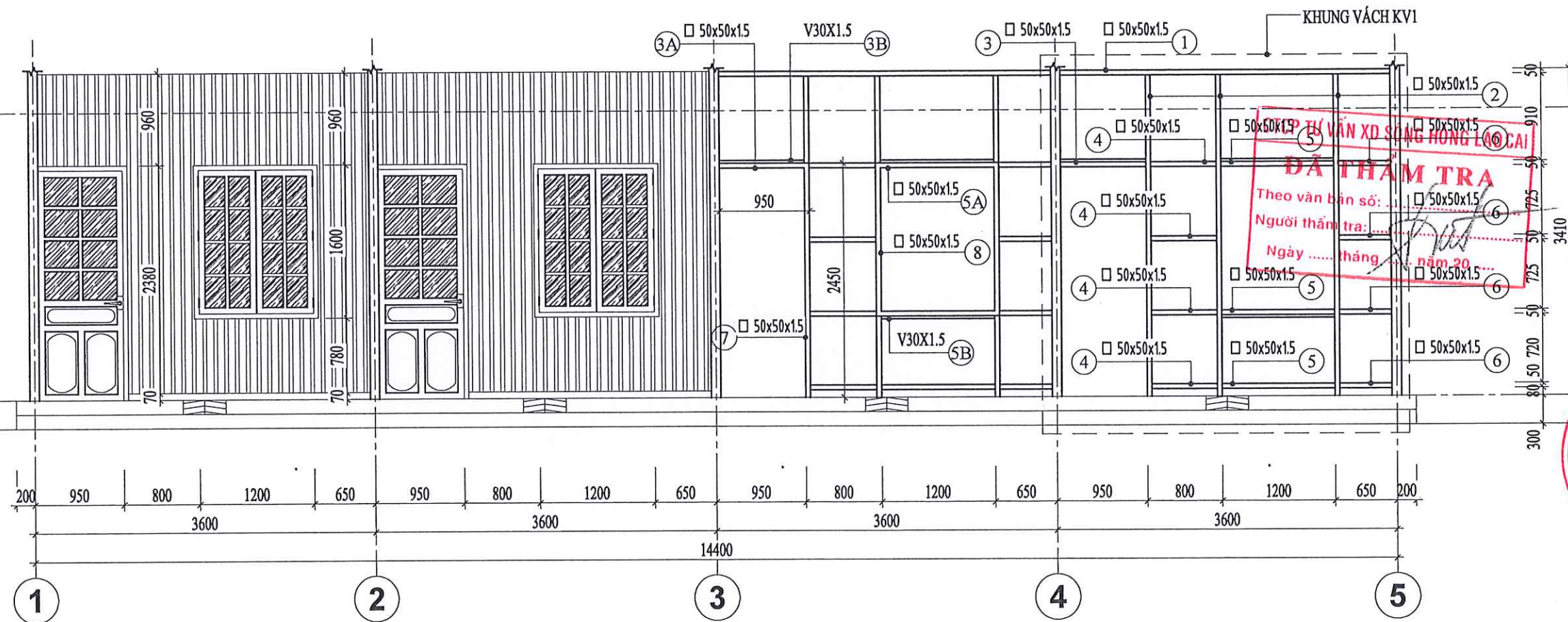
CHI TIẾT KHUNG VÁCH KV1
