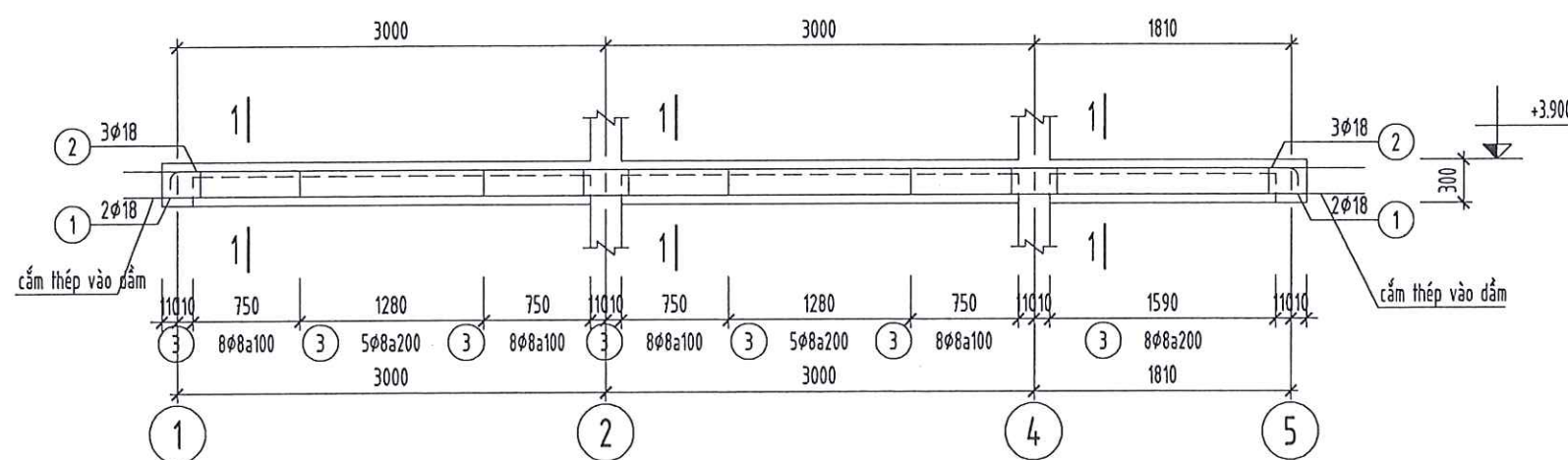
D5-1 (SL= 02, L= 8.03m)
