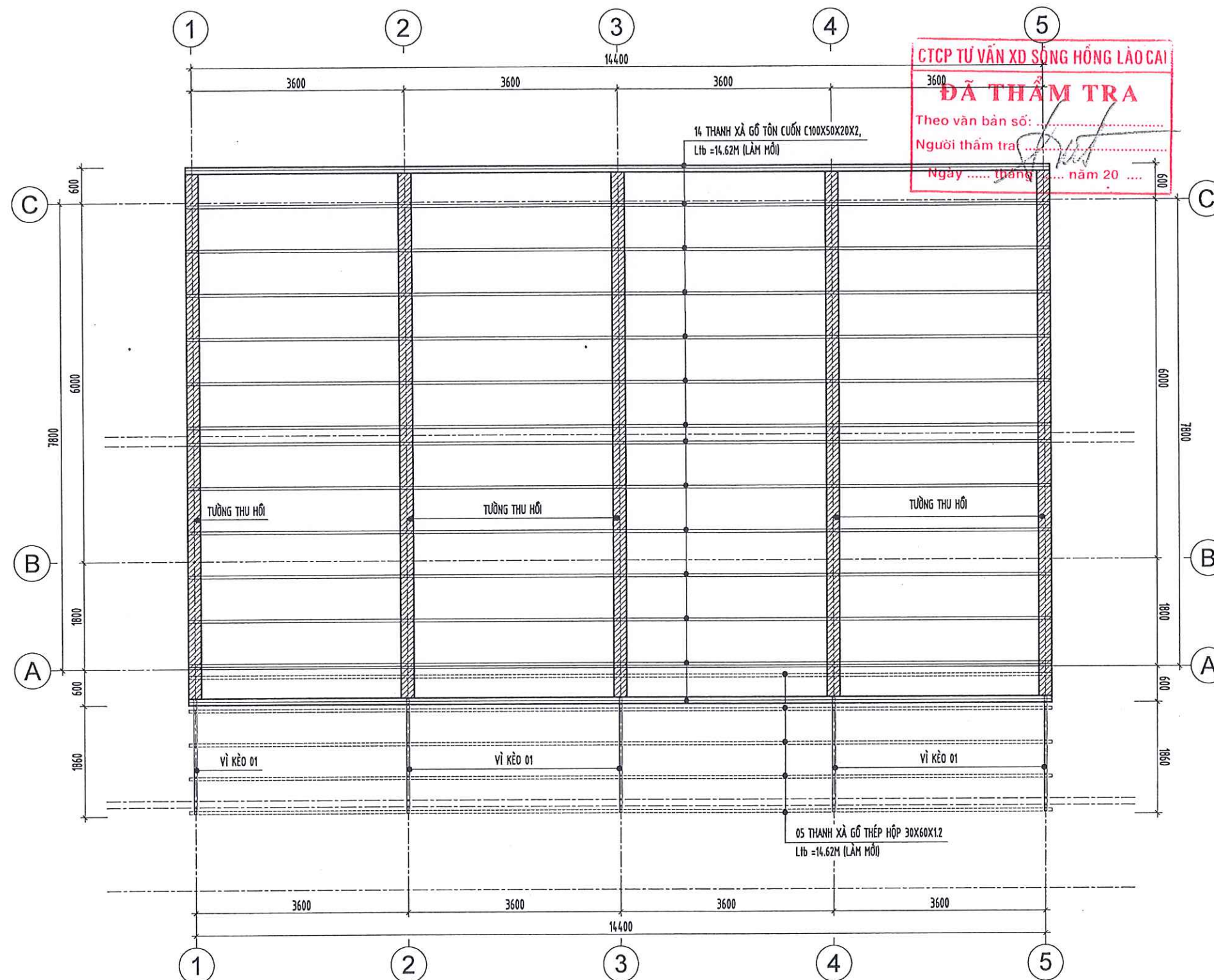
MẶT BẰNG VÍ KÈO + TƯỜNG THU HỒI NHÀ BÁN TRÚ SỐ 3
