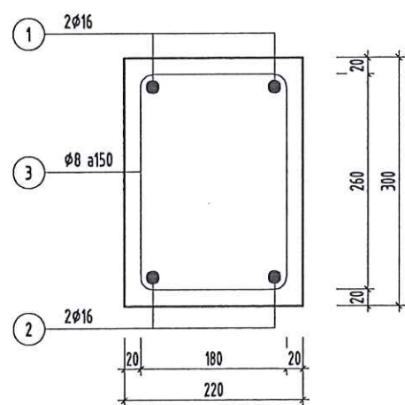
CHI TIẾT D1 L=14.58M
