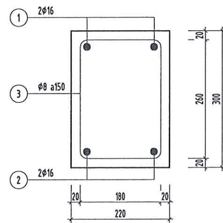
CHI TIẾT D2 L=7.98M
