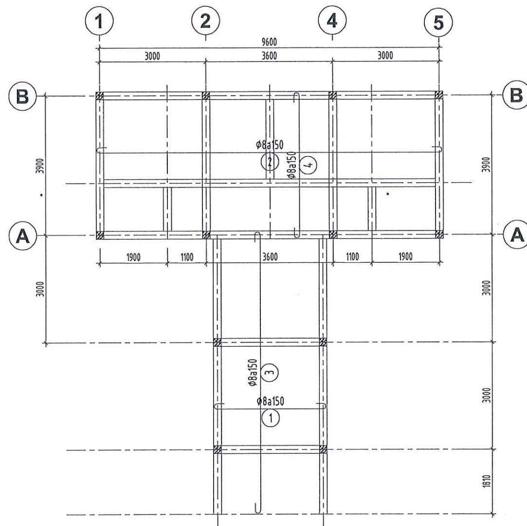
MẶT BẰNG THÉP SÀN LỚP DƯỚI CỐT +3.900
