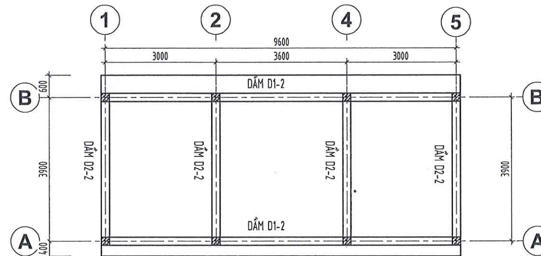
MẶT BẰNG KẾT CẤU CỐT +7.200
