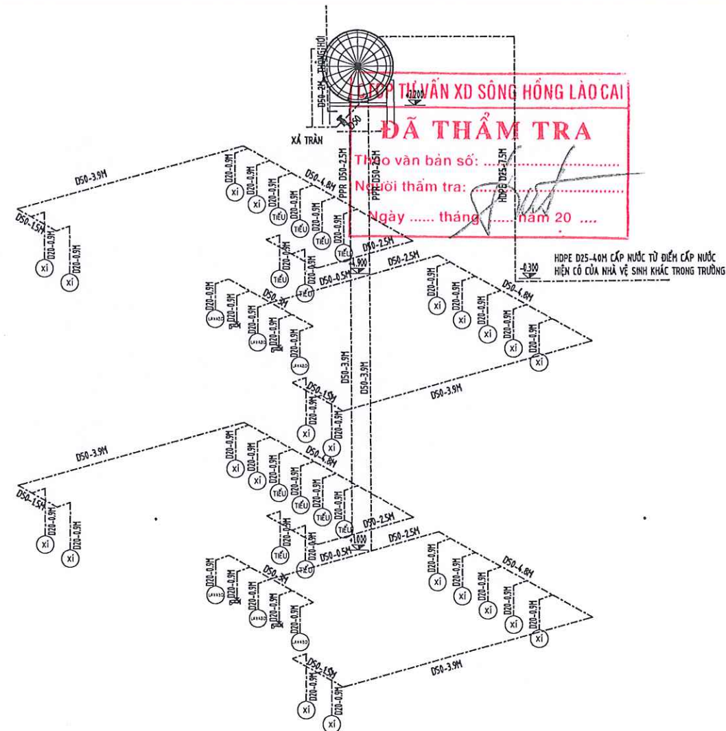
SƠ ĐỒ CẤP NƯỚC
