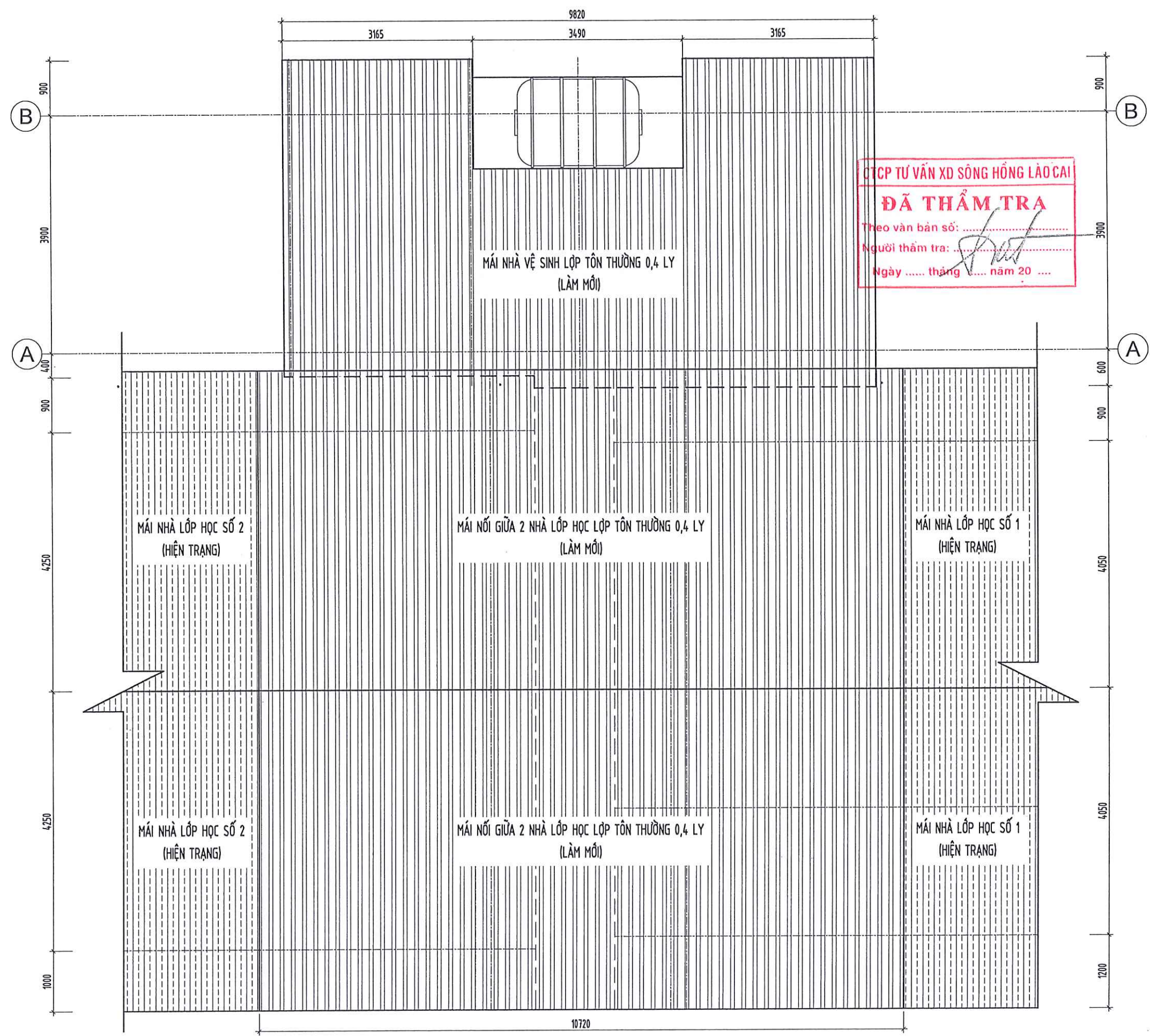
MẶT BẰNG MÁI NHÀ VỆ SINH + MÁI NỐI GIỮA 2 NHÀ LỚP HỌC
