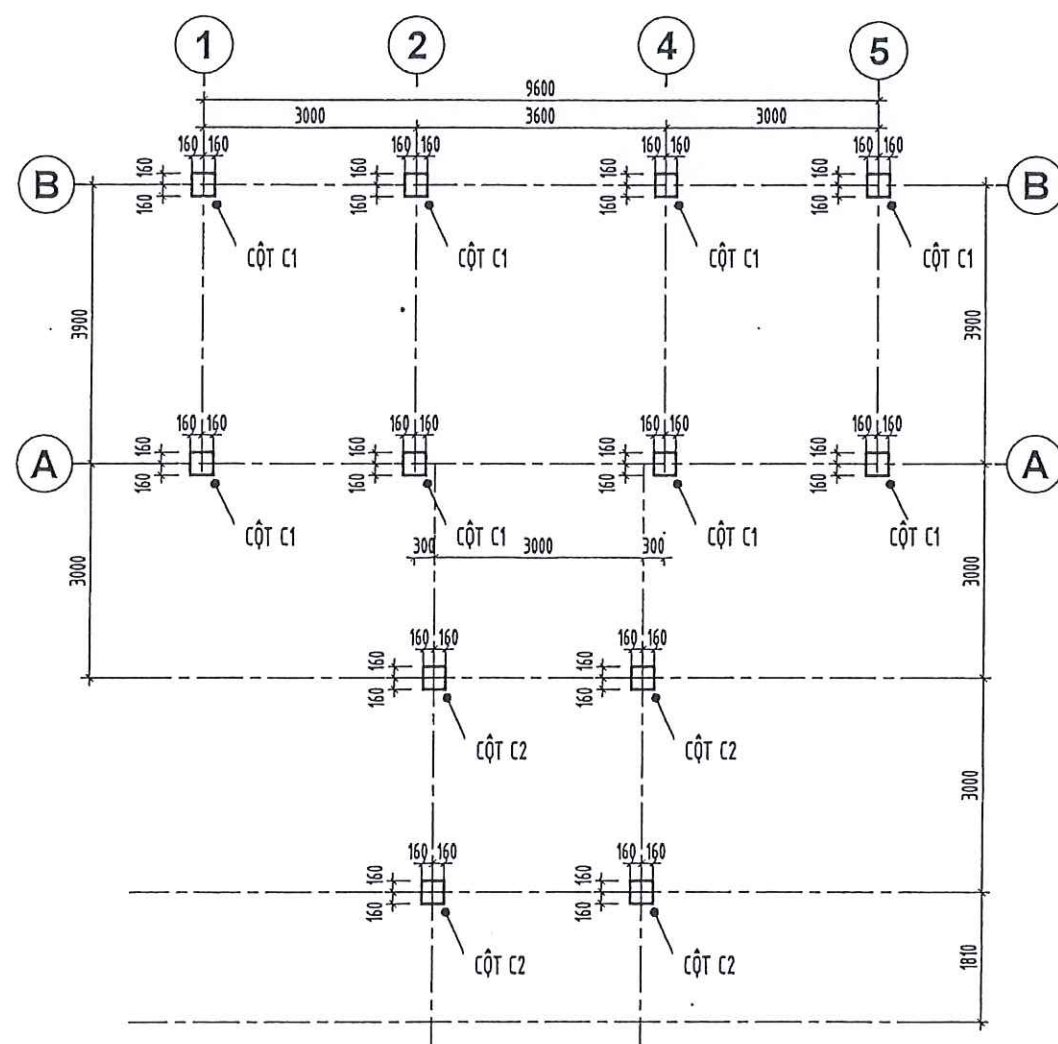
MẶT BẰNG ĐỊNH VỊ CỘT CỘT
