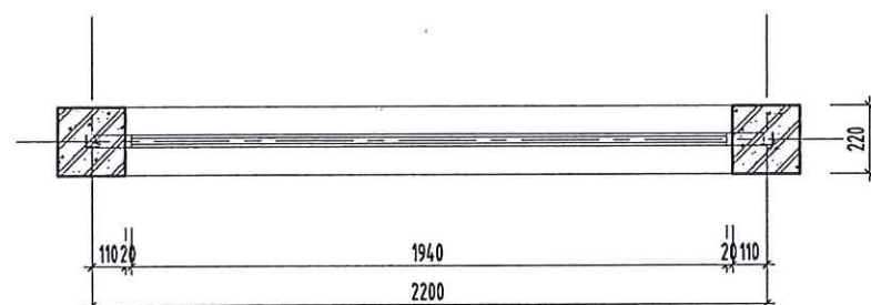
MẶT BẰNG ĐOẠN HÀNG RÀO A - B (L = 2.2M)
