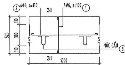
CT NẮP ĐAN RÃNH SL: 29
