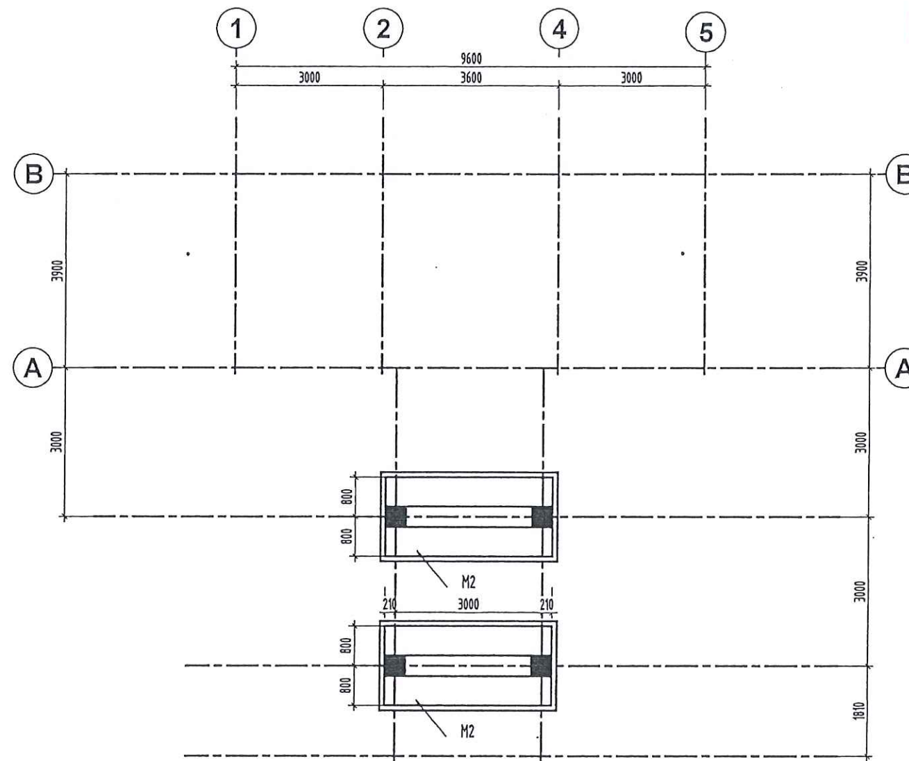
MẶT BẰNG MÓNG CỘT -1.600
