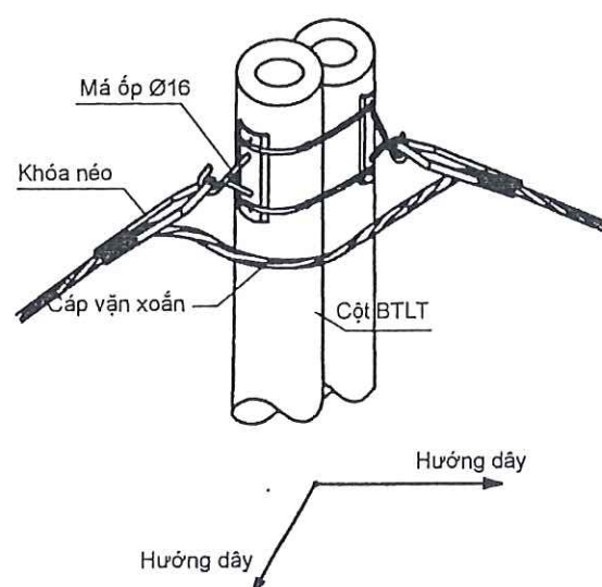
VỊ TRÍ CỘT NEO GÓC
