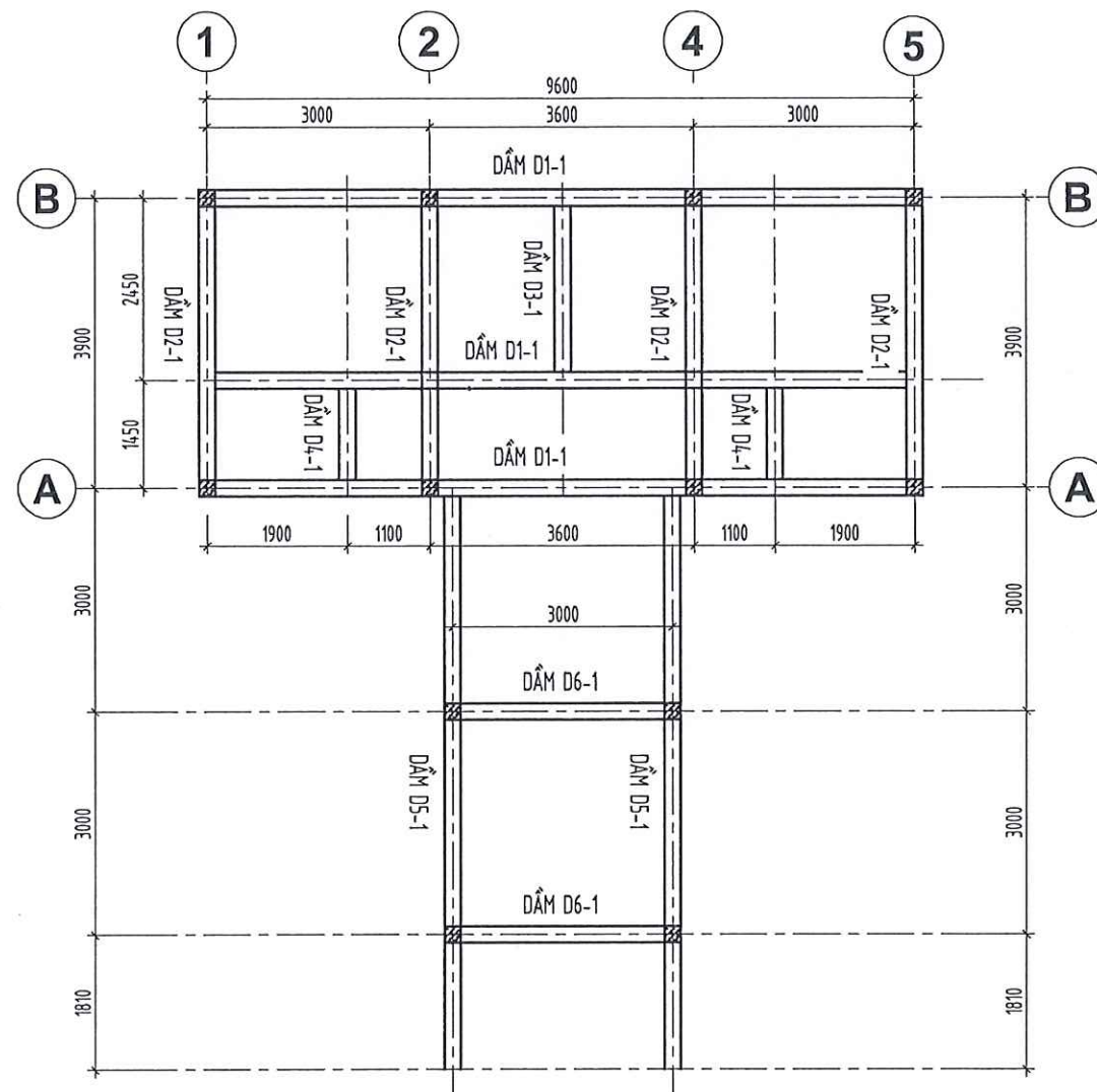
MẶT BẰNG KẾT CẤU CỐT +3.900
