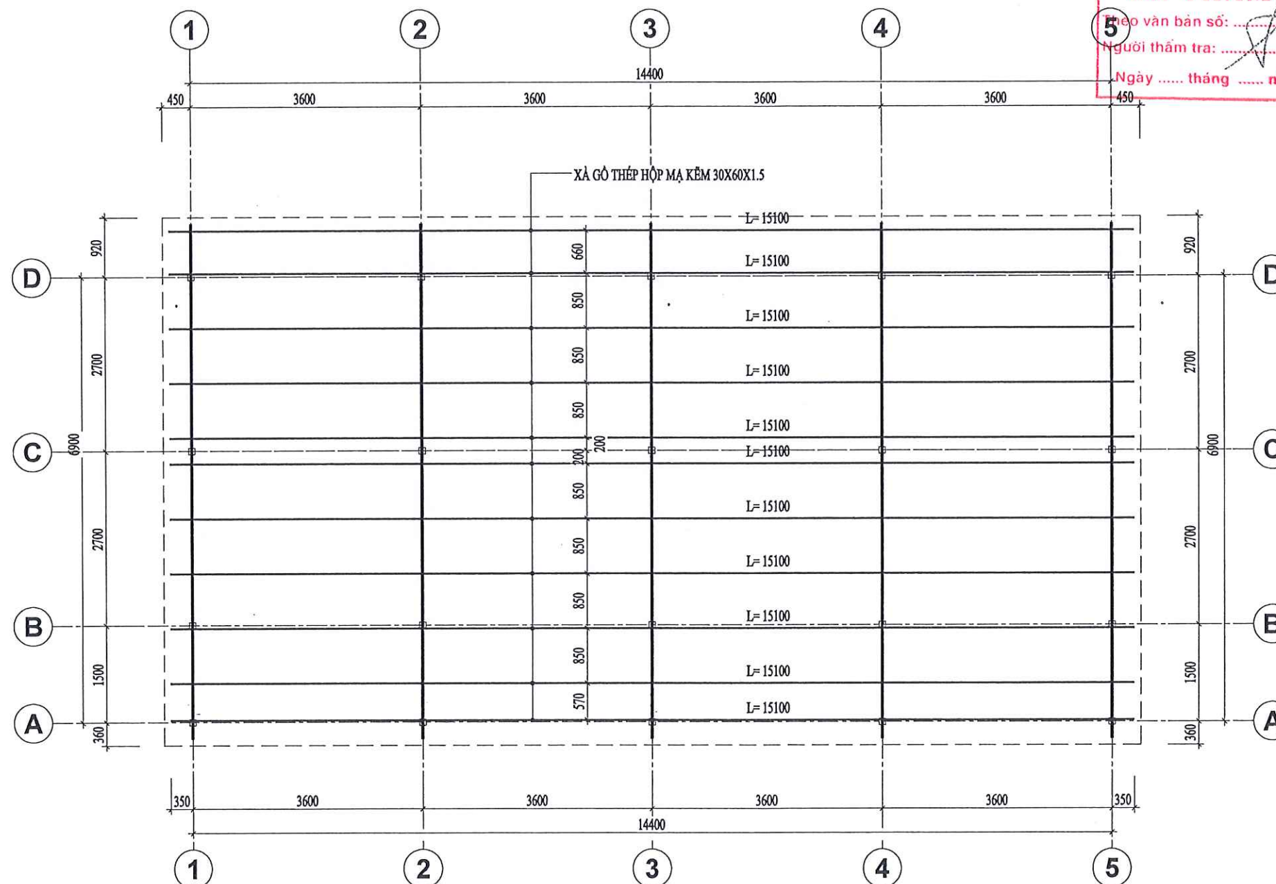
MẶT BẰNG BỐ TRÍ XÀ GÔ
