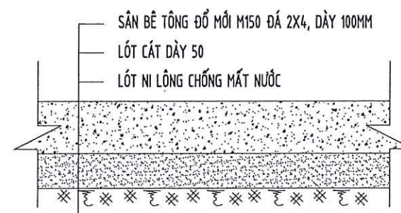
MẶT CẮT SÂN BÊ TÔNG S= 154 M2( LÀM MỚI )
