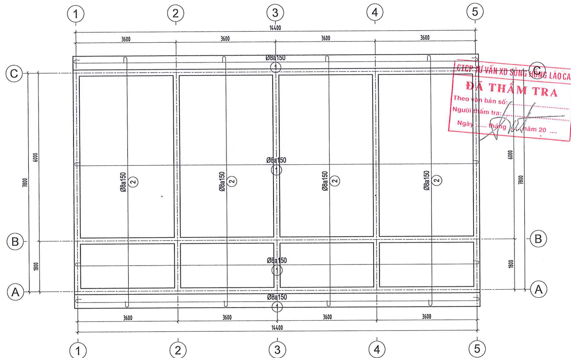
MẶT BẰNG THÉP MÁI NHÀ BÁN TRÚ SỐ 3
