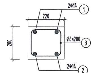
CHI TIẾT GIẺNG MÓNG
