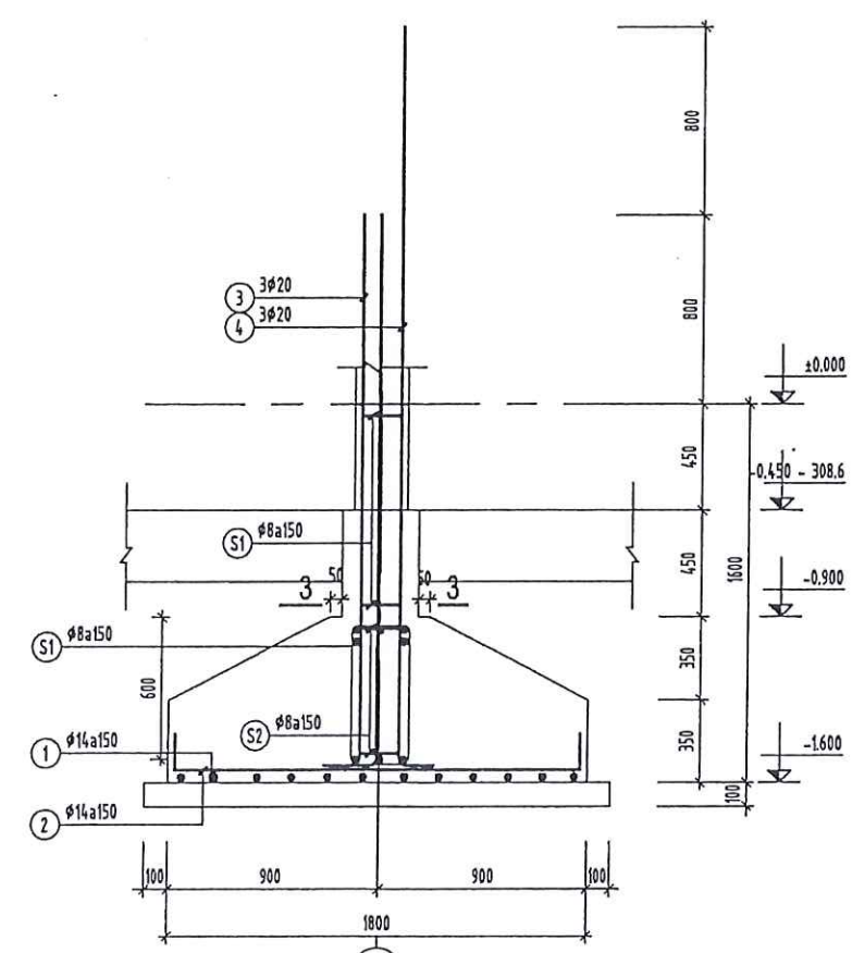
MẶT CẮT 2-2
