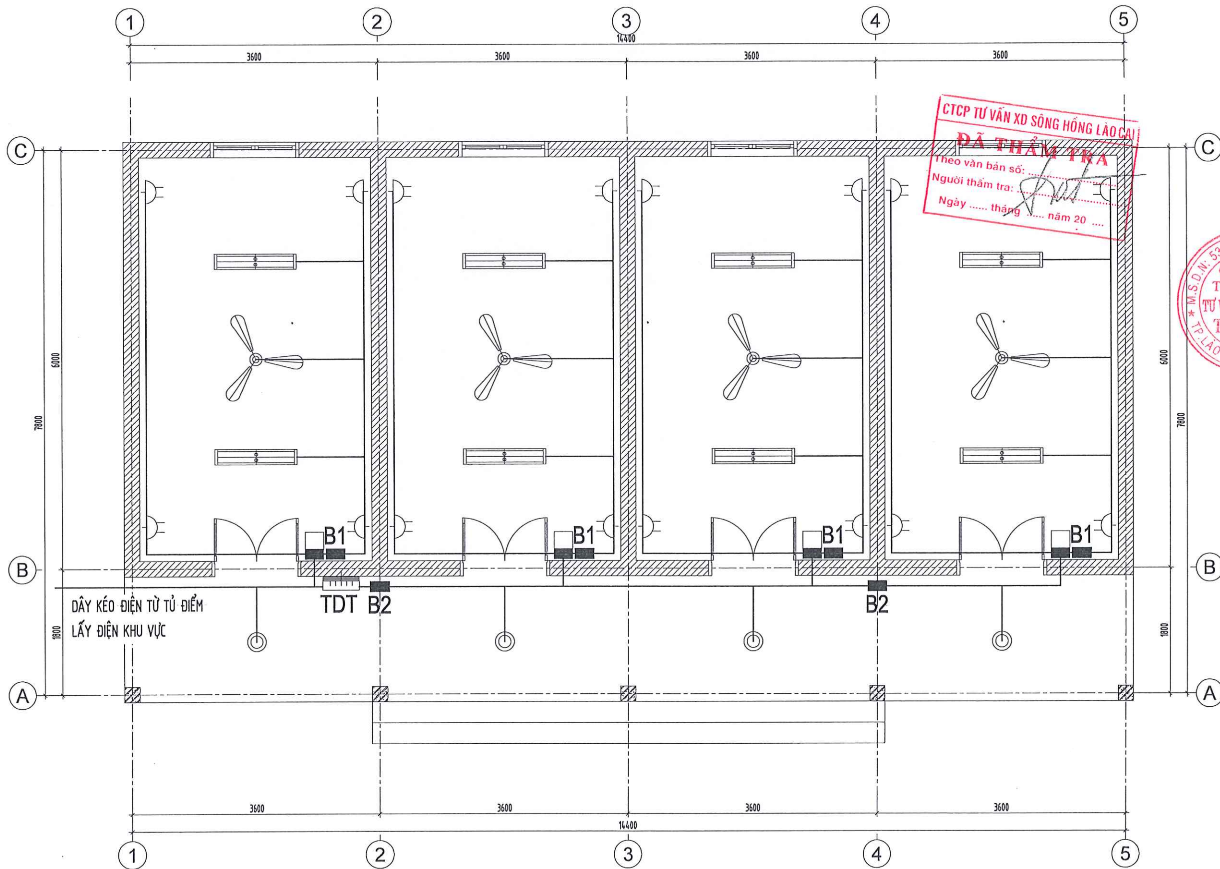
MẶT BẰNG CẤP ĐIỆN NHÀ BÁN TRÚ 3
