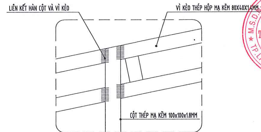
CHI TIẾT LIÊN KẾT CỘT
