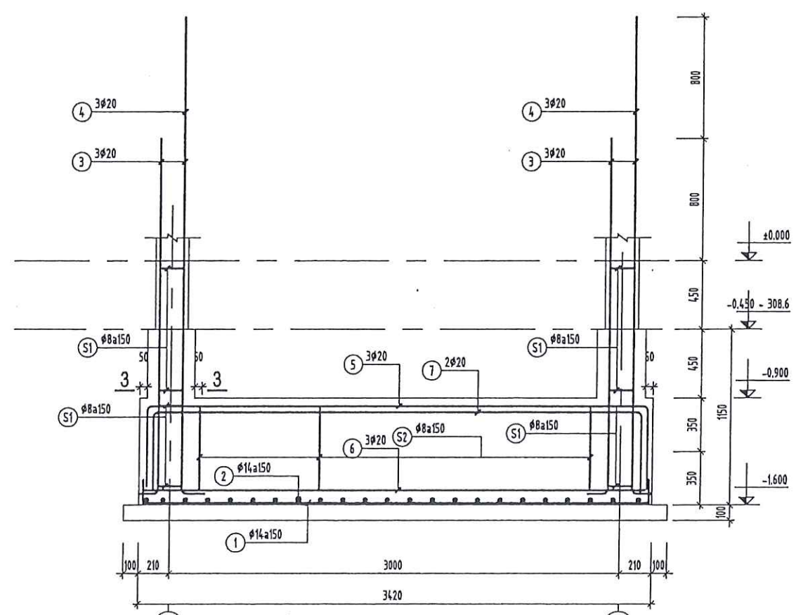
MẶT CẮT 1-1
