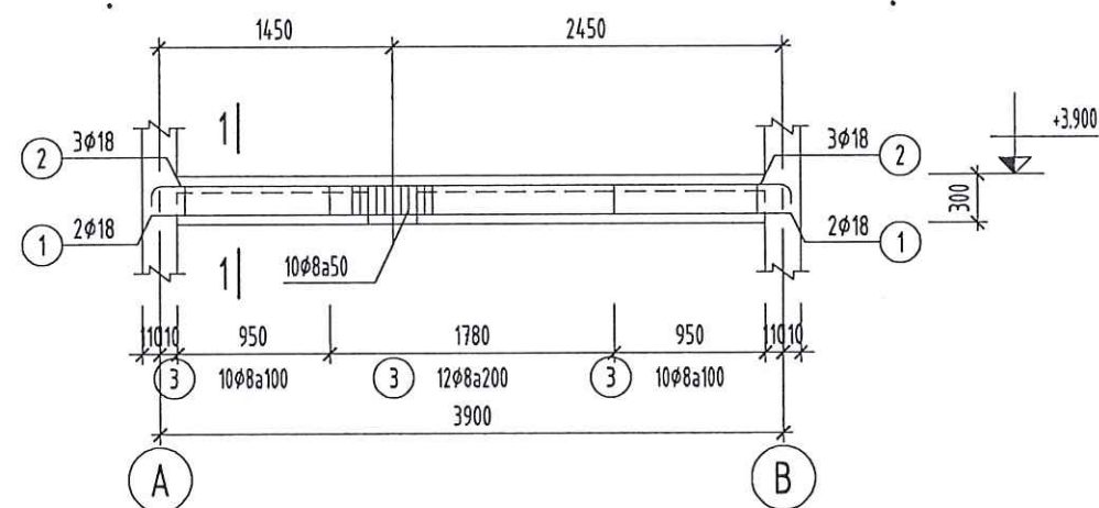
D2-1 (SL= 04, L= 4.12m)
