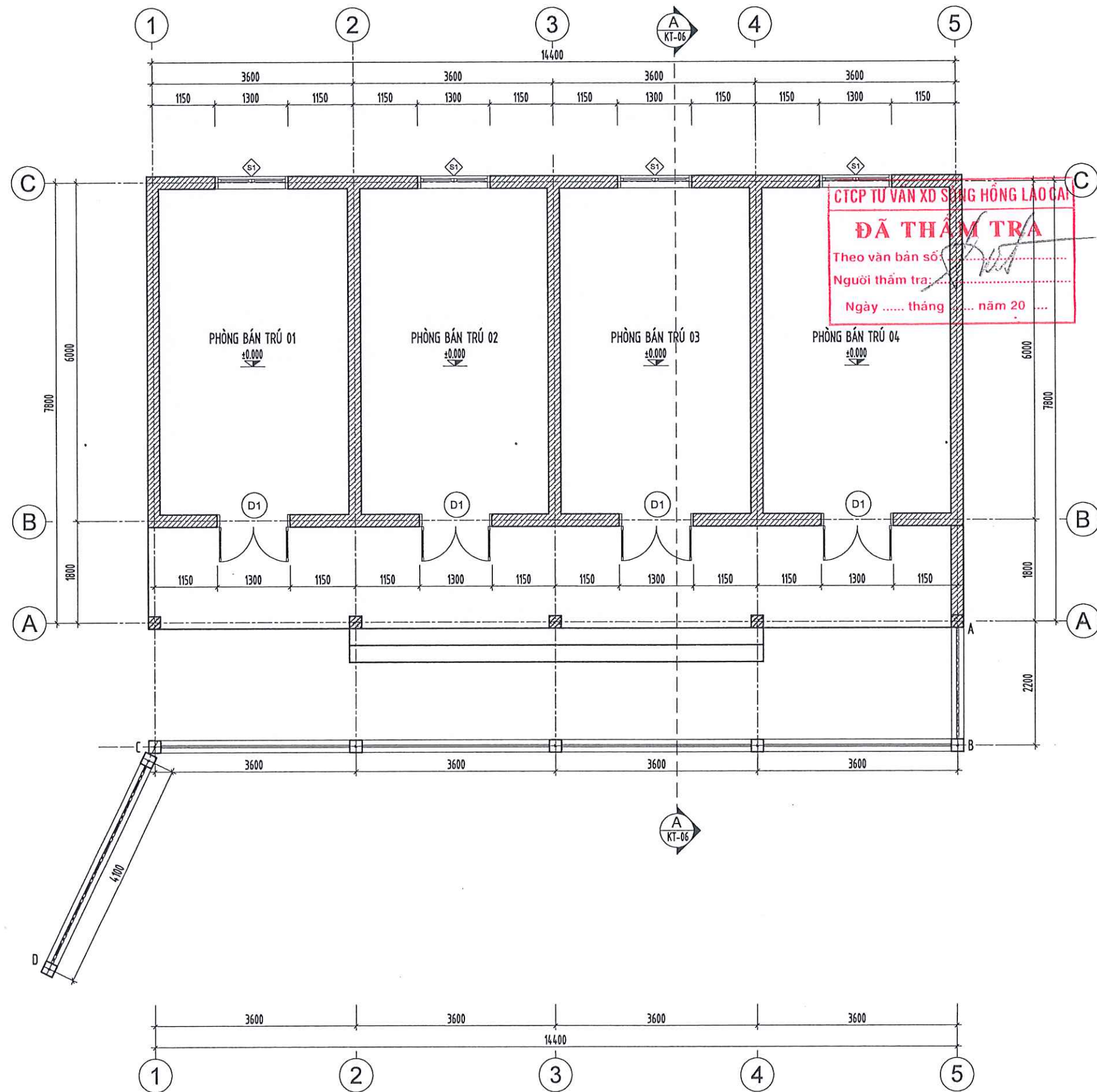
MẶT BẰNG NHÀ BÁN TRÚ SỐ 3
