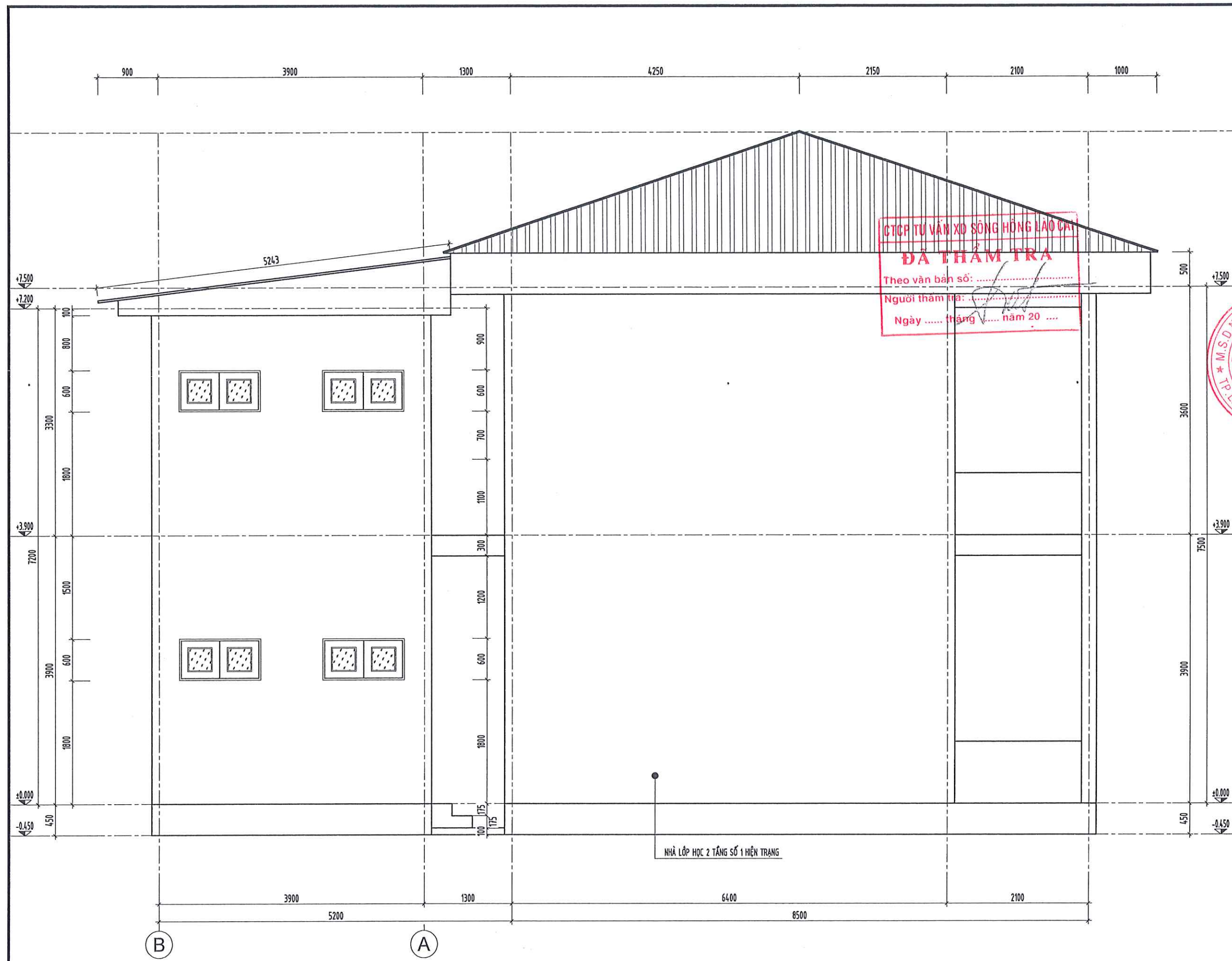
MẶT ĐỨNG B - A NHÀ VỆ SINH
