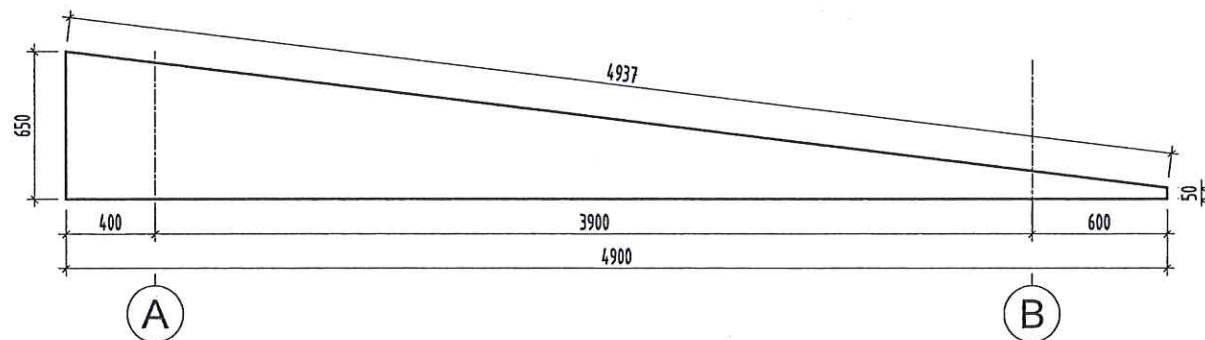
CHI TIẾT TƯỜNG THU HỒI NHÀ VỆ SINH, SL: 04
