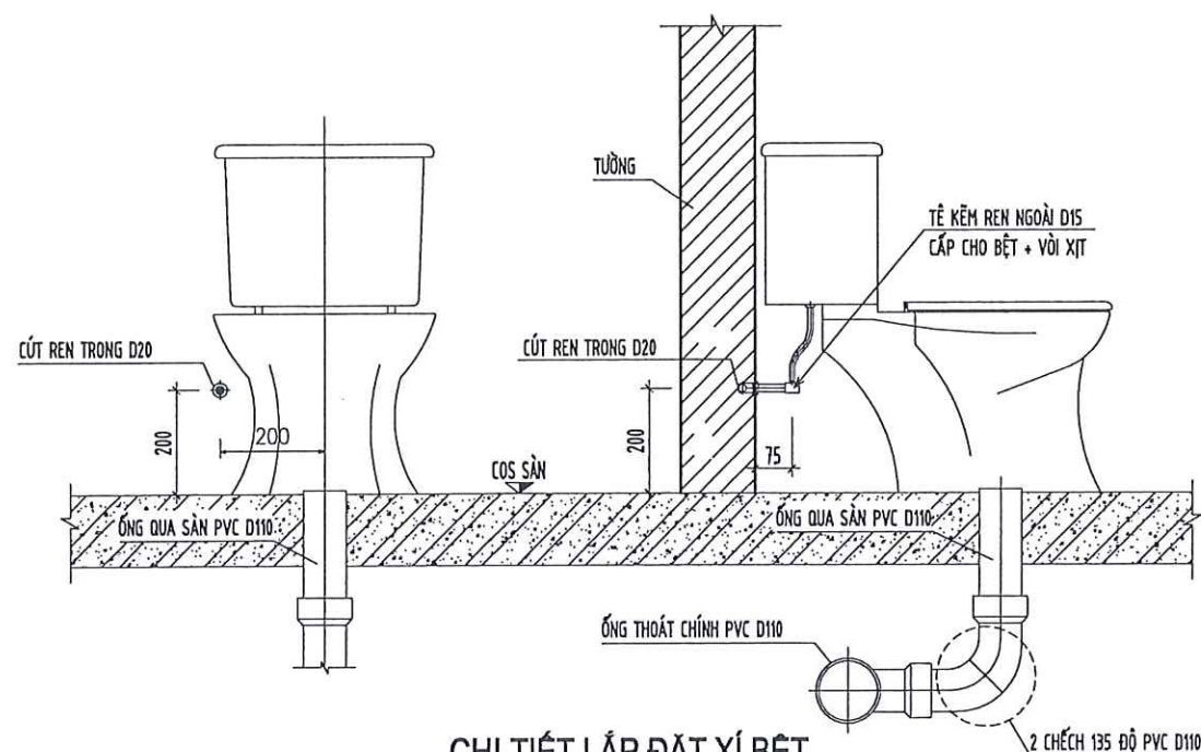
CHI TIẾT LẮP ĐẶT XI BỆT
