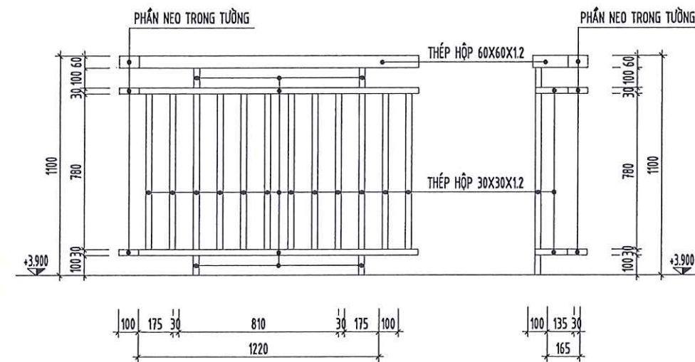
MẶT ĐỨNG LAN CAN 2
