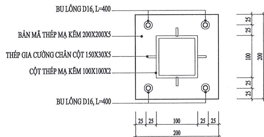
CHI TIẾT CHÂN CỘT
