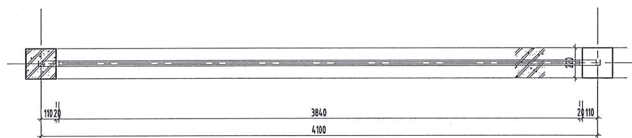
MẶT BẰNG ĐIỂN HÌNH ĐOẠN HÀNG RÀO C - D (L = 4.1M)
