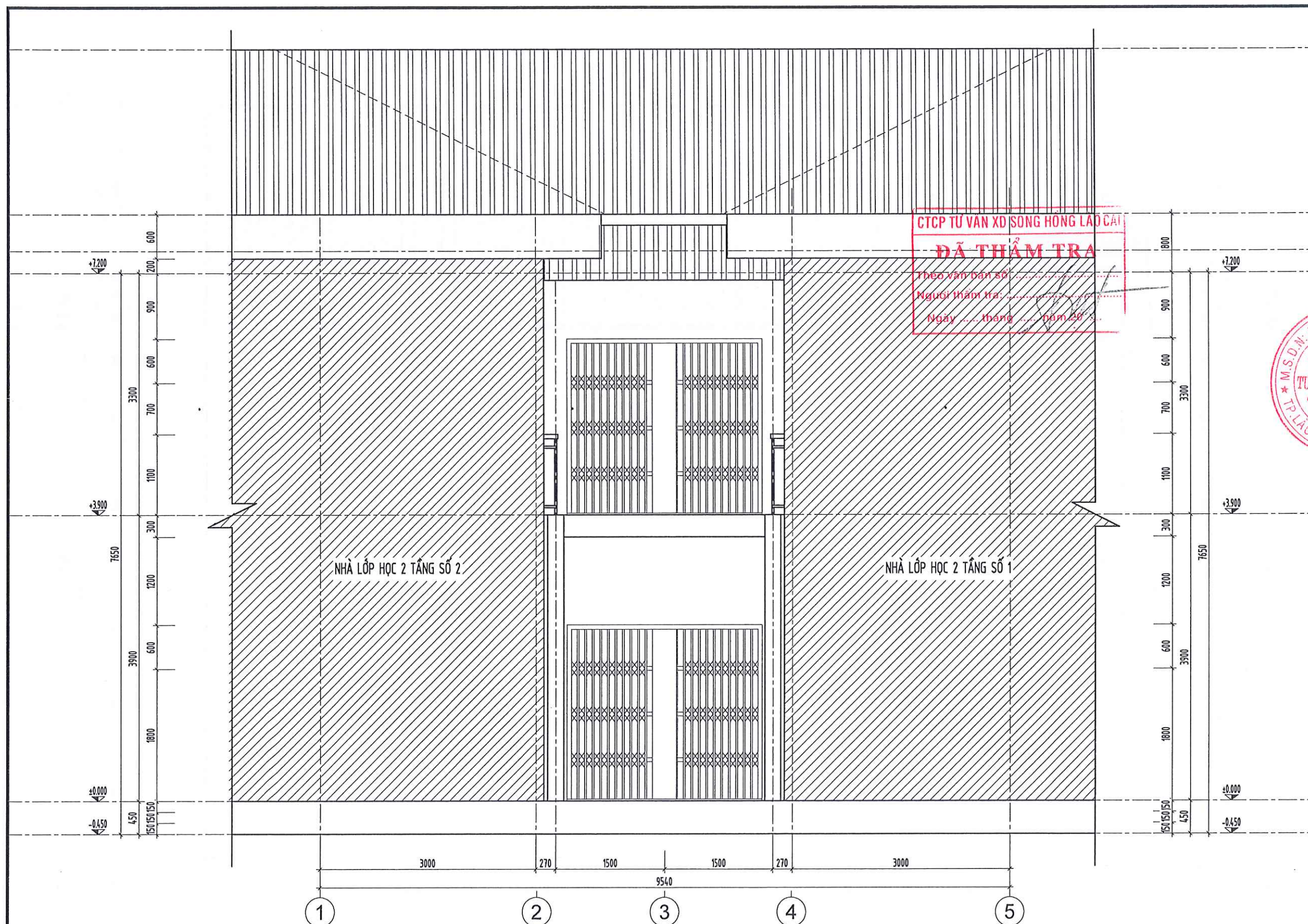
MẶT ĐƯNG 1 - 5 NHÀ VỆ SINH
