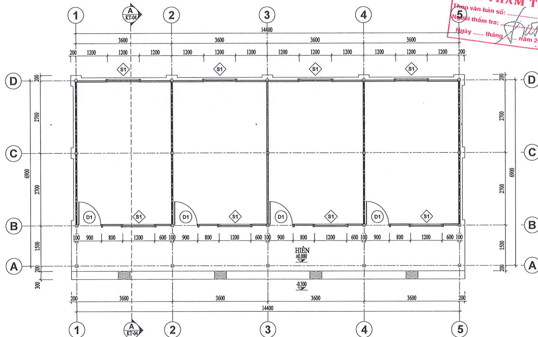
MẶT BẰNG NHÀ BÁN TRÚ PHÁ DỠ
