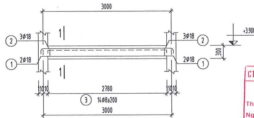
D6-1 (SL= 02, L= 3.22m)
