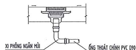
CHI TIẾT LẮP ĐẶT PHỄU THU NƯỚC SÀN
