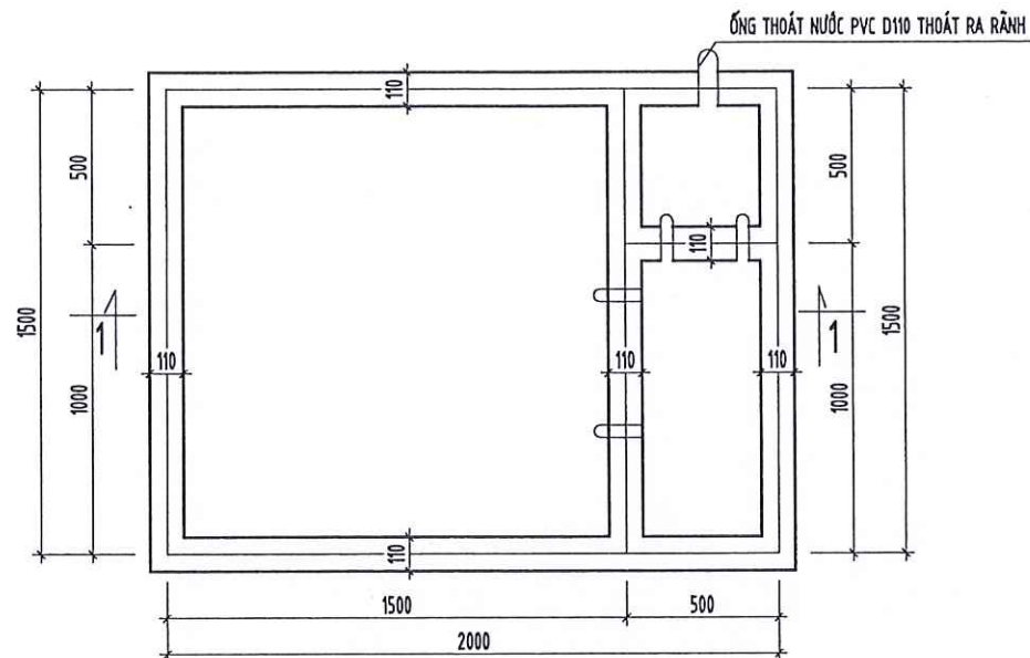
MẶT BẰNG BÊ TỰ HOẠI
