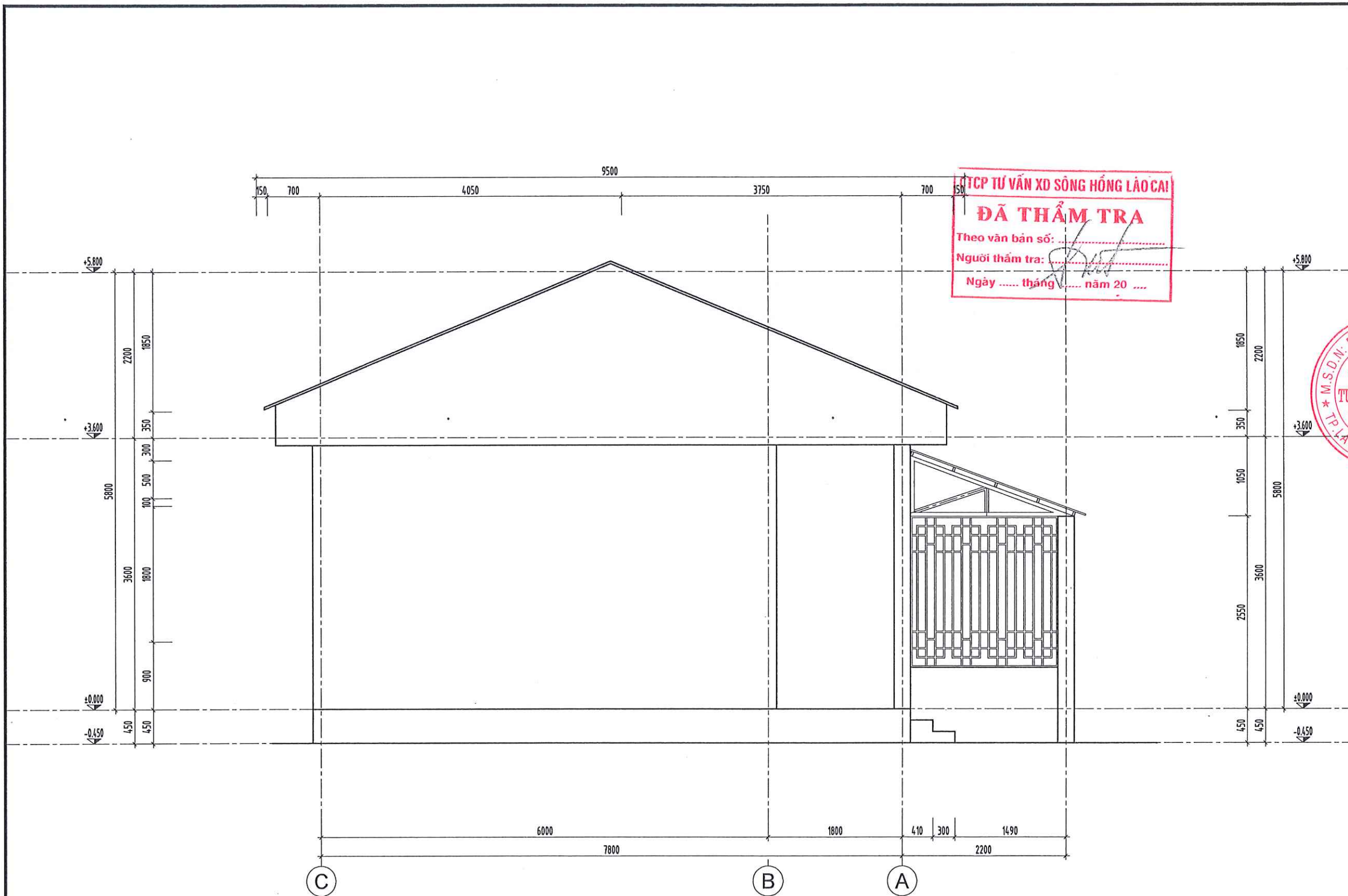
MẶT ĐỨNG C- A NHÀ BÁN TRÚ SỐ 3
