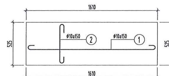
NẮP TẤM ĐẠN BÊ TỰ HOẠI (DÂY 100, 4 TẤM)
