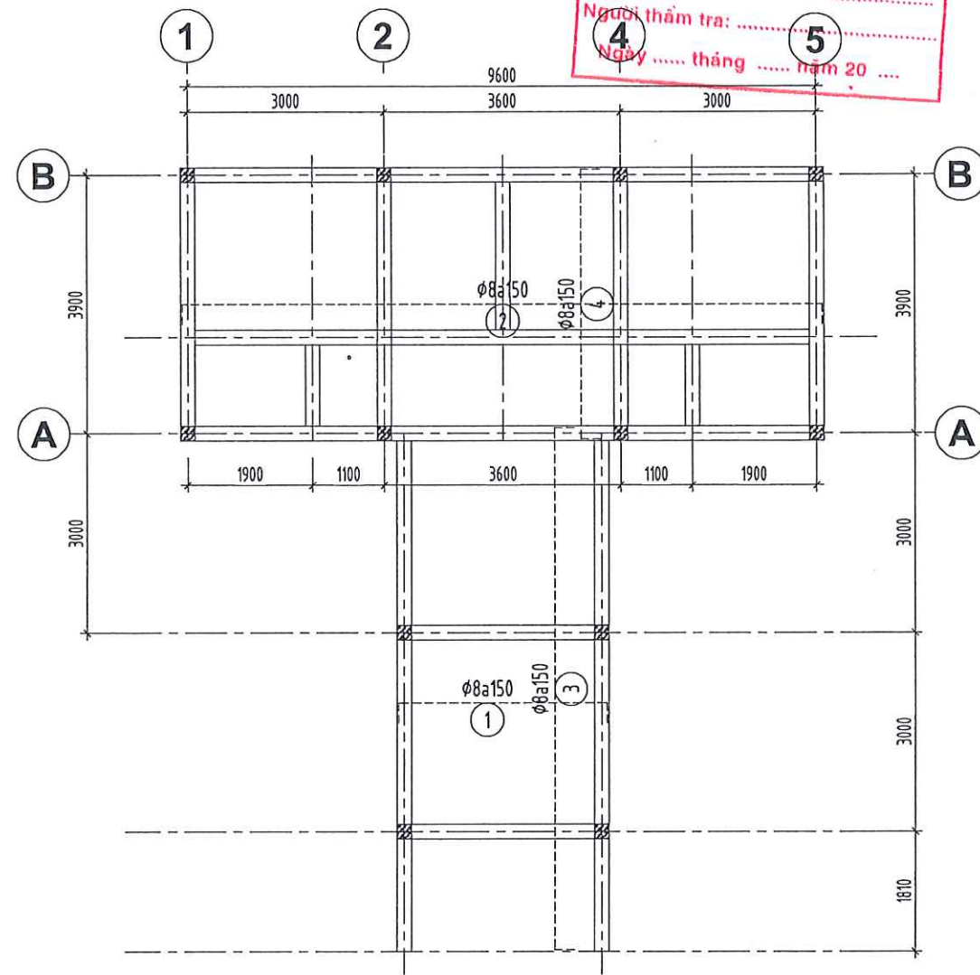
MẶT BẰNG THÉP SÀN LỚP TRÊN CỐT +3.900
