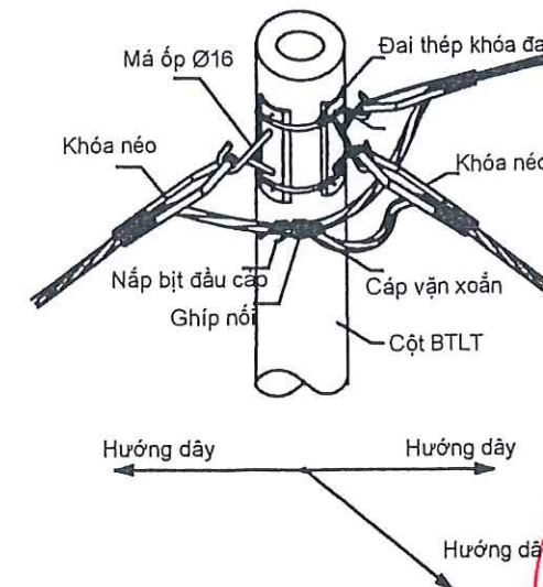
VỊ TRÍ CỘT NEO NHÁNH RẼ
