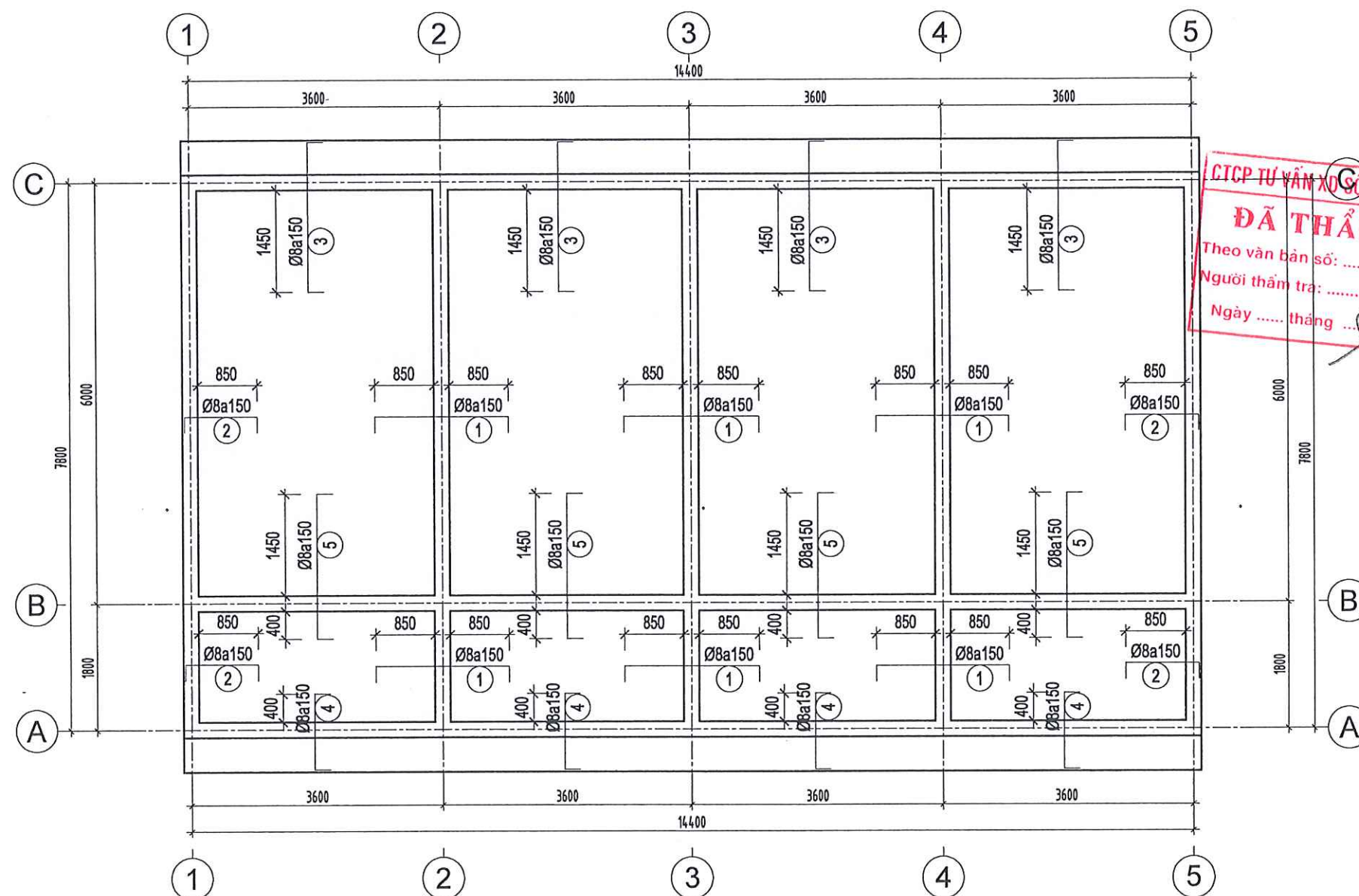
MẶT BẰNG THÉP MÁI NHÀ BÁN TRÚ SỐ 3
