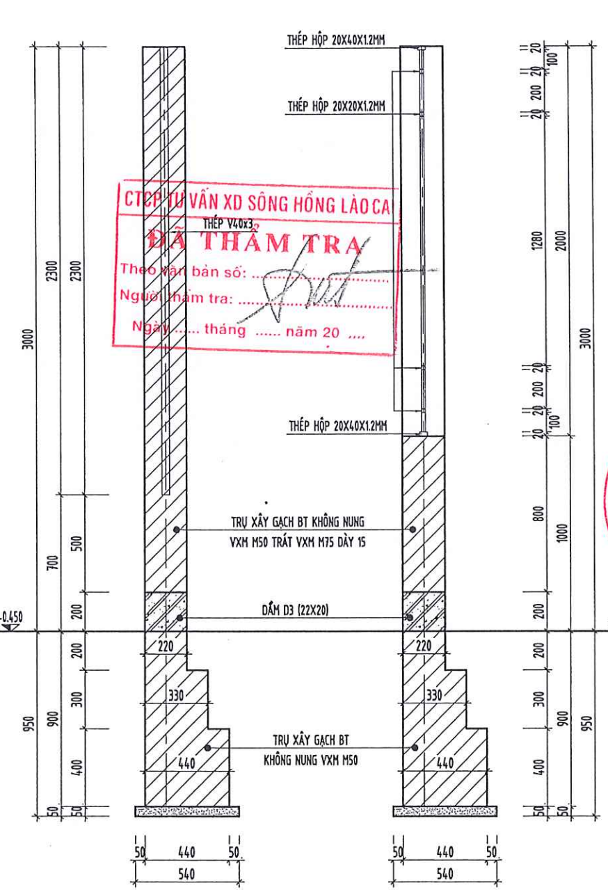
MẶT CẮT 1 - 1
