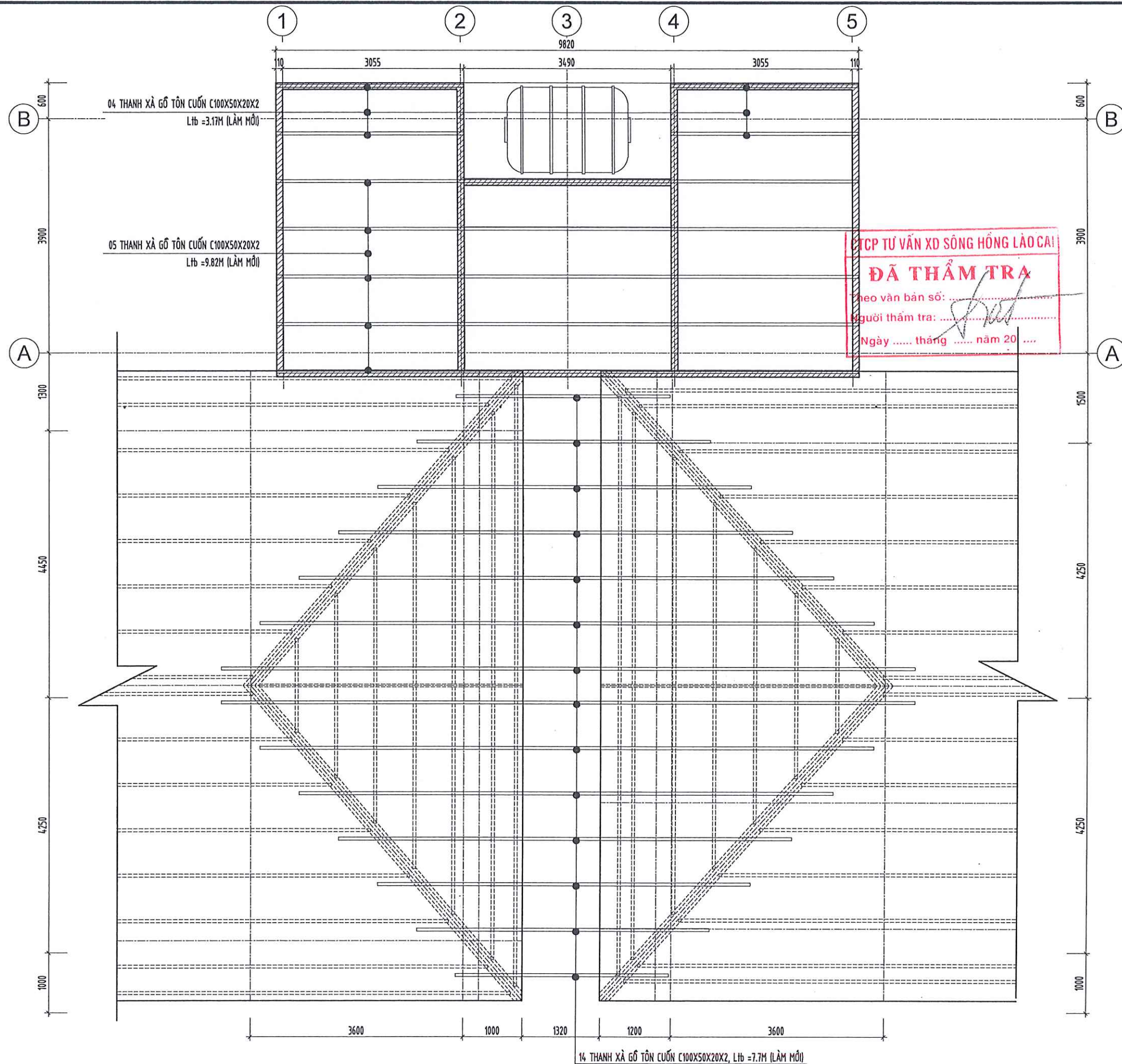
MẶT BẰNG VÌ KÈO + TƯỜNG THU HỒI NHÀ VỆ SINH + MÁI NỐI GIỮA 2 NHÀ LỚP HỌC
