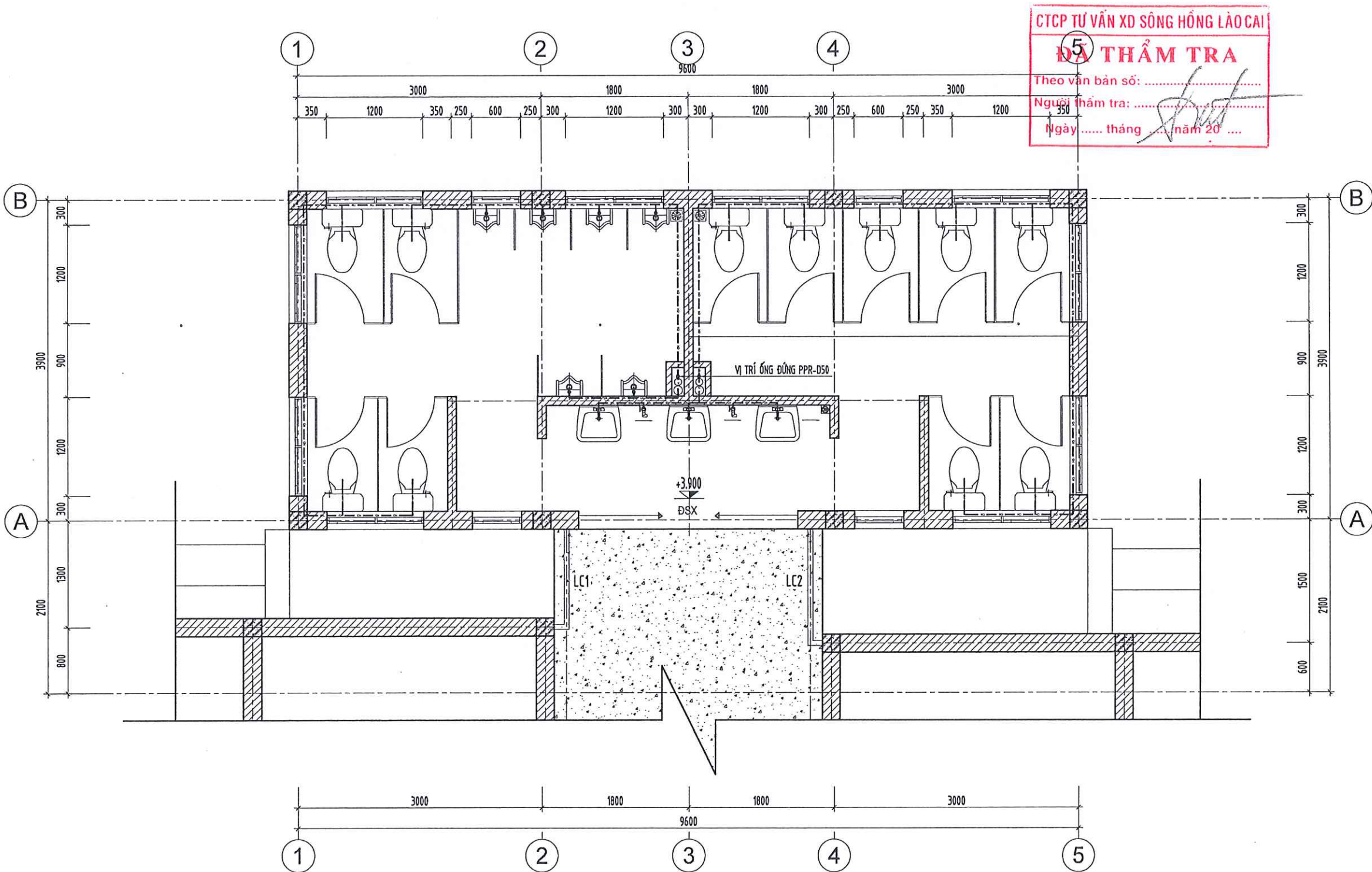
MẶT BẰNG CẤP NƯỚC TẦNG 2
