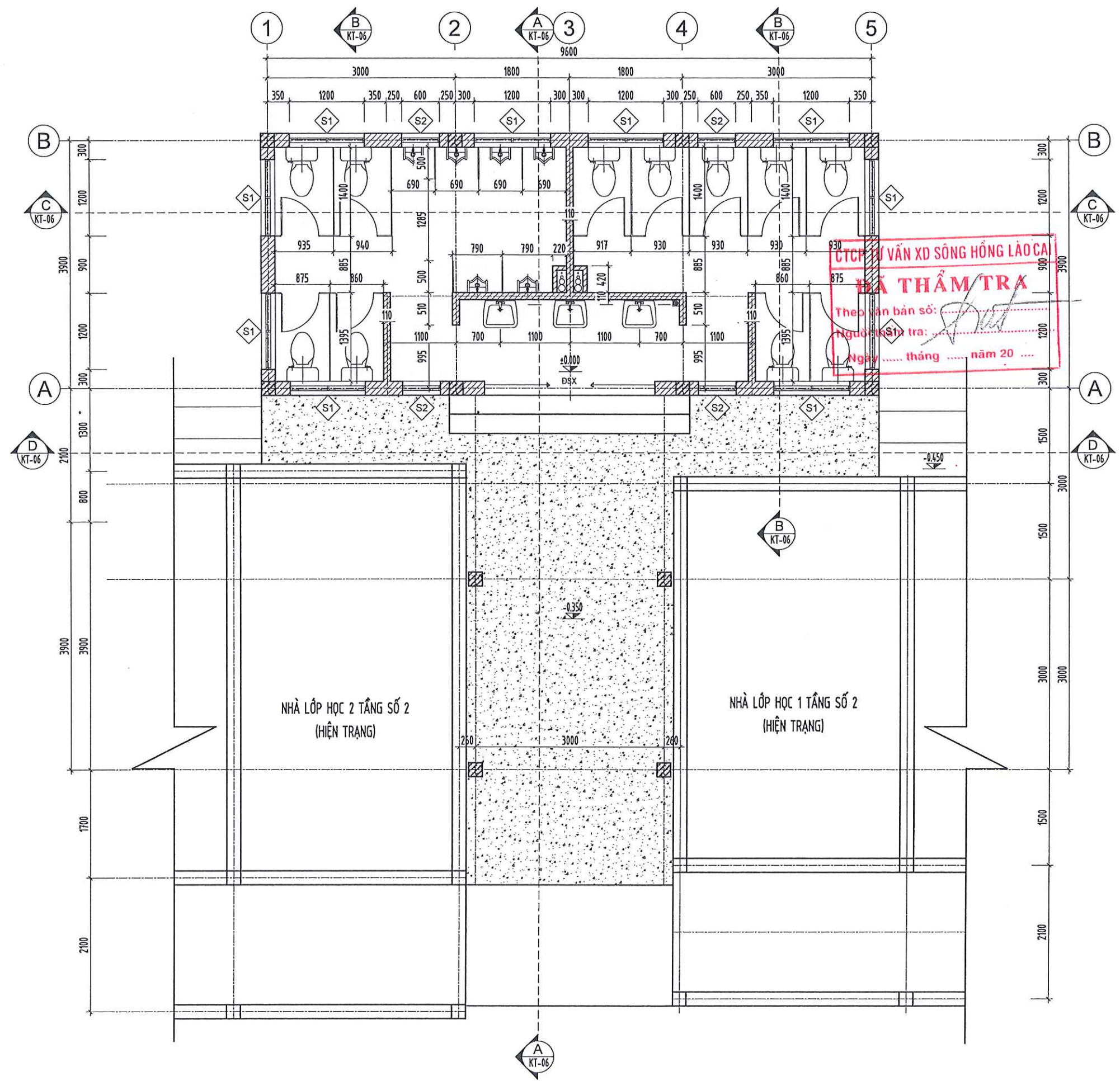
MẶT BẰNG TẦNG 1 NHÀ VỆ SINH + NHÀ CẦU
