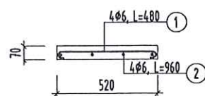
MẶT CẮT 3-3
