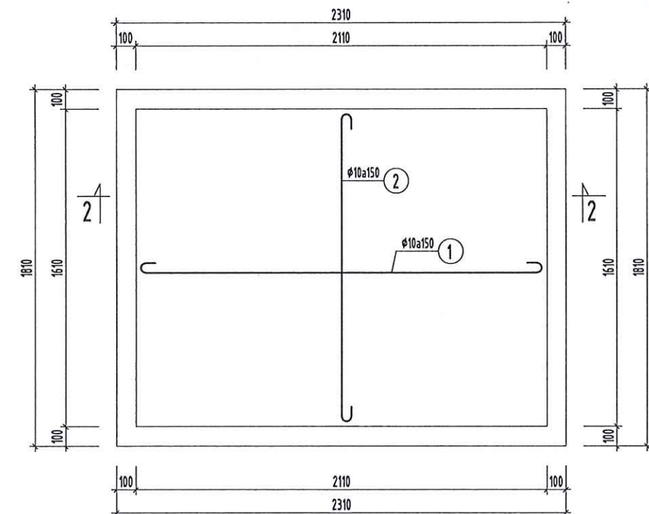
MẶT BẰNG BỐ TRÍ THÉP ĐÁY BÊ TỰ HOẠI
