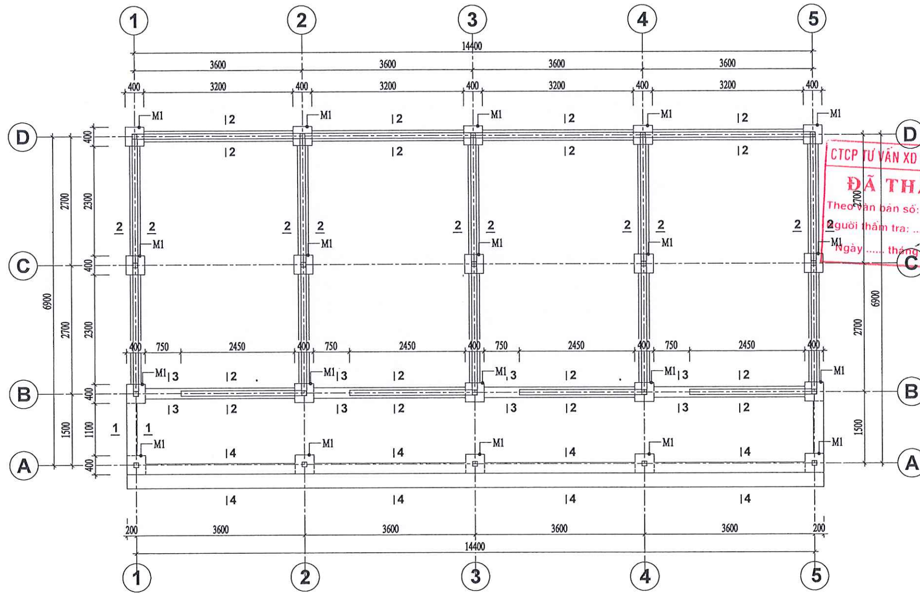
MẶT BẰNG MÓNG
