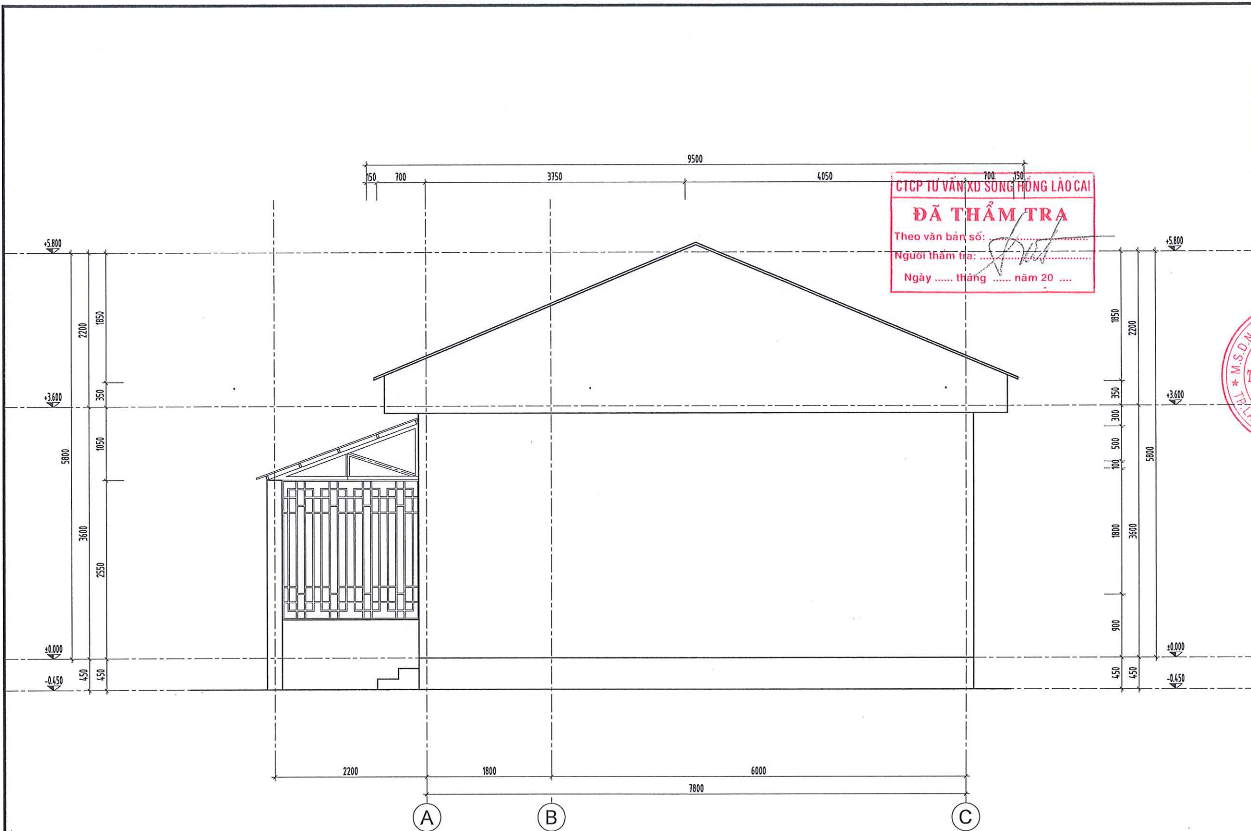
MẶT ĐỨNG A - C NHÀ BÁN TRÚ SỐ 3
