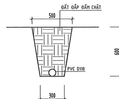
MC RÃNH CHÔN ỐNG THOÁT NƯỚC D110 (L=20m)
