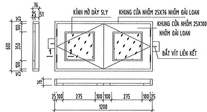
CHI TIẾT CỬA SỔ MỜ 2 CÁNH S1 (SL:20 BỘ)
