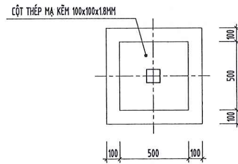
MÓNG M1 (18 CK)
