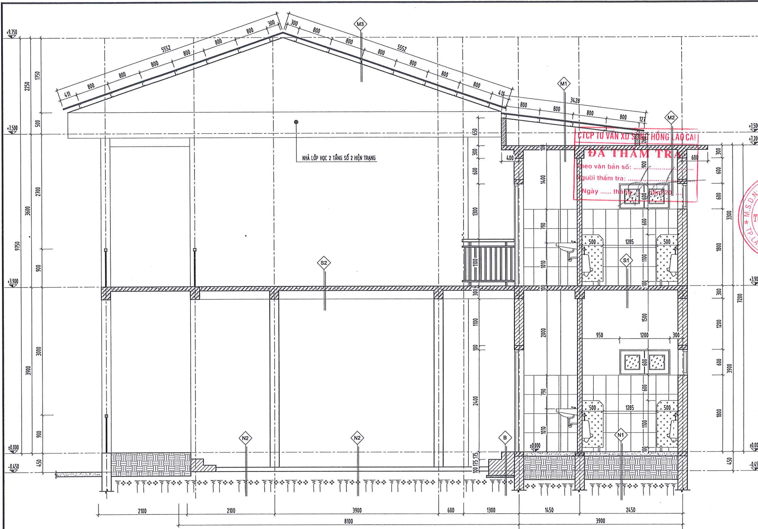
MẶT CẮT A - A
