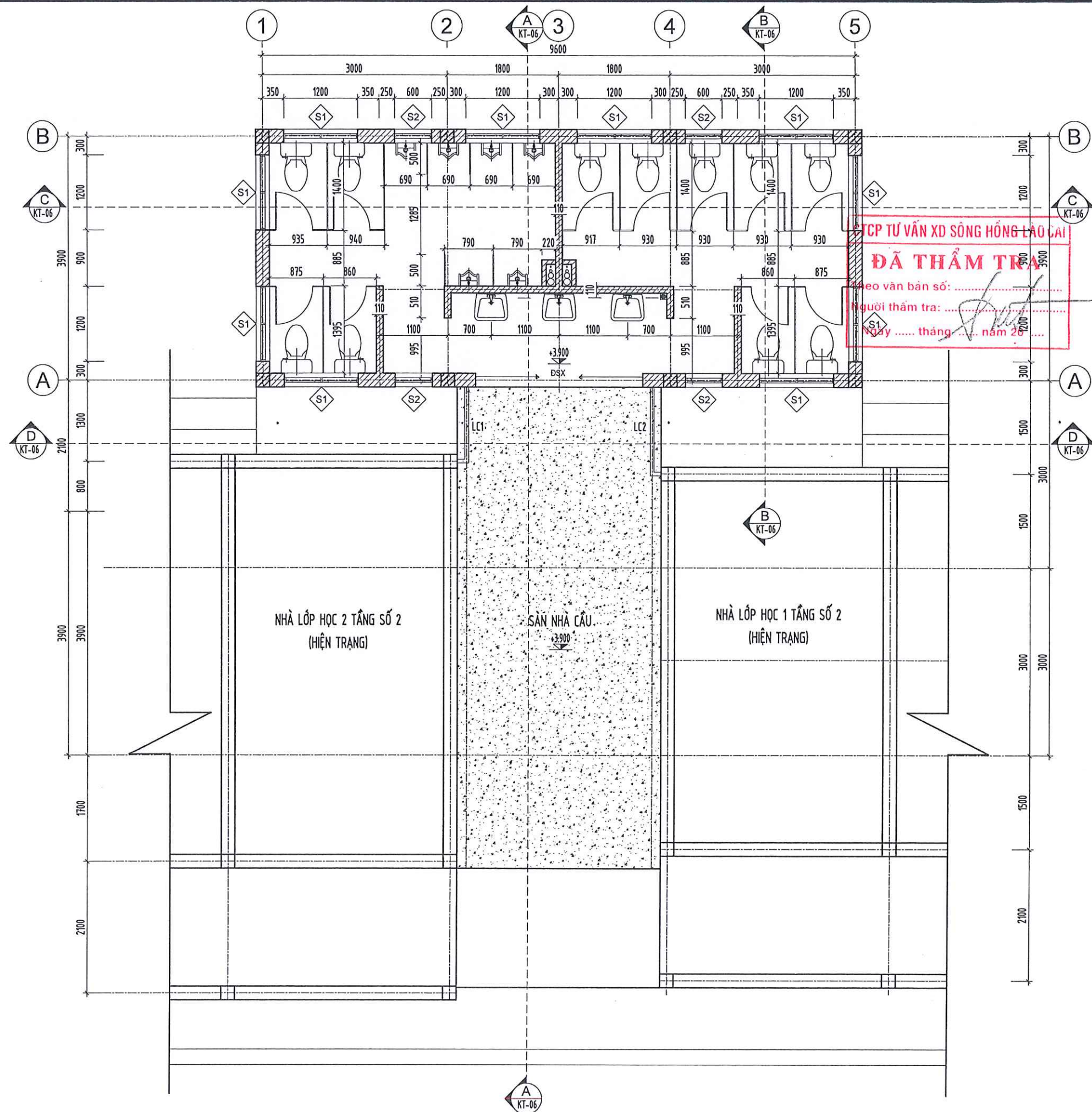
MẶT BẰNG TẦNG 1 NHÀ VỆ SINH + NHÀ CẦU
