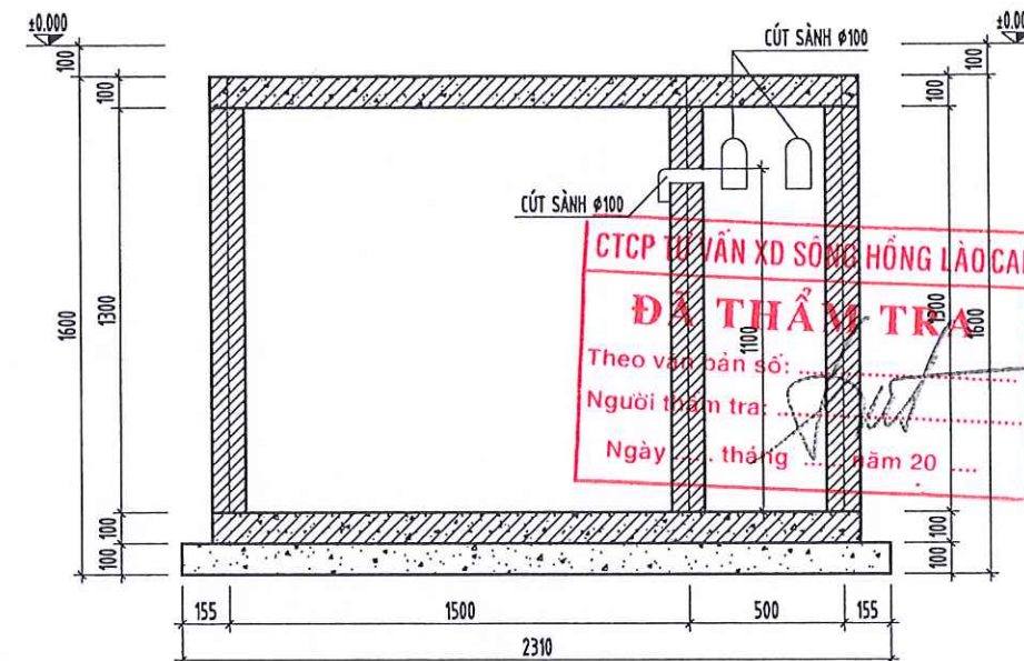
MẶT CẮT 1-1
