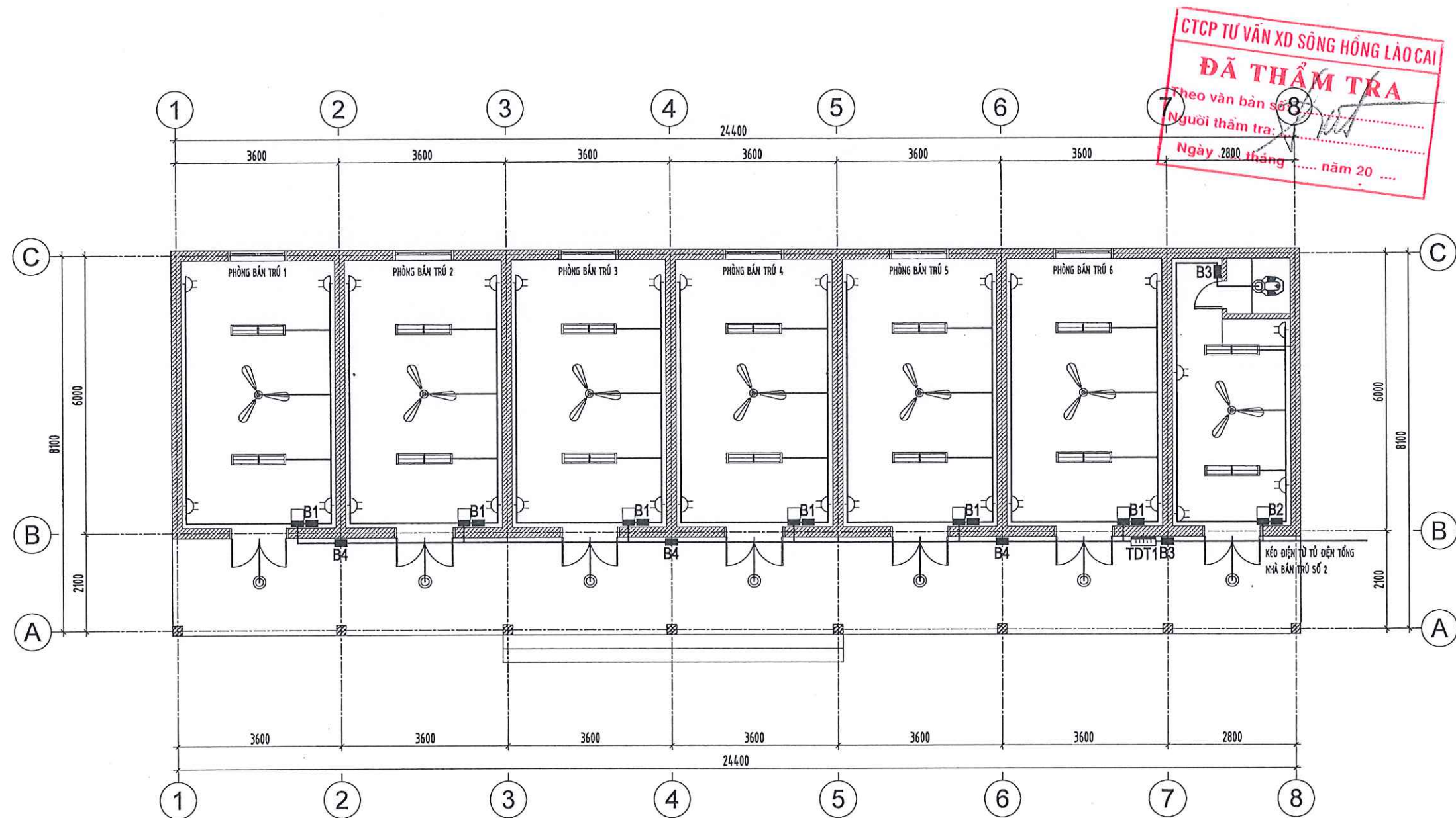
MẶT BẰNG CẤP ĐIỆN NHÀ BÀN TRÚ SỐ 1
