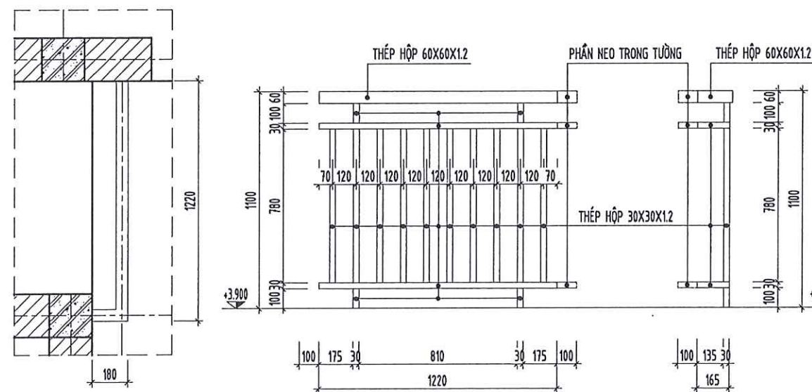
MẶT ĐỨNG LAN CAN 1
