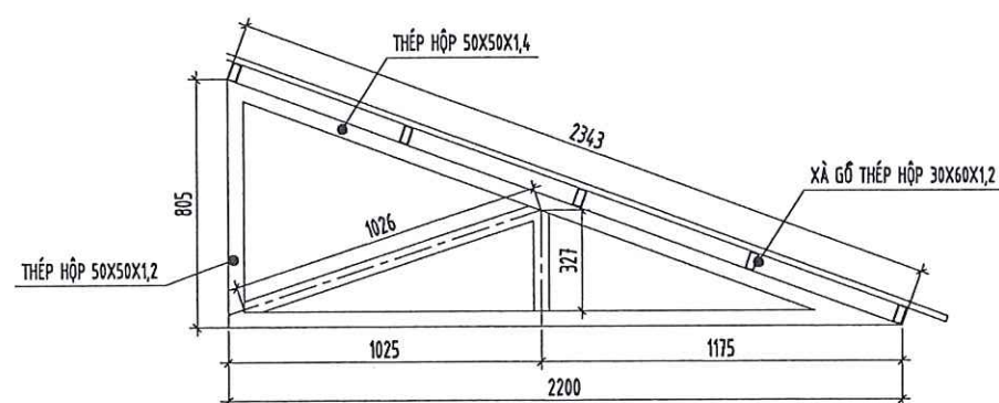
CHI TIẾT VÌ KÈO 1 (SL:05)
