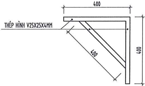
CHI TIẾT CON SON ĐÓN ĐIỆN
