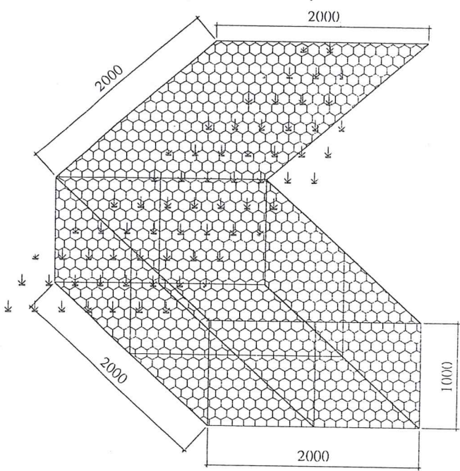
PHỐI CẢNH RỌ ĐÁ
