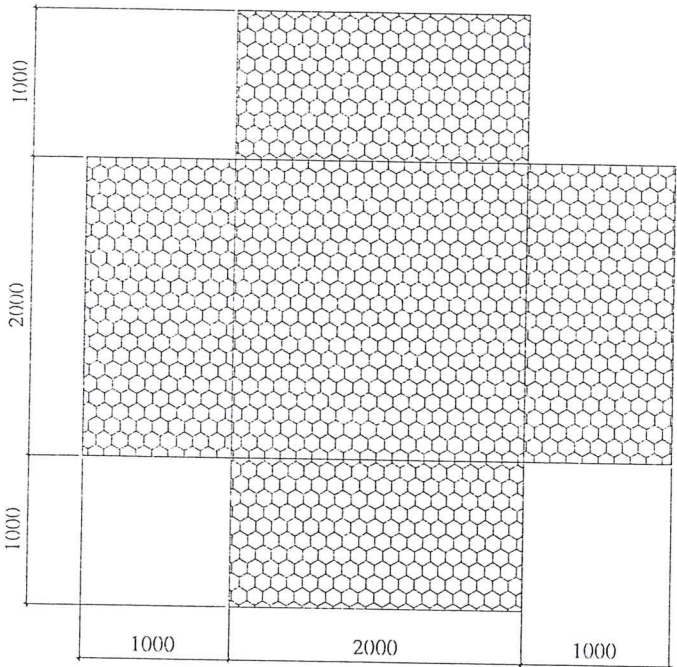
LƯỚI RỌ ĐÁ
