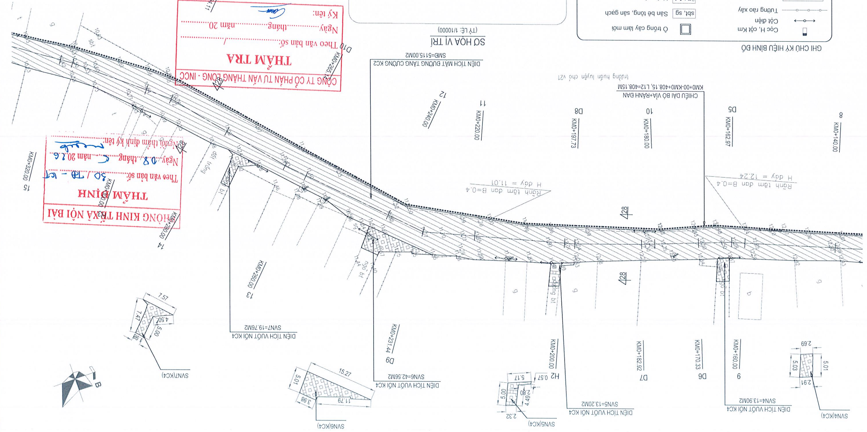
BÌNH DỒ THIẾT KẾ TUYẾN 6 (TỶ LỆ: 1/500)
