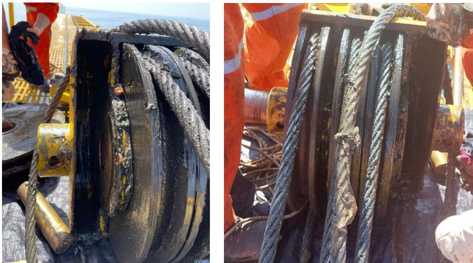
Kiểm tra cụm puly động cáp giăng cần không phát hiện dị vật gây kẹt – mài mòn cáp. Các puly quay tốt, không bị kẹt (Puly NYCAST).
