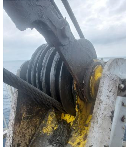
Cụm puly cáp giăng cân đỉnh tháp chữ A quay tốt, không bị kẹt ( Puly NYCAST)
