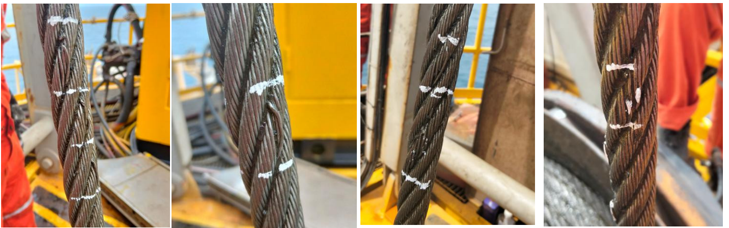
Một số hình ảnh tình trạng cáp bị đứt.
