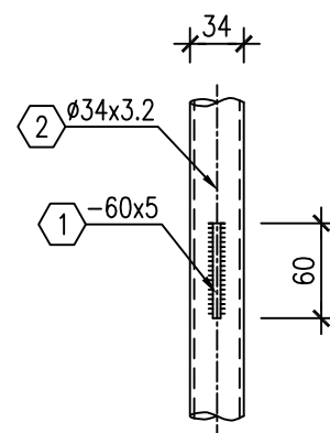
MẶT CẮT 4 - 4
