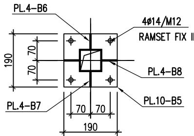
MẶT CẮT 5-5
