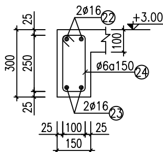
MẶT CẮT 12-12 (D4 150X300, SL=01)
