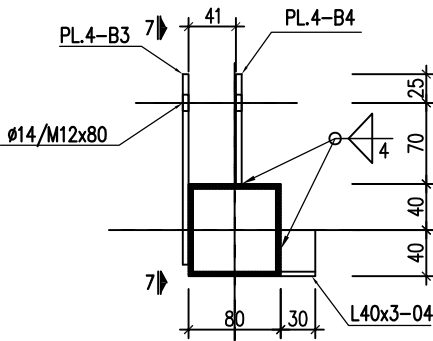
MẶT CẮT 7-7
