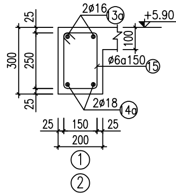
MẶT CẮT 2A-2A (D2 200X300, SL=02)
