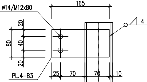
MẶT CẮT 7-7
