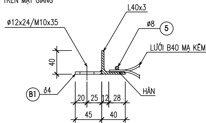
MẶT CẮT 1-1
