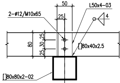
MẶT CẮT 4-4
