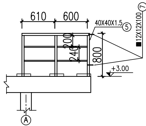
CẤU TẠO LAN CAN HÀNH LANG TRỤC 3
