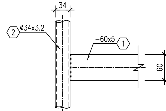
MẶT CẮT 5 - 5
