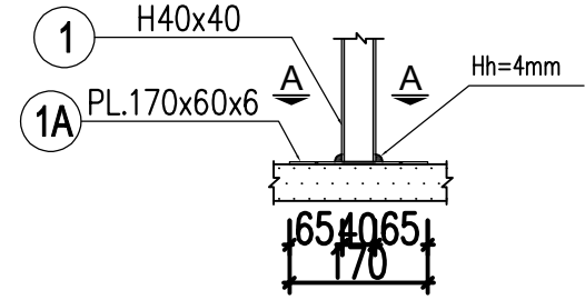
CẤU TẠO CHÂN LAN CAN HÀNH LANG
