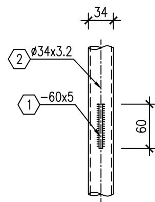
MẶT CẮT 4 - 4
