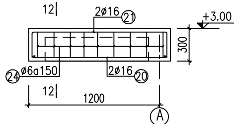
DẦM D4 150X300 (L=1200, SL=01)
