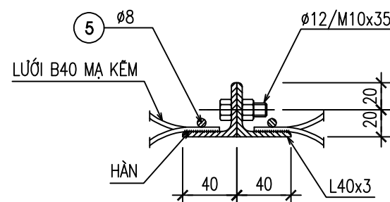
MẶT CẮT 2-2
