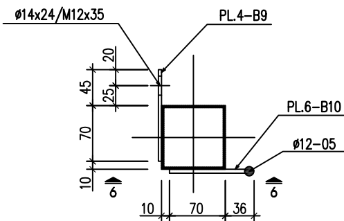
MẶT CẮT 2-2
