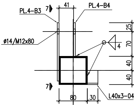
MẶT CẮT 7-7
