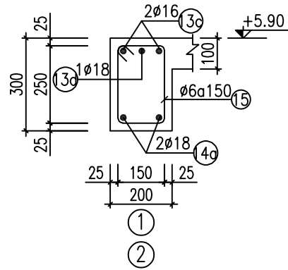
MẶT CẮT 3A-3A (D2 200X300, SL=02)
