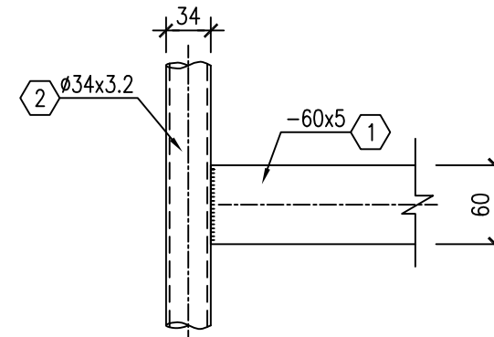
MẶT CẮT 5 - 5
