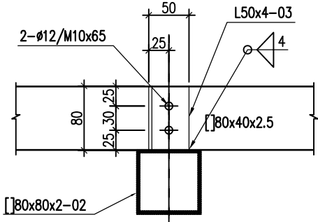
MẶT CẮT 4-4
