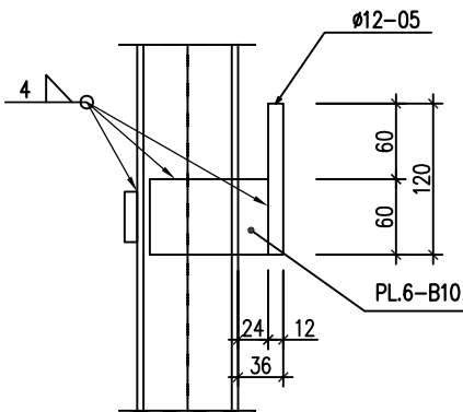
MẶT CẮT 6-6
