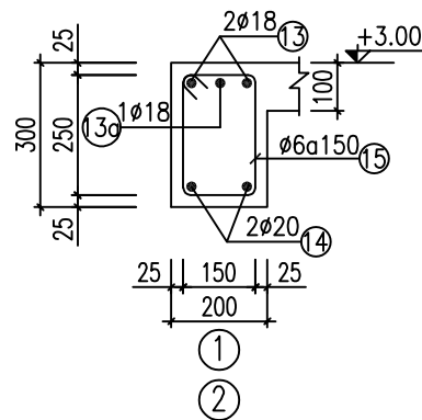
MẶT CẮT 3A-3A (D2 200X300, SL=02)
