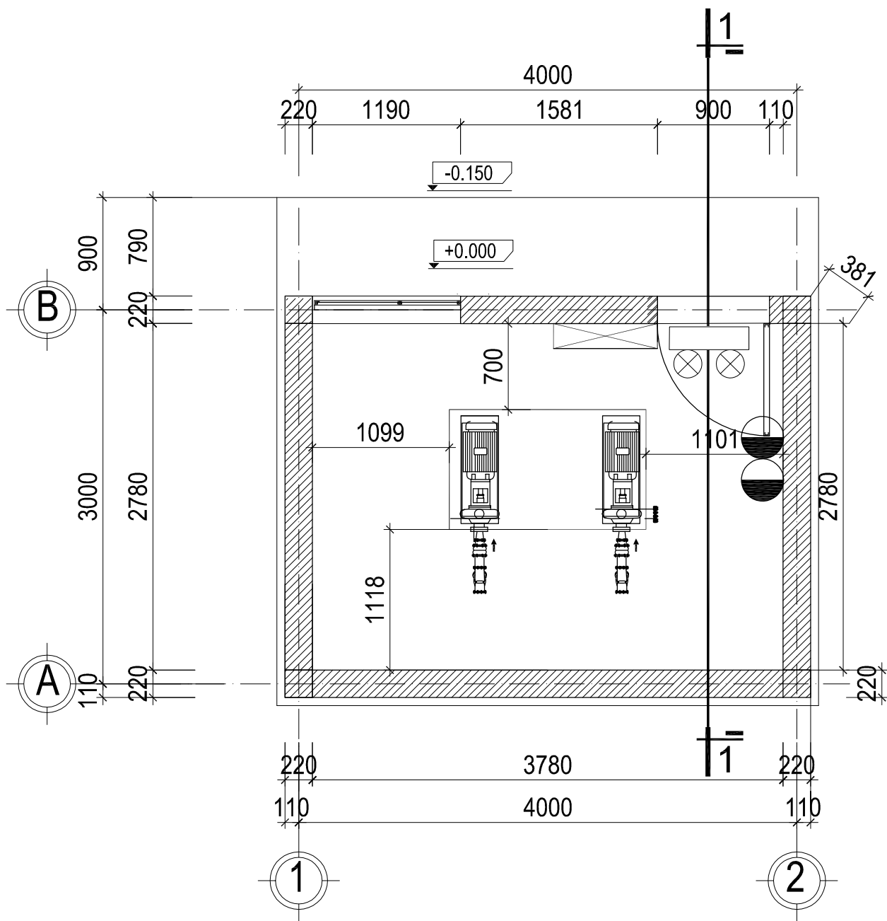
MẶT BẰNG BỐ TRÍ PCCC
