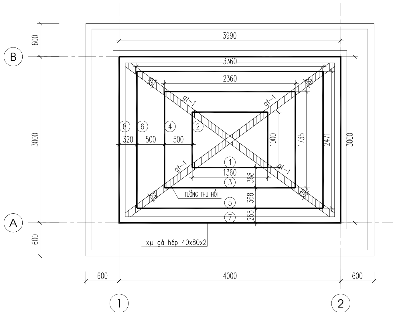
MẶT BẰNG GIẺNG TƯỜNG VÀ XÀ GỖ
