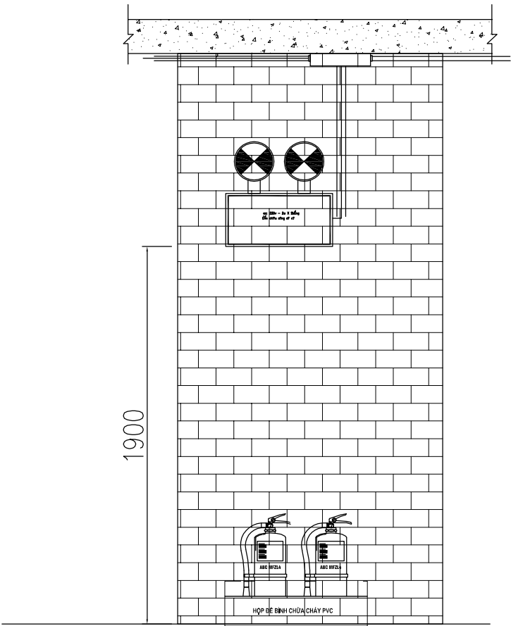
CHI TIẾT LẮP ĐẶT ĐÈN CHIẾU SÁNG SỰ CỐ
