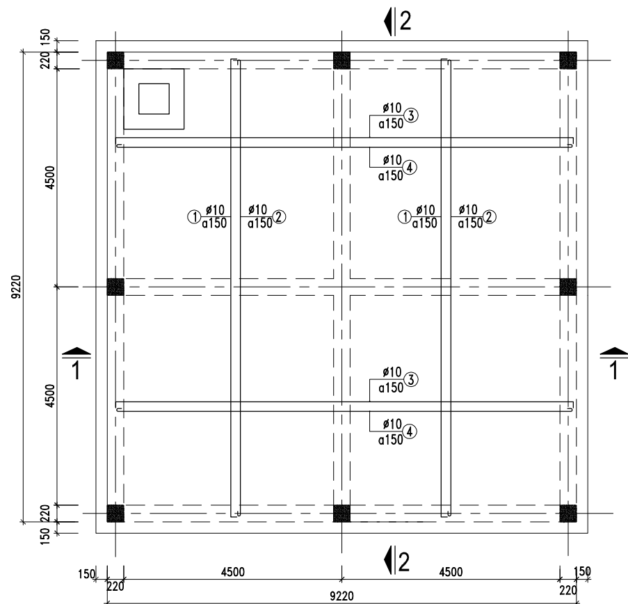
MẶT BẰNG THÉP ĐÁY BỂ NƯỚC NGẦM
