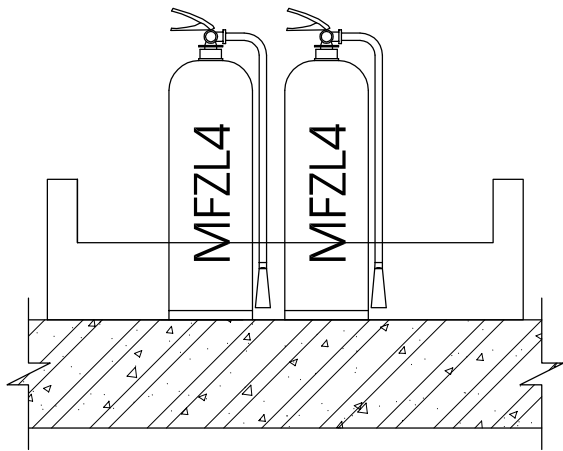
CHI TIẾT TRANG BỊ GIÁ ĐỂ 02 BÌNH MFZL4 - ABC
