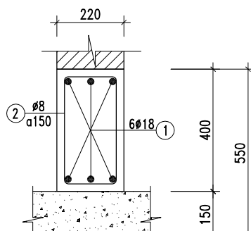
GM1 (L=7220, SL:03C) GM2 (L=7220, SL:03C)
