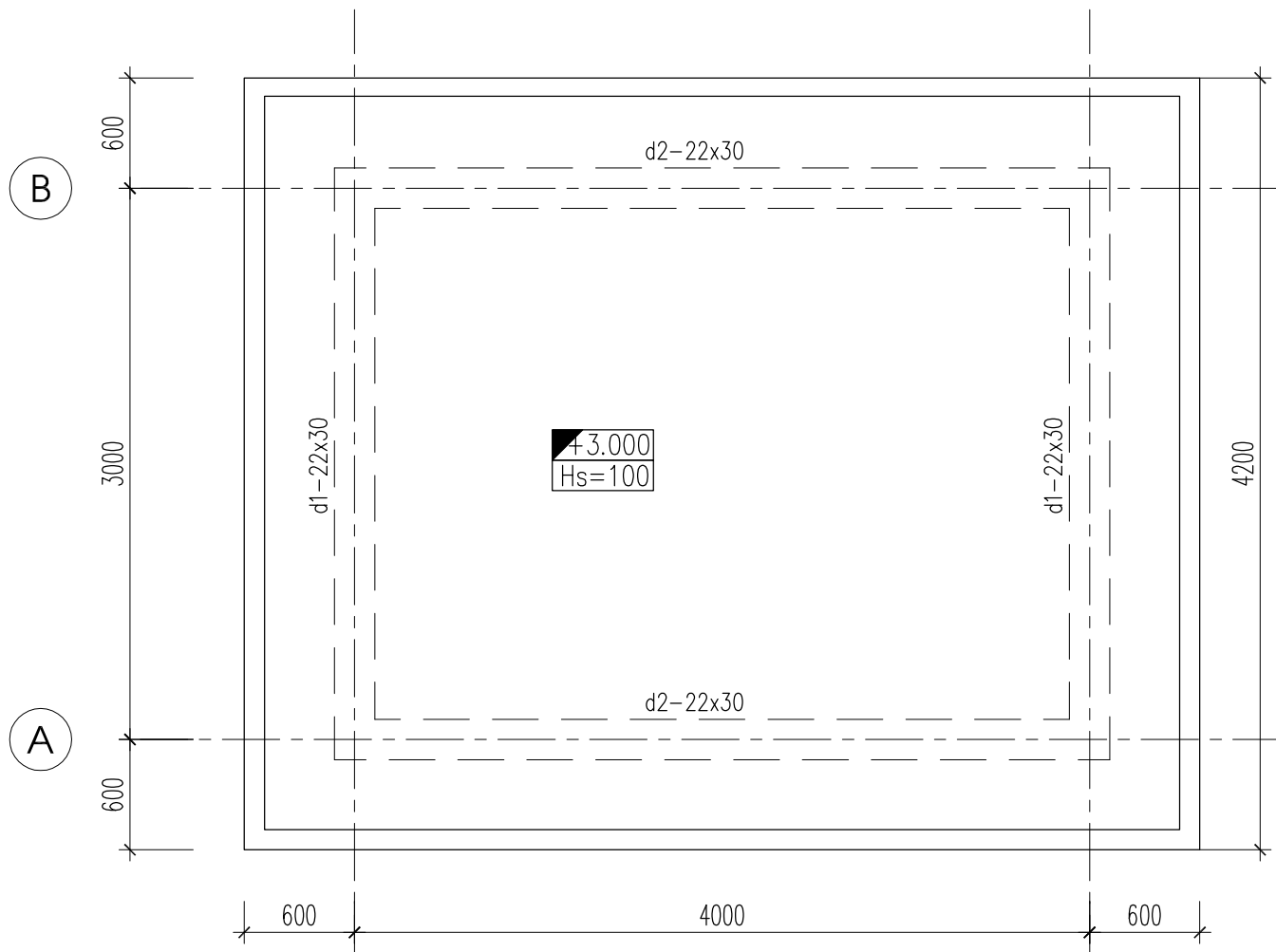
1 MẶT BẰNG KẾT CẤU MÁI
