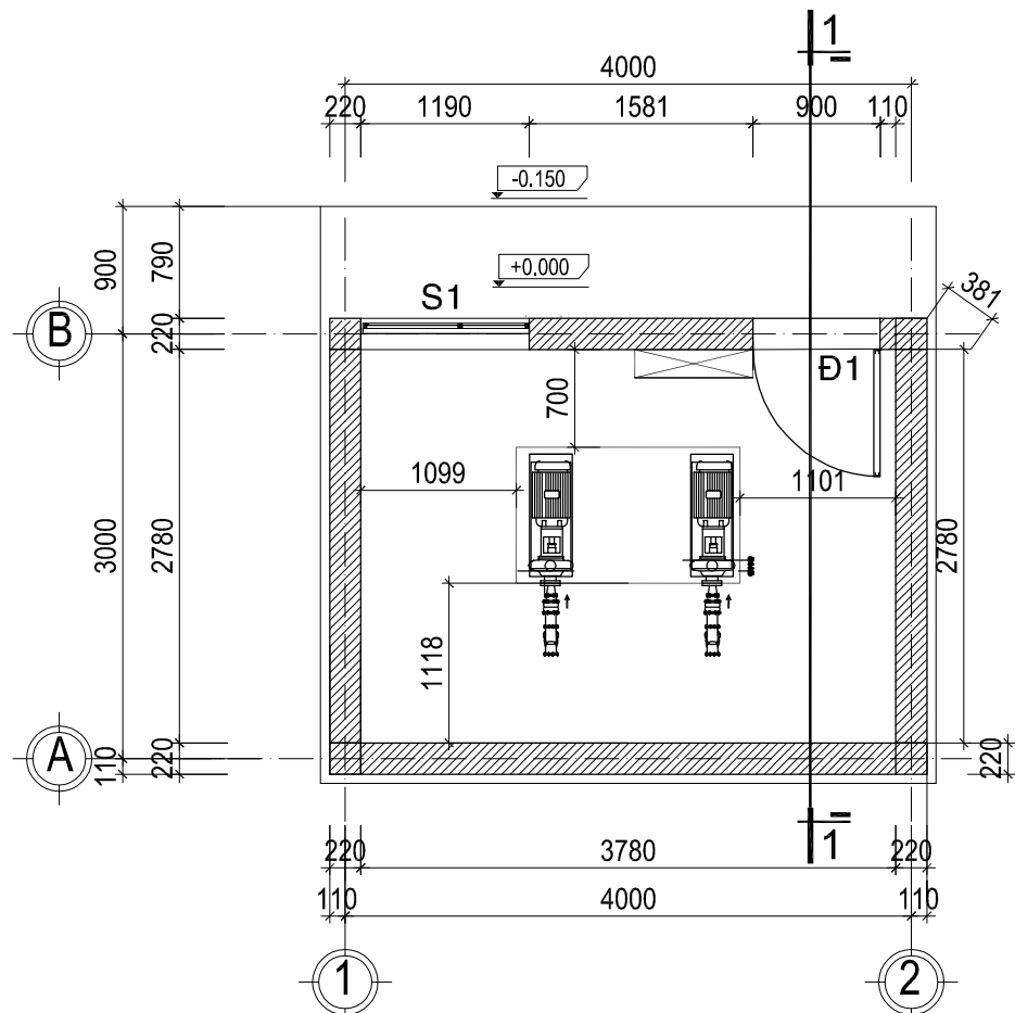
MẶT BẰNG NHÀ TRẠM BƠM
