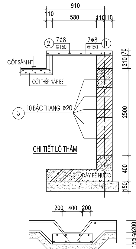
CHI TIẾT CẤU TẠO RỖN BỂ
