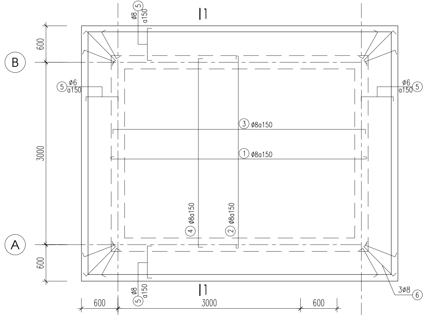
2 MẶT BẰNG THÉP SÀN
