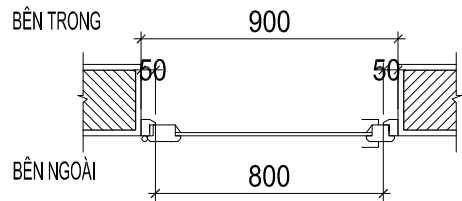
MẶT CẮT 2 - 2
