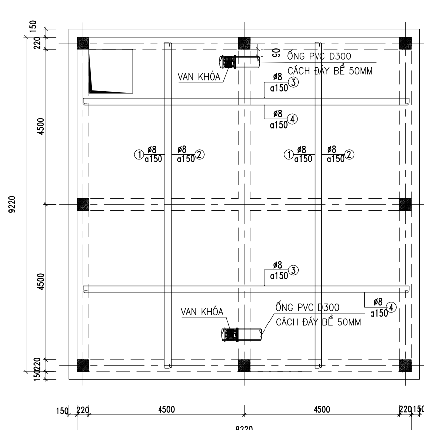
MẶT BẰNG THÉP NẮP BỂ NƯỚC NGẦM
