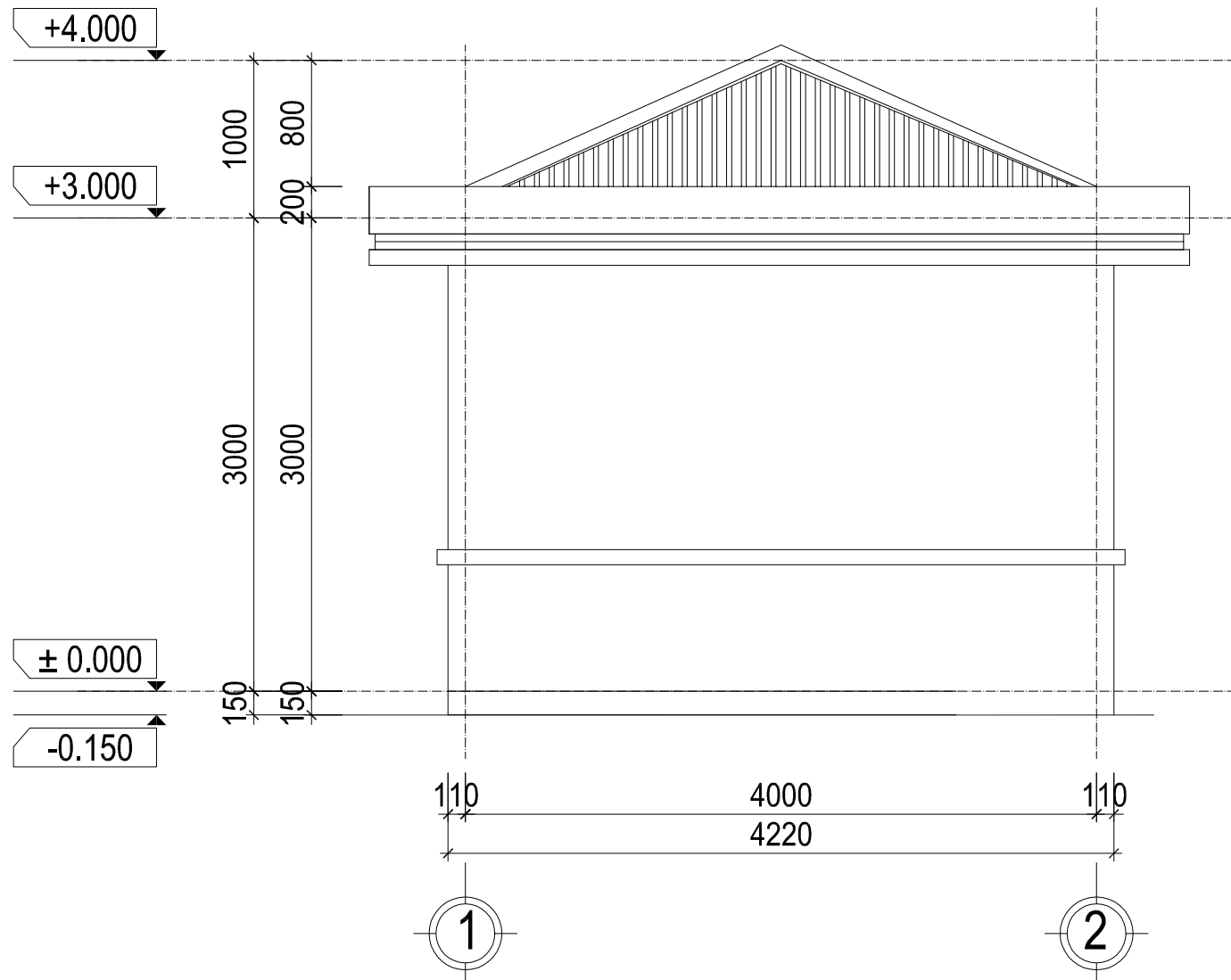
MẶT ĐỨNG TRỰC 1-2
