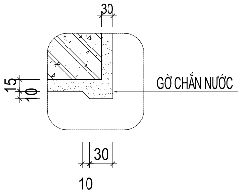
CHI TIẾT CT1
