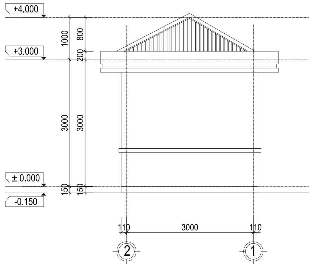
MẶT ĐỨNG TRỰC B-A
