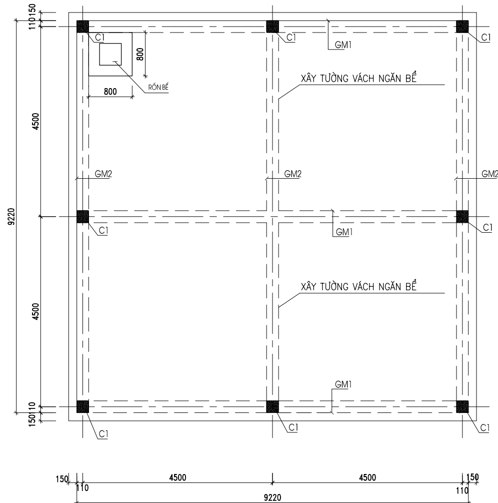
MẶT BẰNG KẾT CẤU ĐÁY BỂ NƯỚC NGẦM
