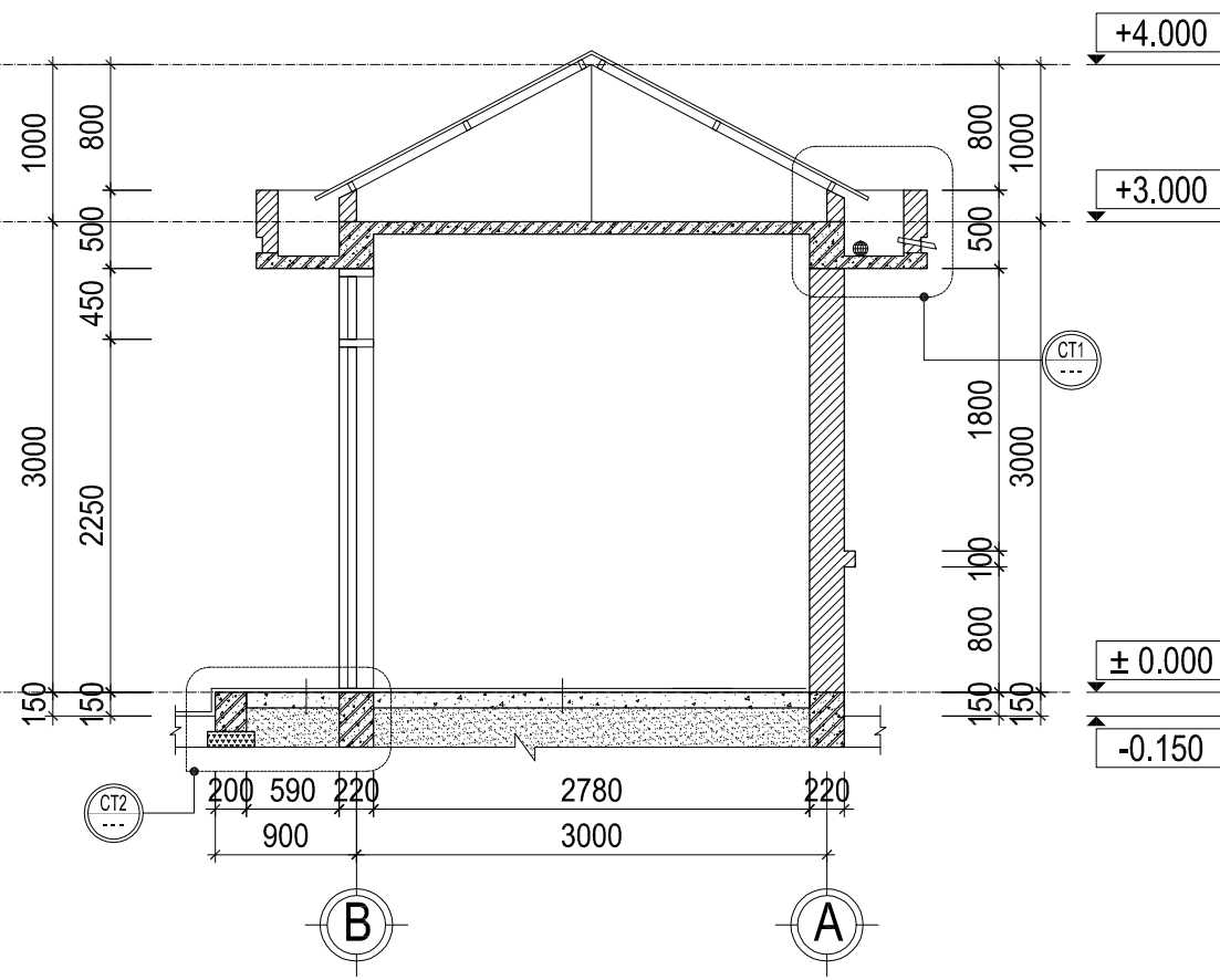
MẶT CẮT 1 - 1
