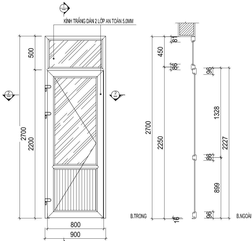
CỬA ĐI D1
