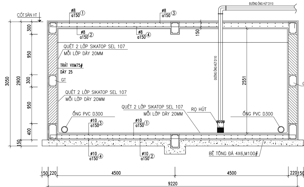
CẮT 2-2
