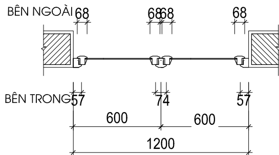
MẶT CẮT 1 - 1
