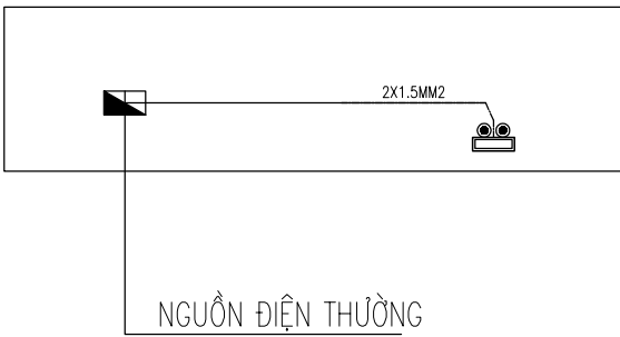
SƠ ĐỒ NGUYÊN LÝ ĐIỆN HÌNH ĐÈN SỰ CỐ
