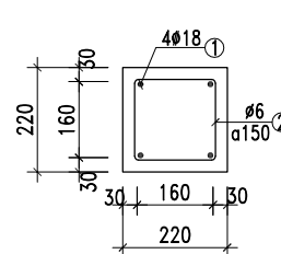
CẮT 1-1
