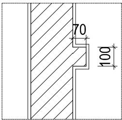
CHI TIẾT GỜ TƯỜNG
