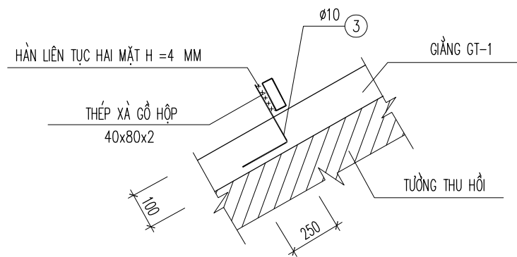
CHI TIẾT LIÊN KẾT GIẺNG VÀ XÀ GỖ
