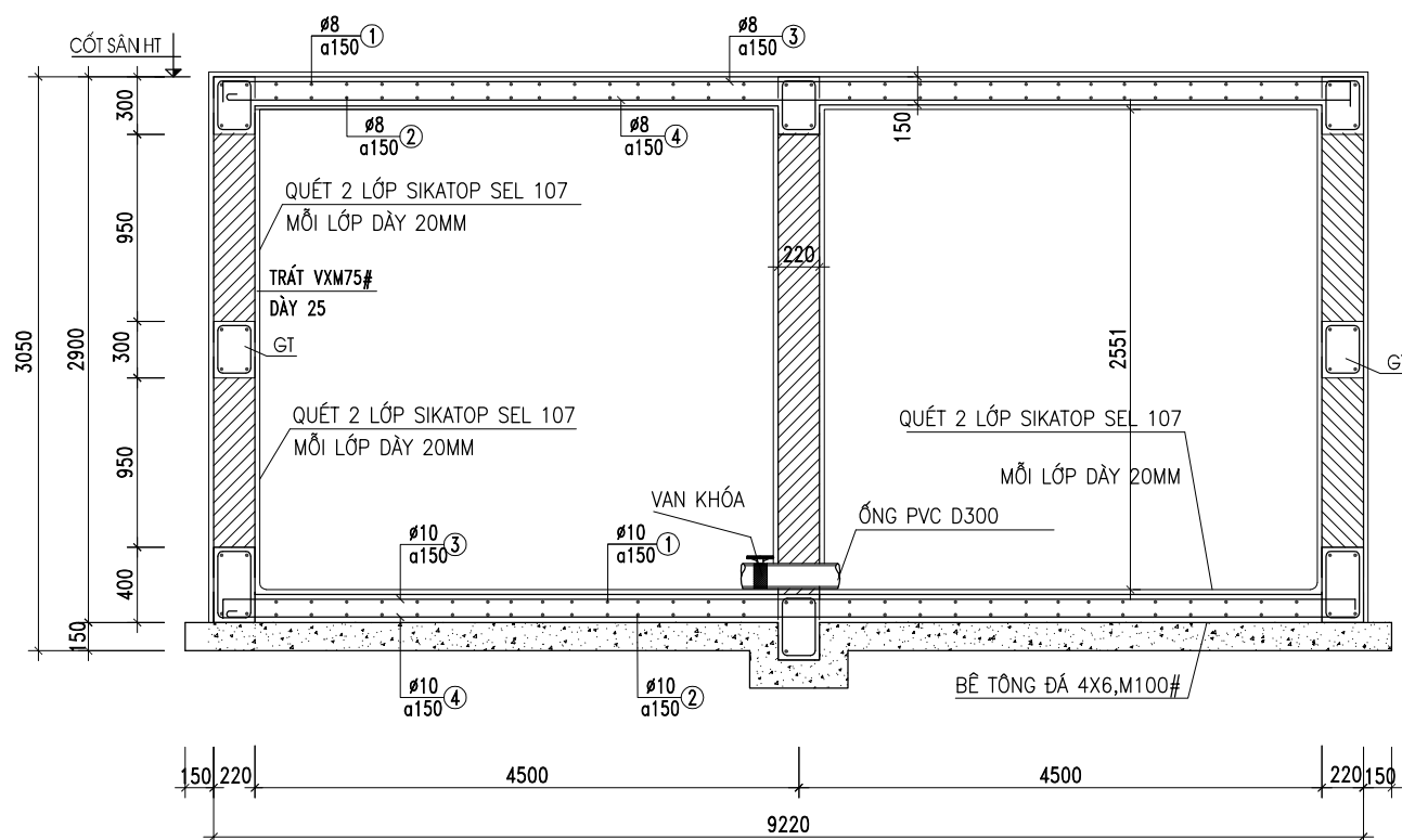
CẮT 1-1
