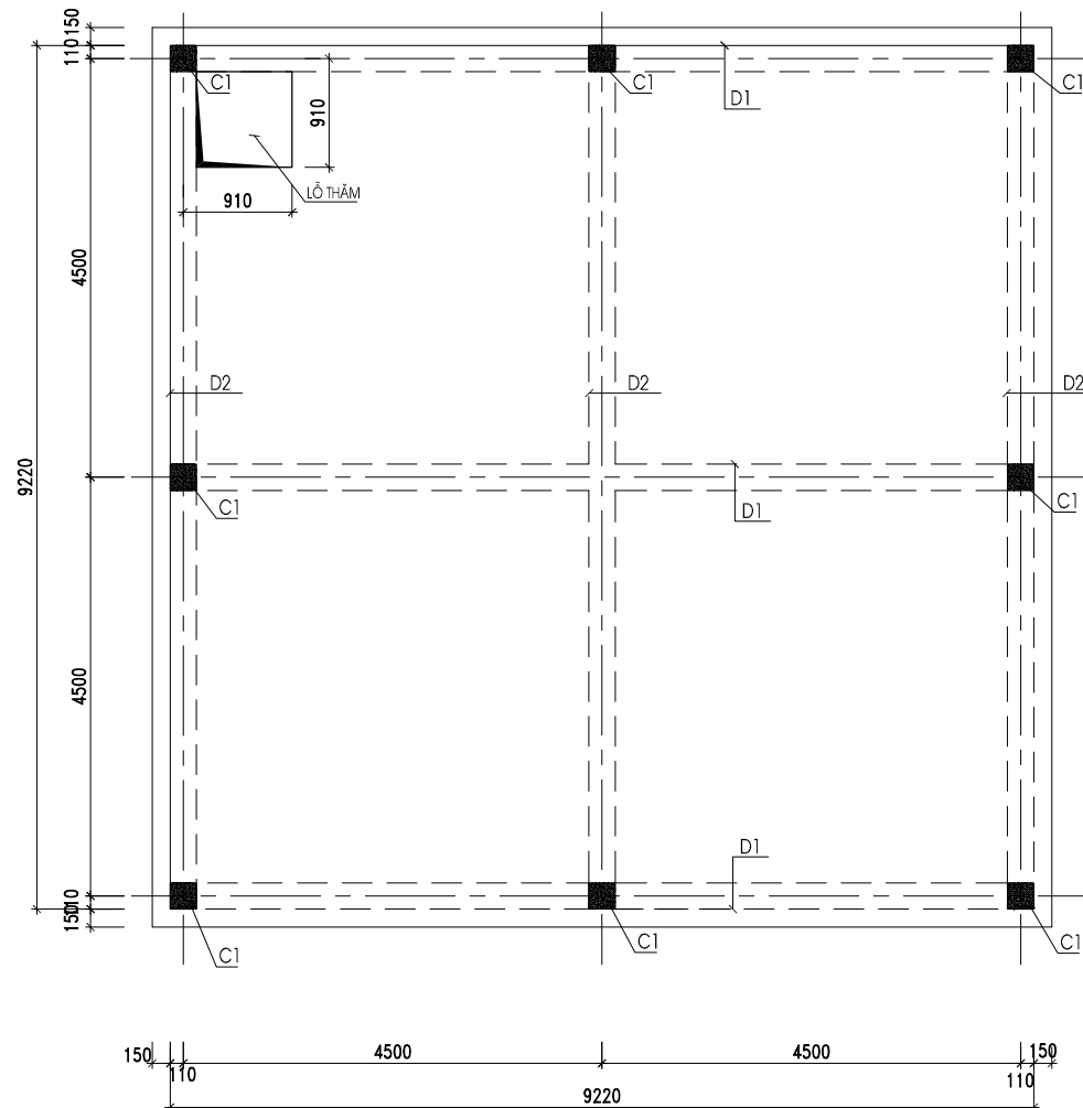
MẶT BẰNG KẾT CẤU NẮP BỂ NƯỚC NGẦM
