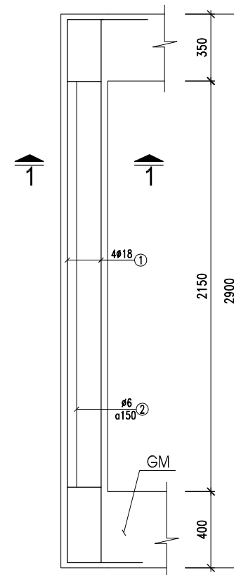
CỘT C1 - SL:08
