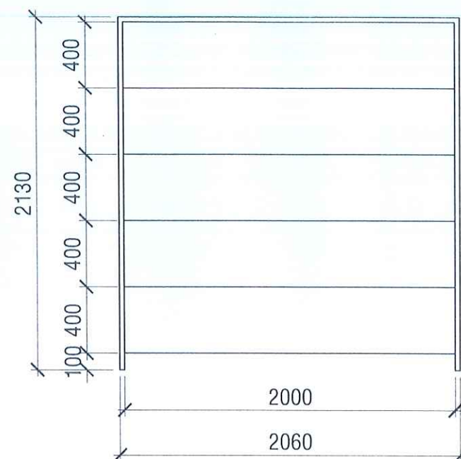
MẶT ĐỨNG
