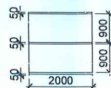
MẶT ĐỨNG
