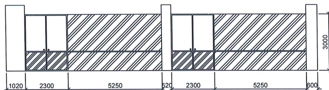
MẶT ĐỨNG CỬA VÀ VÁCH NHÔM KÍNH KHO V.TƯ TRANG TBYT
