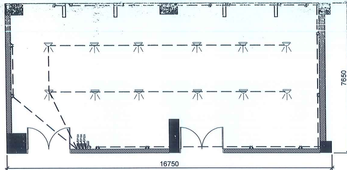
MẶT BẰNG BỐ TRÍ HỆ THỐNG ĐIỆN NHÀ KHO - PHÒNG VẬT TƯ TRANG THIẾT BỊ Y TẾ
