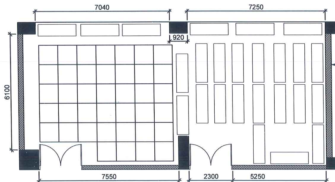
MẶT BẰNG BỐ TRÍ HỆ THỐNG ĐIỆN NHÀ KHO - PHÒNG VẬT TƯ TRANG THIẾT BỊ Y TẾ
