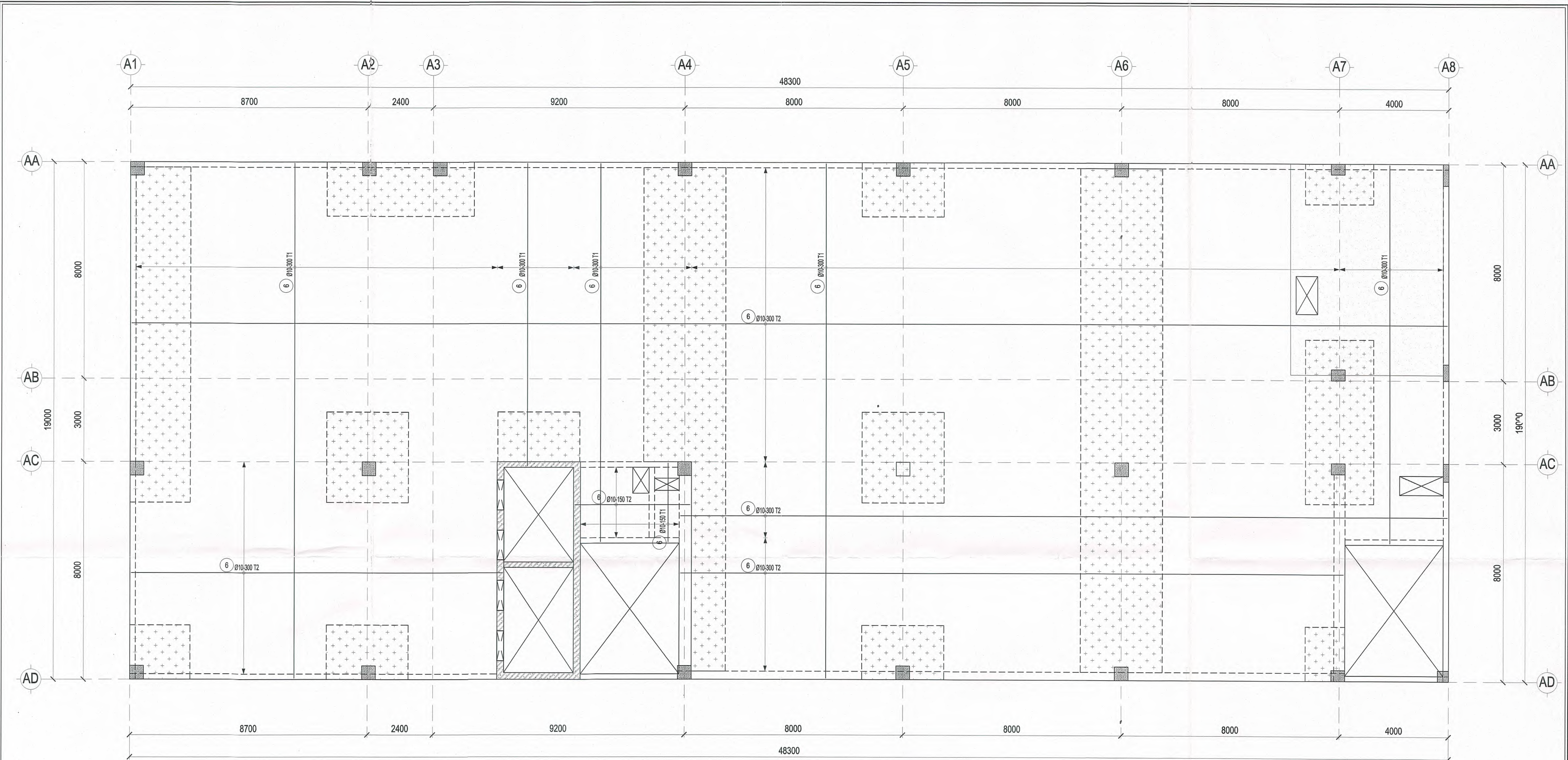
MẶT BẰNG THÉP SÀN LỚP TRÊN TẦNG 7 TL: 1/ 100
