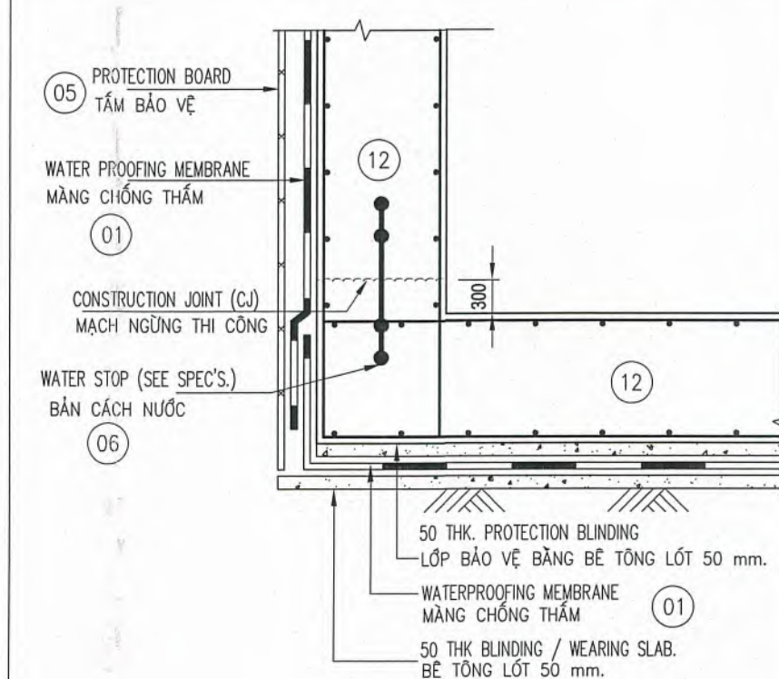
8. CHI TIẾT MỐI NỐI HỒ THU/ SÀN
