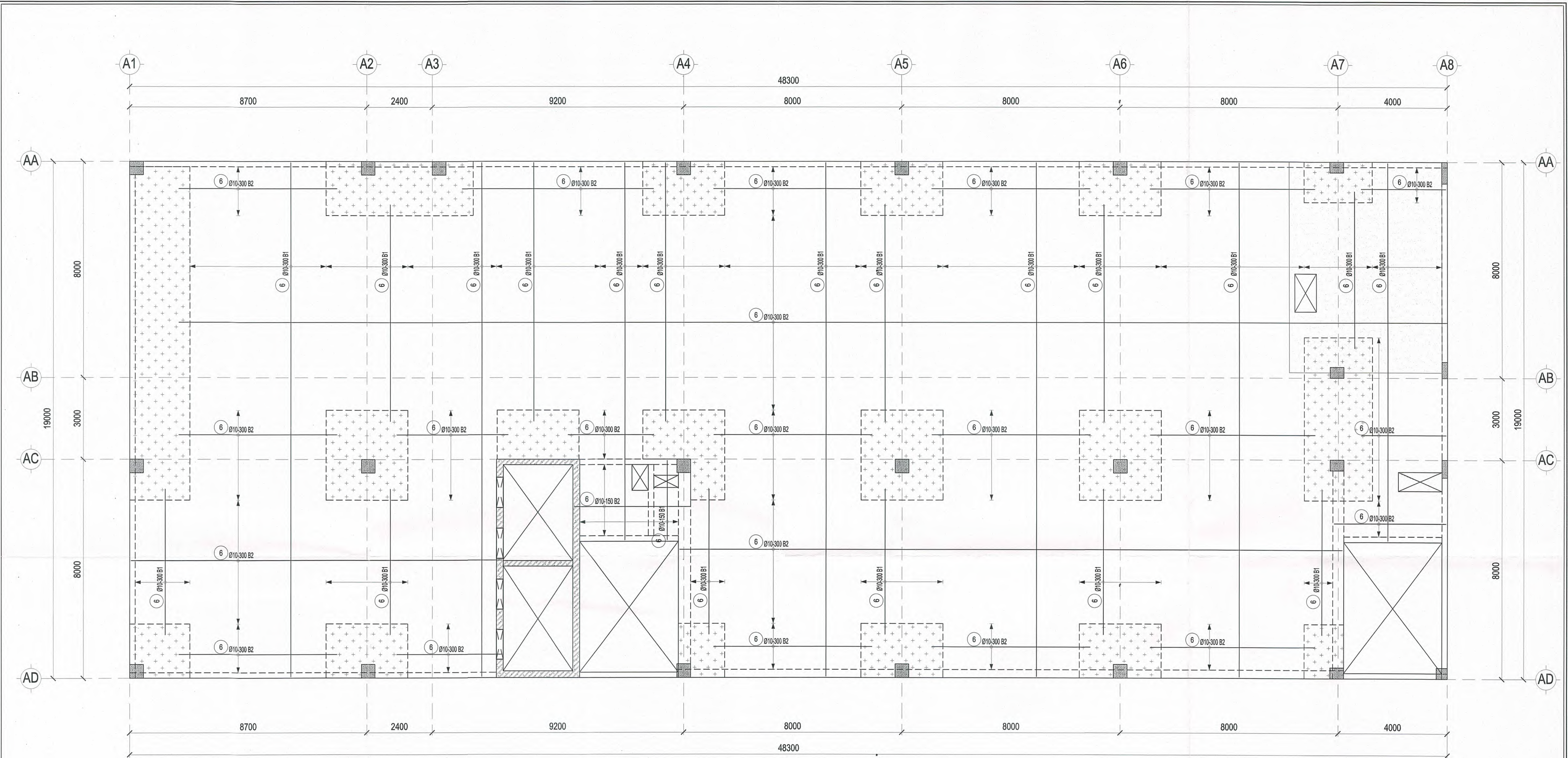
MẶT BẰNG THÉP SÀN LỚP DƯỚI TẦNG 4-6 TL: 1/ 100
