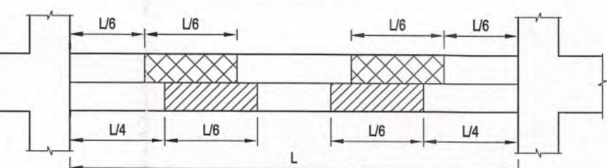
VỊ TRÍ ĐƯỢC NỐI THÉP TRONG SÀN HẦM : BASEMENT FOR SLAB
