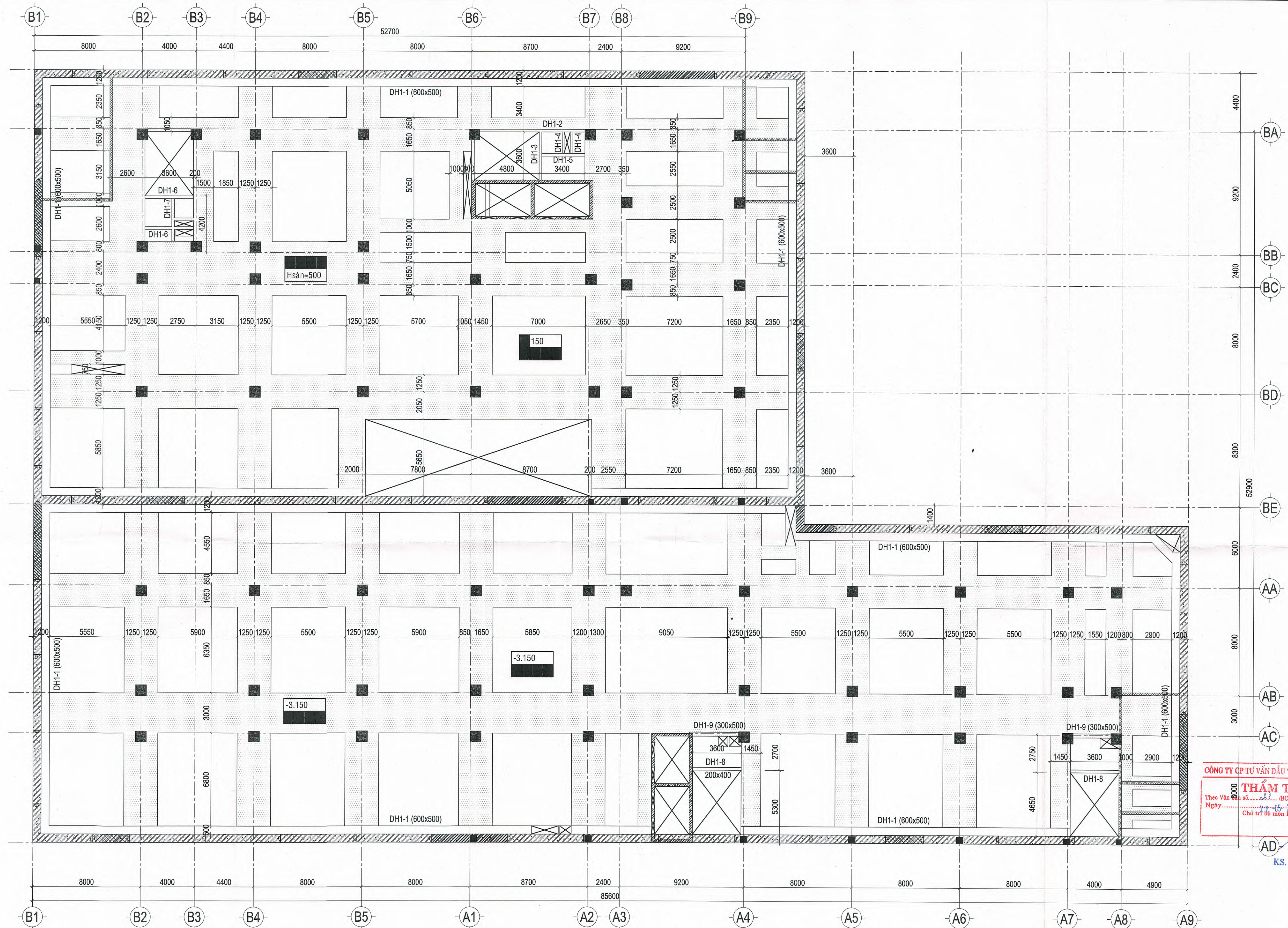
MẶT BẰNG DẦM SÀN HẦM 1 TL: 1/200
