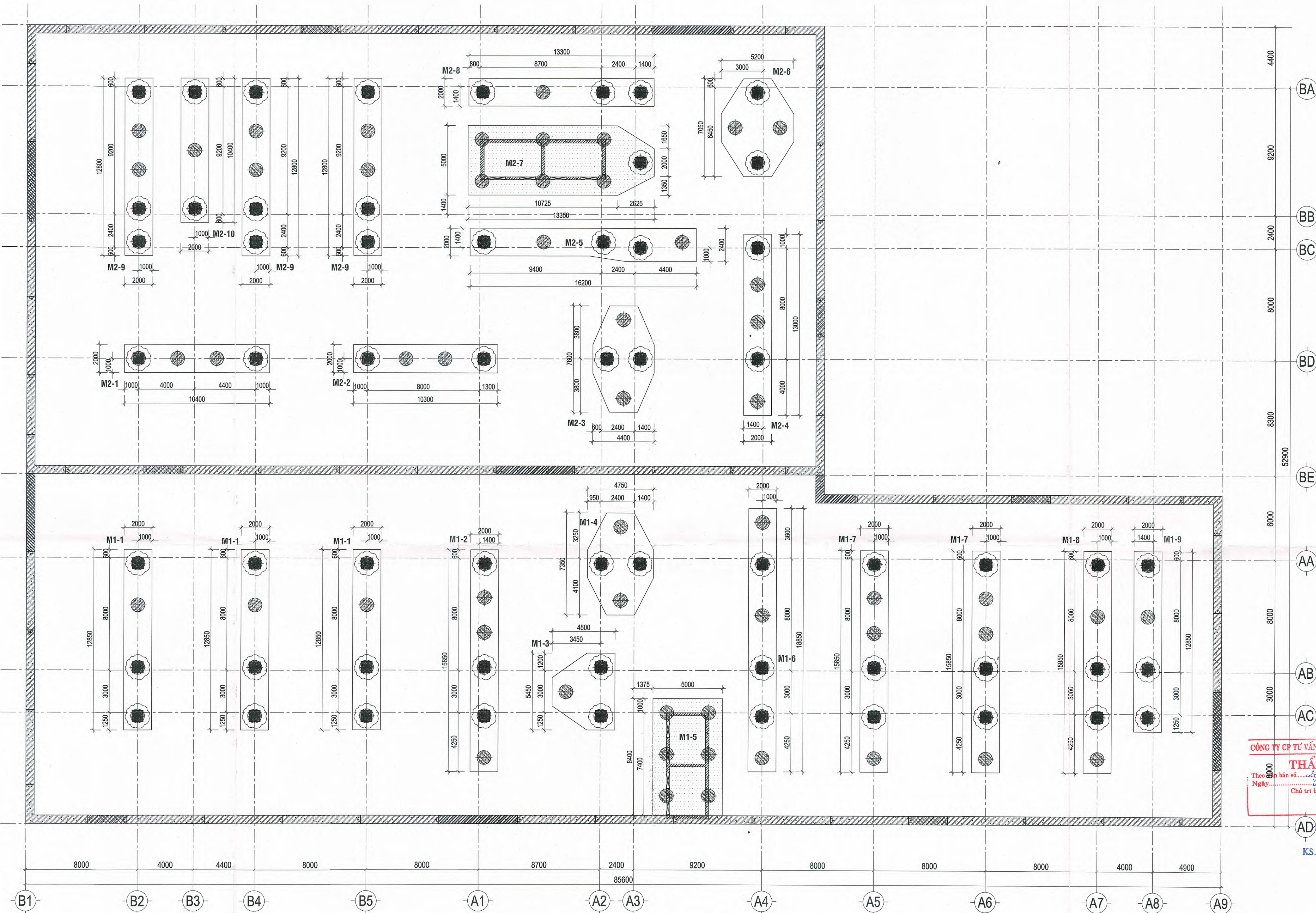
MẶT BẰNG ĐÌNH MÓNG
