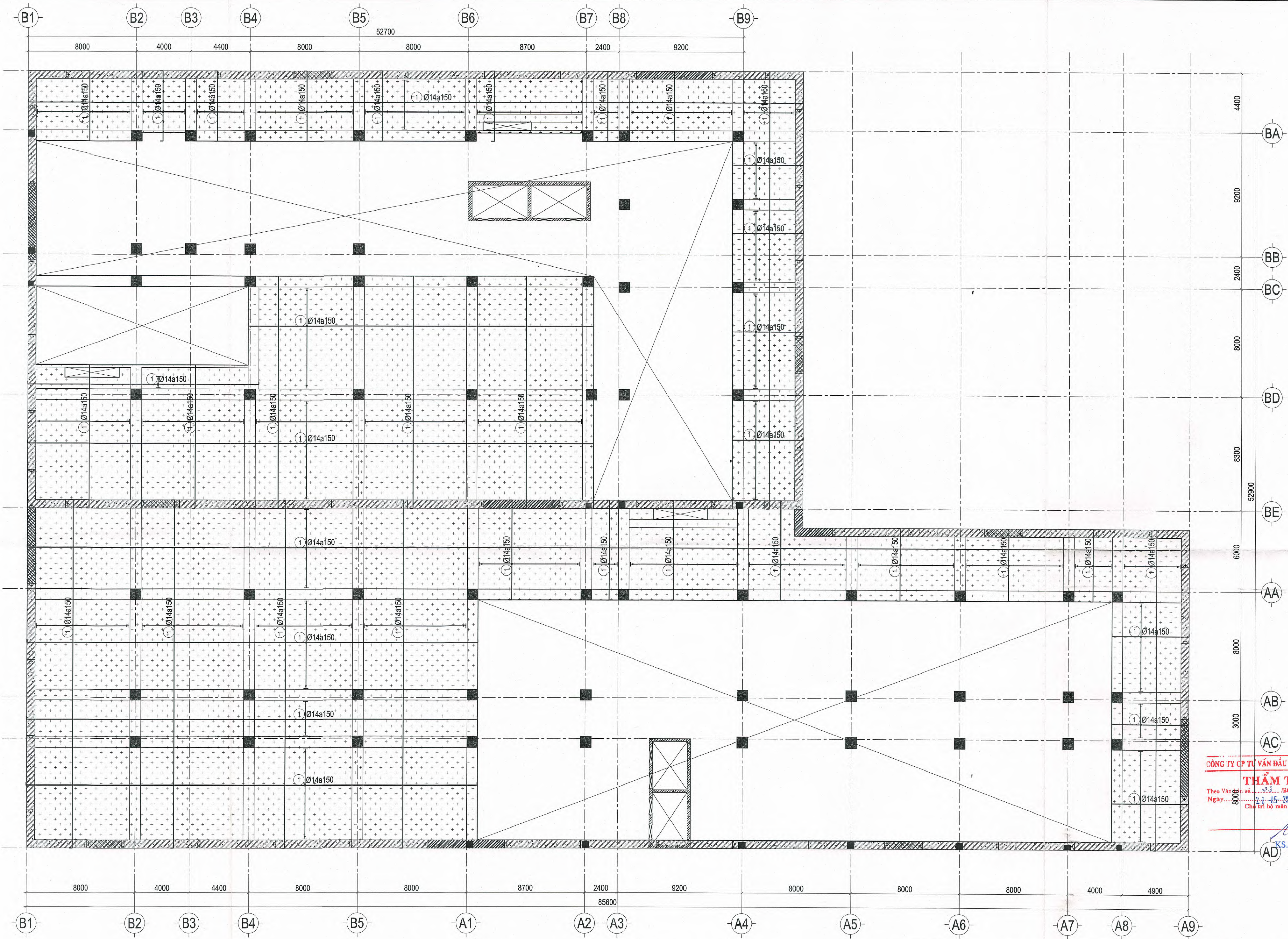
MẶT BẰNG THÉP SÀN LỚP DƯỚI TẦNG 1 COTE -0.050
