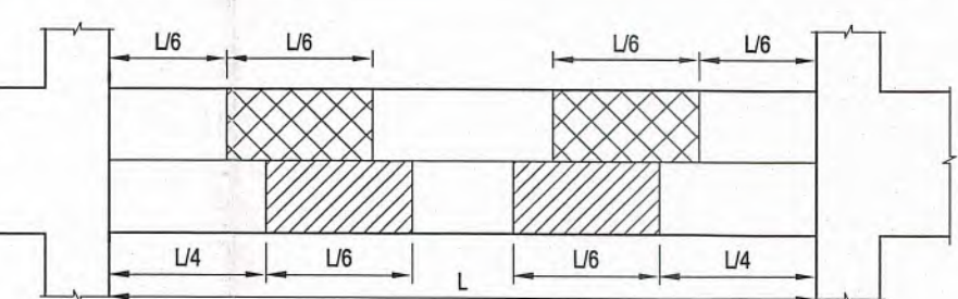
VỊ TRÍ ĐƯỢC NỐI THÉP TRONG DẪM HẦM : BASEMENT FOR BEAM
