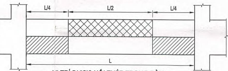
VỊ TRÍ ĐƯỢC NỐI THÉP TRONG DẪM : FOR BEAM
