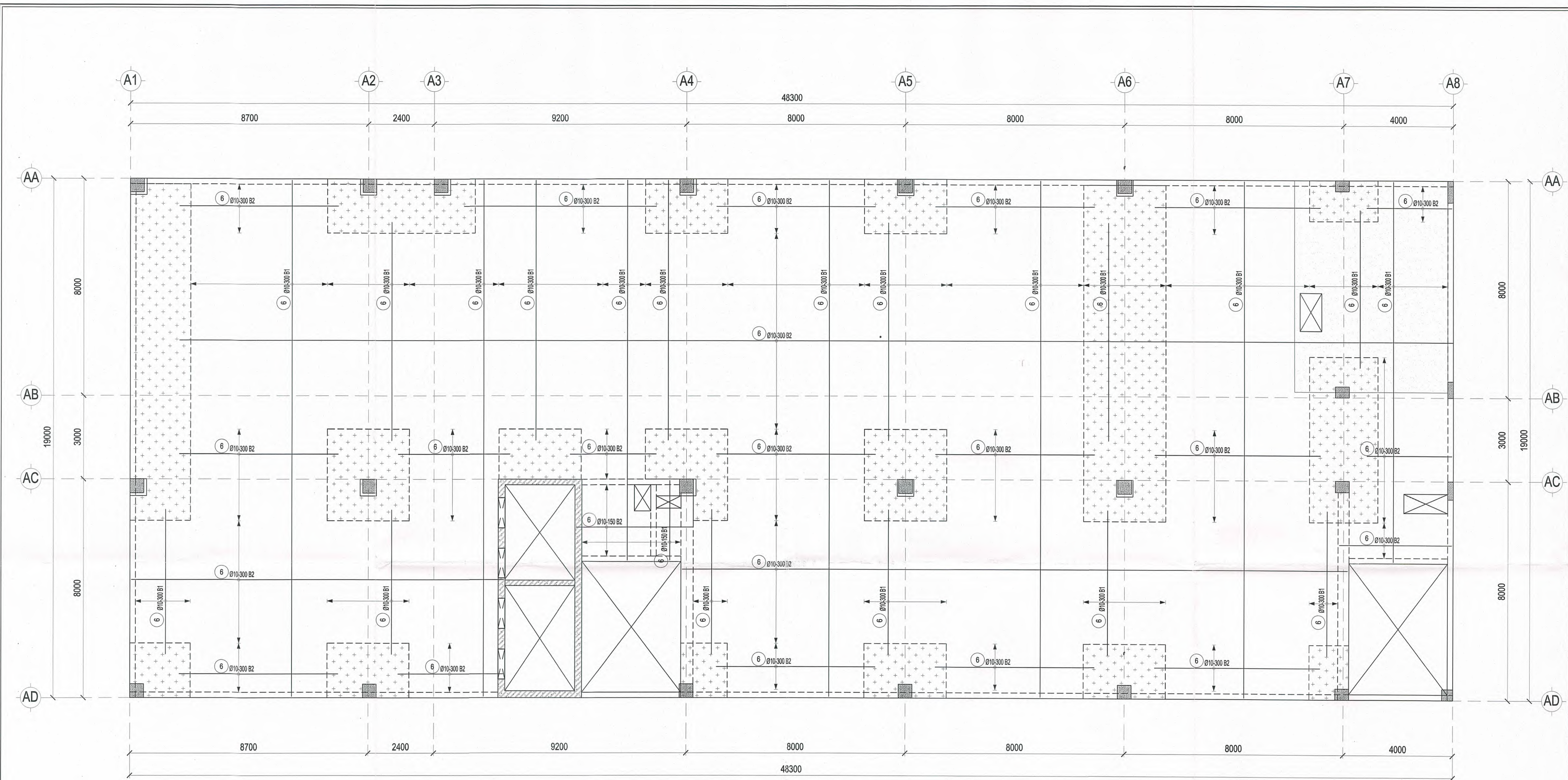
MẶT BẰNG THÉP SÀN LỚP DƯỚI TẦNG 3 TL: 1/ 100
