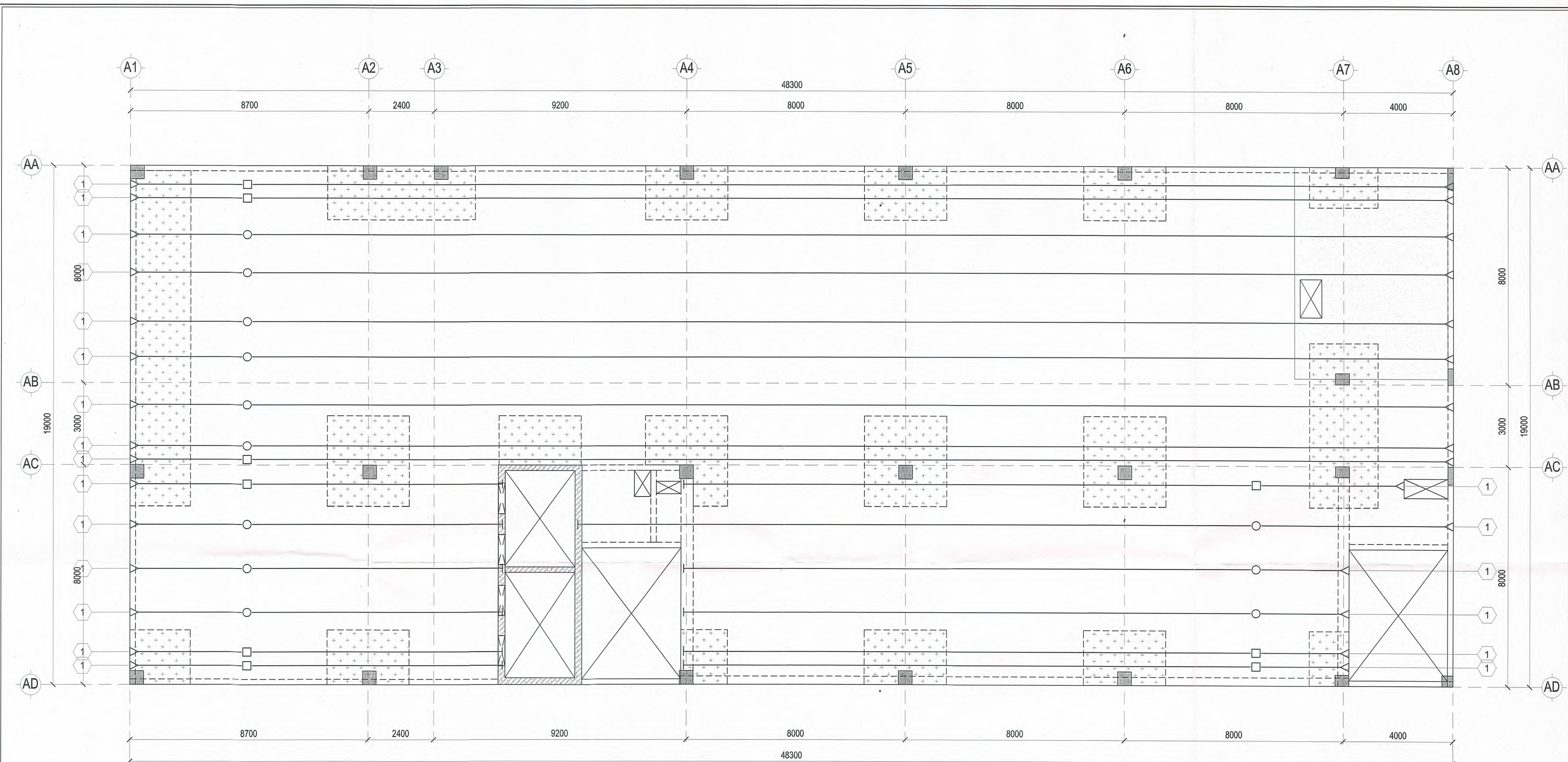
MẶT BẰNG CẤP SÀN PHƯƠNG X TẦNG 4-6 TL: 1/ 100
