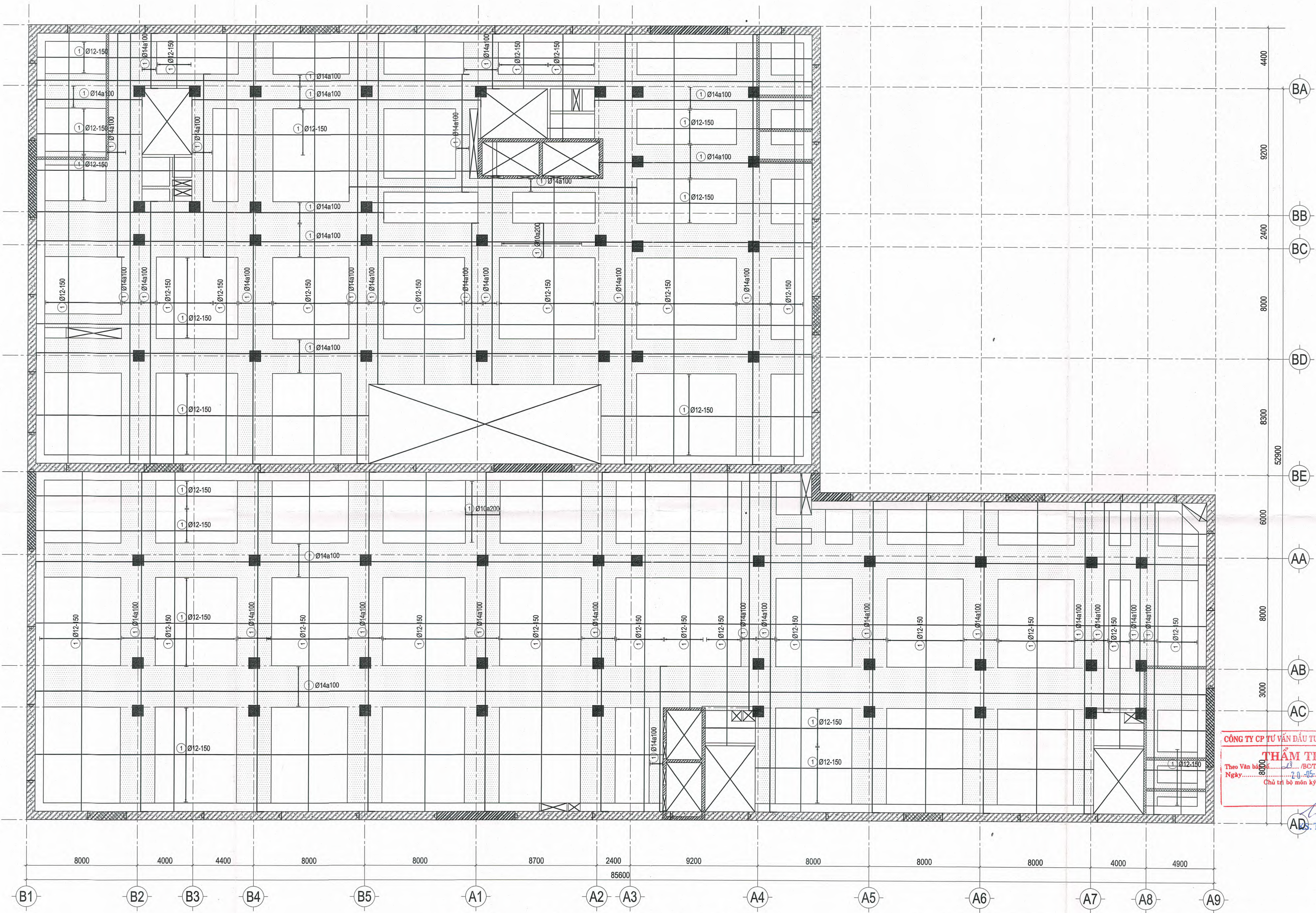
MẶT BẰNG THÉP LỚP TRÊN SÀN HẦM 1 TL: 1/200
