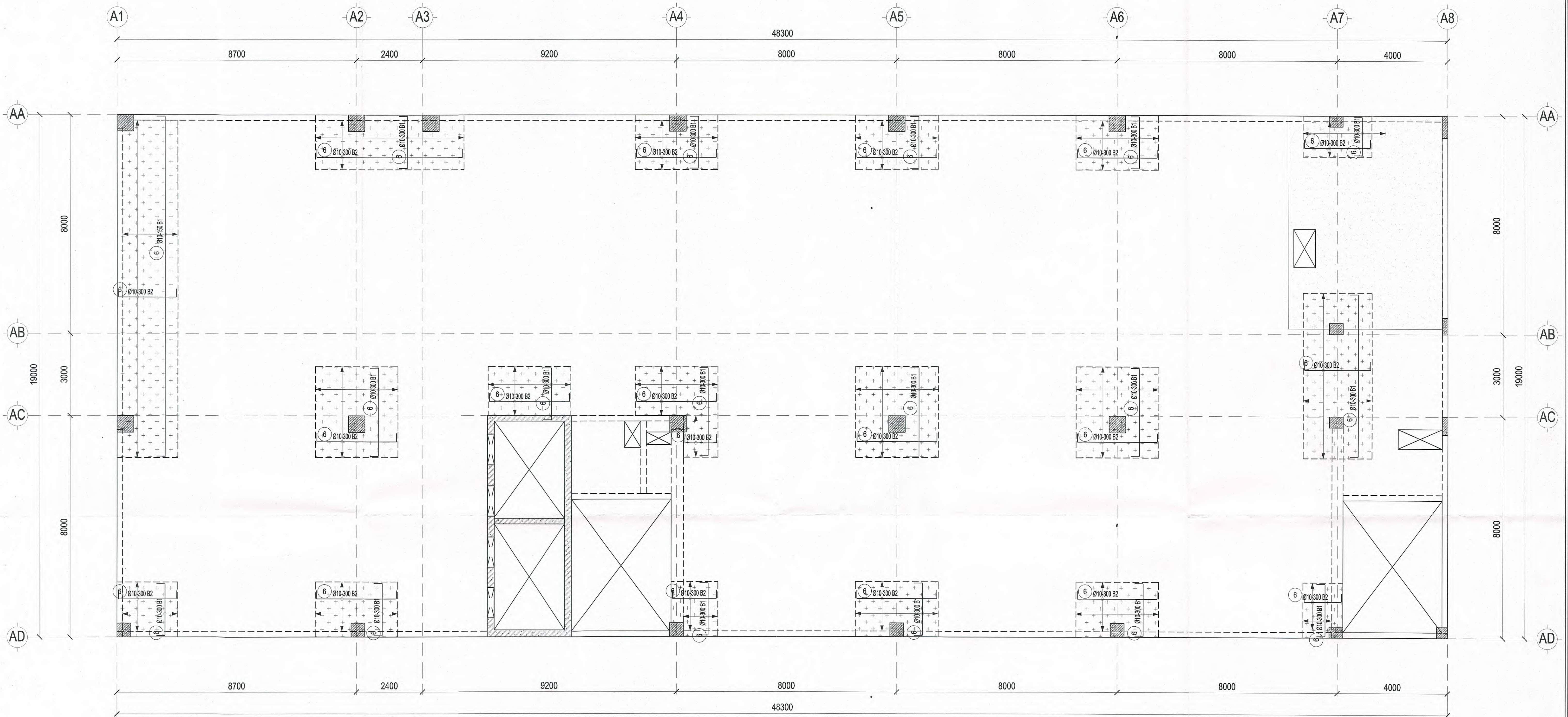
MẶT BẰNG THÉP SÀN TẦNG CƯỜNG LỚP DƯỚI TẦNG 2 TL: 1/ 100
