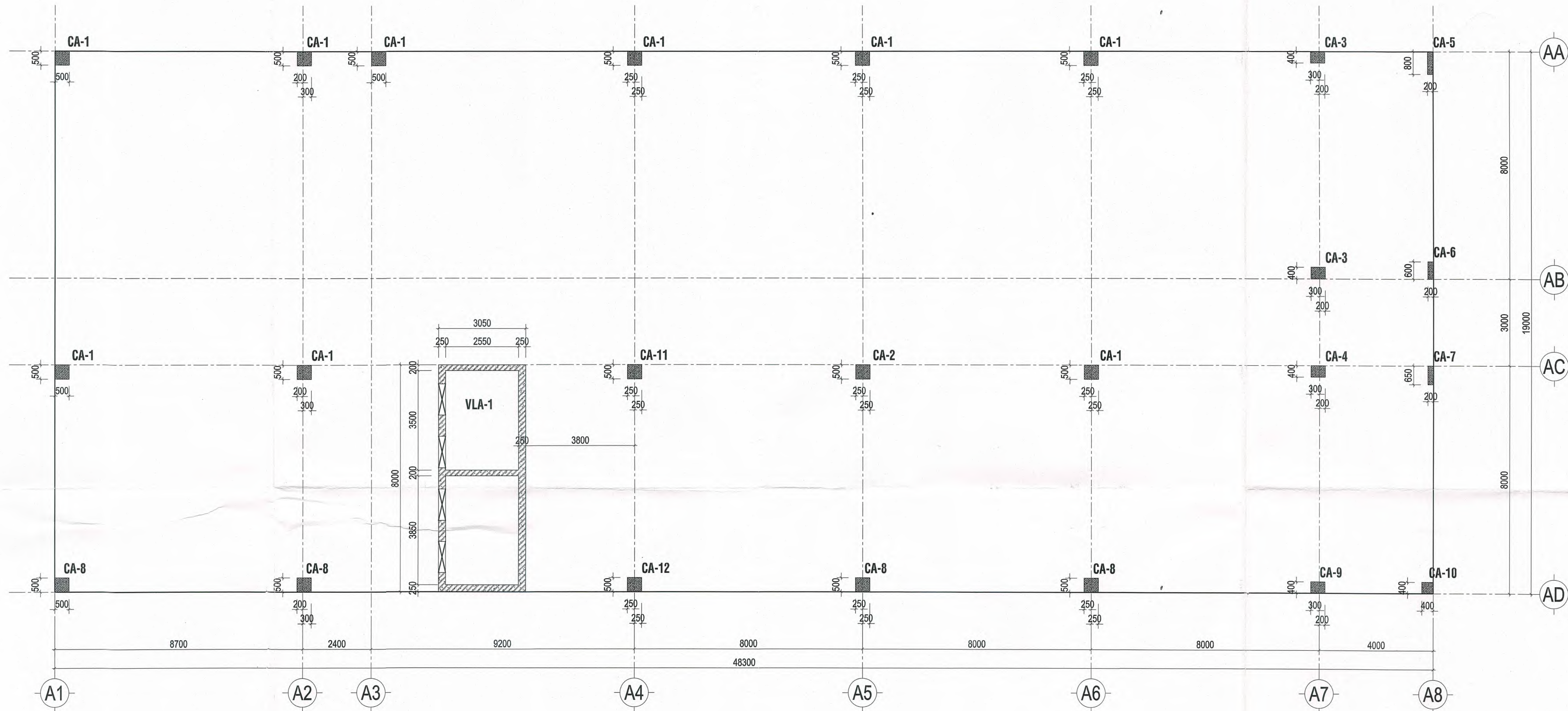
MẶT BẰNG ĐỊNH VỊ CỘT NHÀ A TẦNG 3 -> TẦNG 7
