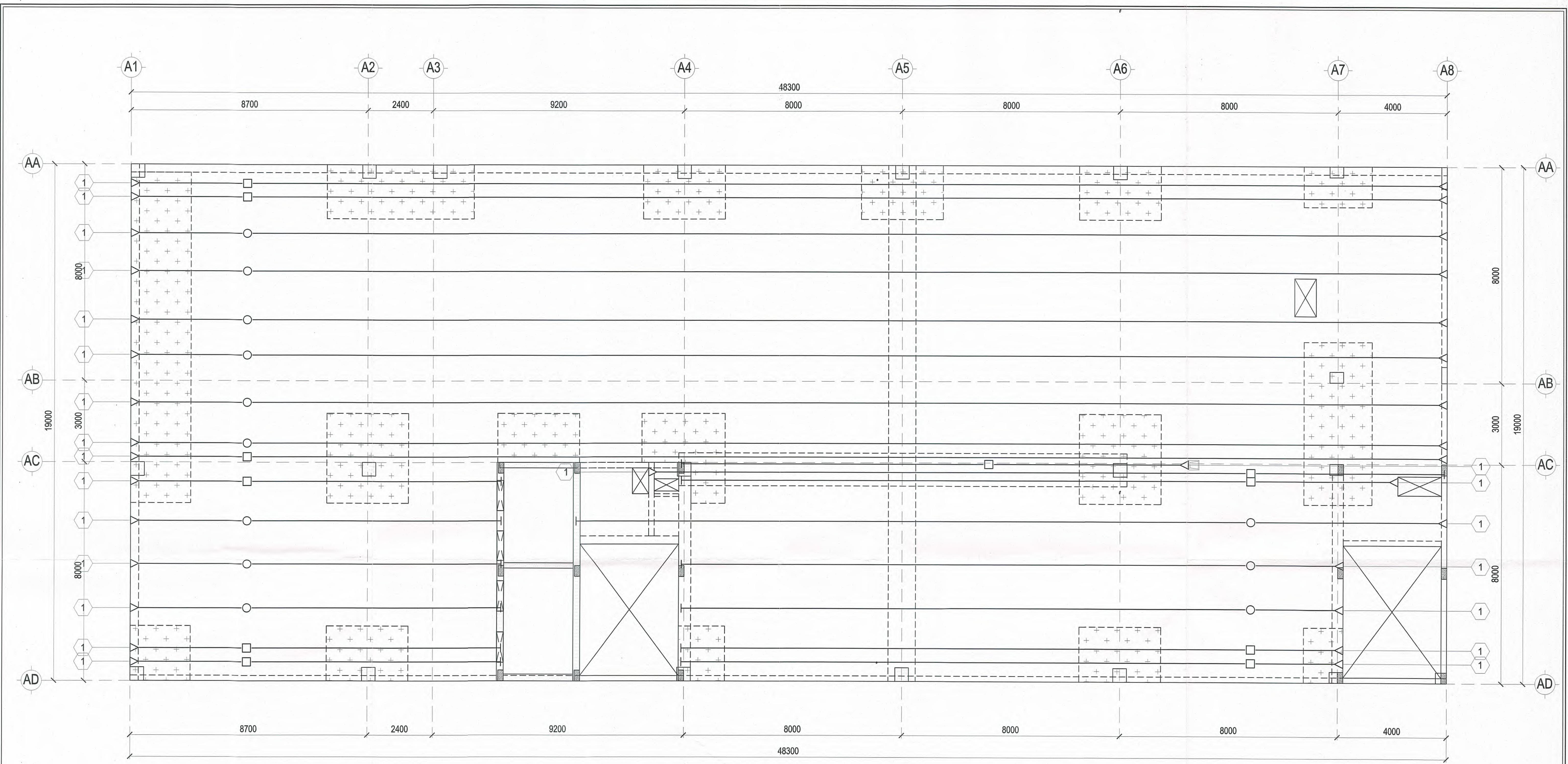
MẶT BẰNG CẤP SÀN PHƯƠNG X TẦNG TUM TL: 1/ 100
