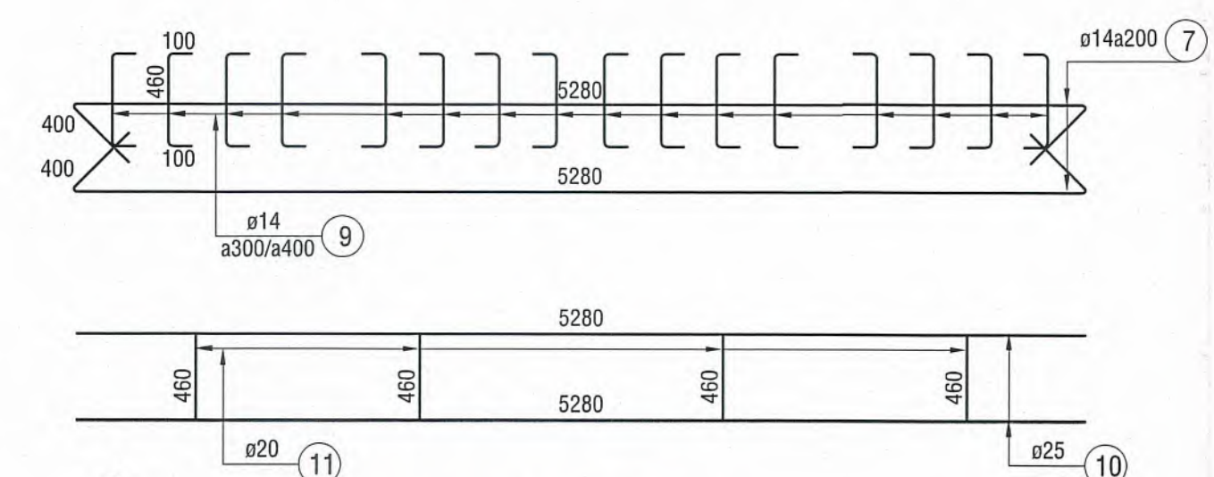
CHI TIẾT THẾP ĐAI
