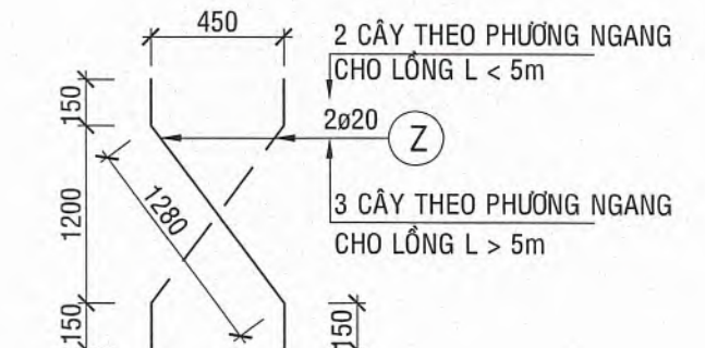
THÉP TĂNG CỨNG
