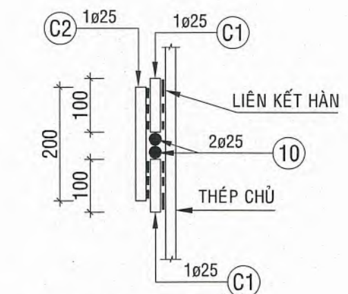
CHI TIẾT CON CHẶN (MỖI THANH U TREO LỒNG BỐ TRÍ 2 VỊ TRÍ CON CHẶN)
