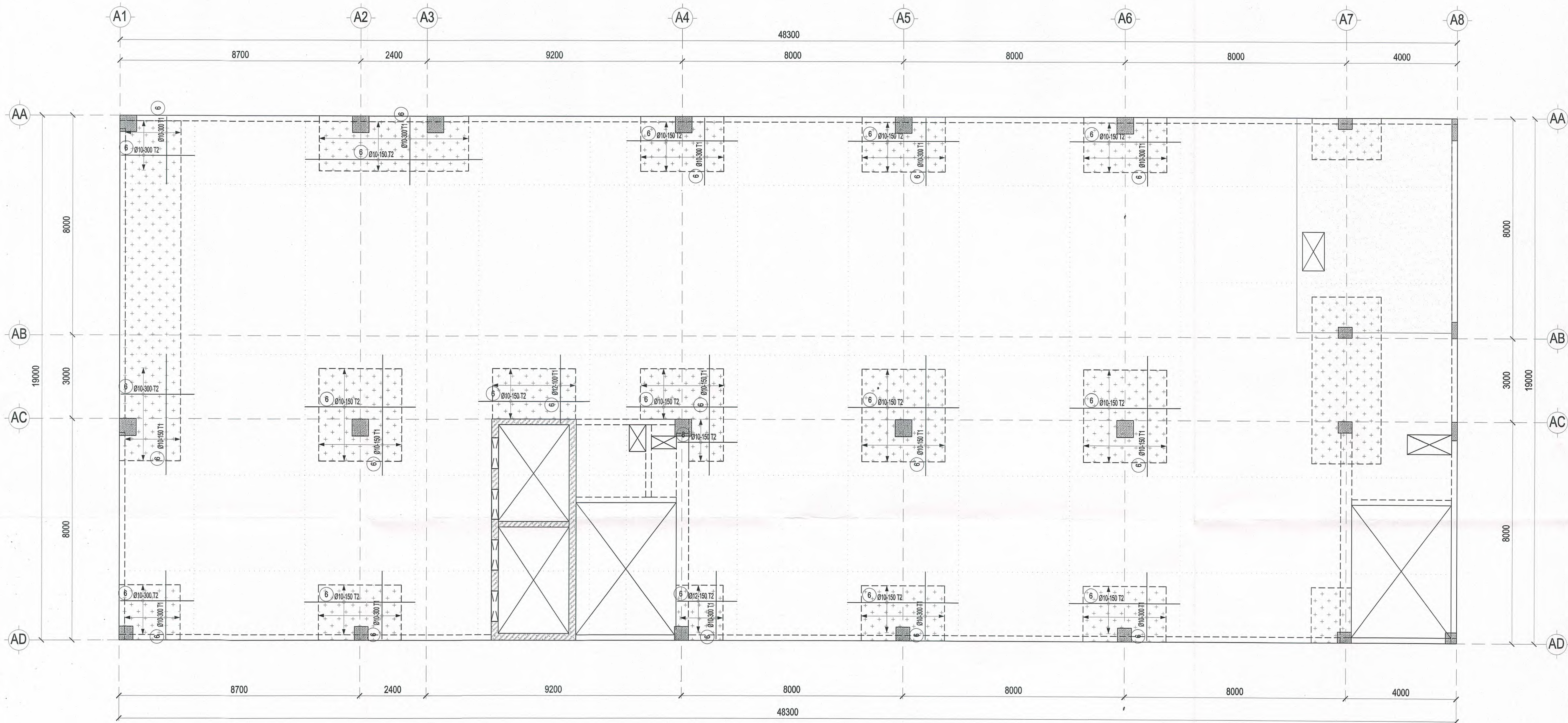
MẶT BẰNG THÉP SÀN TẦNG CƯỜNG LỚP TRÊN TẦNG 2 TL: 1/ 100
