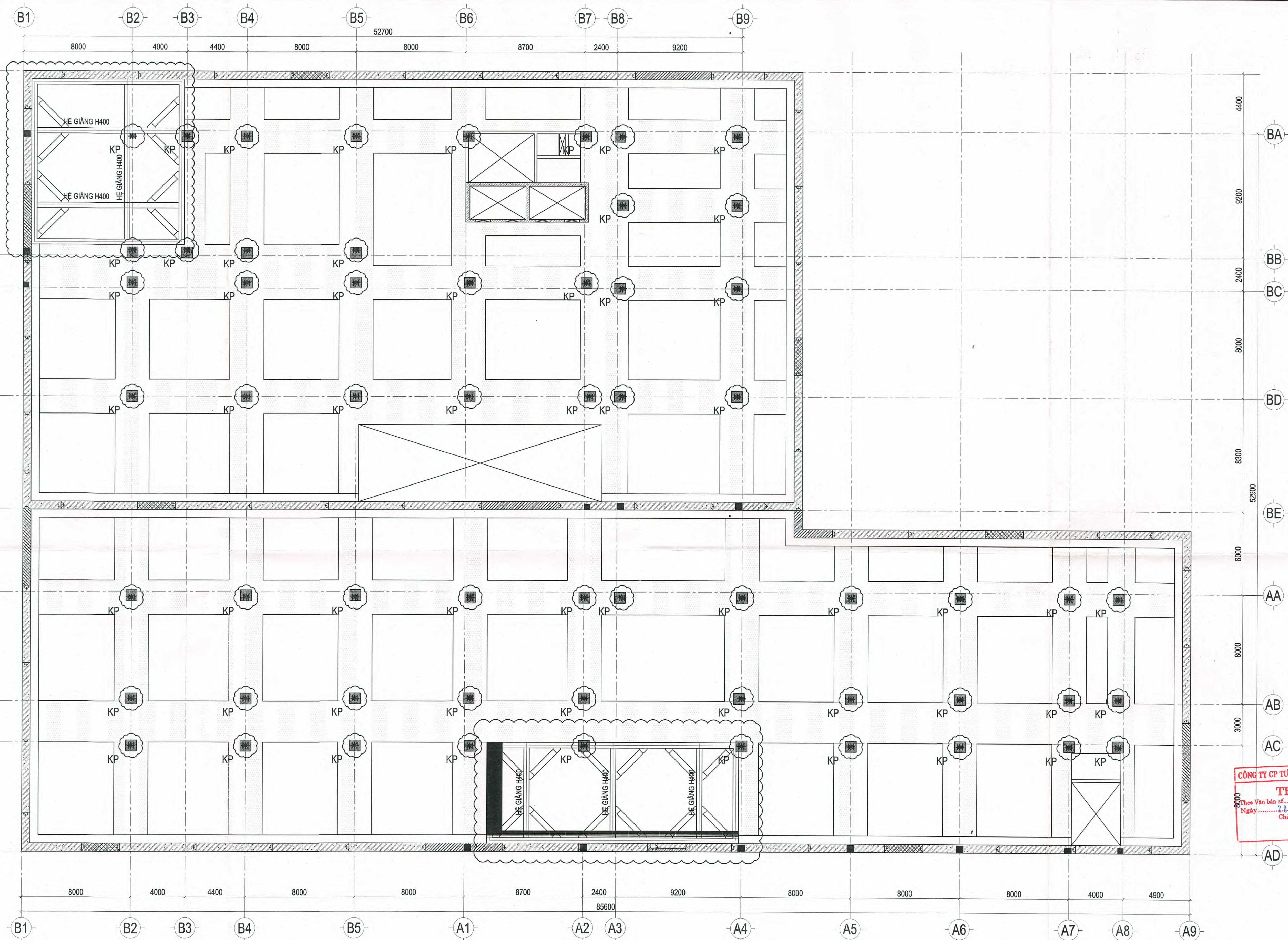
MẶT BẰNG SHORING HẦM 1 TL: 1/200
