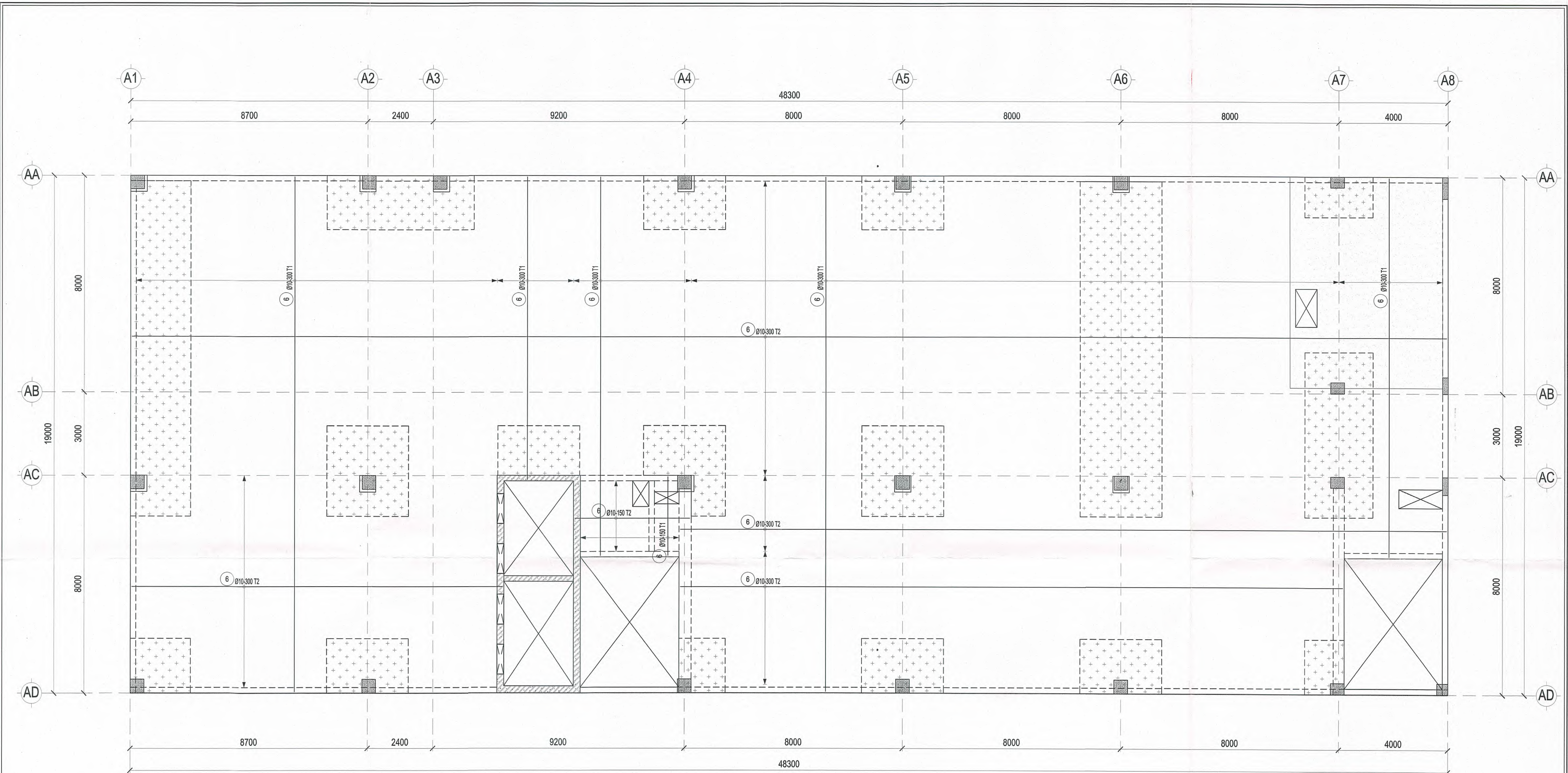
MẶT BẰNG THÉP SÀN LỚP TRÊN TẦNG 3 TL: 1/ 100
