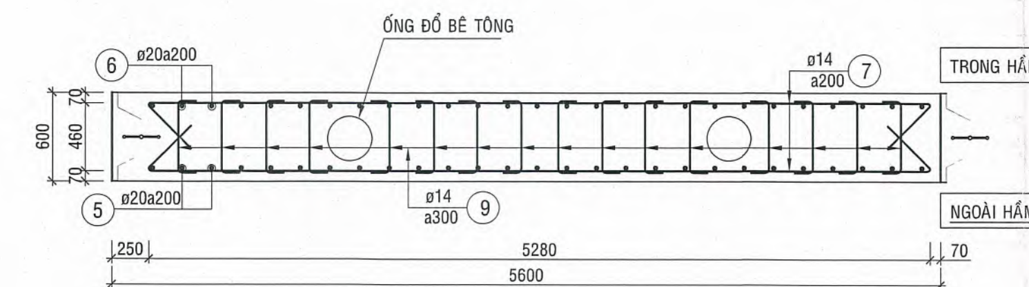
MẶT CẮT 3 - 3
