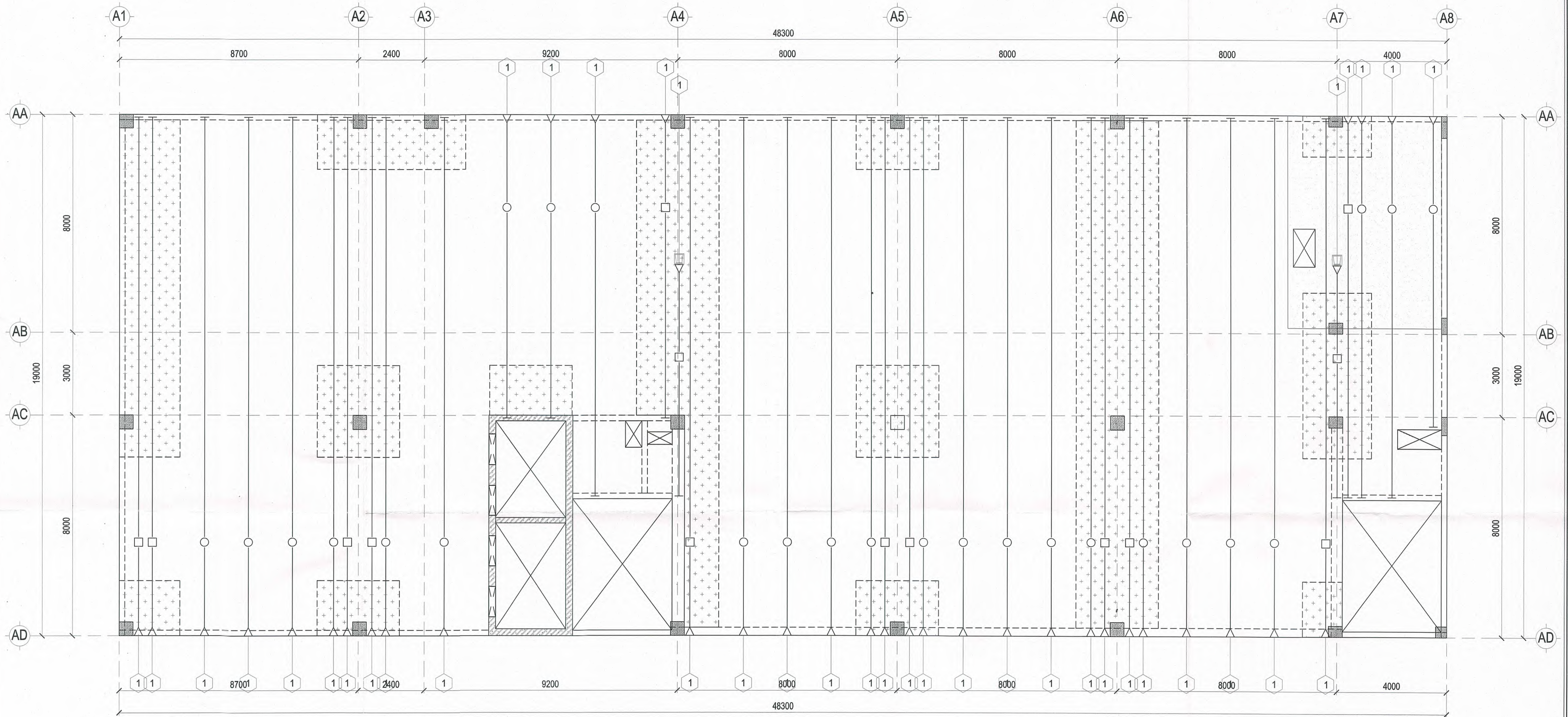
MẶT BẰNG CÁP SÀN PHƯƠNG Y TẦNG 7 TL: 1/ 100
