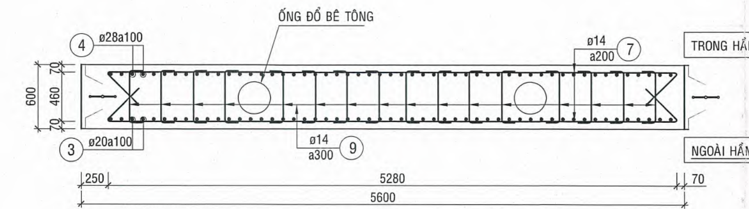
MẶT CẮT 2 - 2
