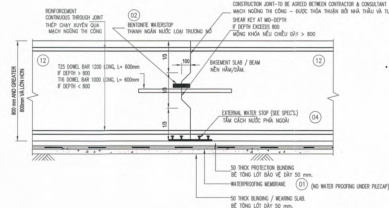
4. CHI TIẾT MẠCH NGỪNG THI CÔNG 4. CONSTRUCTION JOINT DETAIL
