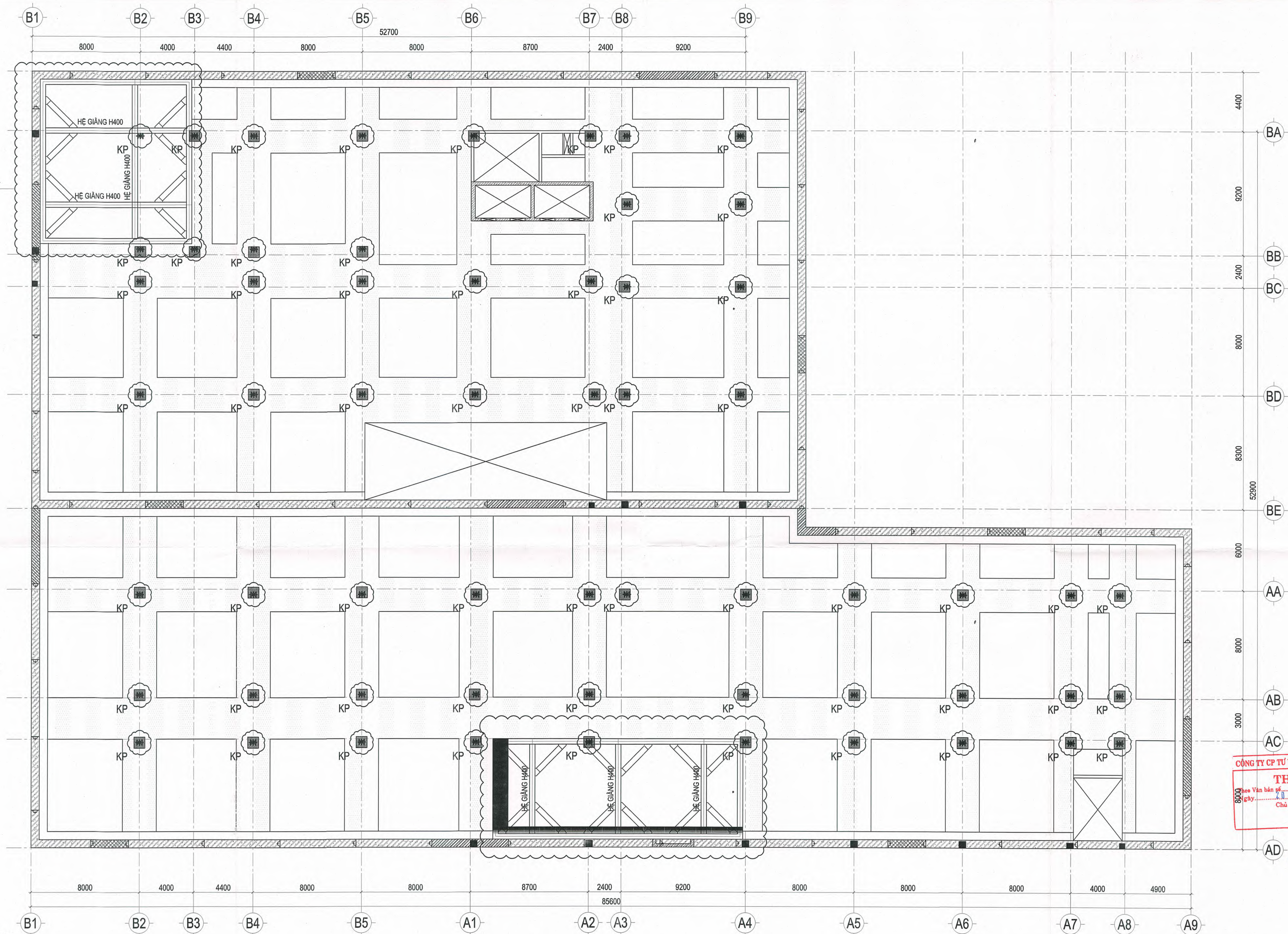
MẶT BẰNG SHORING HẦM 2 TL: 1/200
