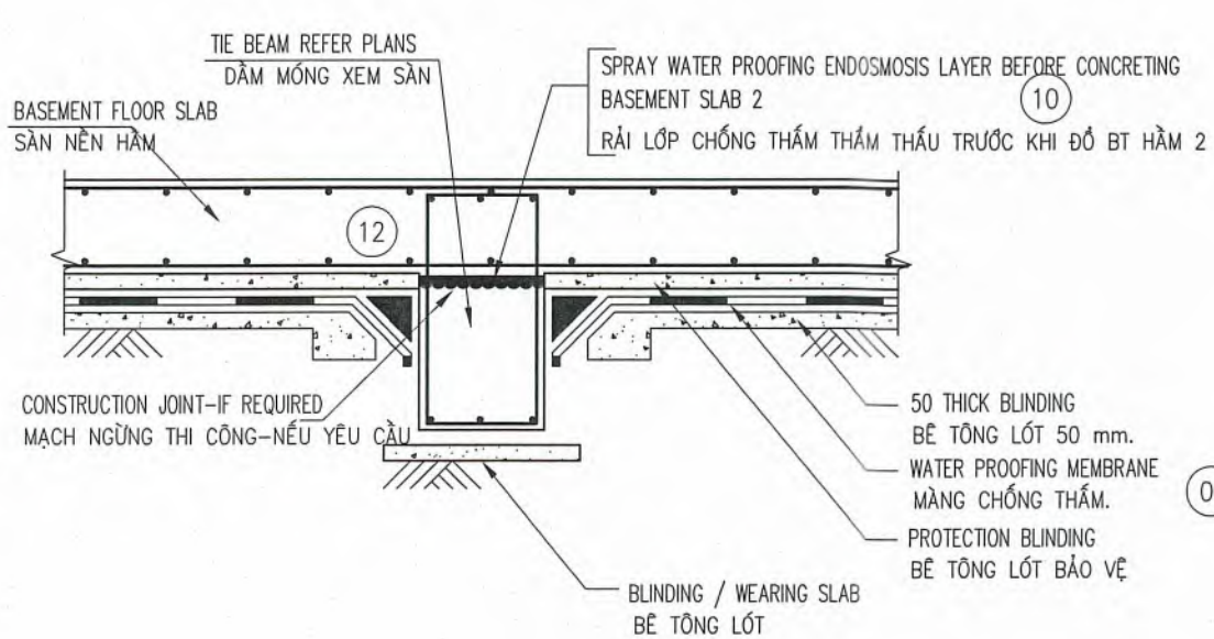
7. CHI TIẾT MỐI NỐI DẦM MÓNG/ SÀN 7. TIE BEAM/ SLAB JOINT DETAIL
