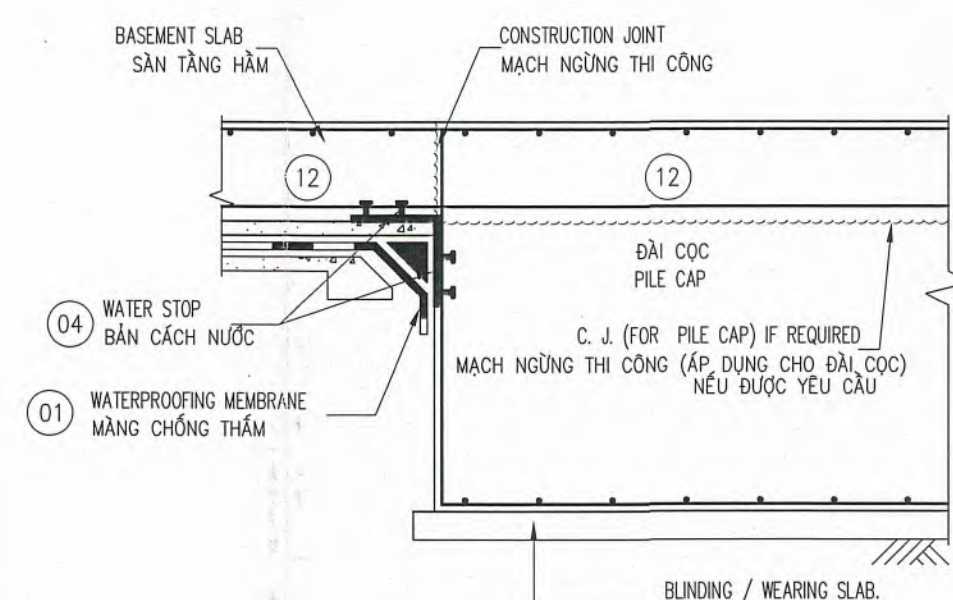
2. CHI TIẾT MÔI NỐI SÀN/ ĐÀI CỌC 2. PILECAP /SLAB JOINT DETAIL
