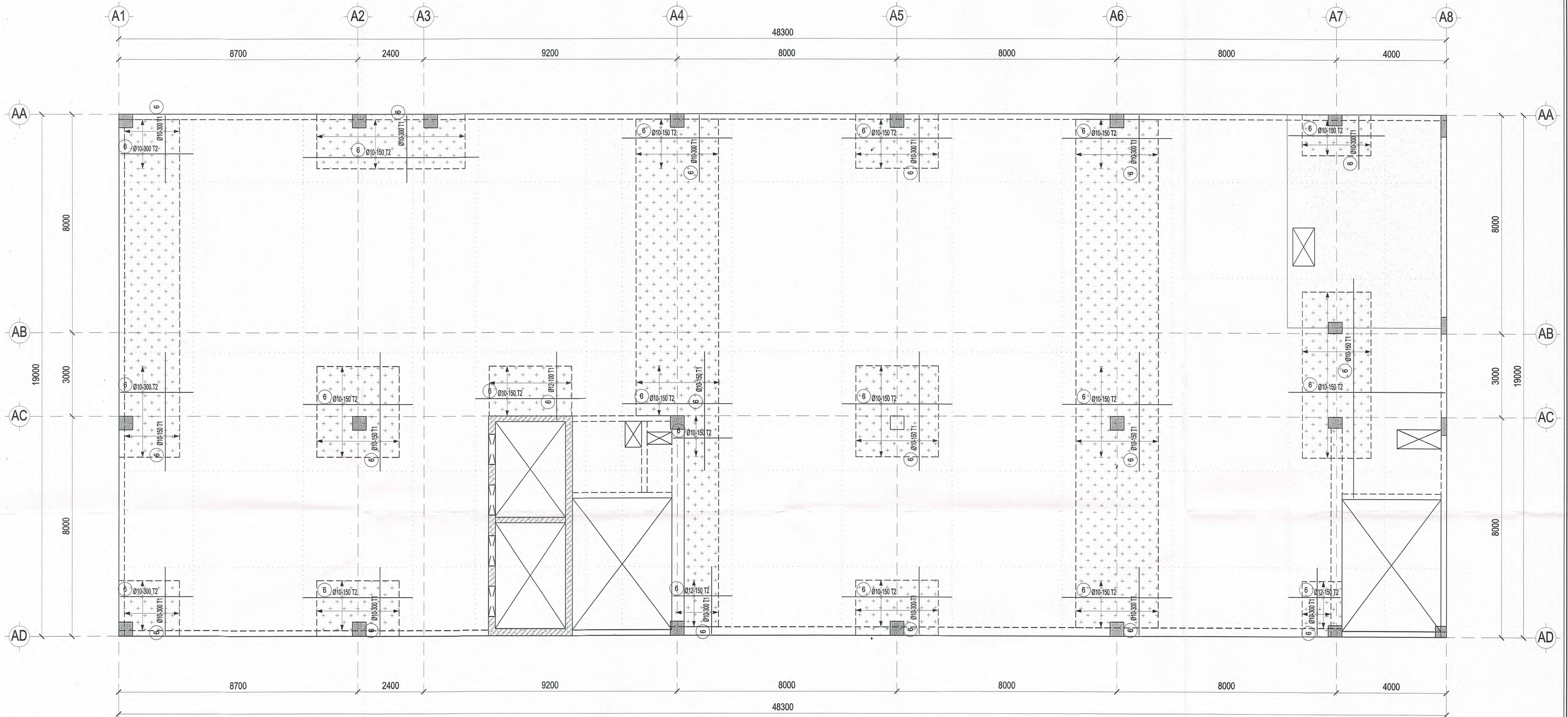
MẶT BẰNG THÉP SÀN TĂNG CƯỜNG LỚP TRÊN TẦNG 7 TL: 1/ 100
