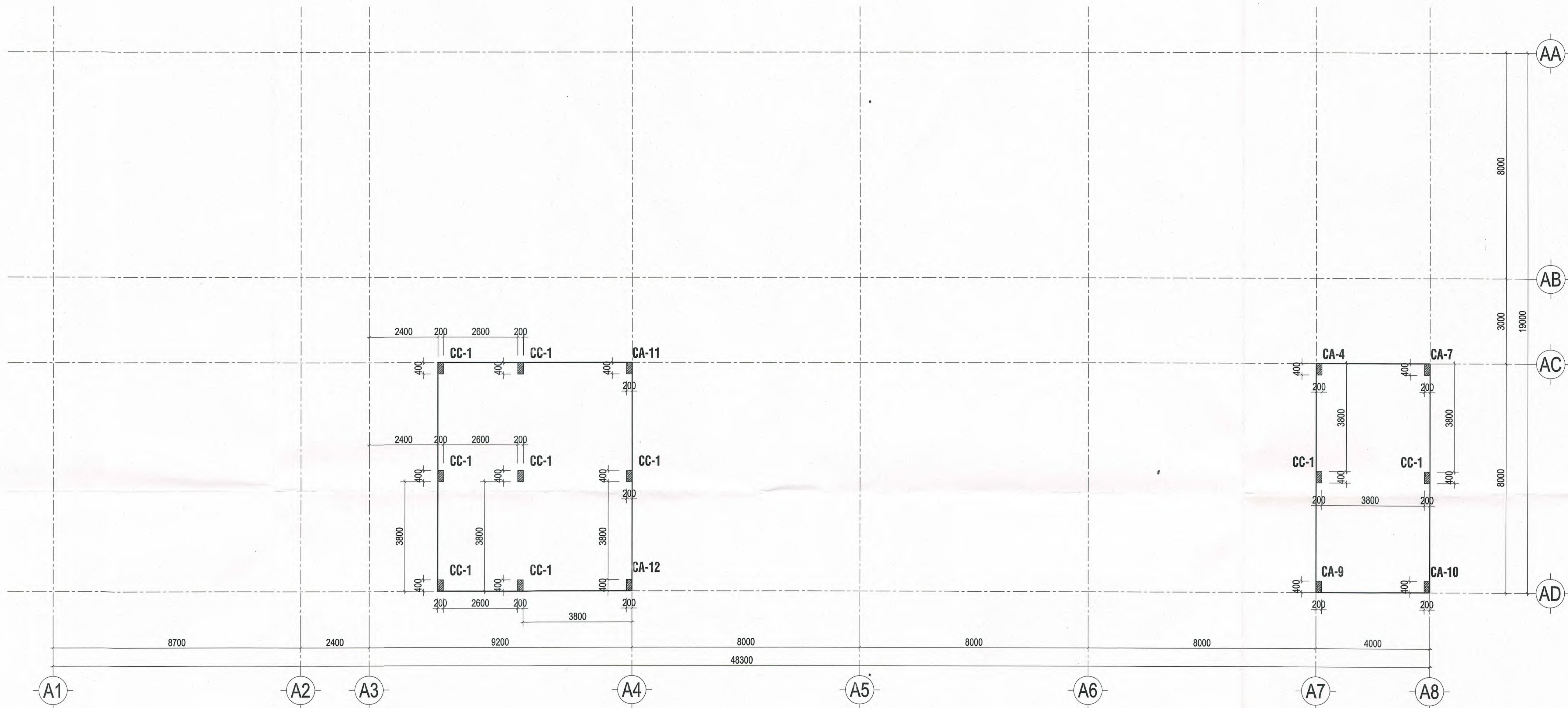
MẶT BẰNG ĐỊNH VỊ CỘT NHÀ A TUM -> MÁI
