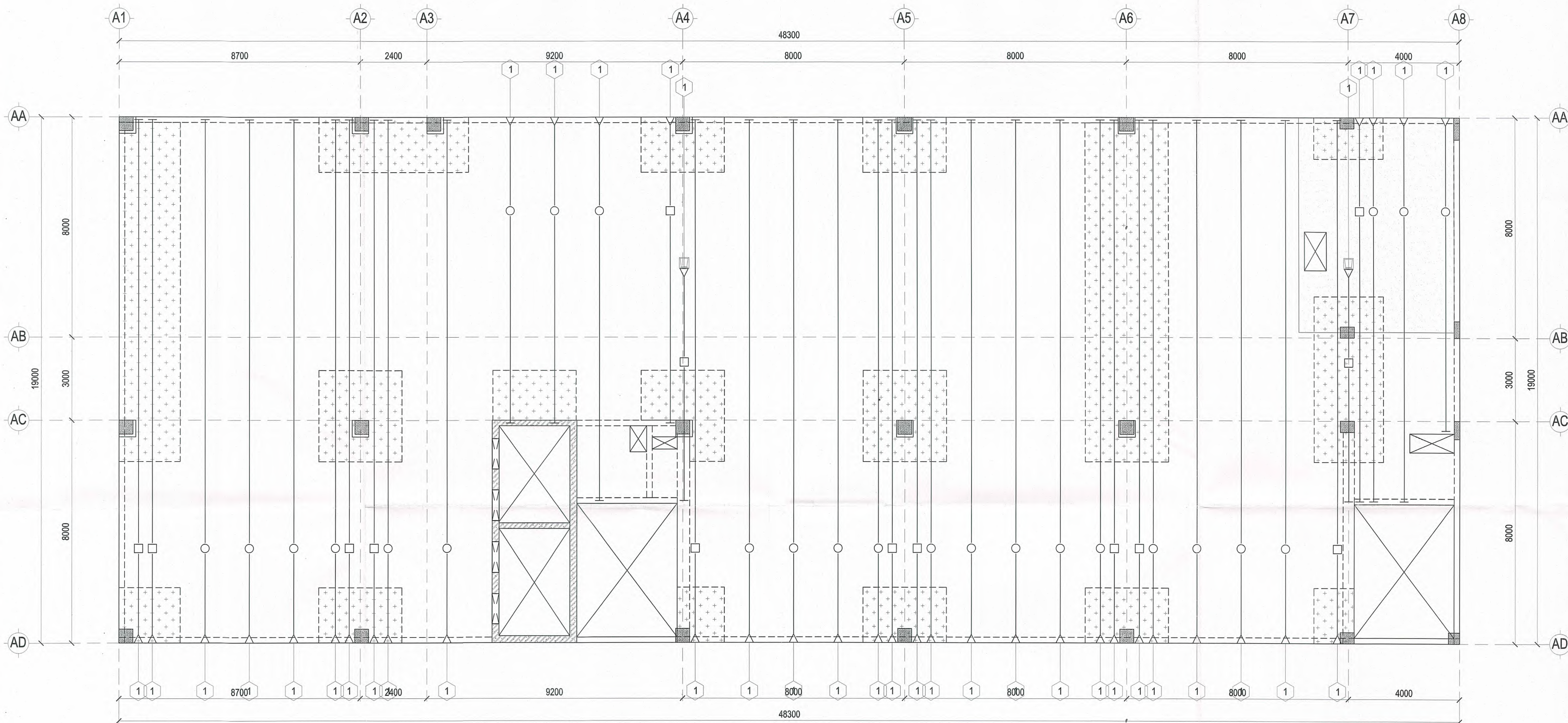
MẶT BẰNG CẤP SÀN PHƯƠNG Y TẦNG 3 TL: 1/ 100
