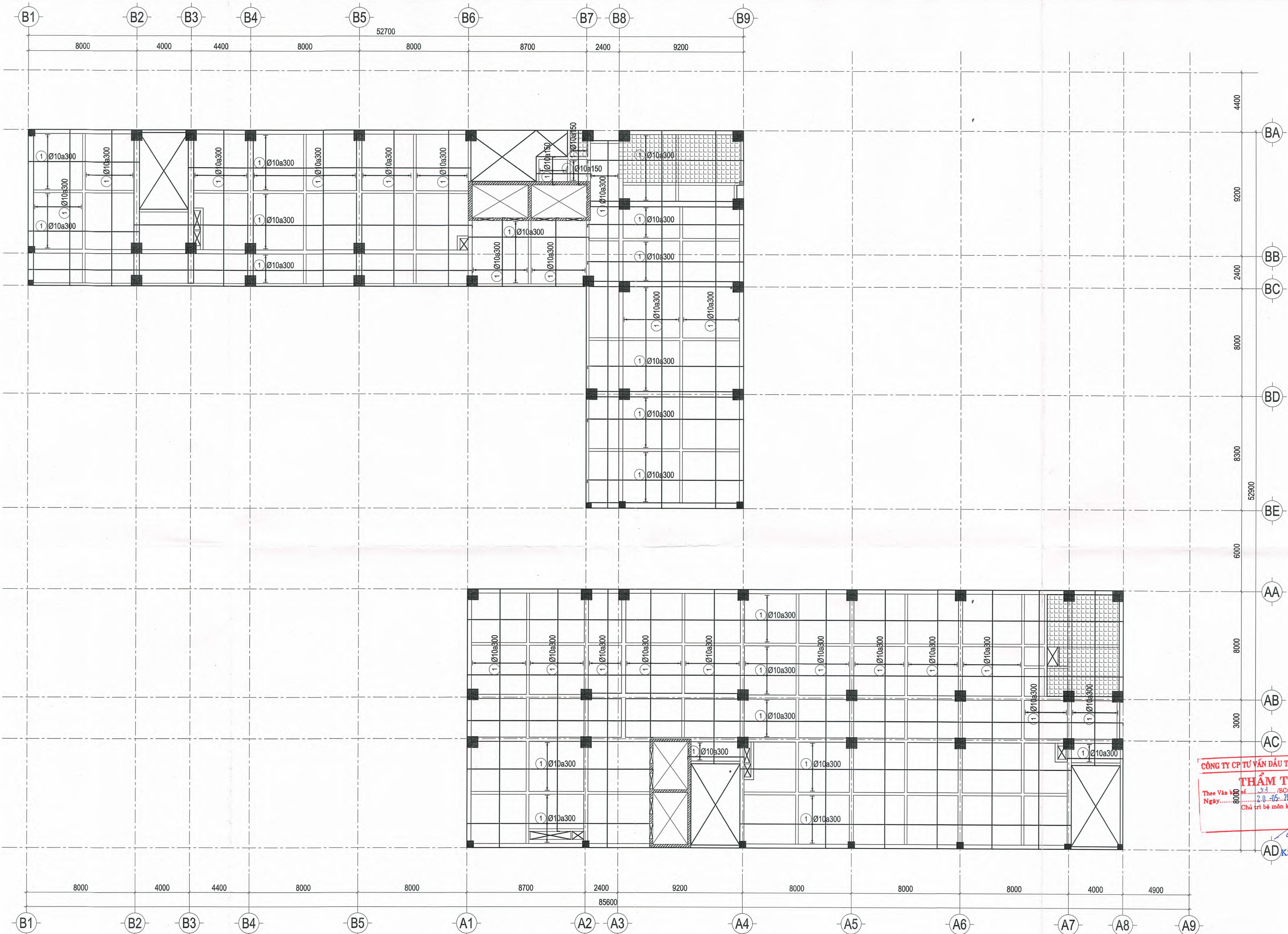
MẶT BẰNG THÉP PHÂN BỐ ĐỀU LỚP TRÊN SÀN TẦNG 1 COTE +1.150 TL: 1/200
