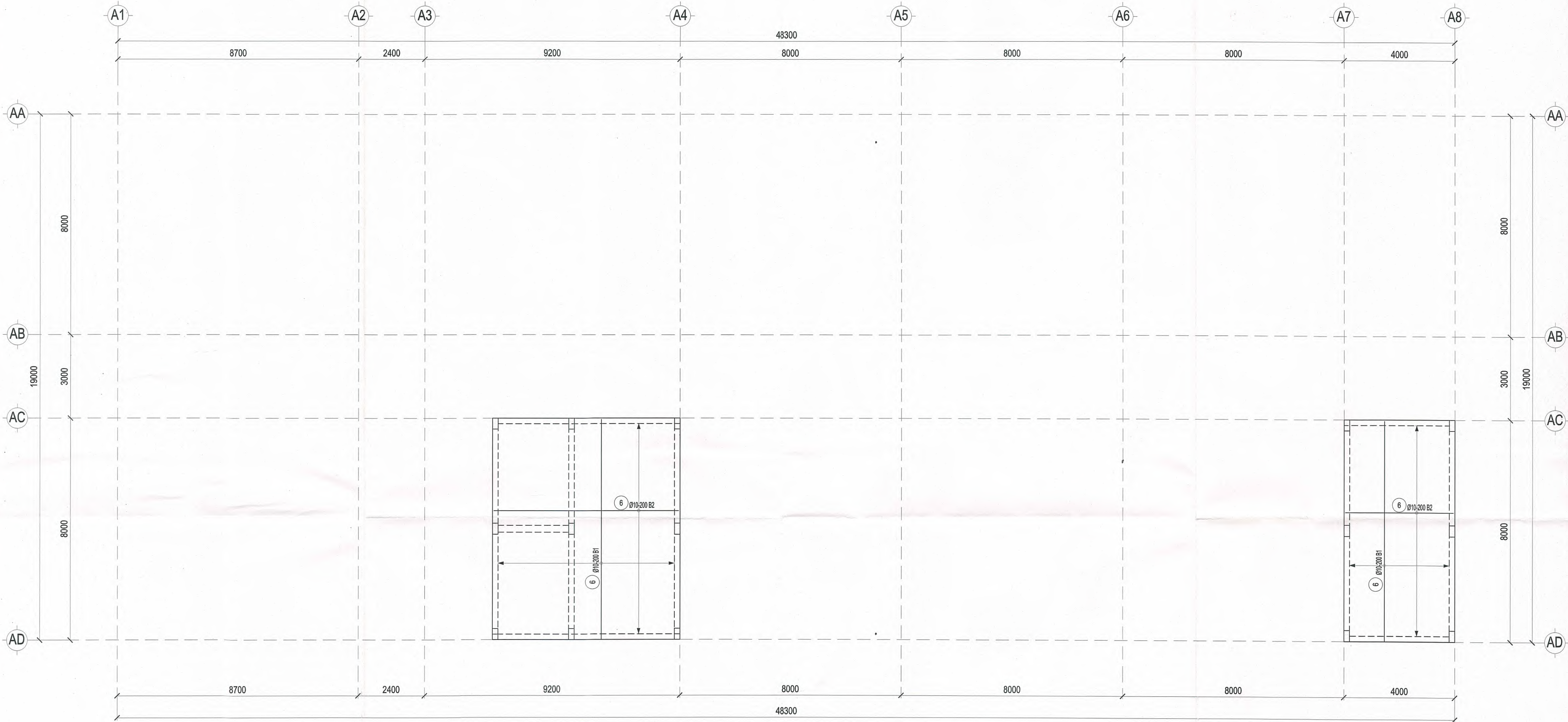
MẶT BẰNG THÉP SÀN LỚP DƯỚI TẦNG MÁI TL: 1/ 100
