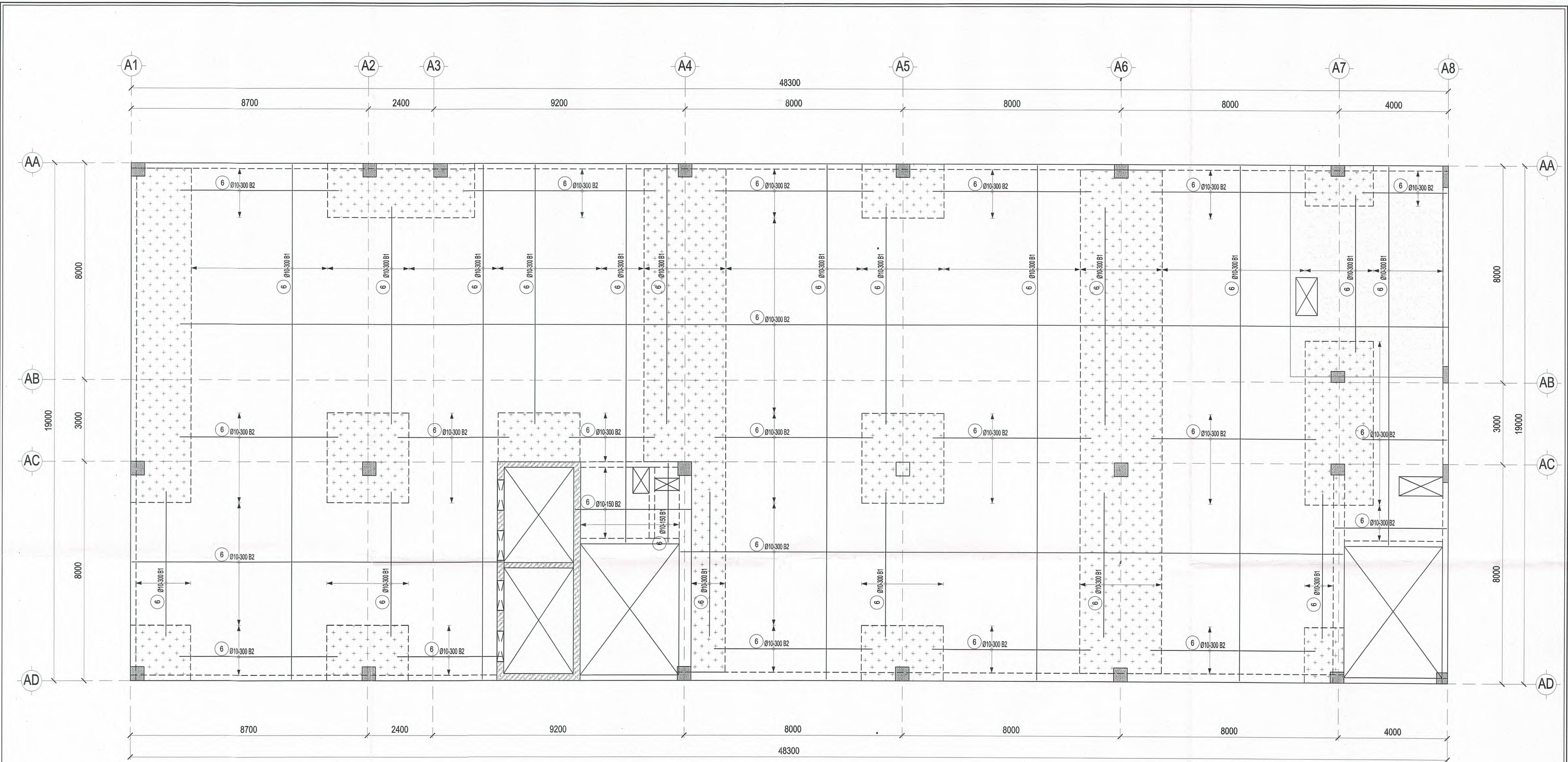
MẶT BẰNG THÉP SÀN LỚP DƯỚI TẦNG 7 TL: 1/ 100
