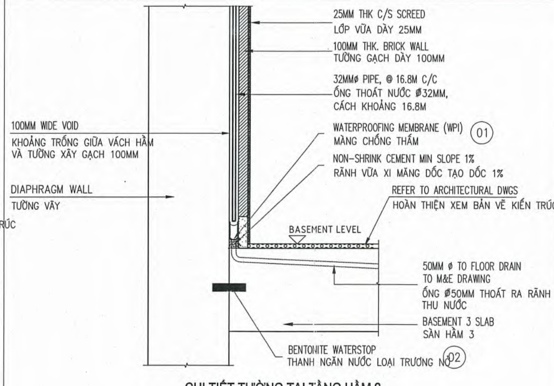
CHI TIẾT TƯỜNG TẠI TẦNG HẦM : WALL DETAIL AT BASEMENT 2
