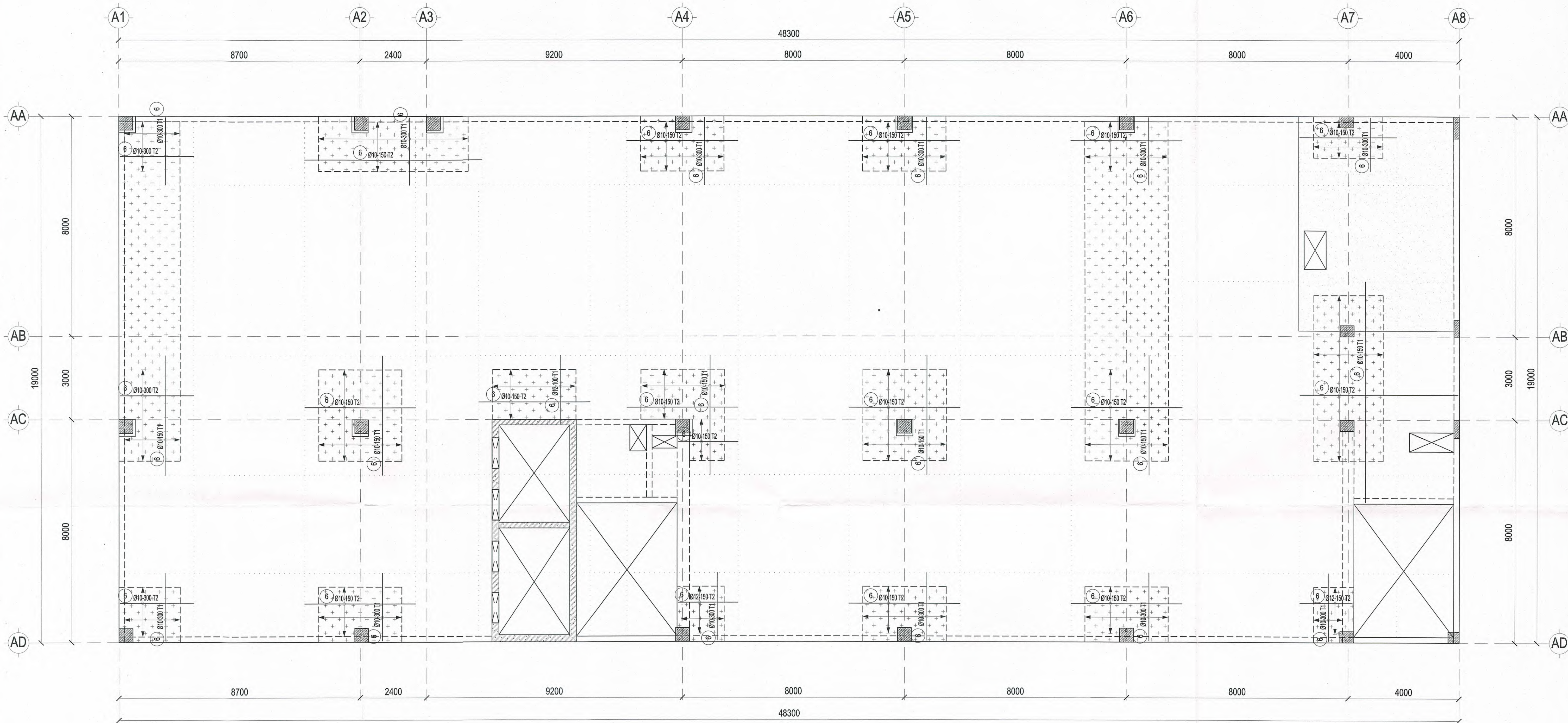
MẶT BẰNG THÉP SÀN TĂNG CƯỜNG LỚP TRÊN TẦNG 3 TL: 1/ 100
