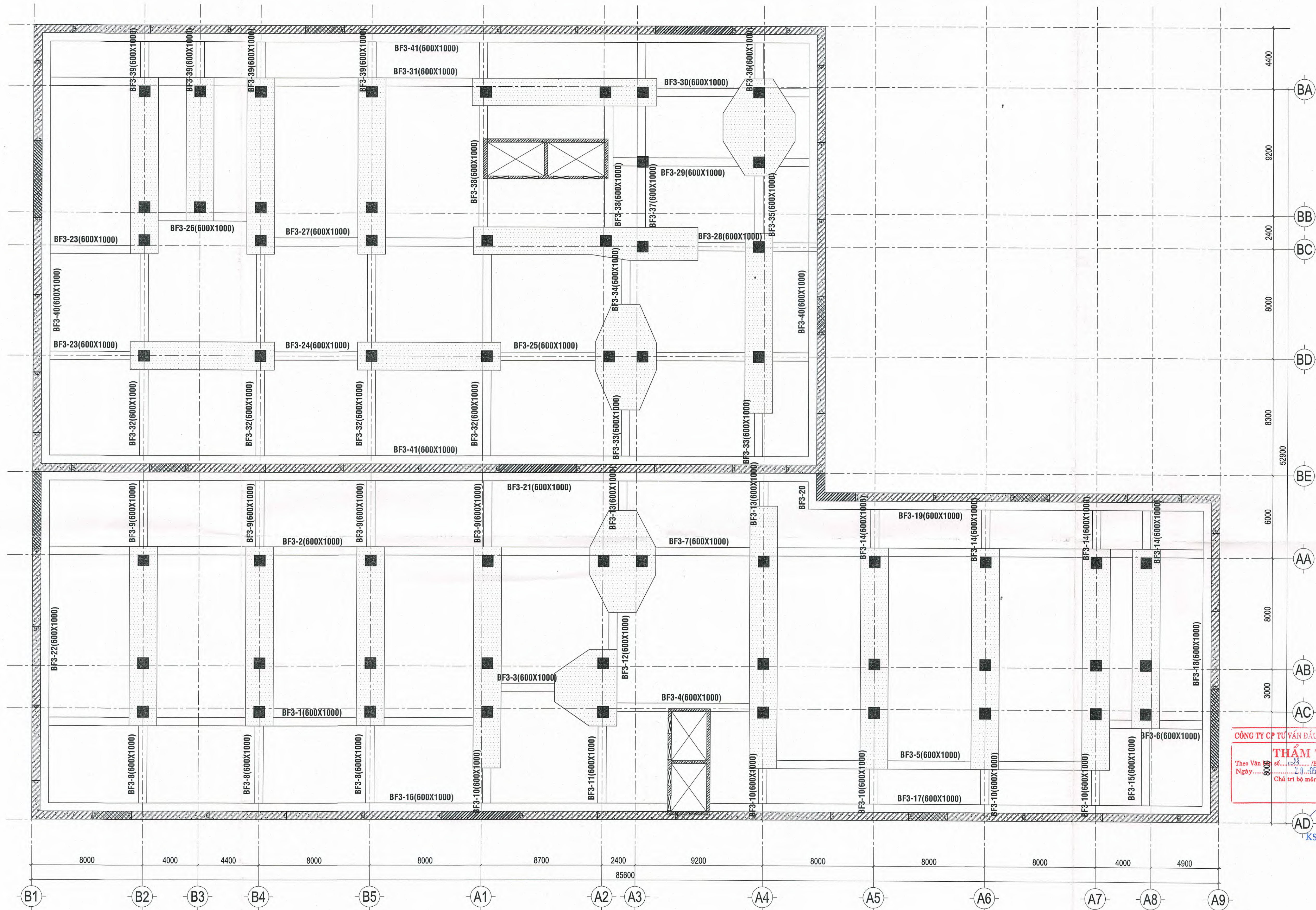
MẶT BẰNG DẦM SÀN HẦM 3 TL: 1/100
