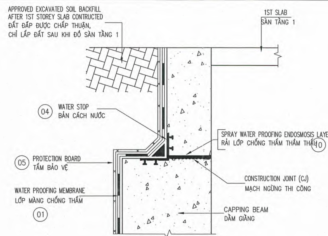
CHI TIẾT CHỐNG THẨM TẠI KHU VỰC ĐẤT ĐẬP WATER PROOFING AT EXCAVATED SOIL ZONE DETAILS
