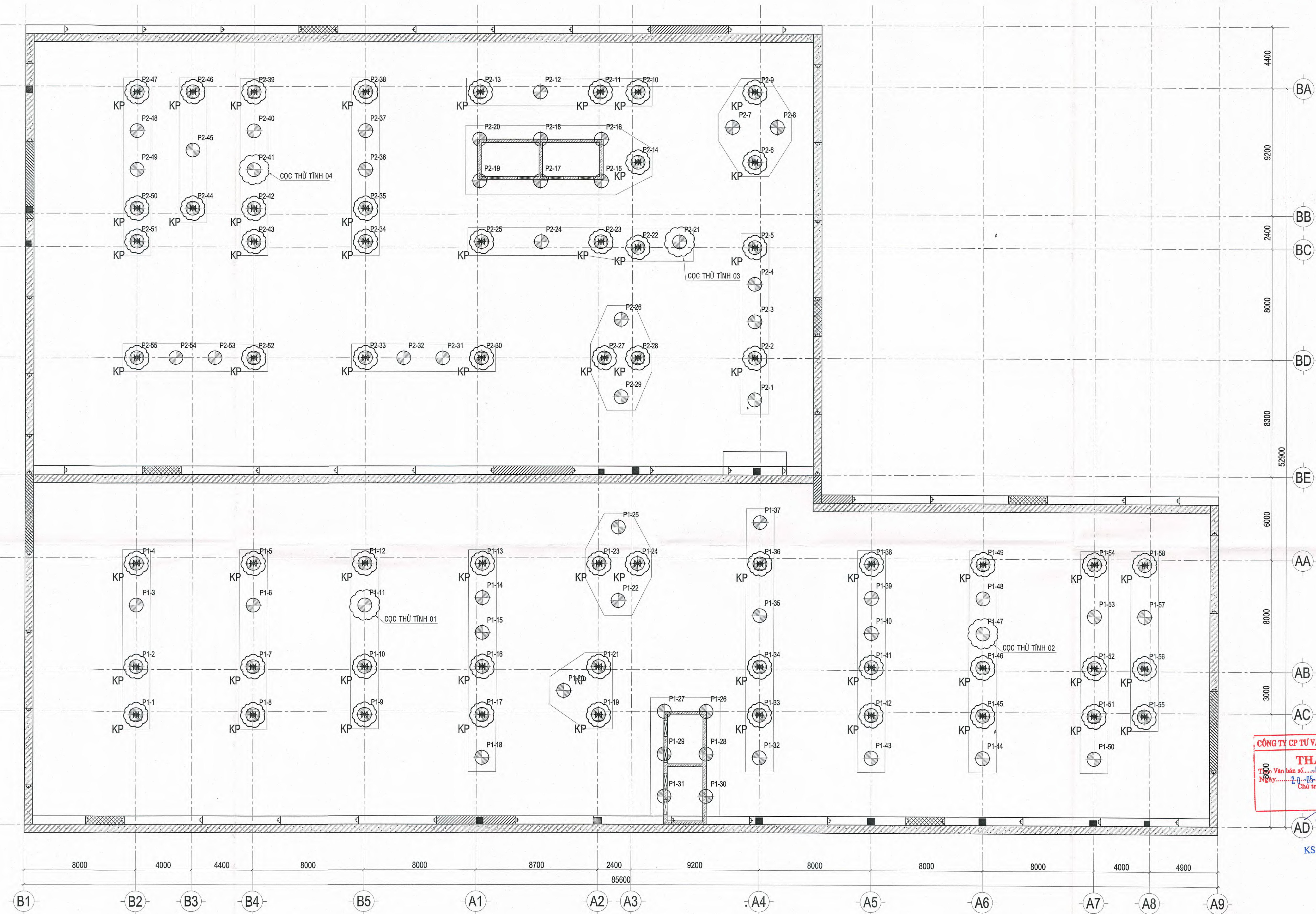
MẶT BẰNG ĐỊNH VỊ CỌC KINGPOST TL: 1/200
