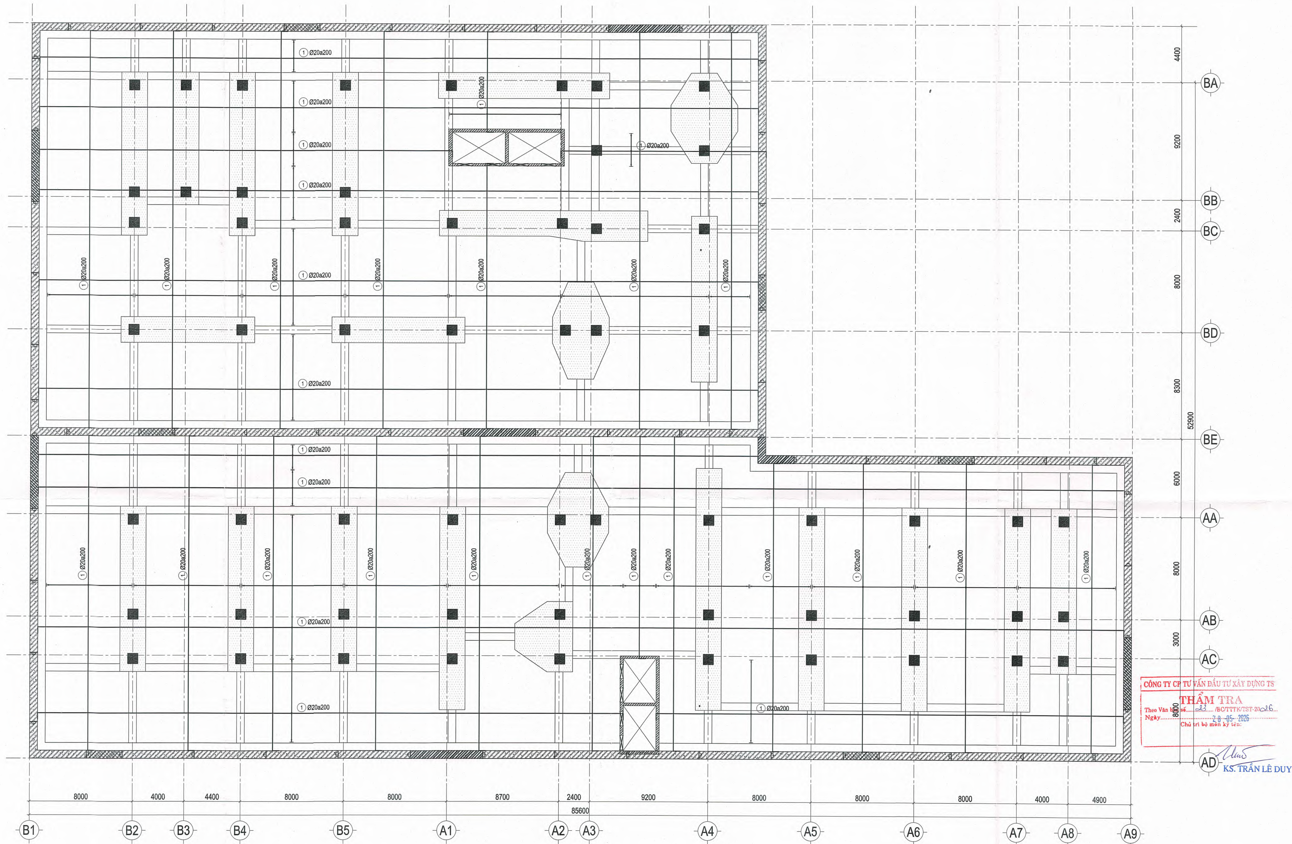
MẶT BẰNG THÉP LỚP TRÊN SÀN HẦM 3 TL: 1/100
