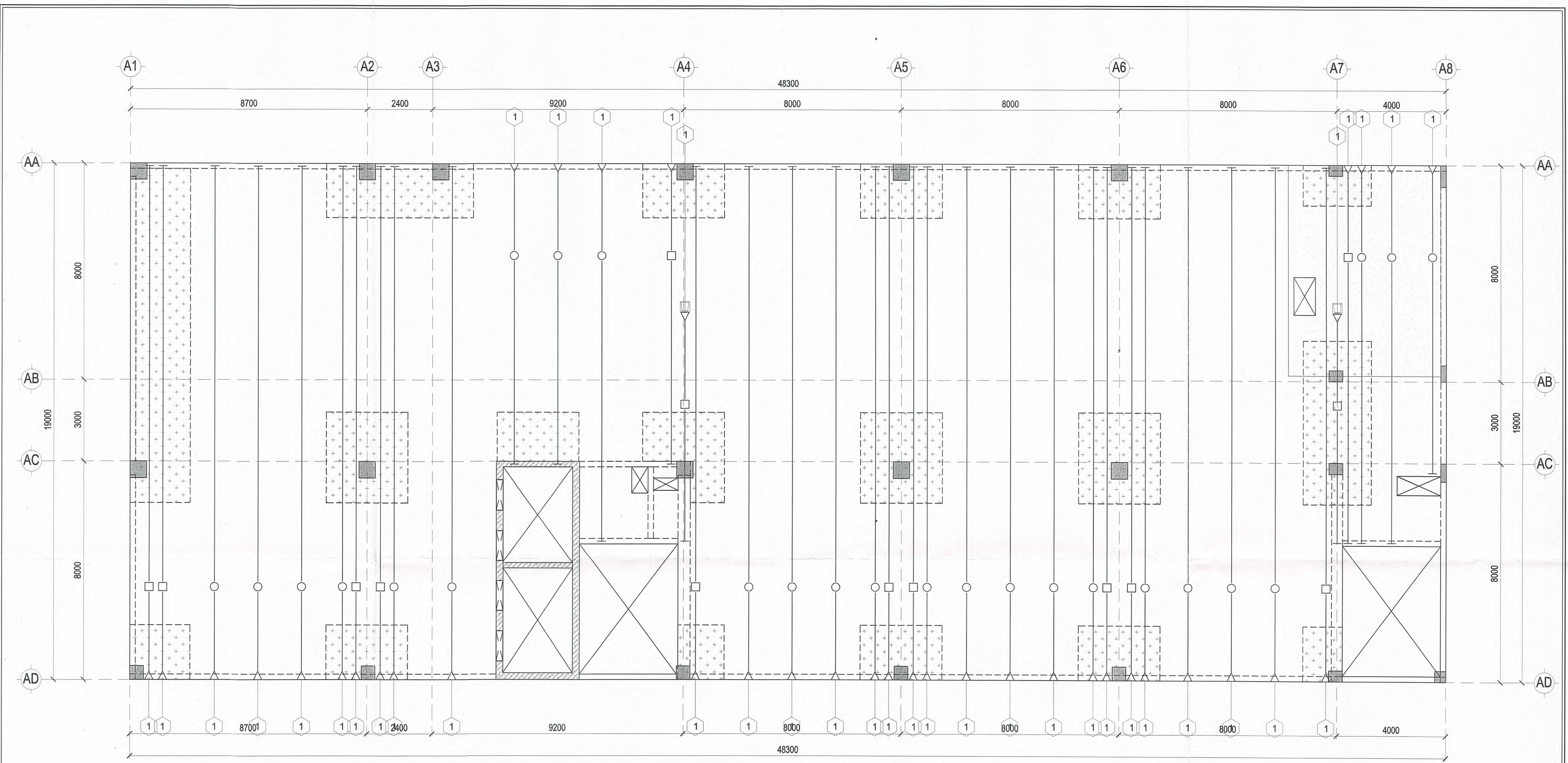
MẶT BẰNG CẤP SÀN PHƯƠNG Y TẦNG 2 TL: 1/ 100
