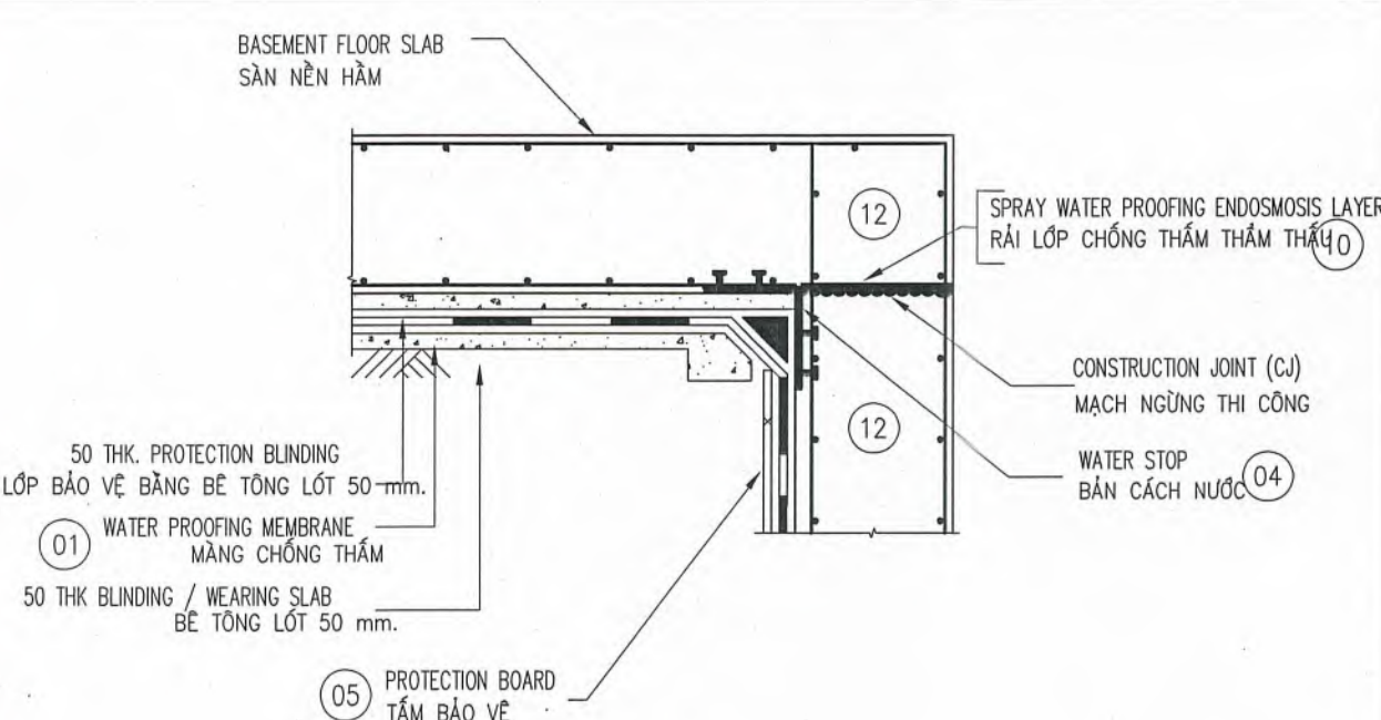
5. CHI TIẾT MỐI NỐI SÀN/ TƯỜNG HỒ THU 5. SLAB/ PIT WALL JOINT DETAIL
