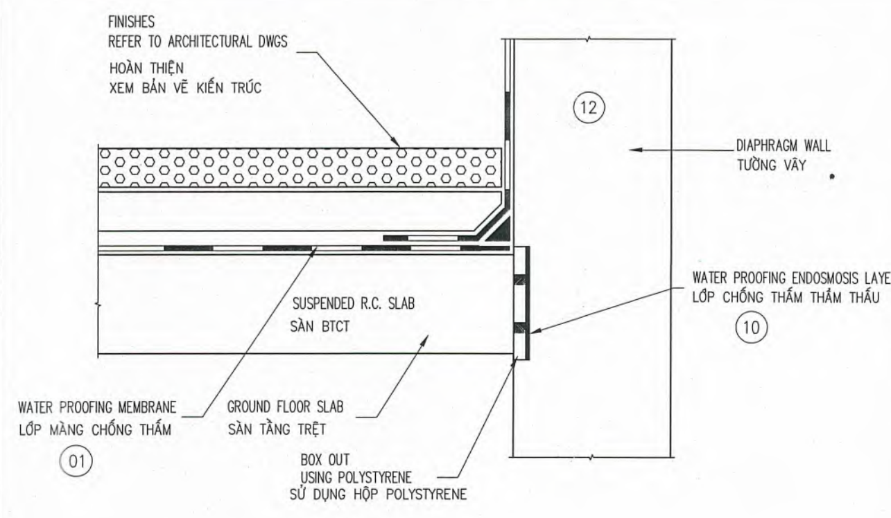
9. CHI TIẾT MỐI NỐI SÀN TREO/ TƯỜNG 9. SUSPENDED SLAB /WALL JOINT DETAIL
