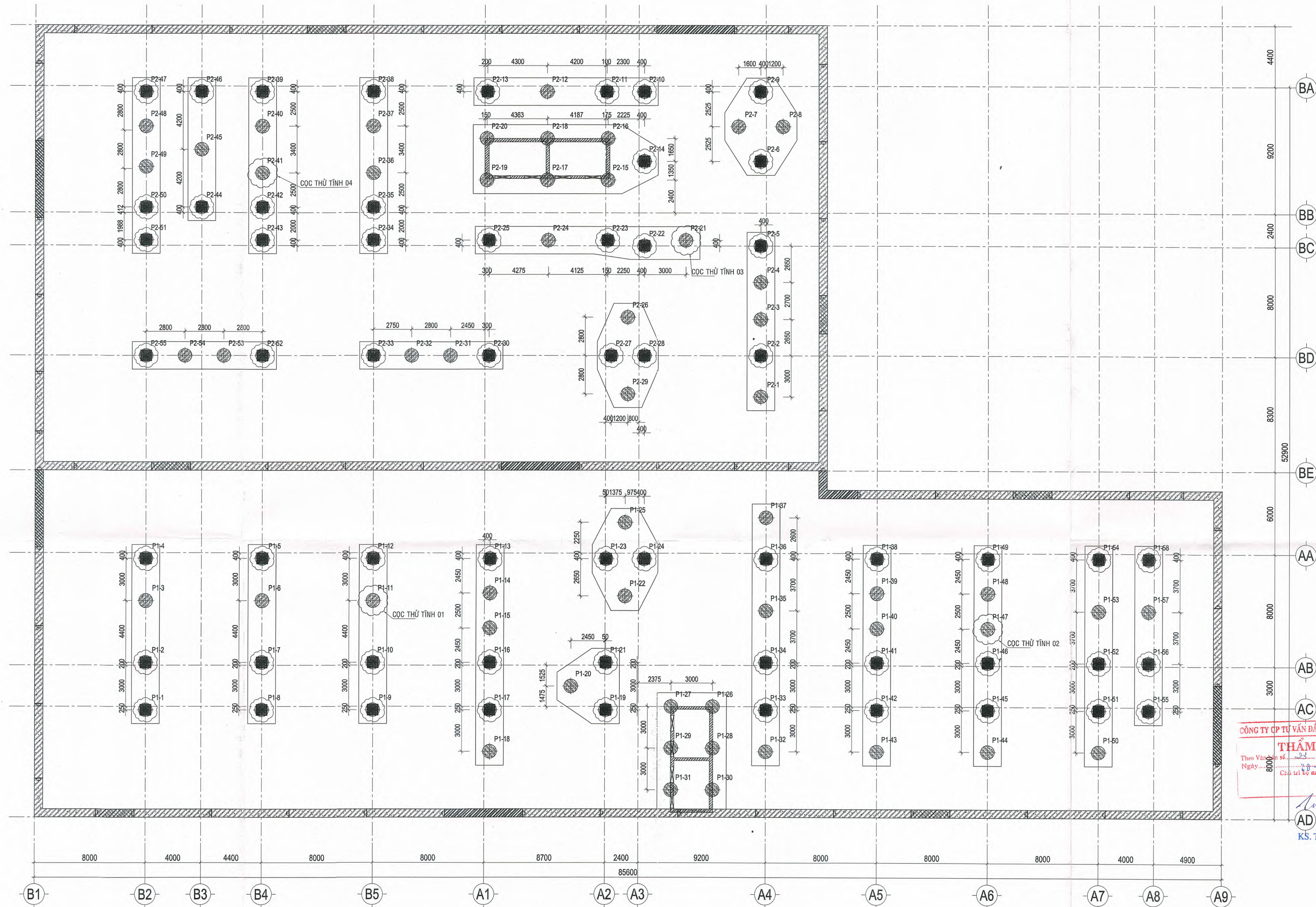
MẶT BẰNG ĐỊNH VỊ CỘC TL: 1/100
