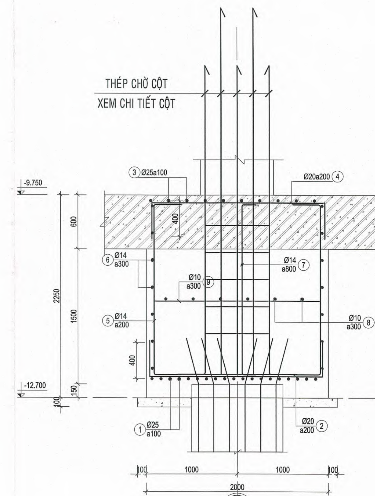
MC 1-1 TL: 1/25
