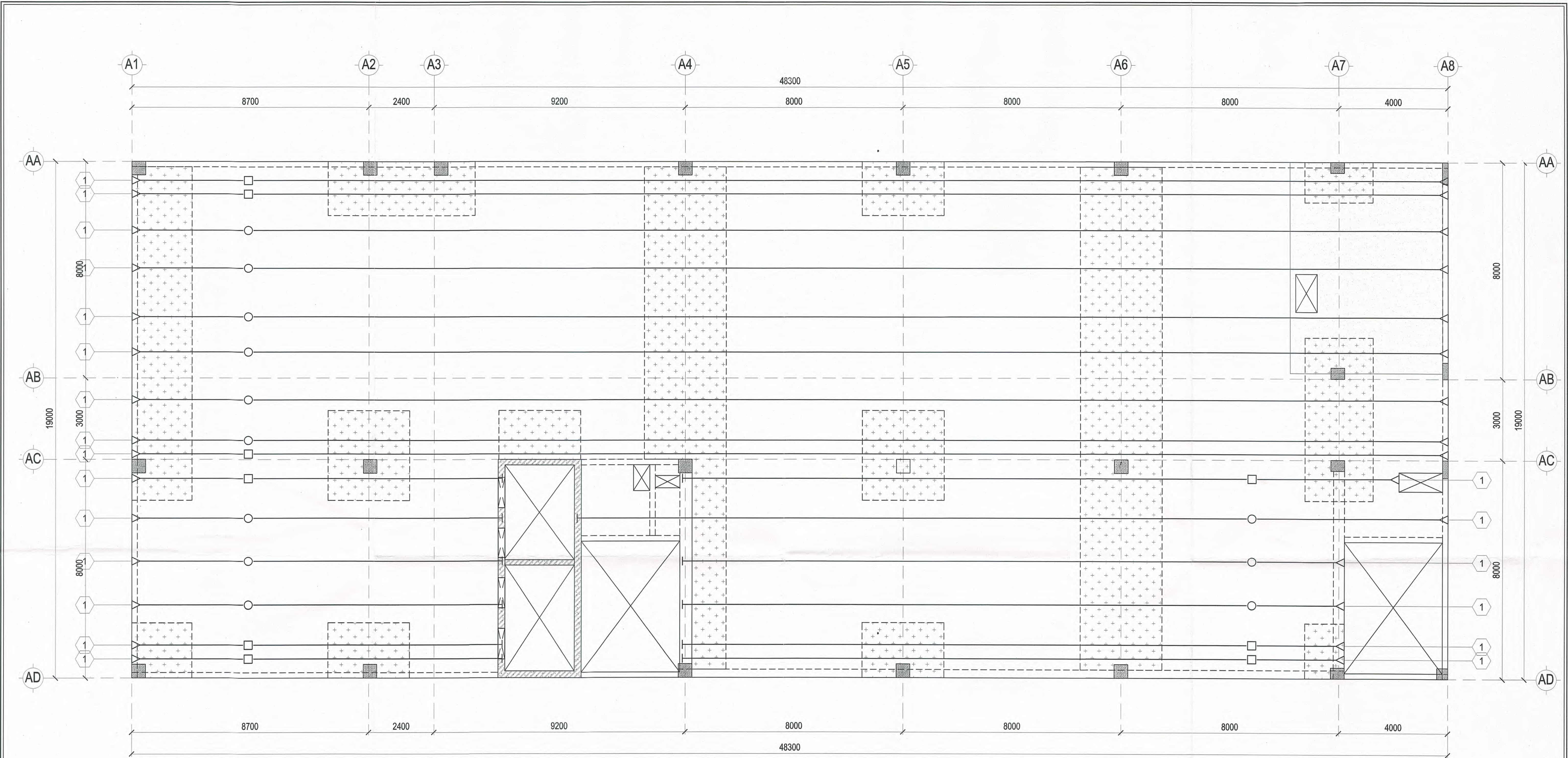
MẶT BẰNG CẤP SÀN PHƯƠNG X TẦNG 7 TL: 1/ 100
