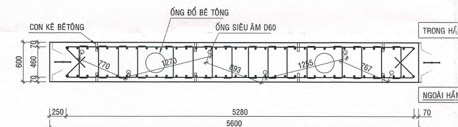
CHI TIẾT ỔNG SIÊU ÂM VÀ CON KÊ BÊ TÔNG
