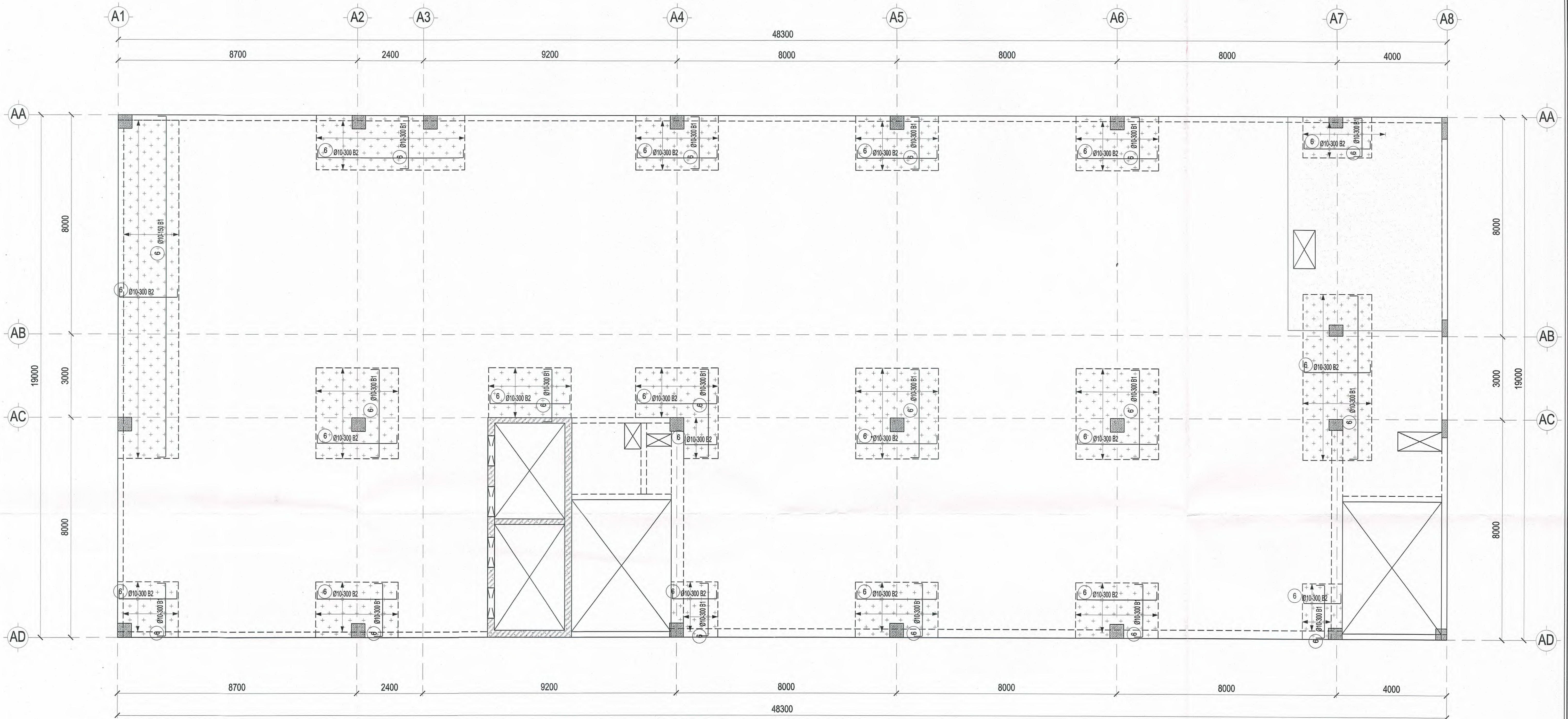
MẶT BẰNG THÉP SÀN TẦNG CƯỜNG LỚP DƯỚI TẦNG 4-6 TL: 1/ 100
