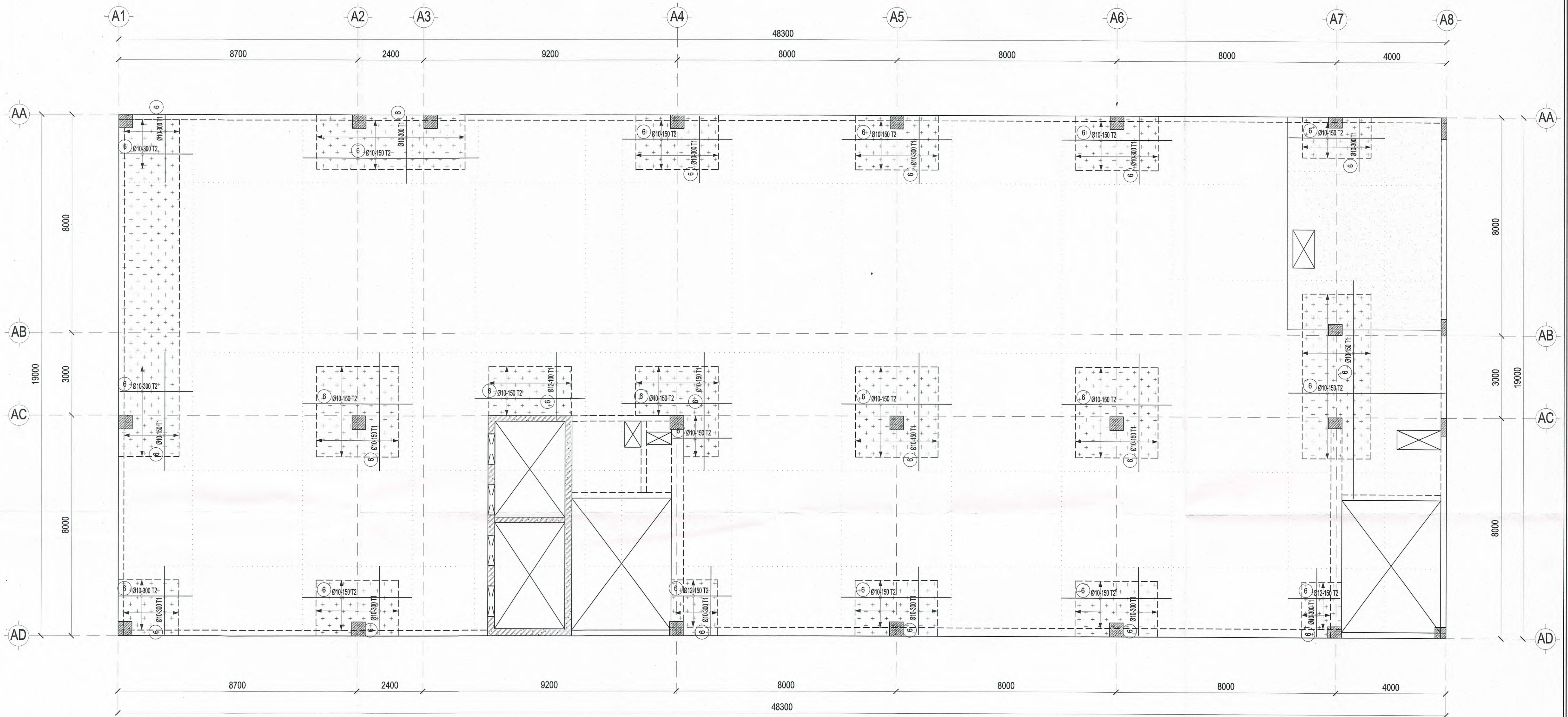
MẶT BẰNG THÉP SÀN TẦNG CƯỜNG LỚP TRÊN TẦNG 4-6 TL: 1/ 100
