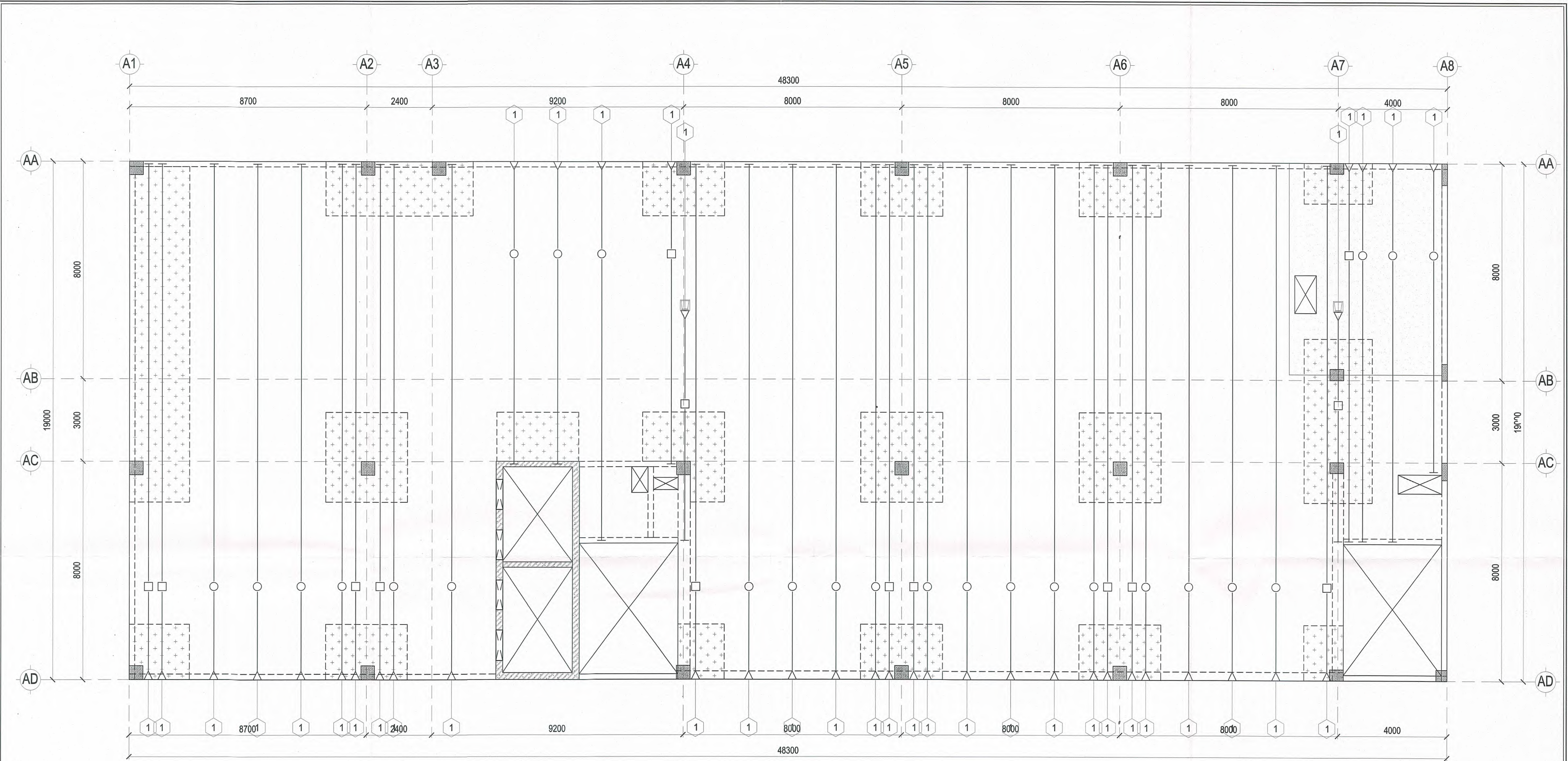
MẶT BẰNG CẤP SÀN PHƯƠNG Y TẦNG 4-6 TL: 1/ 100
