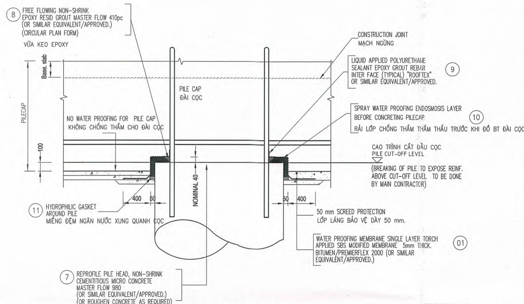
3. CHI TIẾT MỐI NỐI CỌC/ ĐÀI CỌC 3. PILE/ PILECAP JOINT DETAIL
