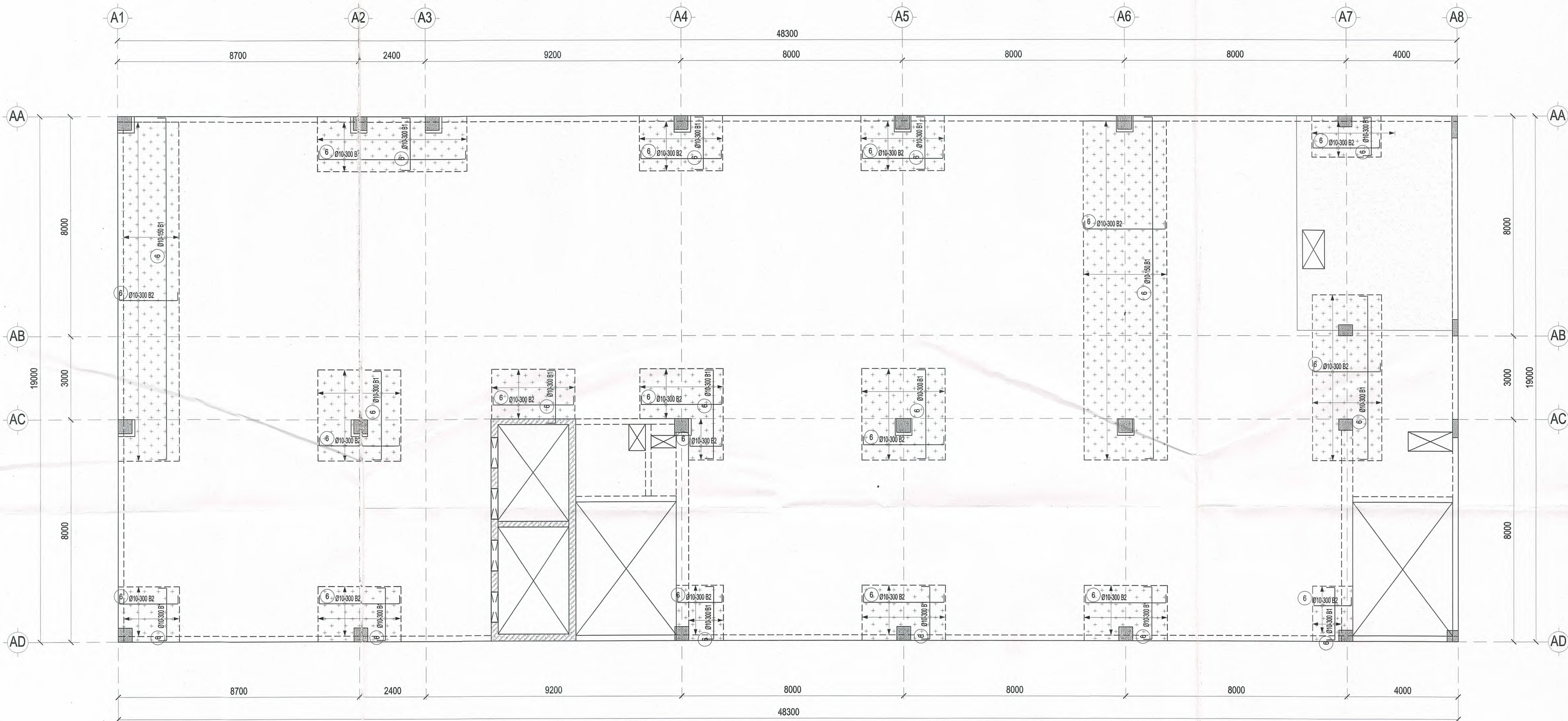
MẶT BẰNG THÉP SÀN TẦNG CƯỜNG LỚP DƯỚI TẦNG 3 TL: 1/ 100
