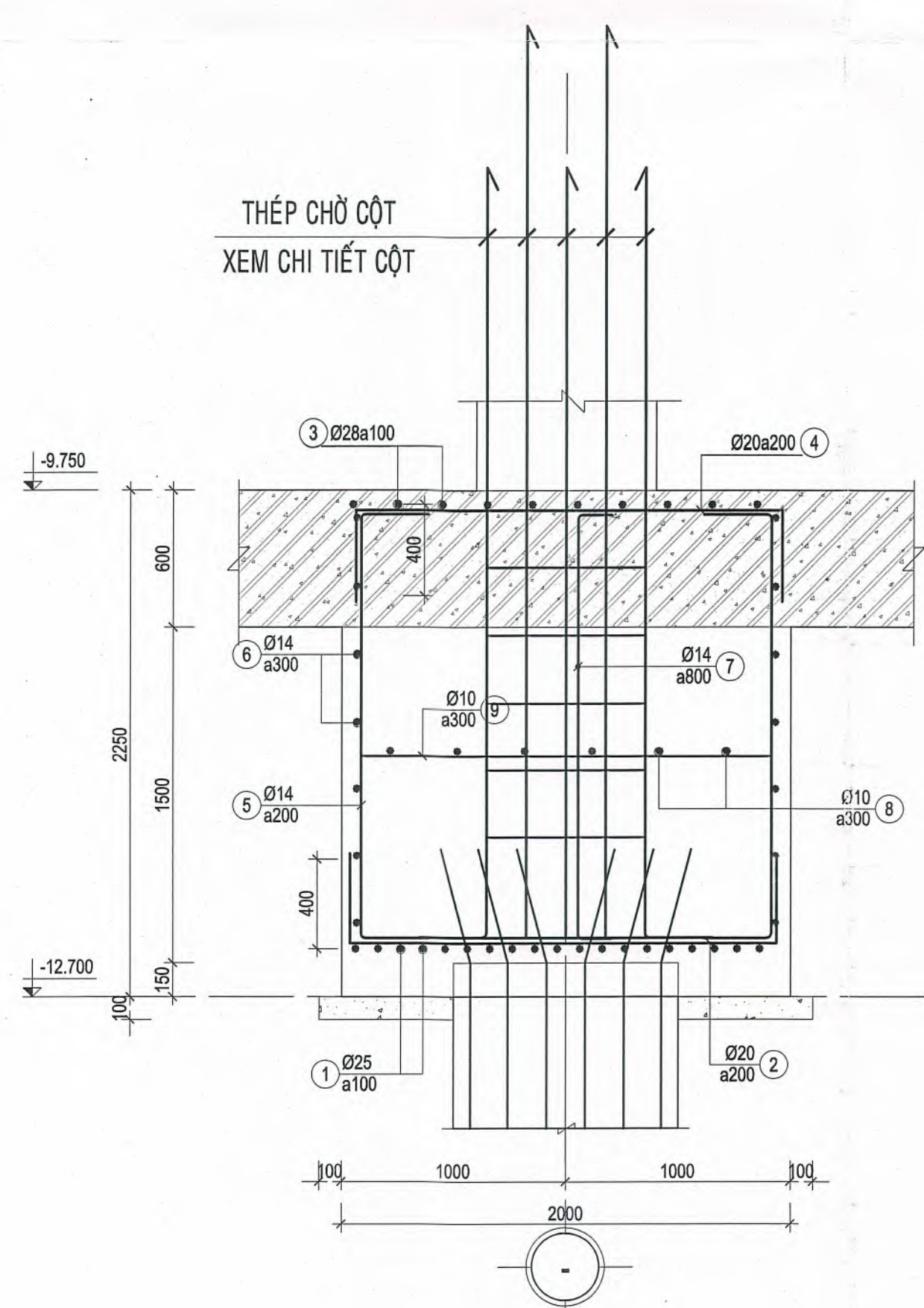
MC 2-2 TL: 1/25
