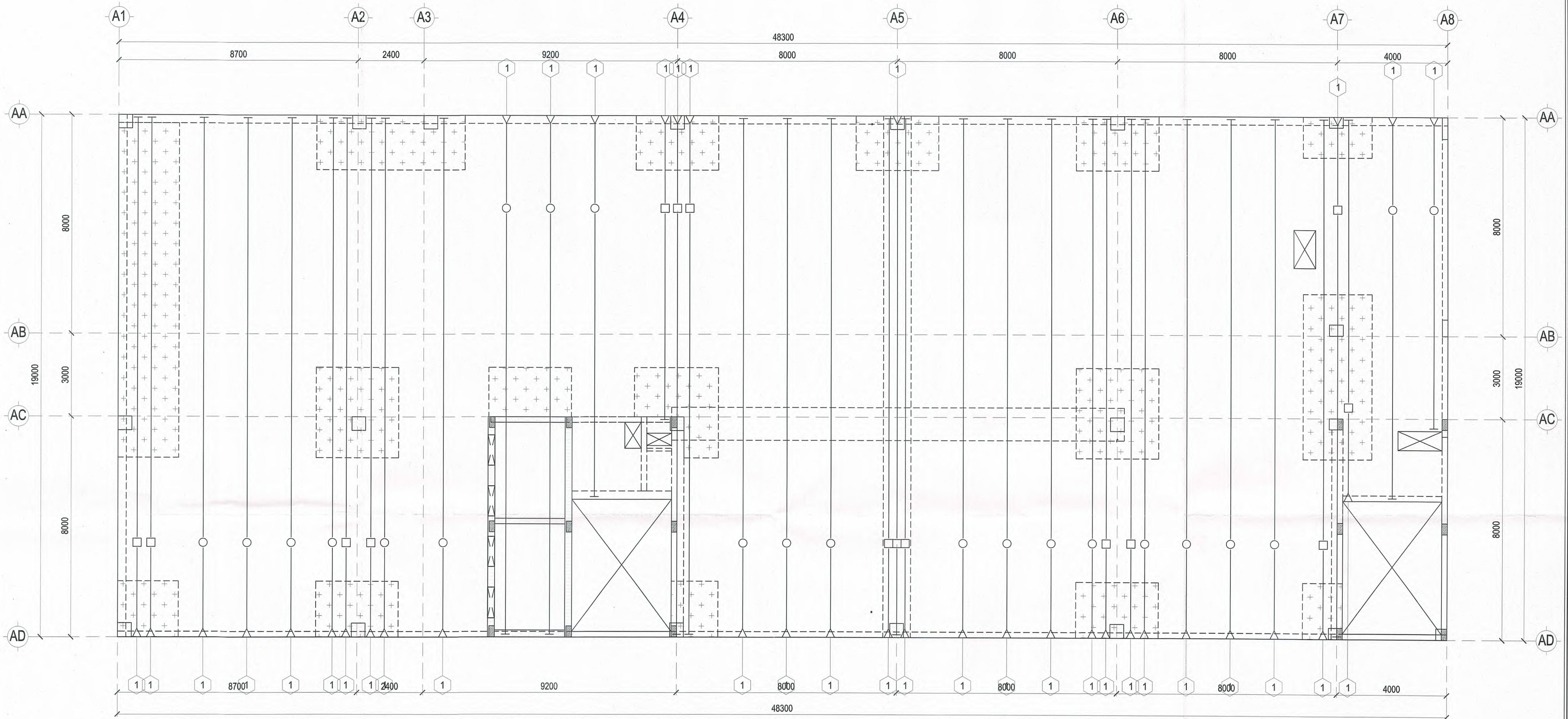
MẶT BẰNG CẤP SÀN PHƯƠNG Y TẦNG TUM TL: 1/ 100
