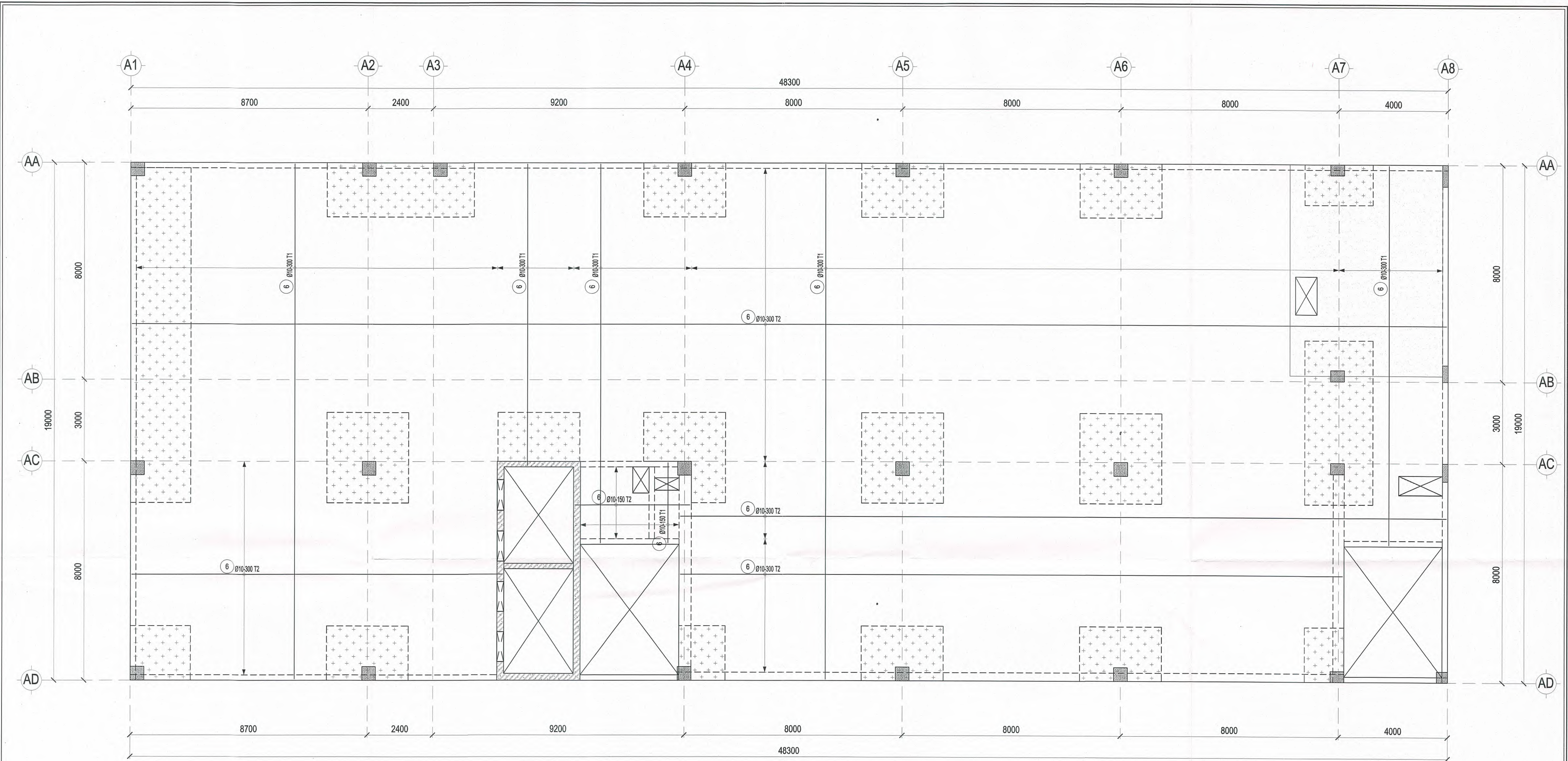
MẶT BẰNG THÉP SÀN LỚP TRÊN TẦNG 4-6 TL: 1/ 100
