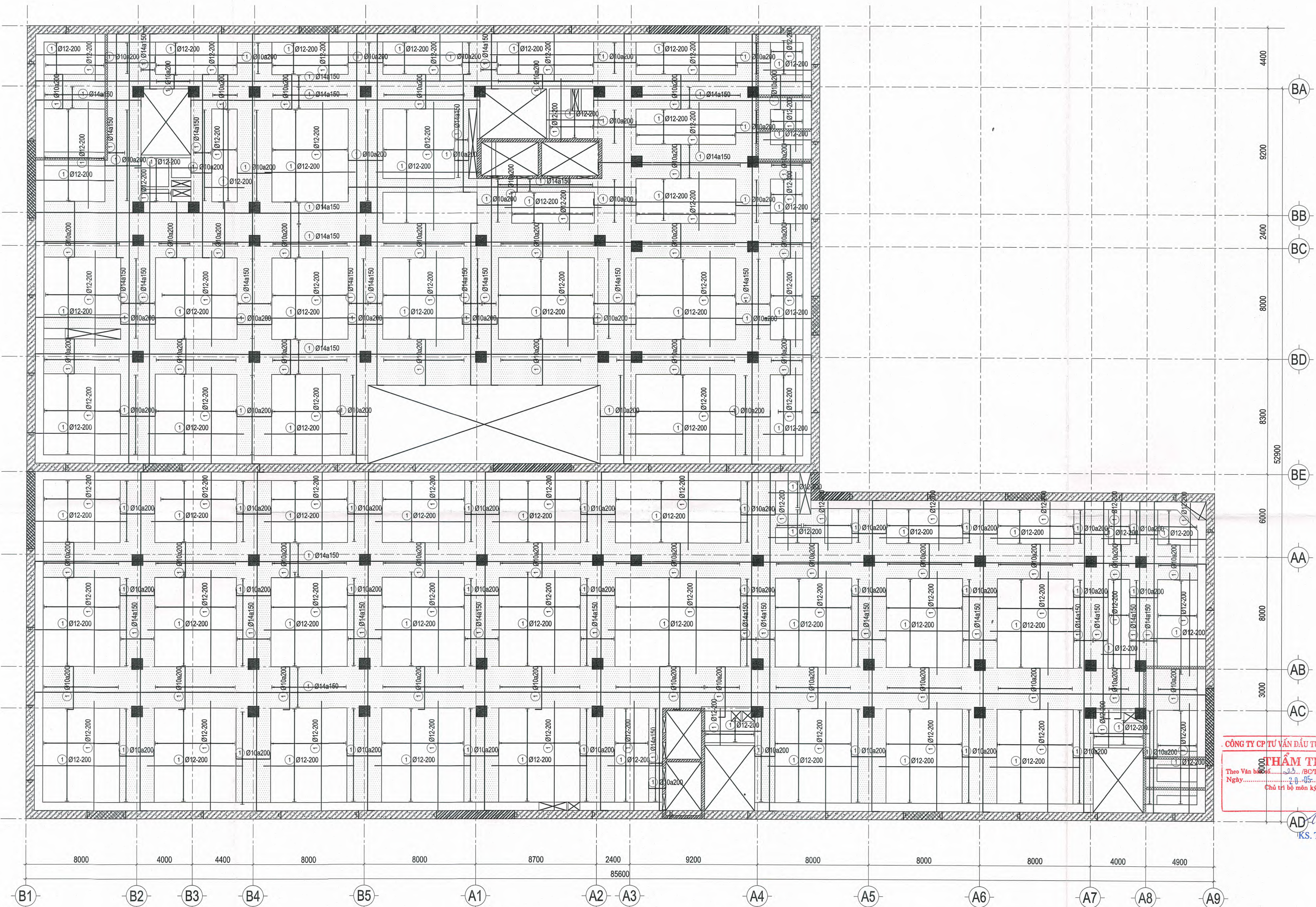
MẶT BẰNG THÉP LỚP DƯỚI SÀN HẦM 1 TL: 1/200
