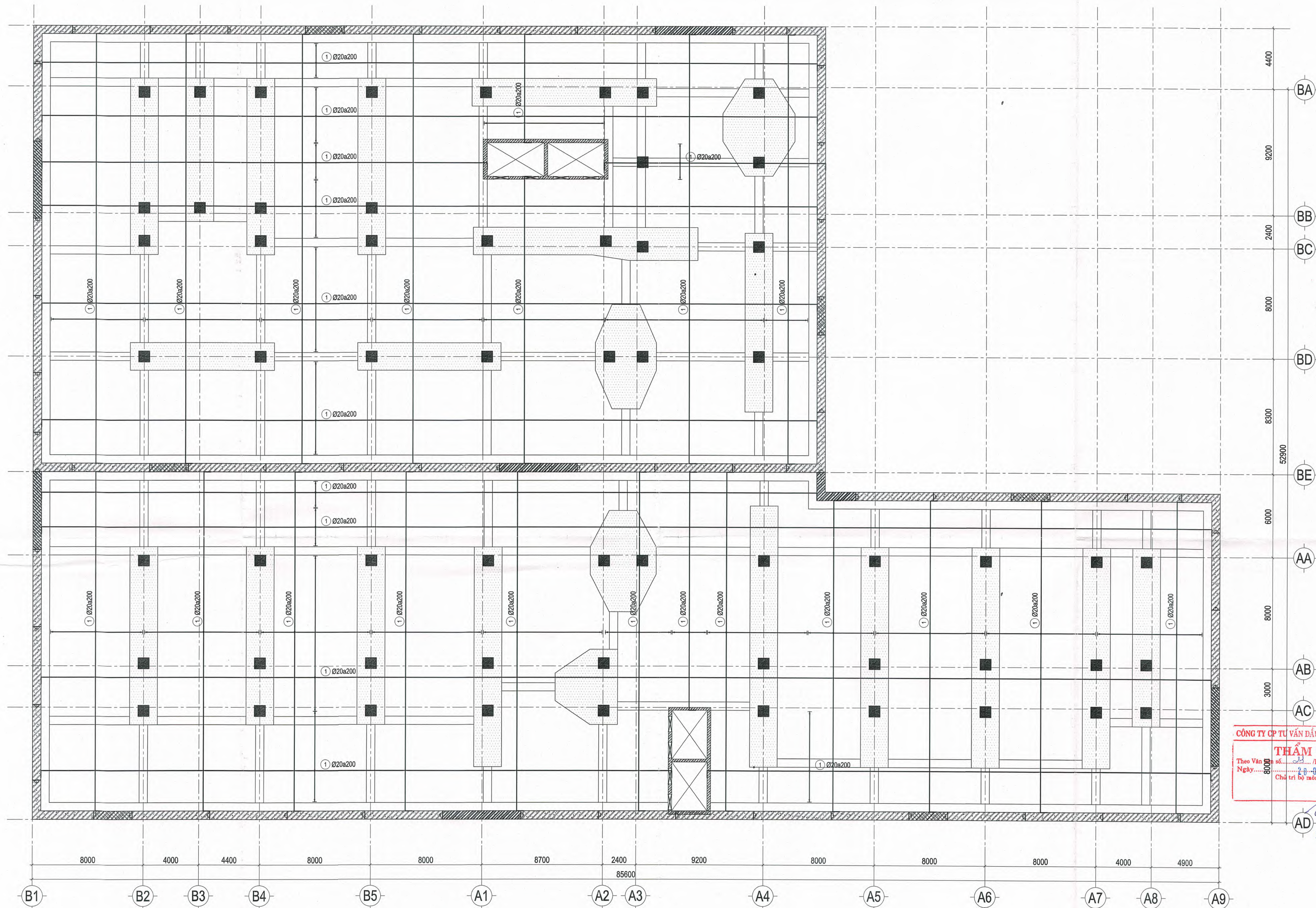
MẶT BẰNG THÉP LỚP DƯỚI SÀN HẦM 3 TL: 1/100
