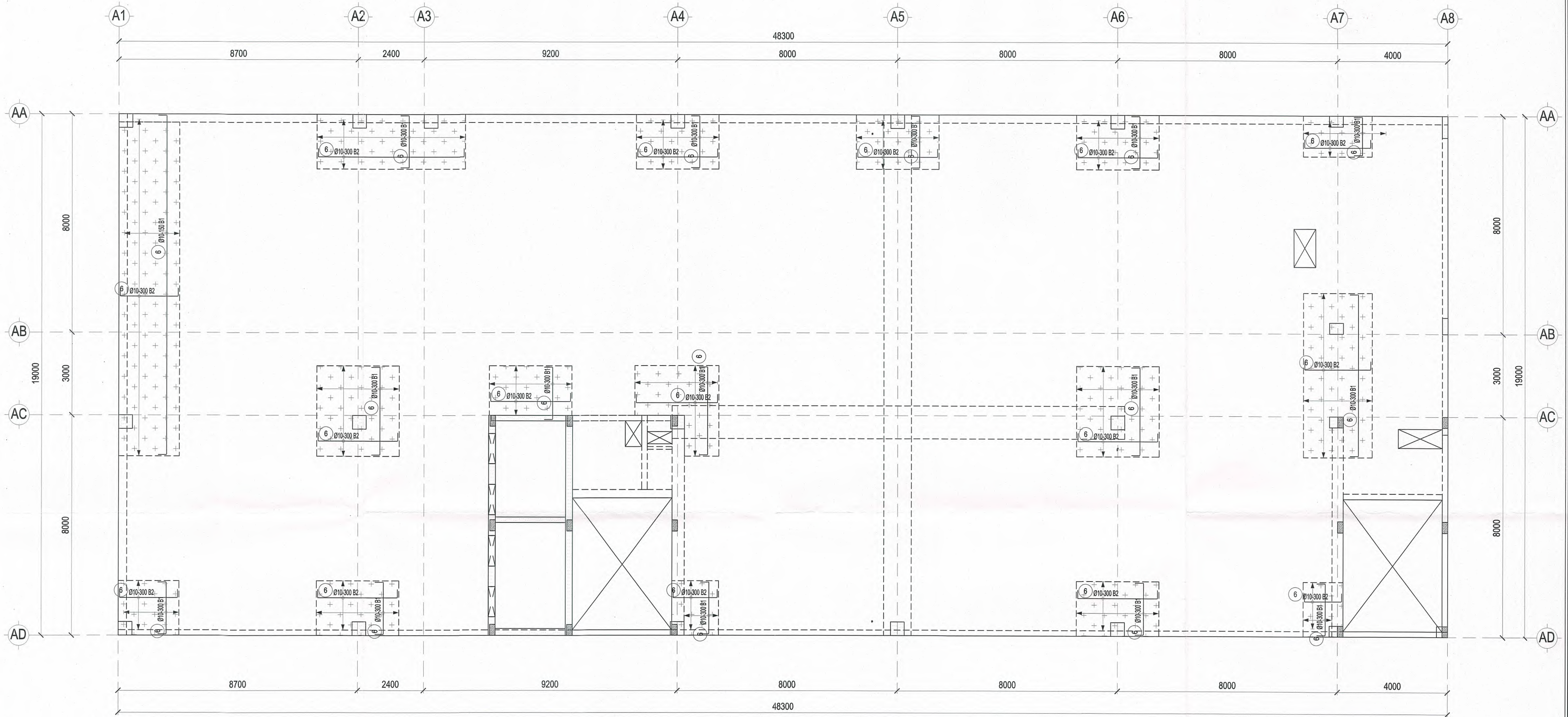
MẶT BẰNG THÉP SÀN TẦNG CƯỜNG LỚP DƯỚI TẦNG TUM
