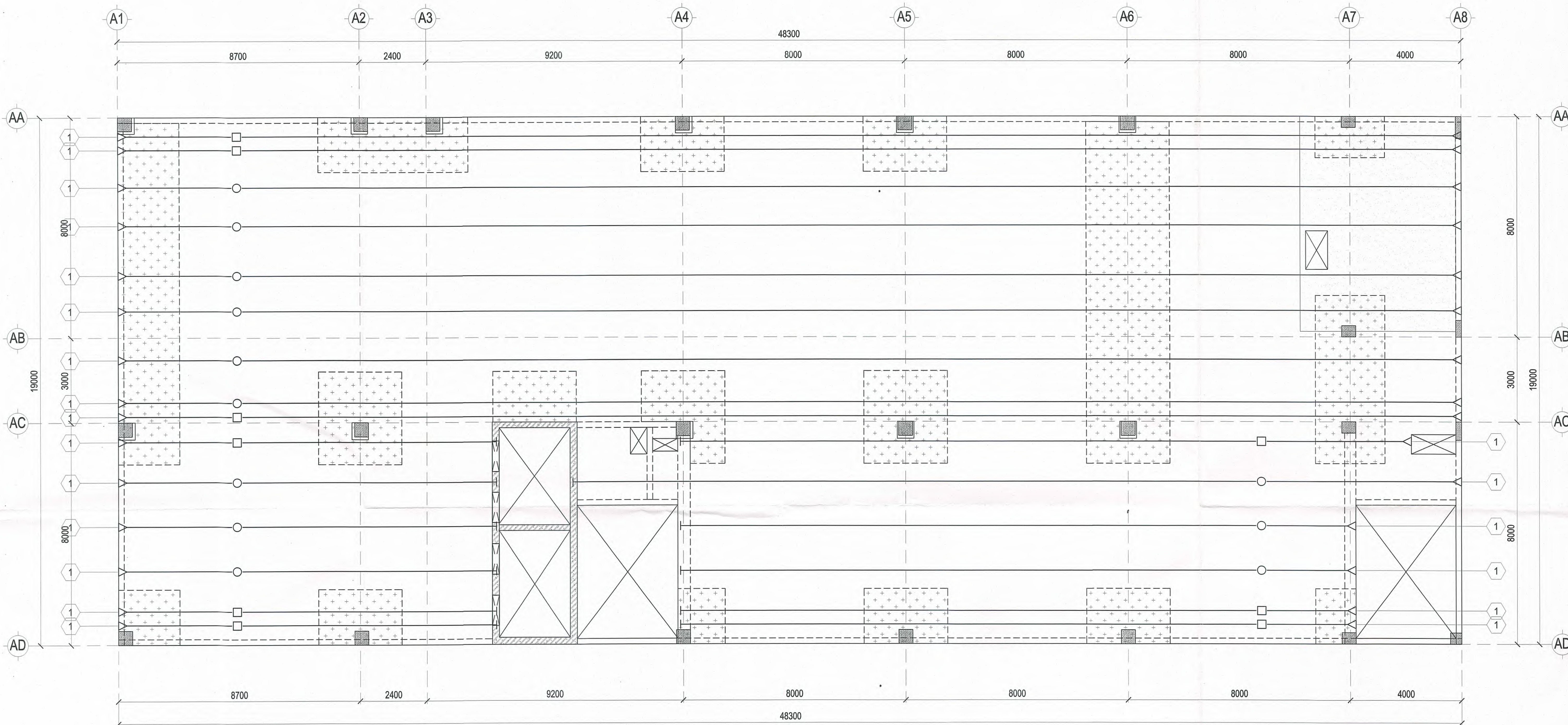
MẶT BẰNG CÁP SÀN PHƯƠNG X TẦNG 3 TL: 1/ 100
