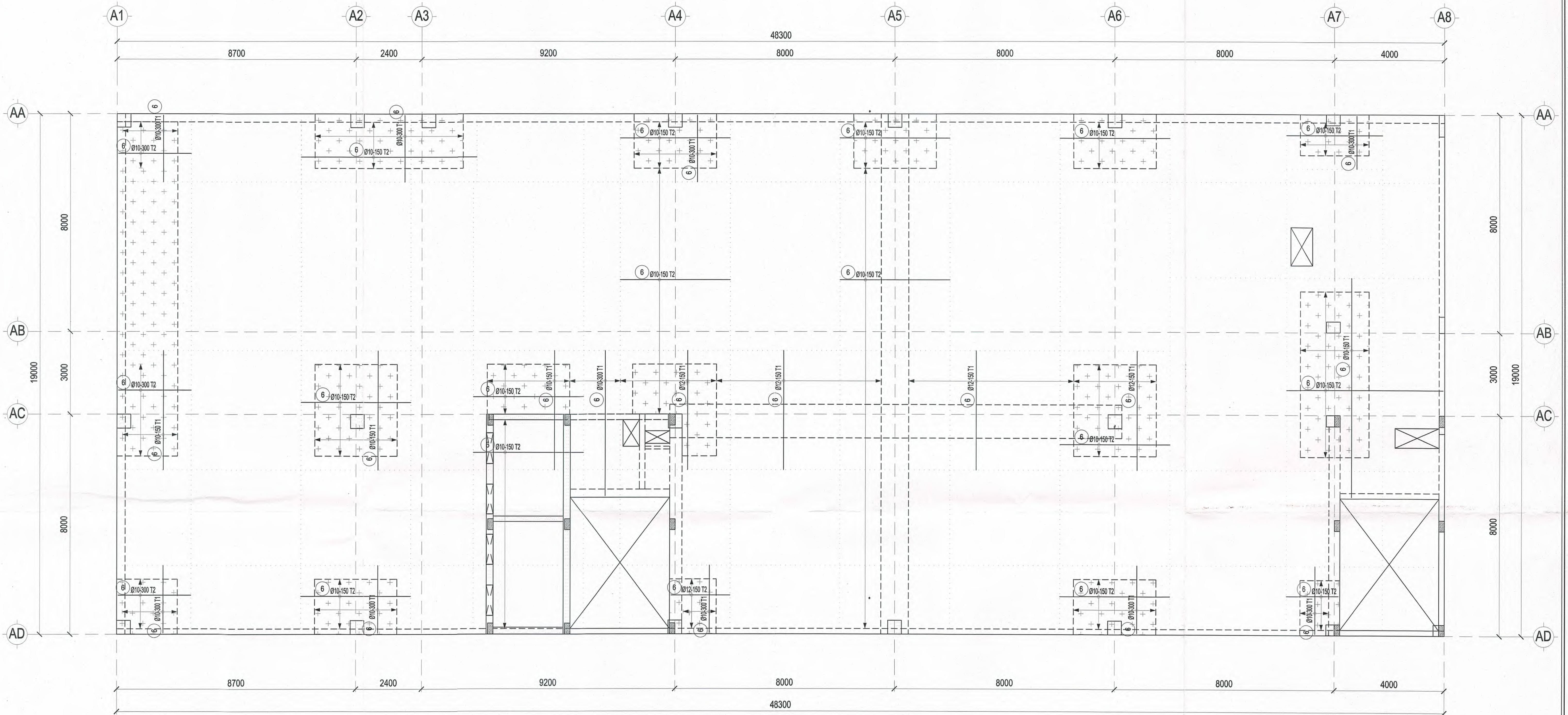
MẶT BẰNG THÉP SÀN TẦNG CƯỜNG LỚP TRÊN TẦNG TUM TL: 1/ 100
