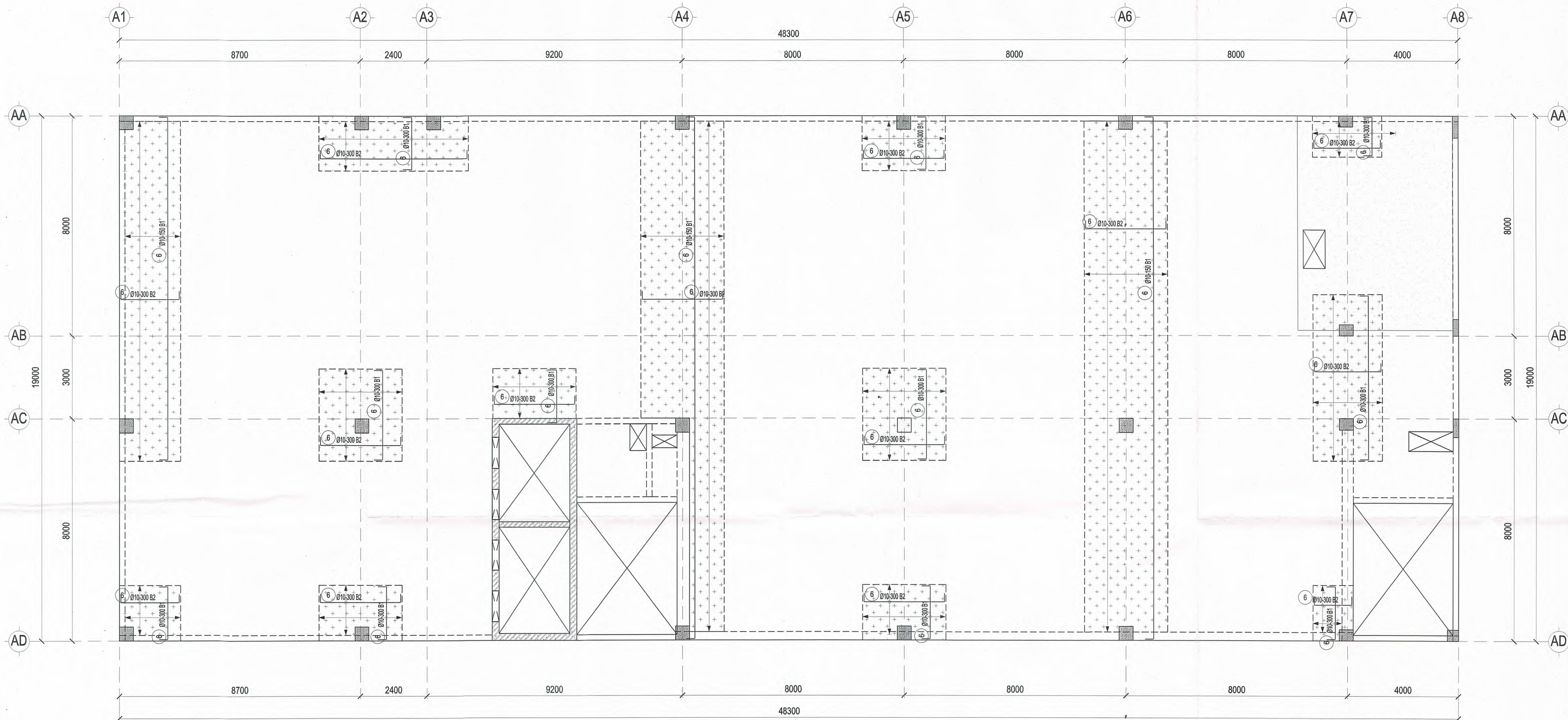
MẶT BẰNG THÉP SÀN TẦNG CƯỜNG LỚP DƯỚI TẦNG 7 TL: 1/ 100
