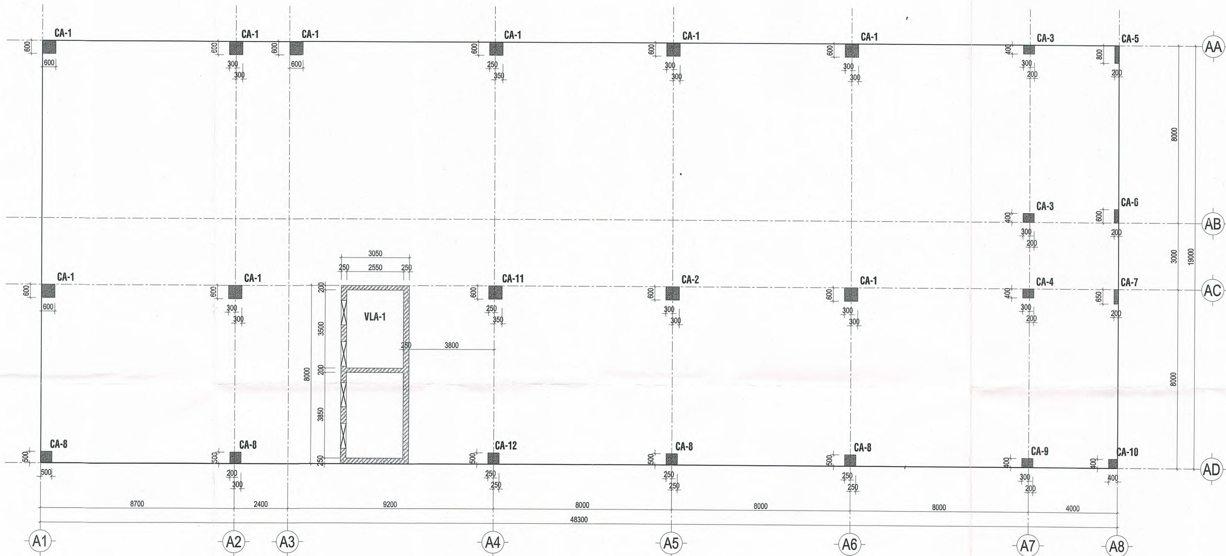
MẶT BẰNG ĐỊNH VỊ CỘT NHÀ A TẦNG 1 -> TẦNG 3
