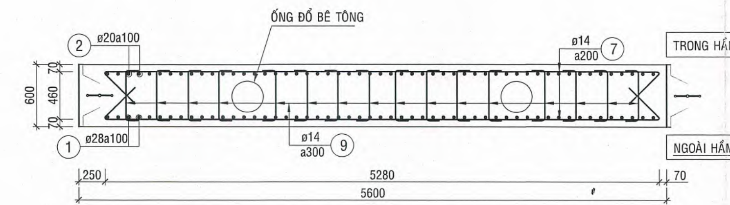
MẶT CẮT 1 - 1
