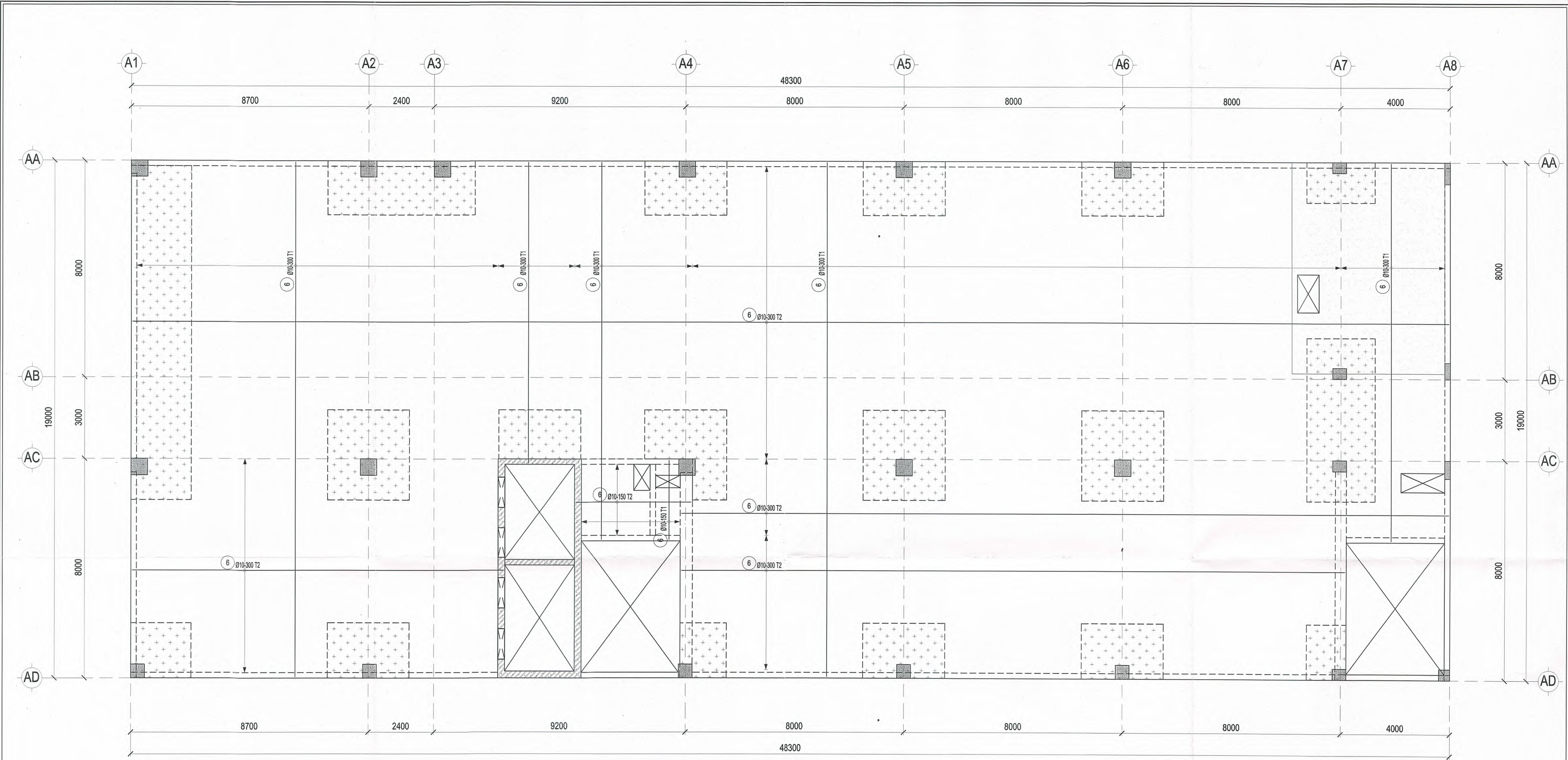
MẶT BẰNG THÉP SÀN LỚP TRÊN TẦNG 2 TL: 1/ 100
