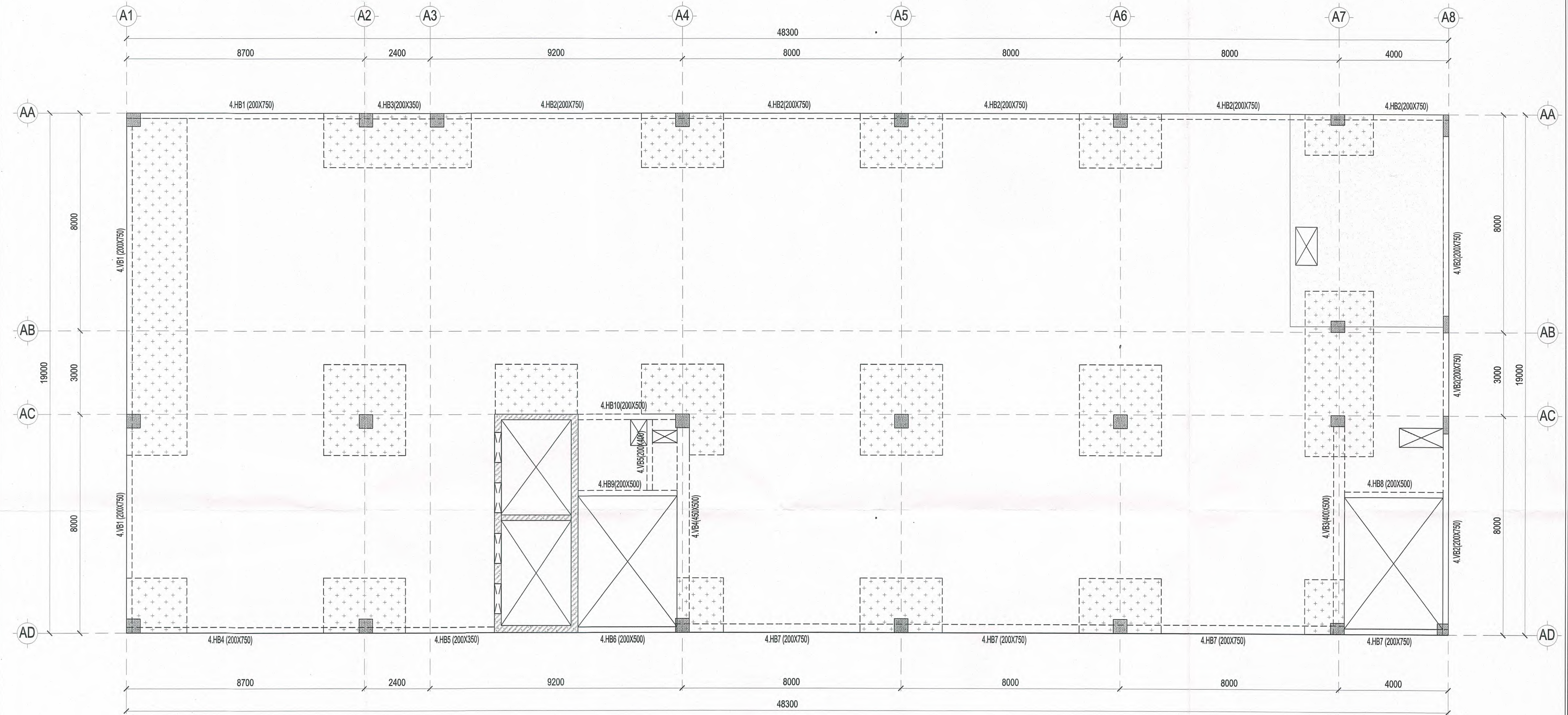
MẶT BẰNG DẦM SÀN TẦNG 4-6 TL: 1/ 100
