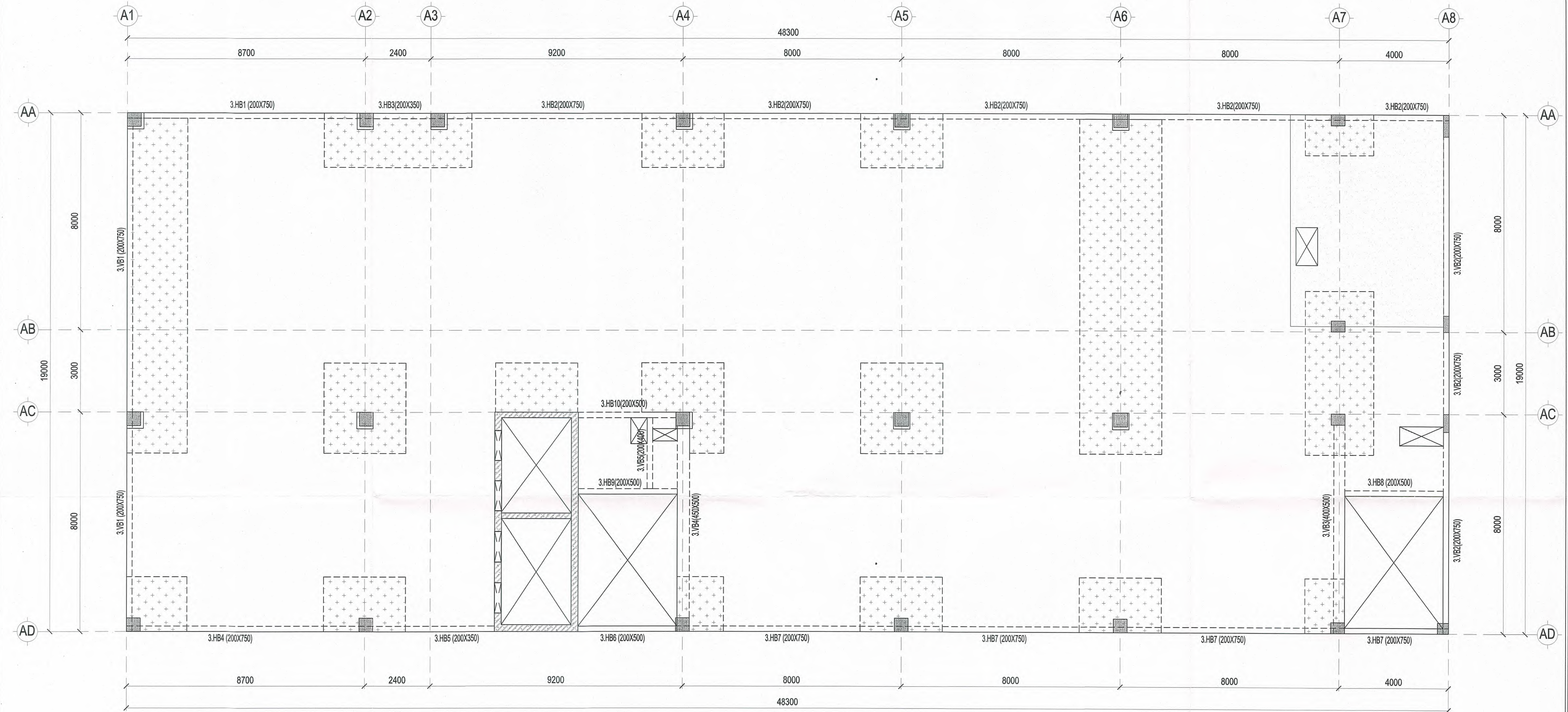
MẶT BẰNG DẦM SÀN TẦNG 3 TL: 1/ 100
