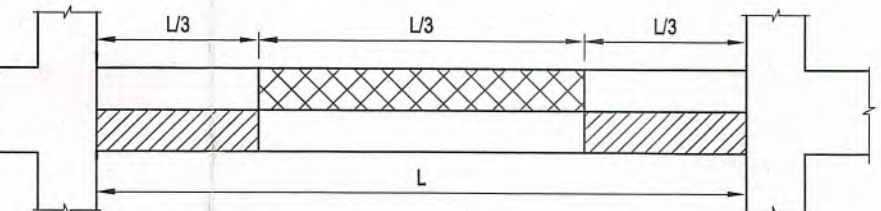
VỊ TRÍ ĐƯỢC NỐI THÉP TRONG SÀN : FOR SLAB
