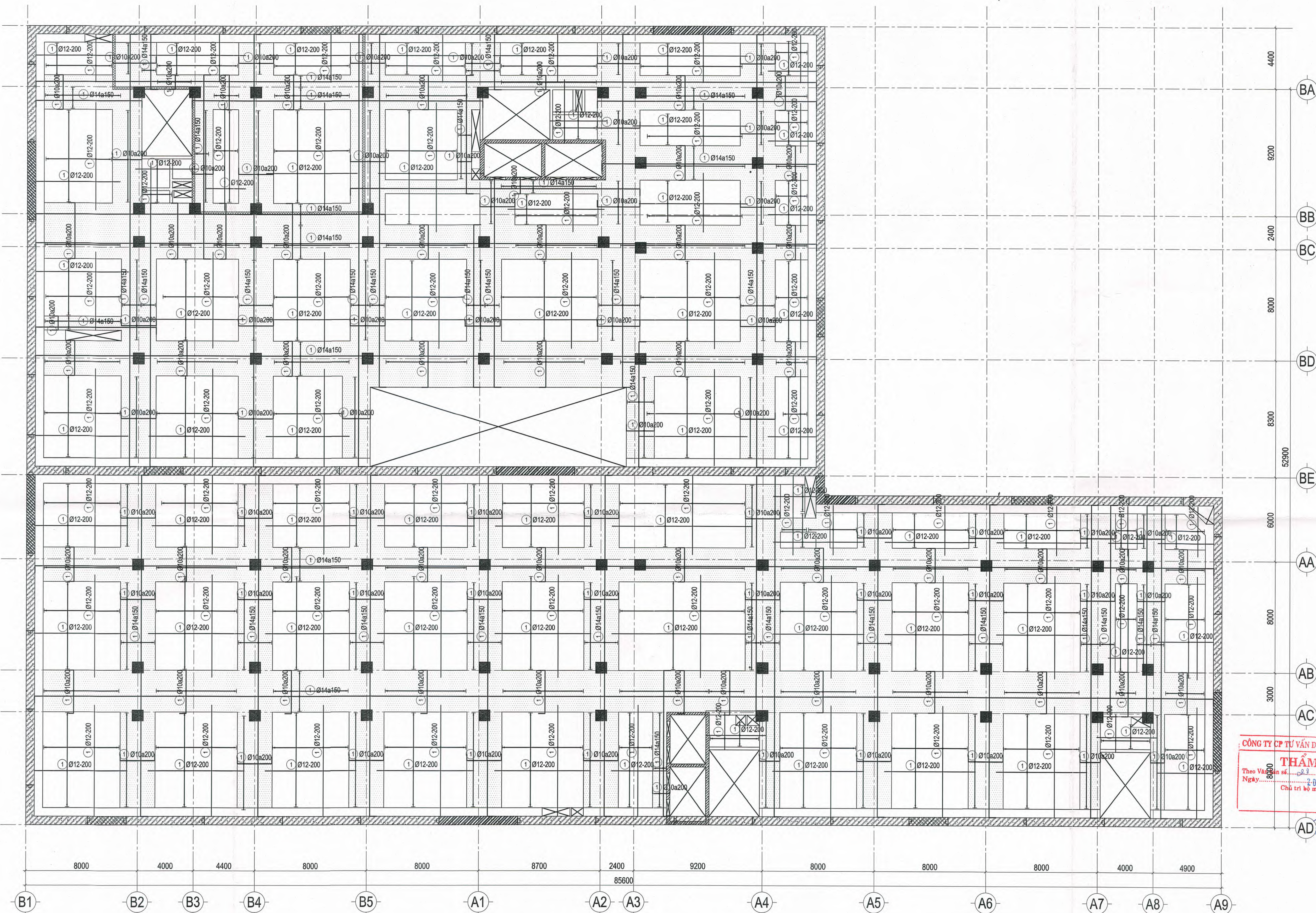
MẶT BẰNG THÉP LỚP DƯỚI SÀN HẦM 2 TL: 1/200
