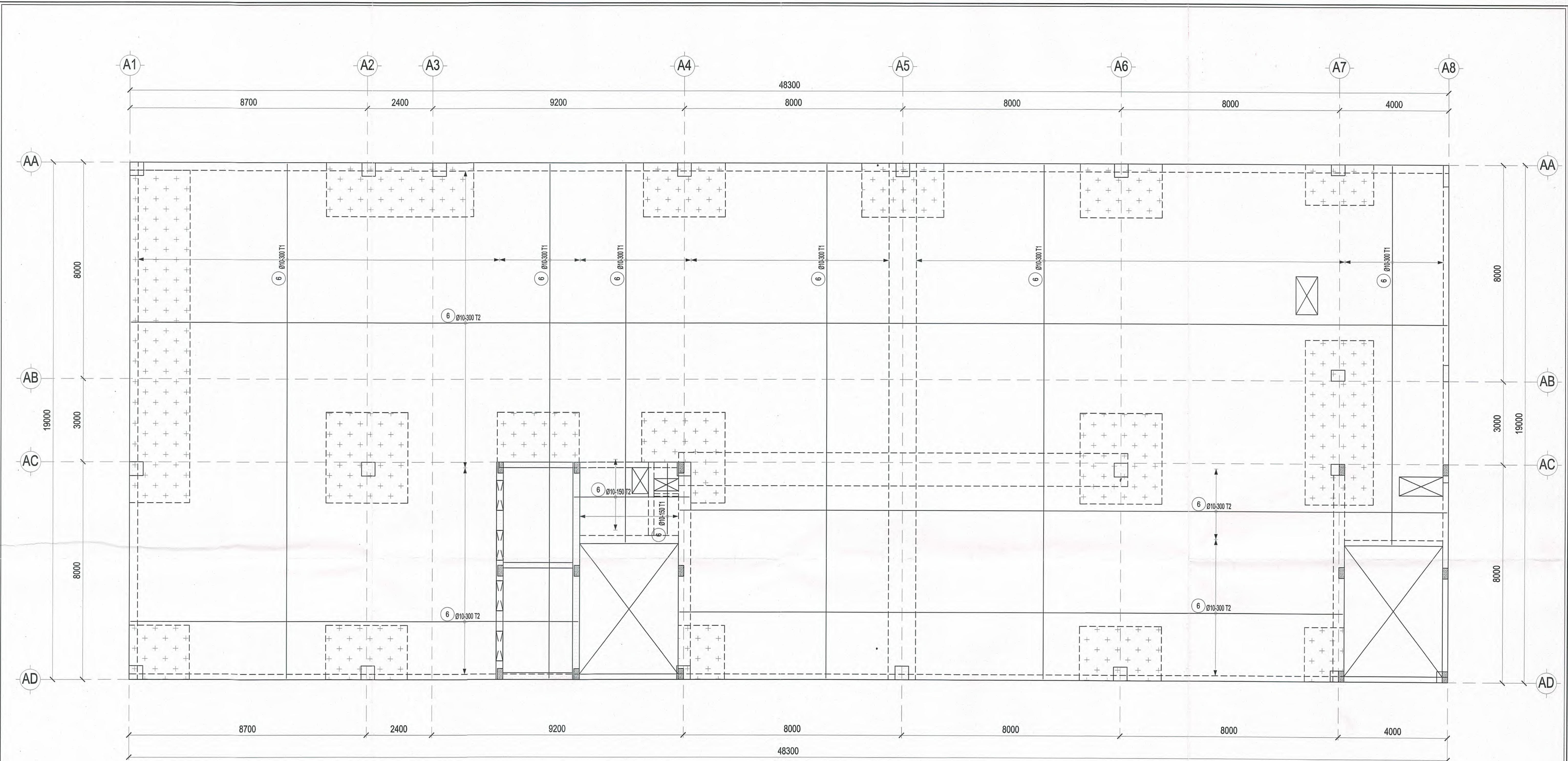
MẶT BẰNG THÉP SÀN LỚP TRÊN TẦNG TUM TL: 1/ 100
