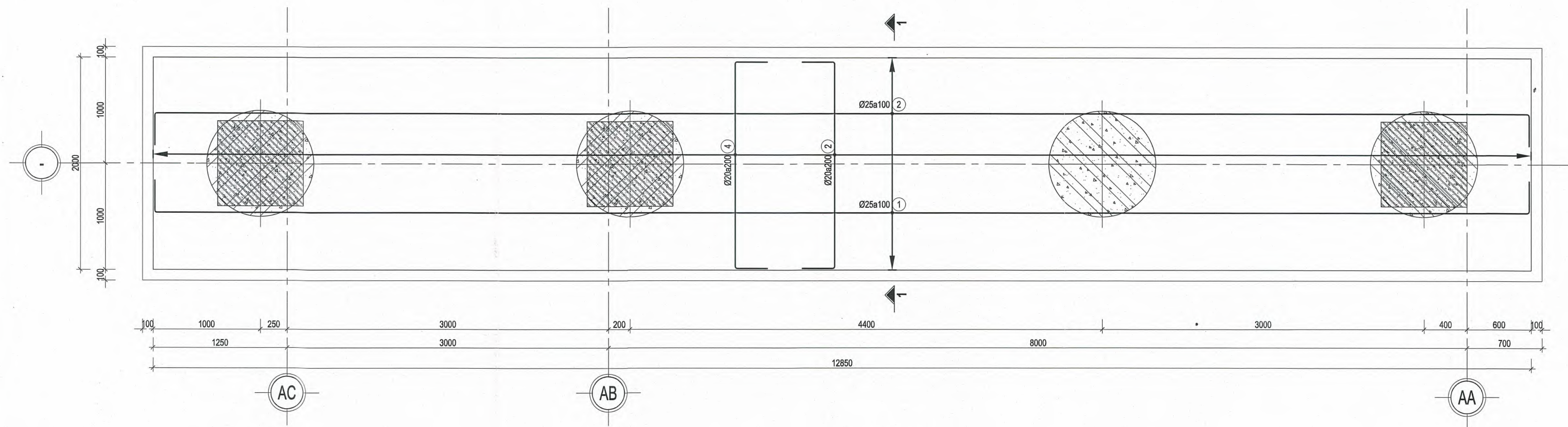
MÓNG M1-1 (SL=3) TL: 1/25
