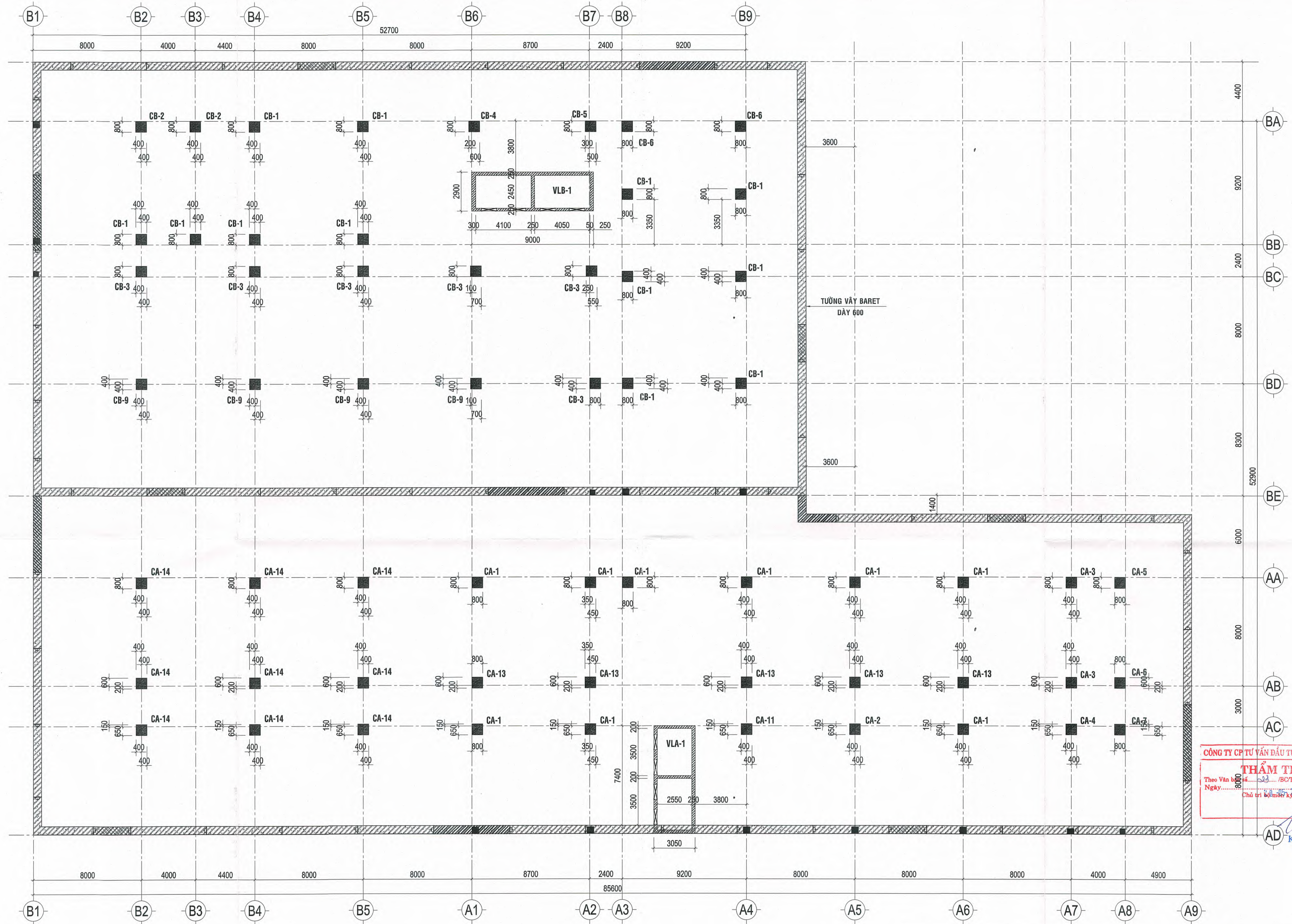
MẶT BẰNG ĐỊNH VỊ CỘT HẦM 3 -> TẦNG 1 TL: 1/100
