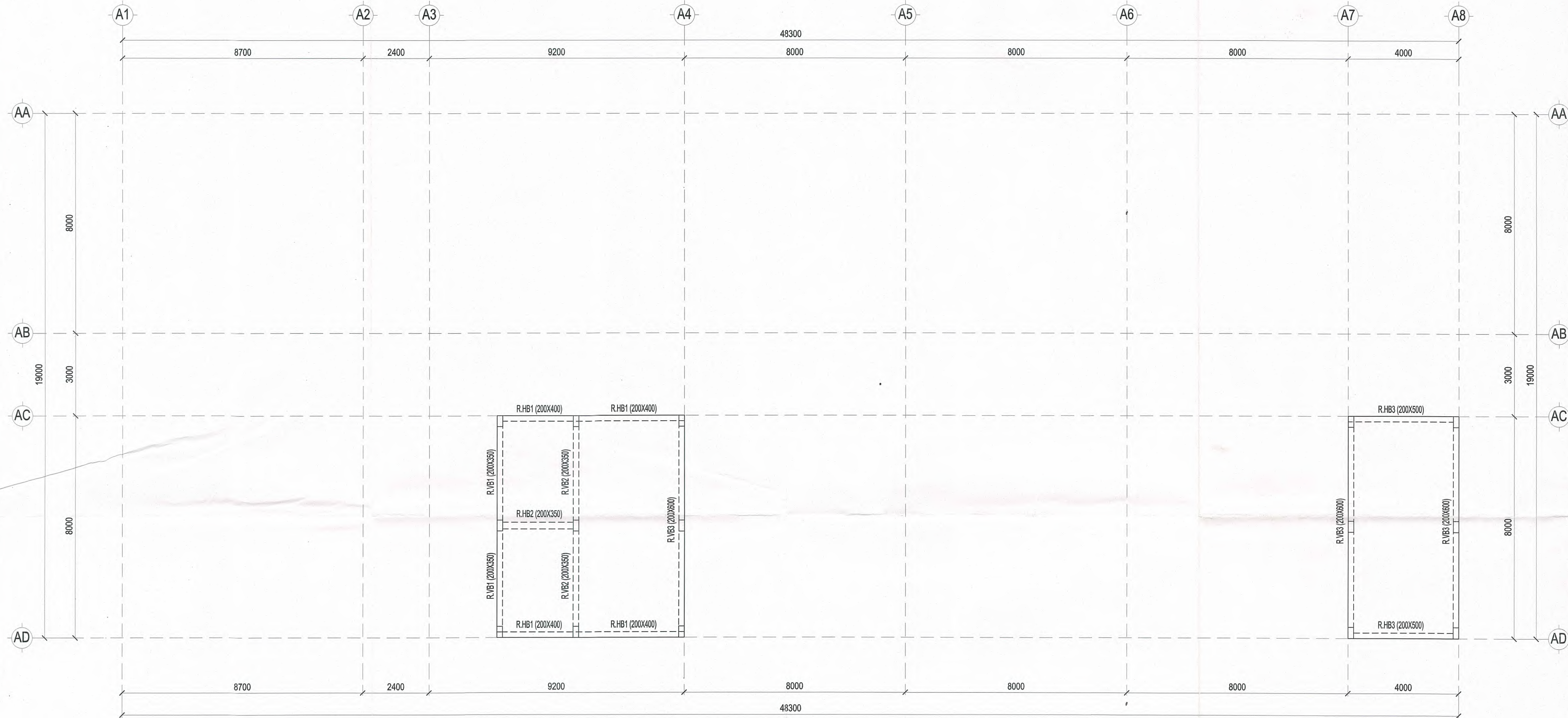
MẶT BẰNG DẦM SÀN TẦNG MÁI
