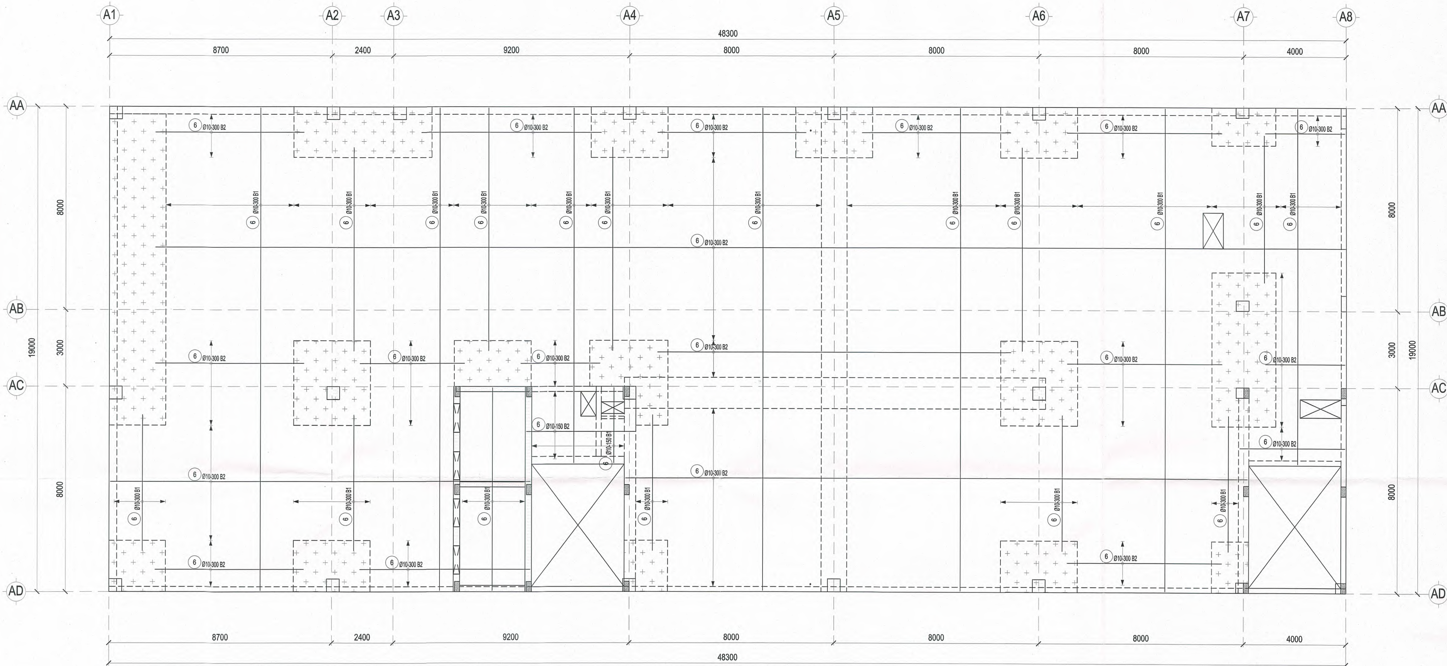
MẶT BẰNG THÉP SÀN LỚP DƯỚI TẦNG TUM TL: 1/ 100
