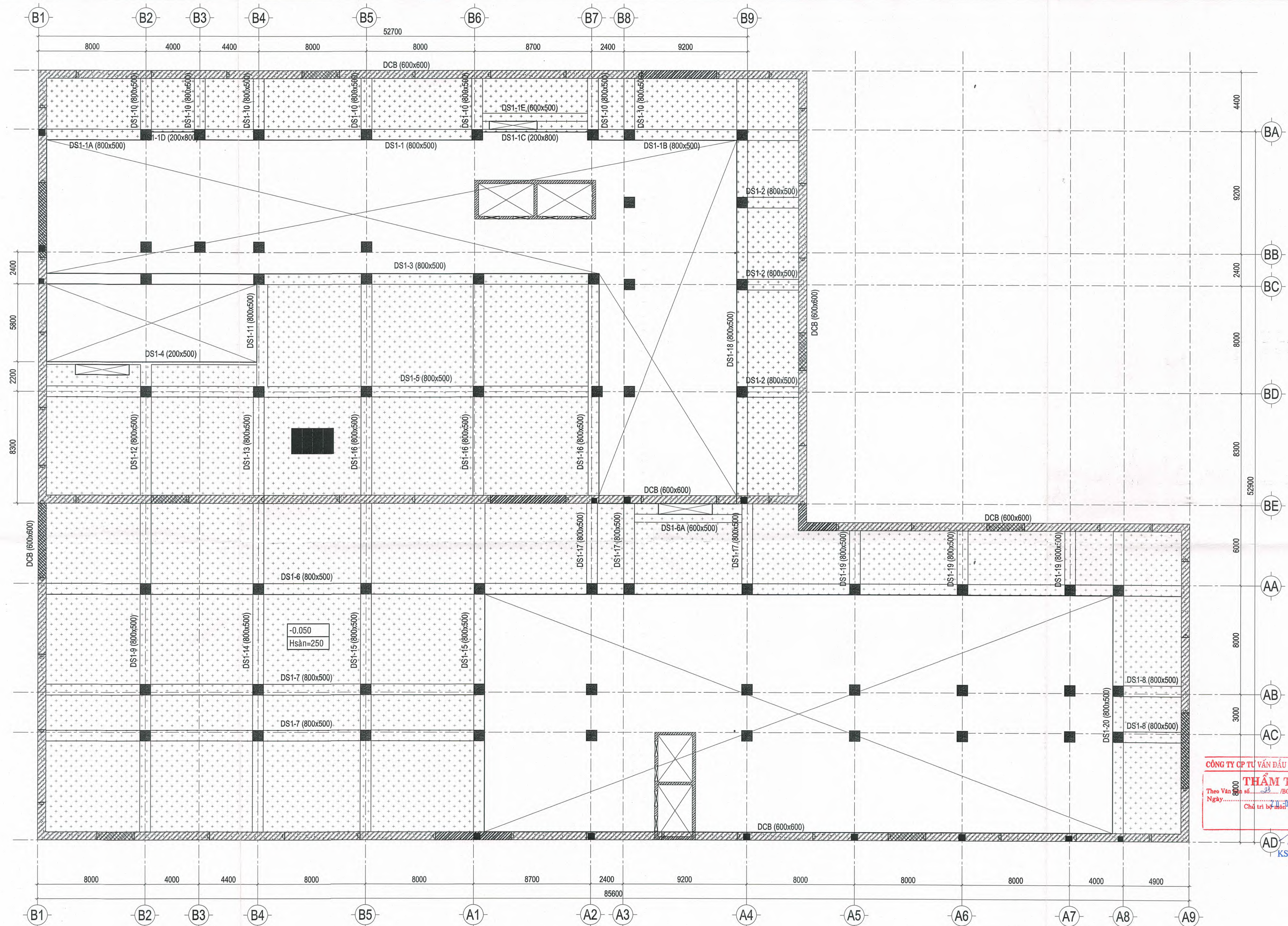
MẶT BẰNG DẦM SÀN TẦNG 1 COTE -0.050 TL: 1/200
