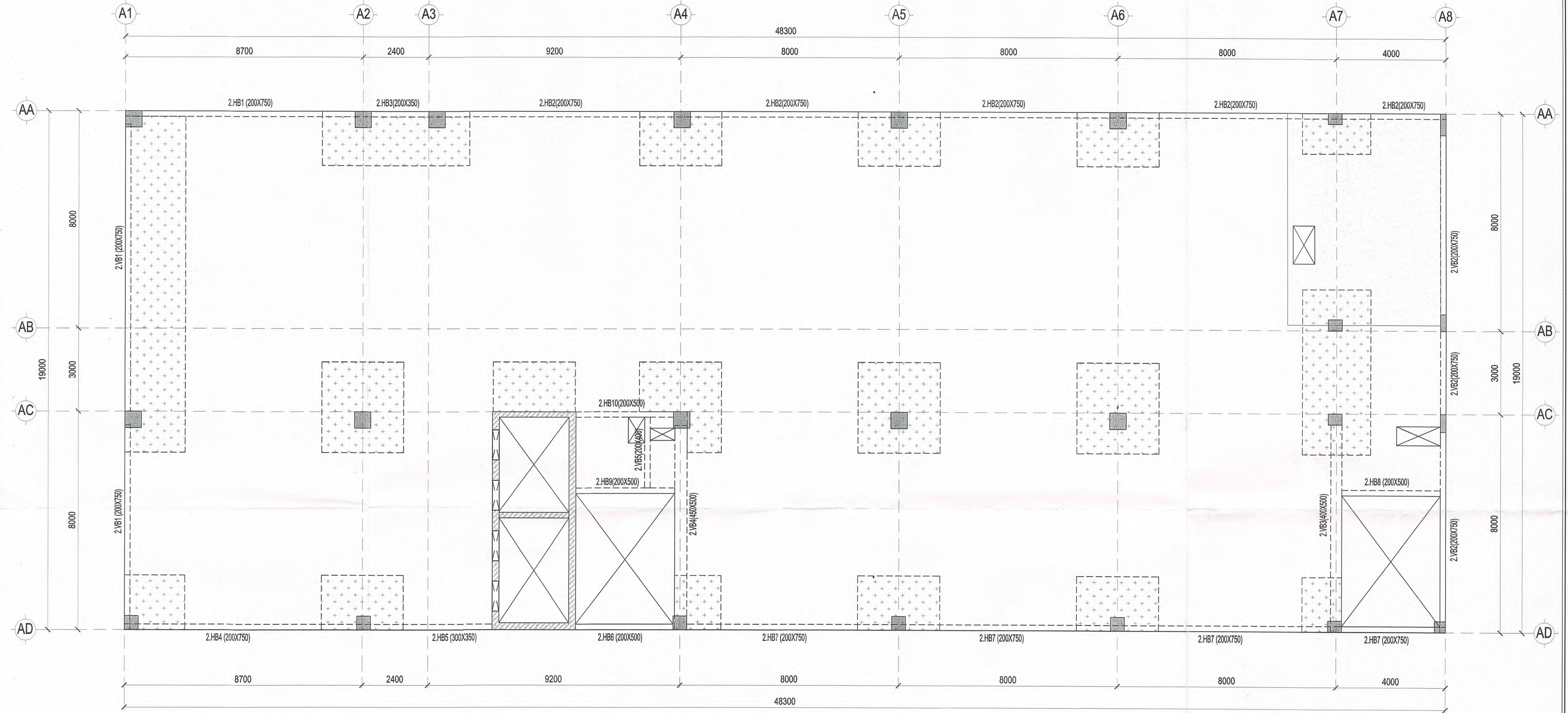
MẶT BẰNG DẦM SÀN TẦNG 2 TL: 1/ 100
