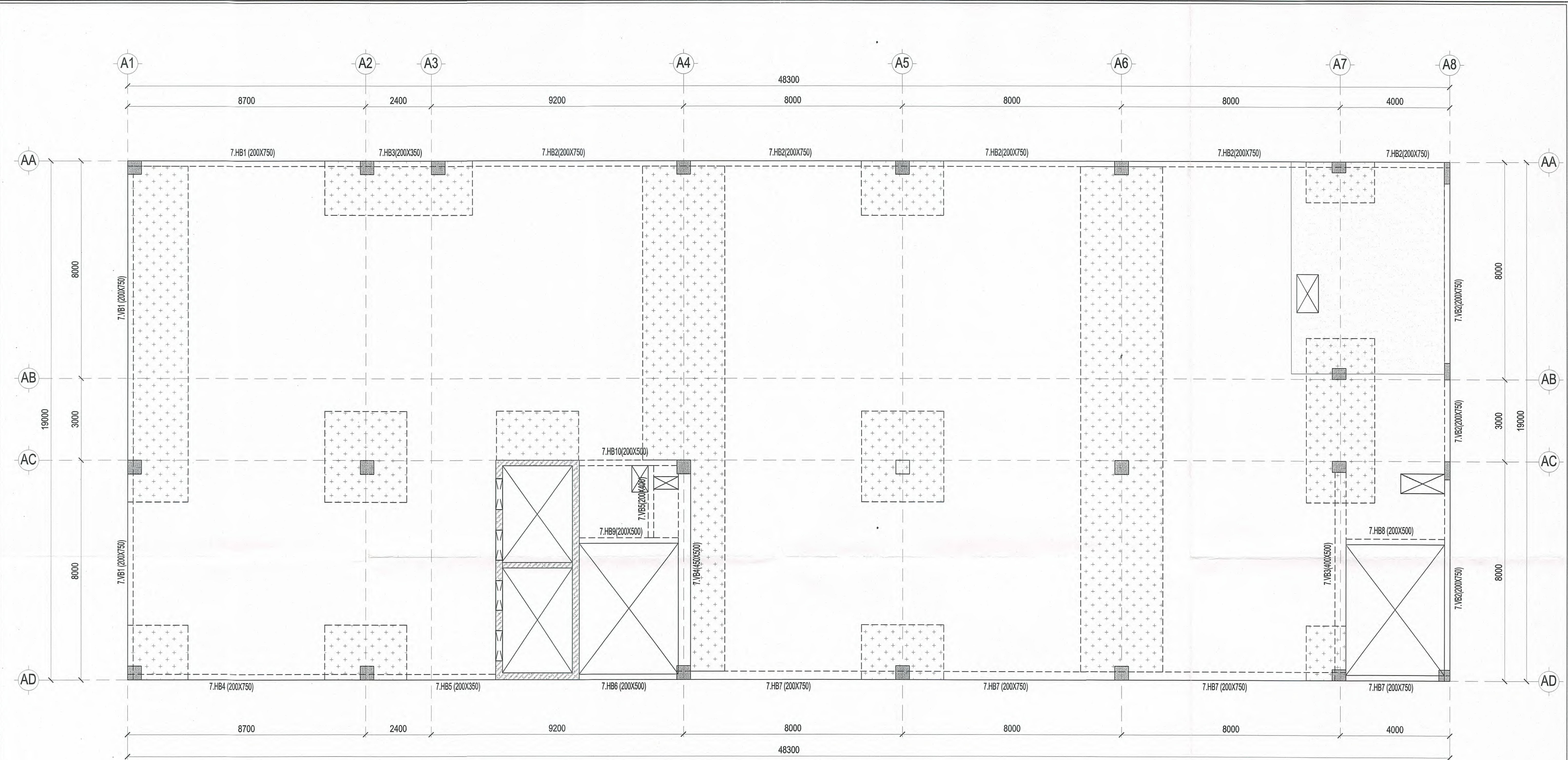
MẶT BẰNG DẦM SÀN TẦNG 7 TL: 1/ 100
