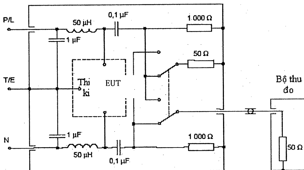
Hình 2b - Ví dụ mô phỏng mạng nguồn giả V_{50 \Omega/50 \mu H + 5 \Omega} sử dụng trong dải tần số từ 150 kHz đến 30 MHz
