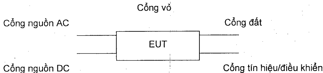
Hình 1 - Các cổng trong phép thử miễn nhiễm và phát xạ điện từ
