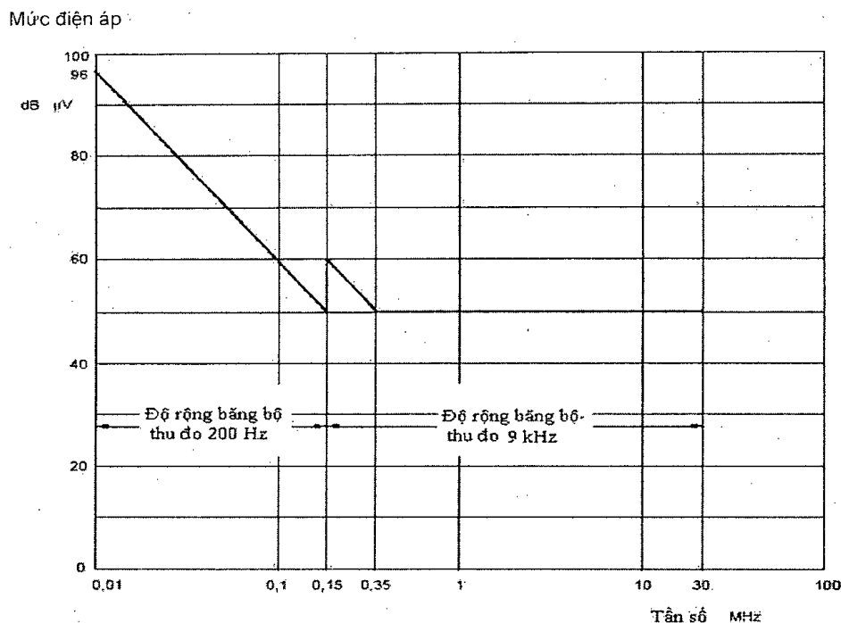
Hình 3 - Giới hạn điện áp của phát xạ dẫn tại các cực cổng nguồn
